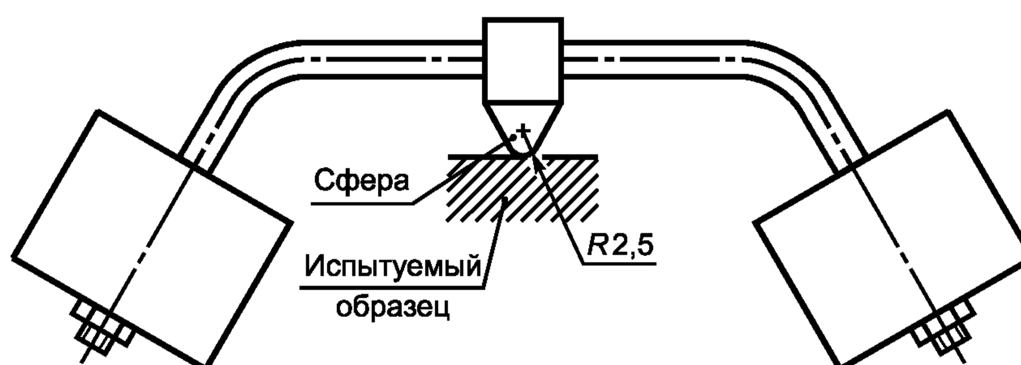
Рисунок 1 — Установка для испытания на теплостойкость
