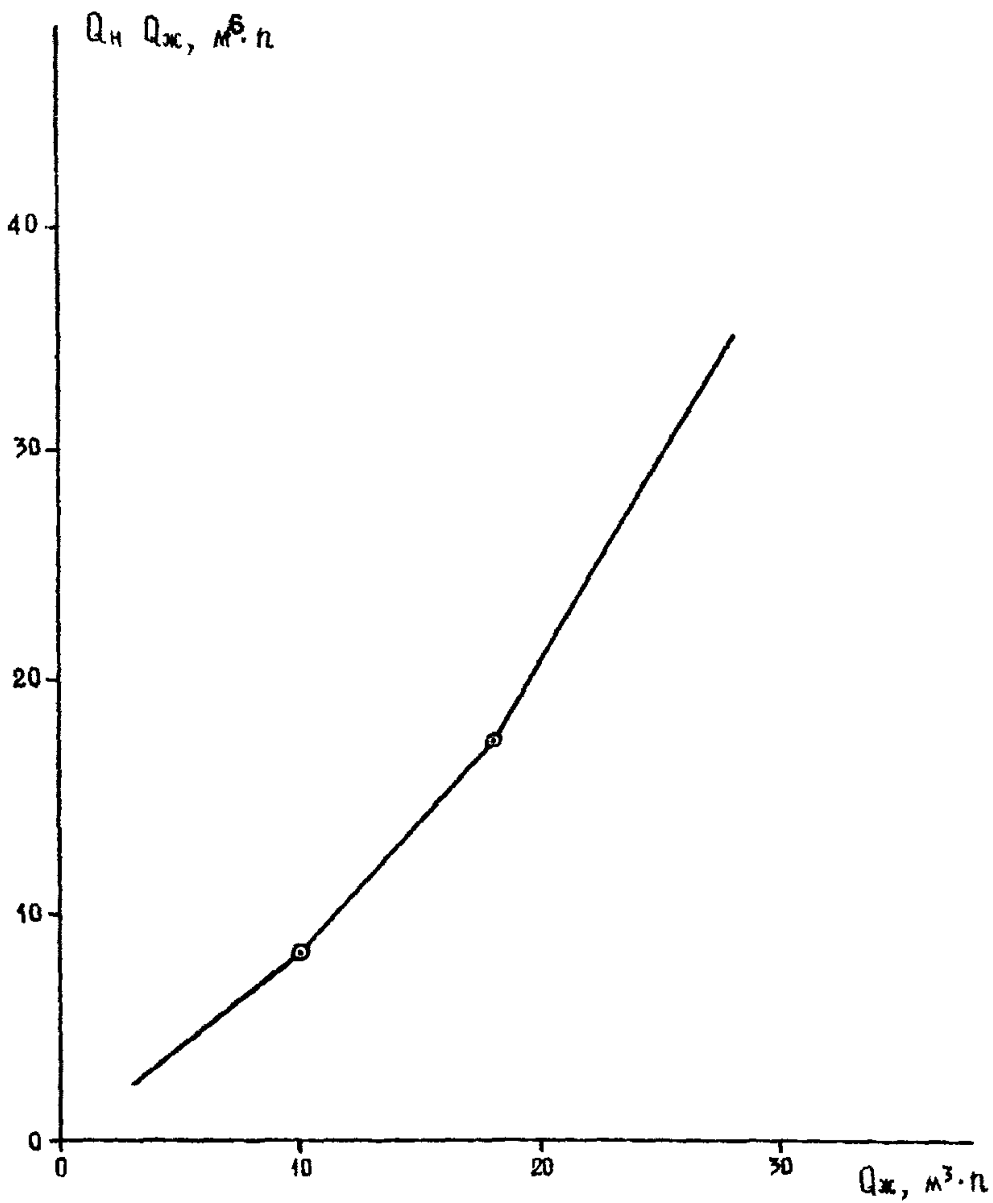
Рис.2. Характеристика вытеснения в координатах Q_{\text{н}} Q_{\text{ж}} от Q_{\text{ж}} .
