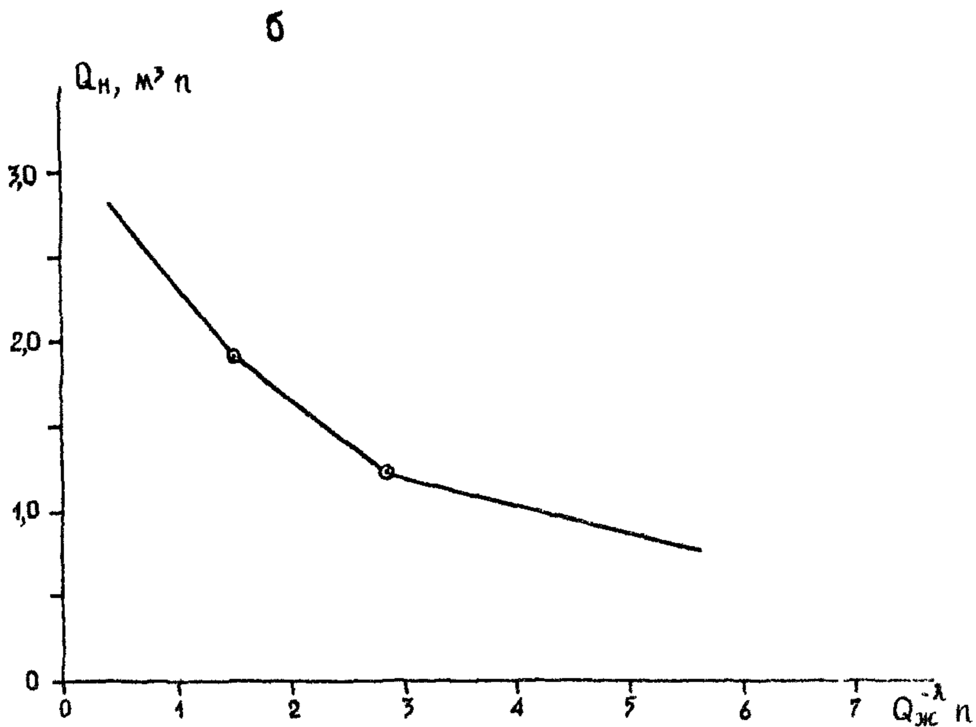
Рис. 3. Характеристика вытеснения в координатах Q_n от Q_{жс}^{-\lambda}
