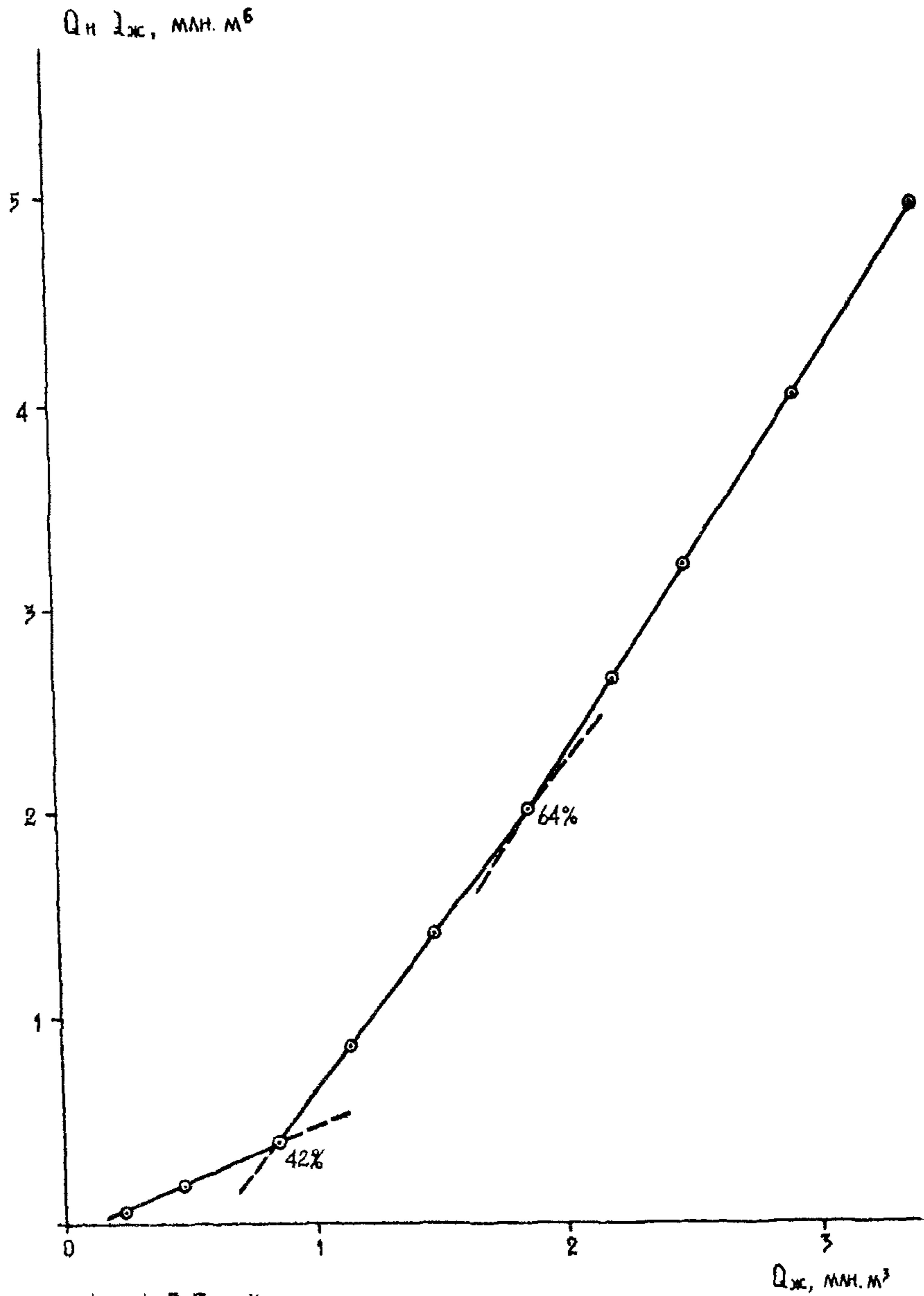
рис. II.3.3. Характеристика вытеснения по гипотетической залежи нефти в координатах Q_n \cdot Q_{ж} от Q_{ж}
