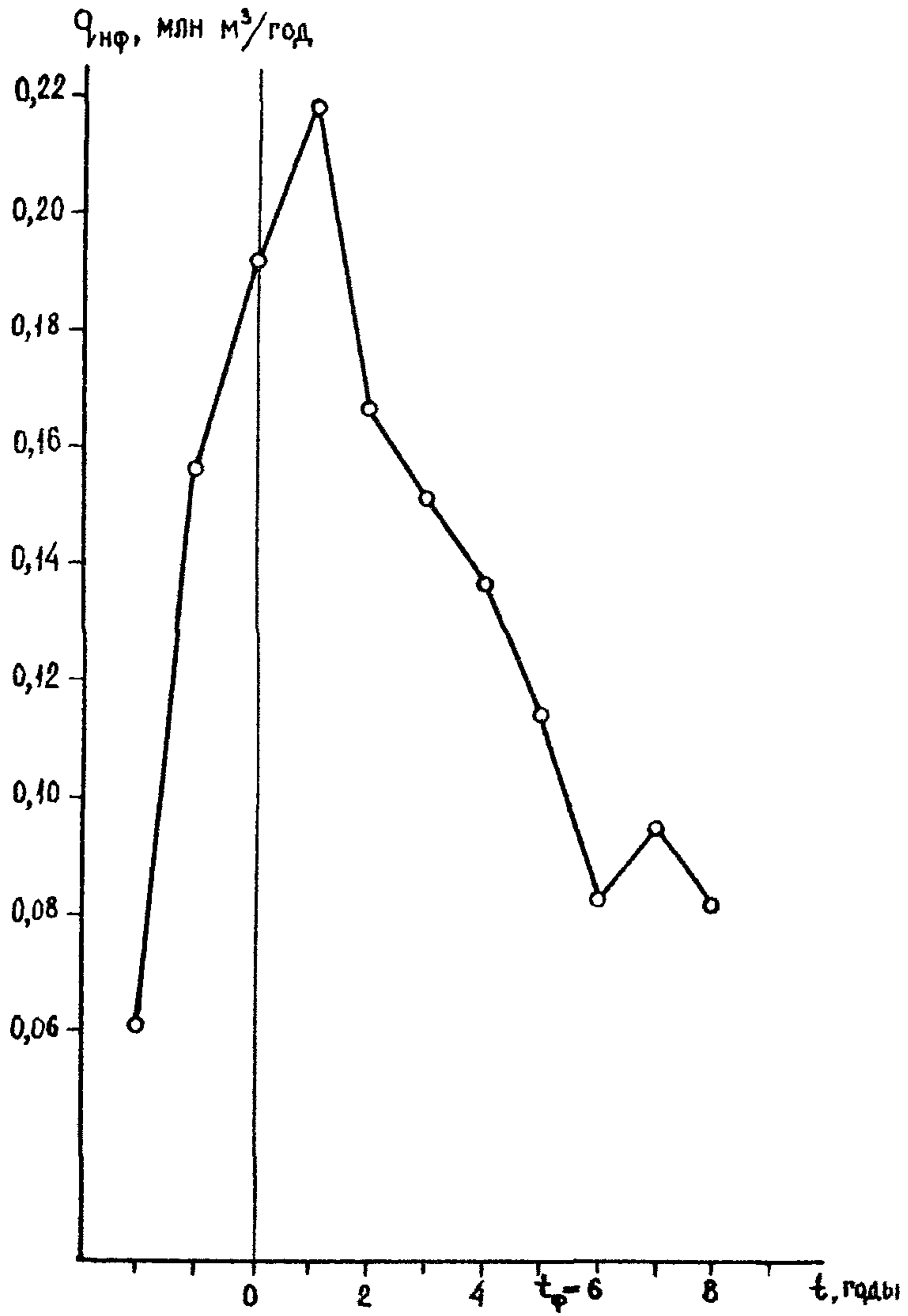
Рис. П.3.2. Сравнительное изменение годовых отборов негтя из гипотетической залежи во времени.
