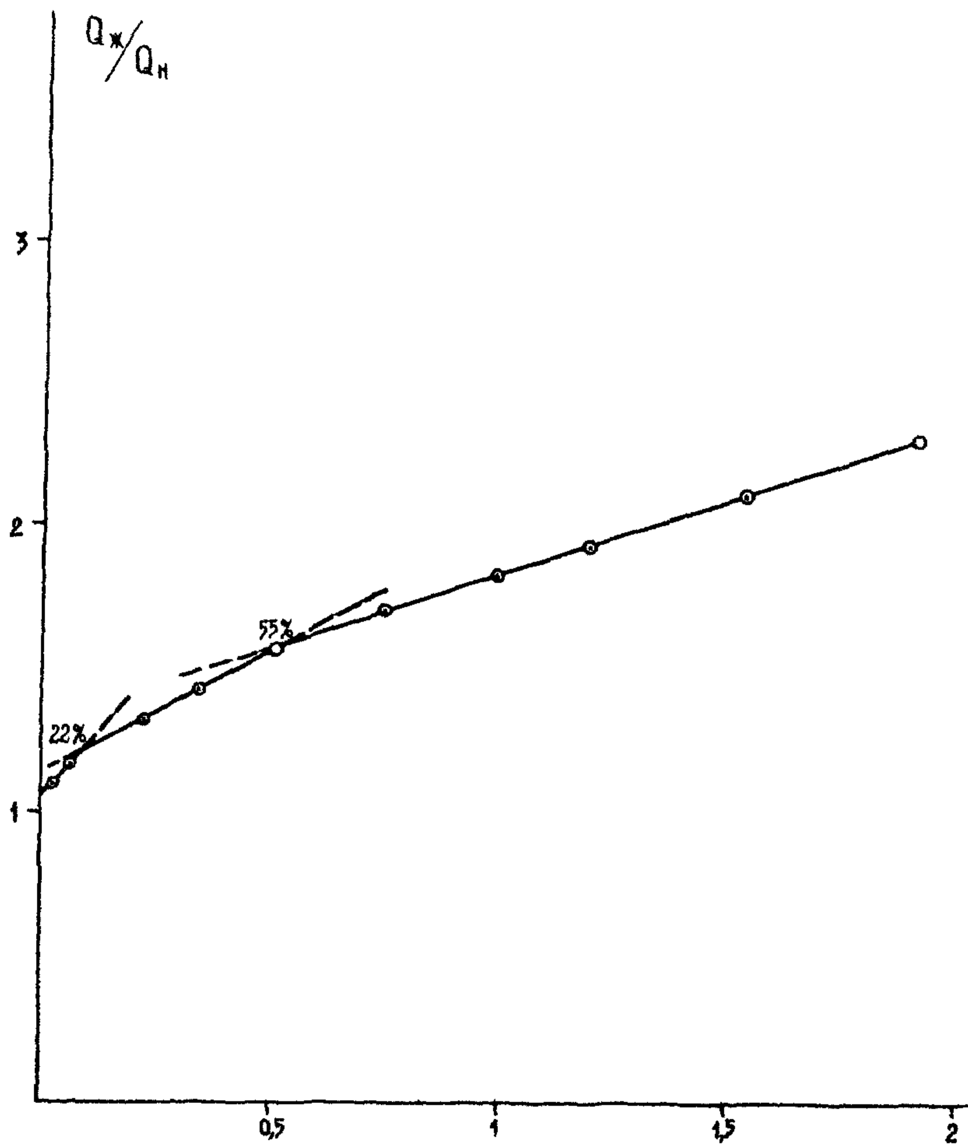
Рис. П.3.1. Характеристика вытеснения по гипотетической залежи в координатах Q_{ж}/Q_{н} от Q_{б}
