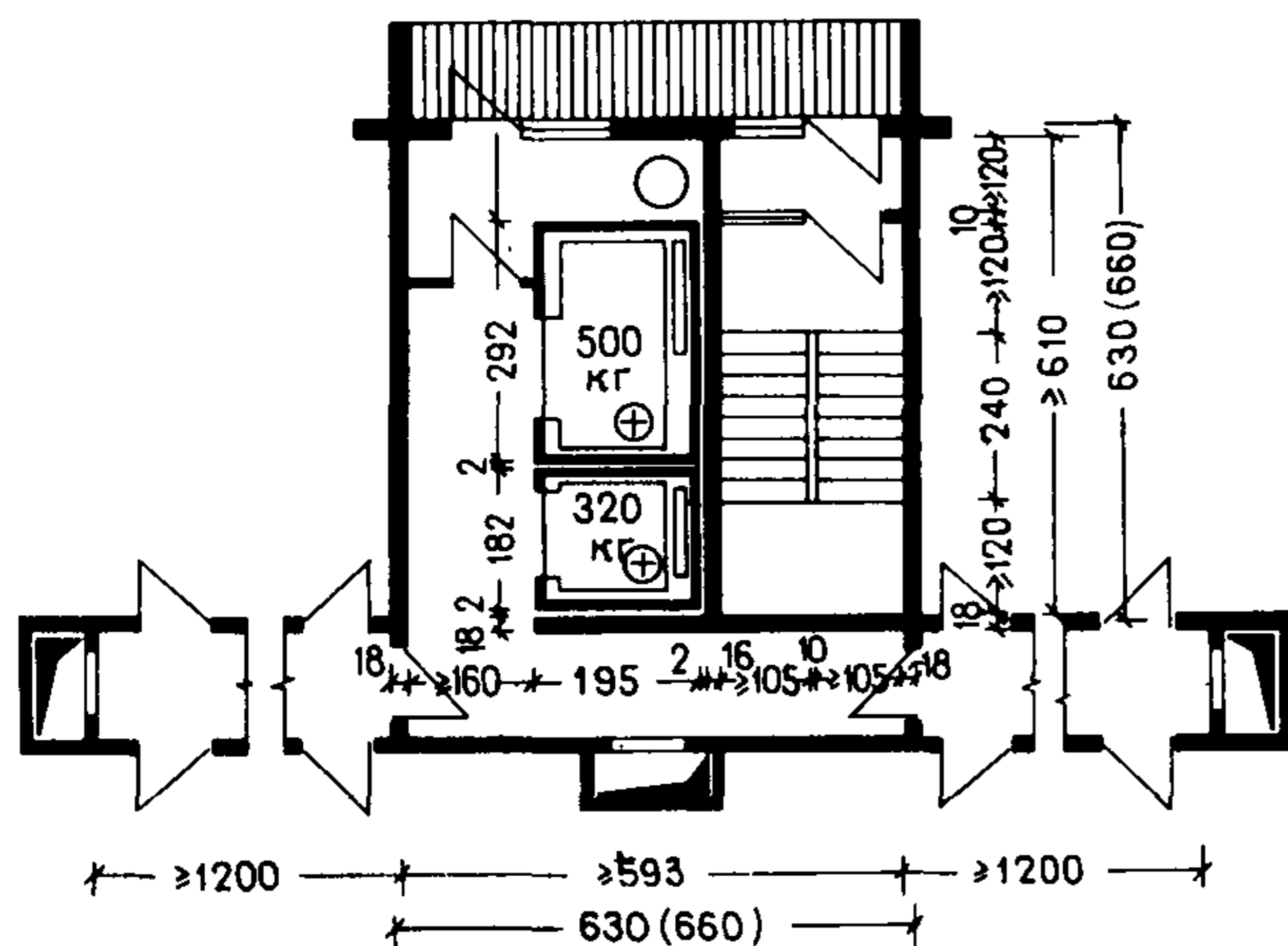
Типовой этаж
