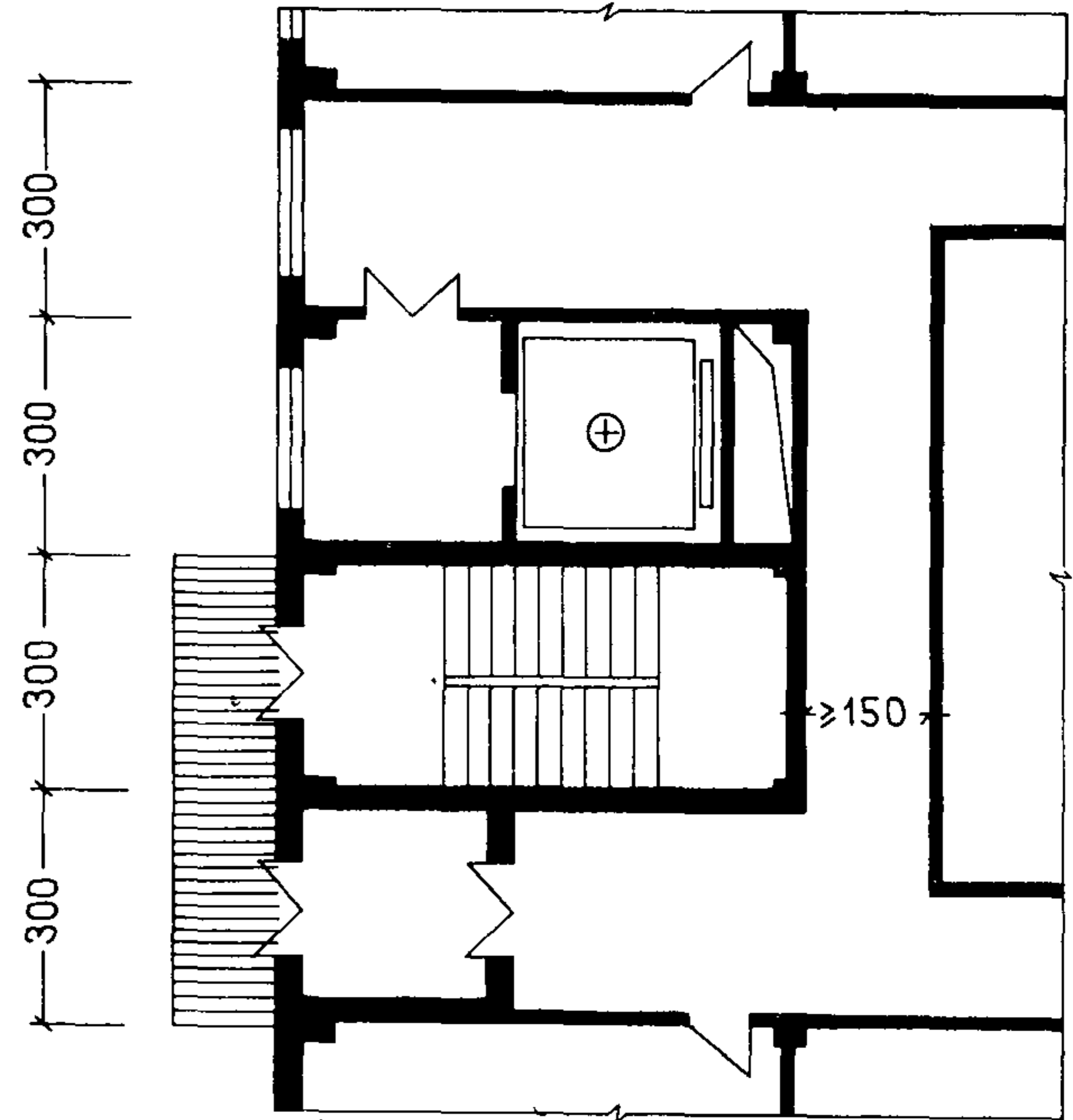
Типовой этаж
