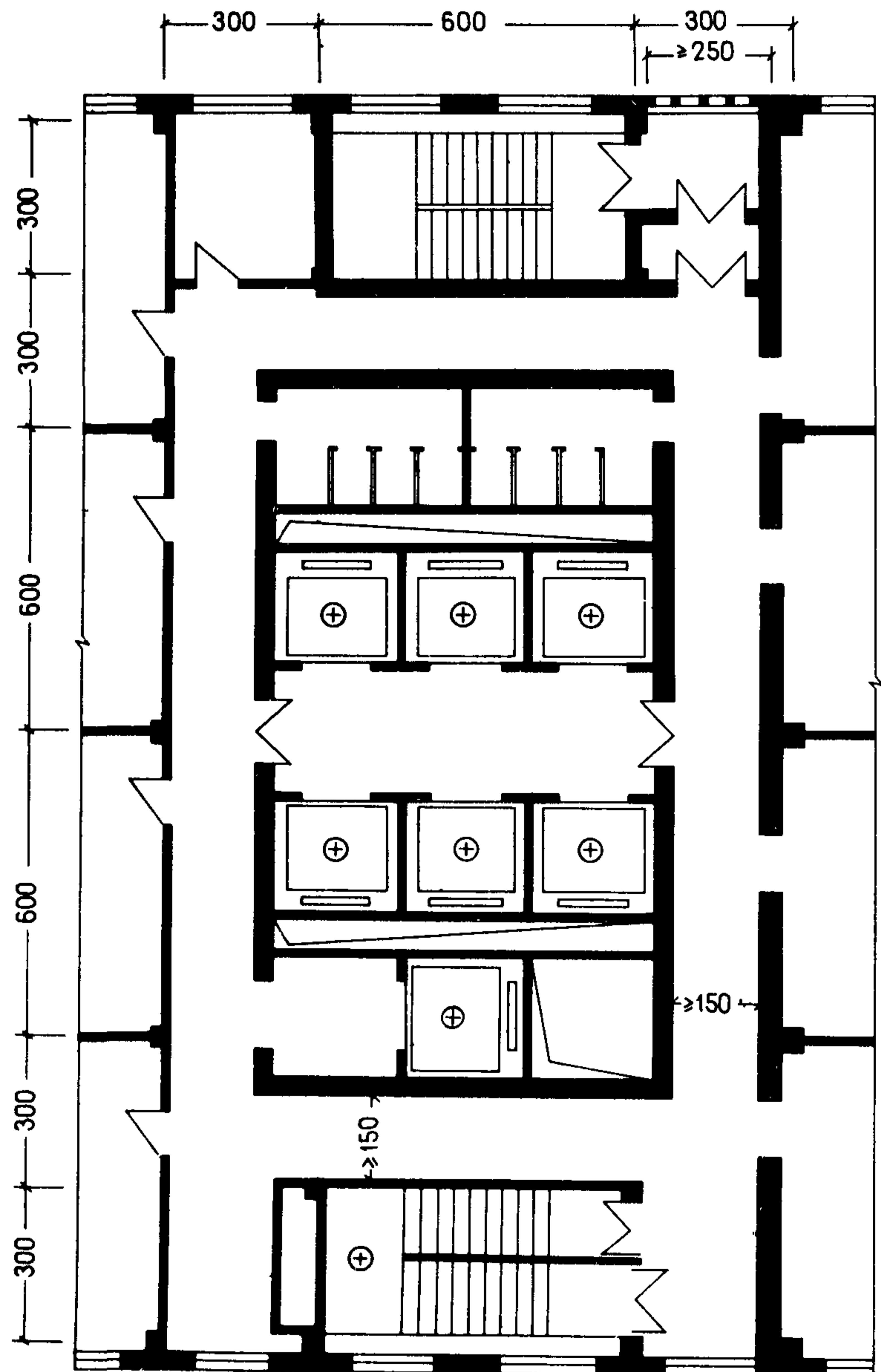
Пример планировки лестнично-лифтового узла
