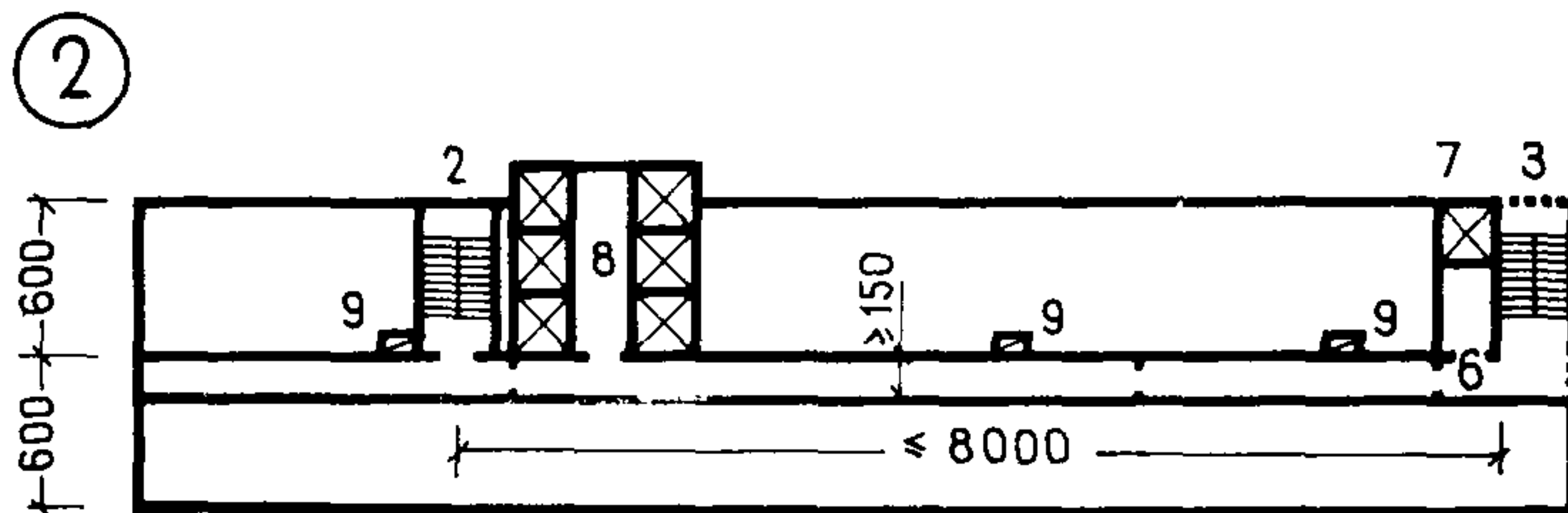
Протяженная трехпролетная схема с одним коридором
