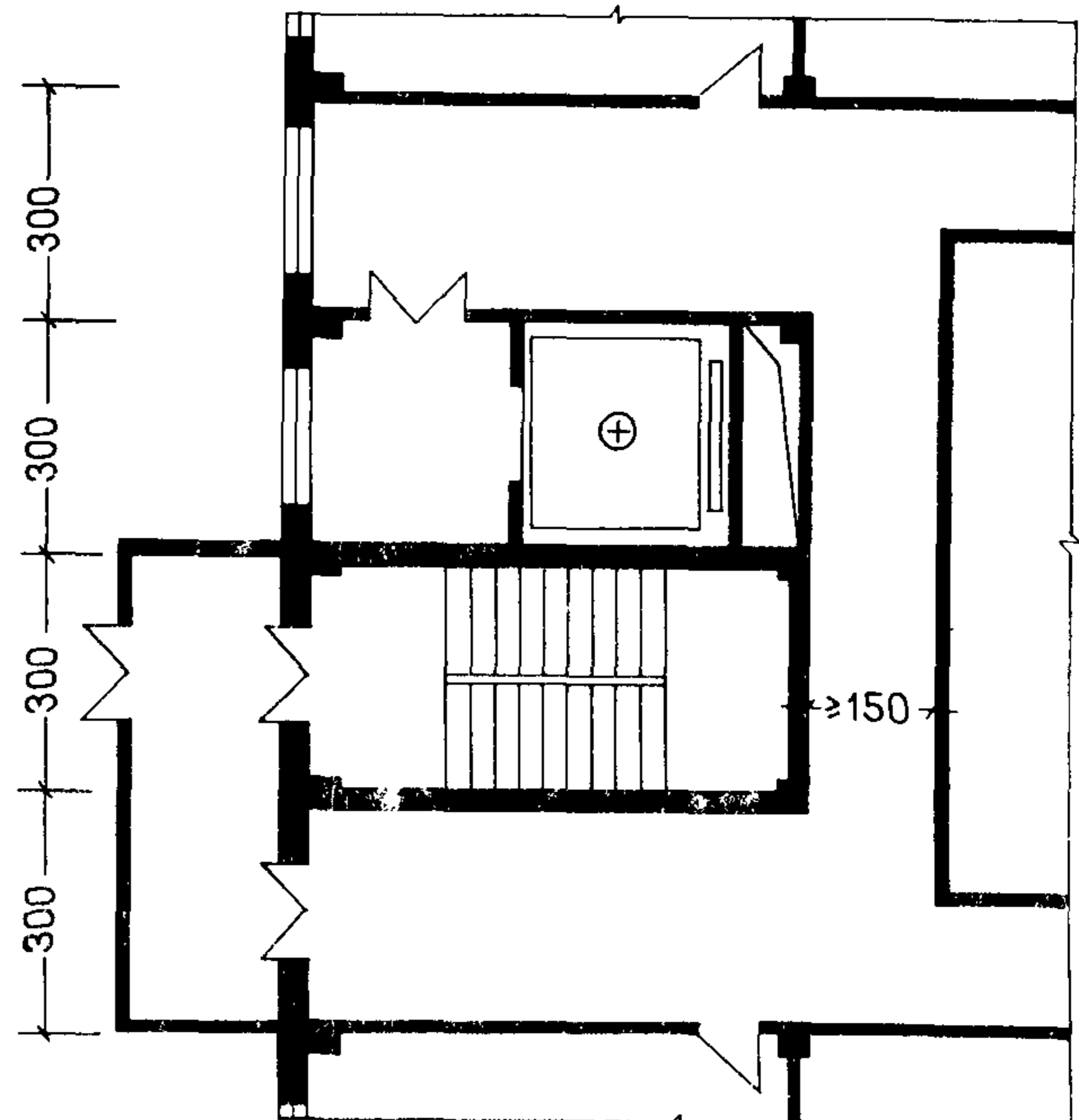
Первый этаж
