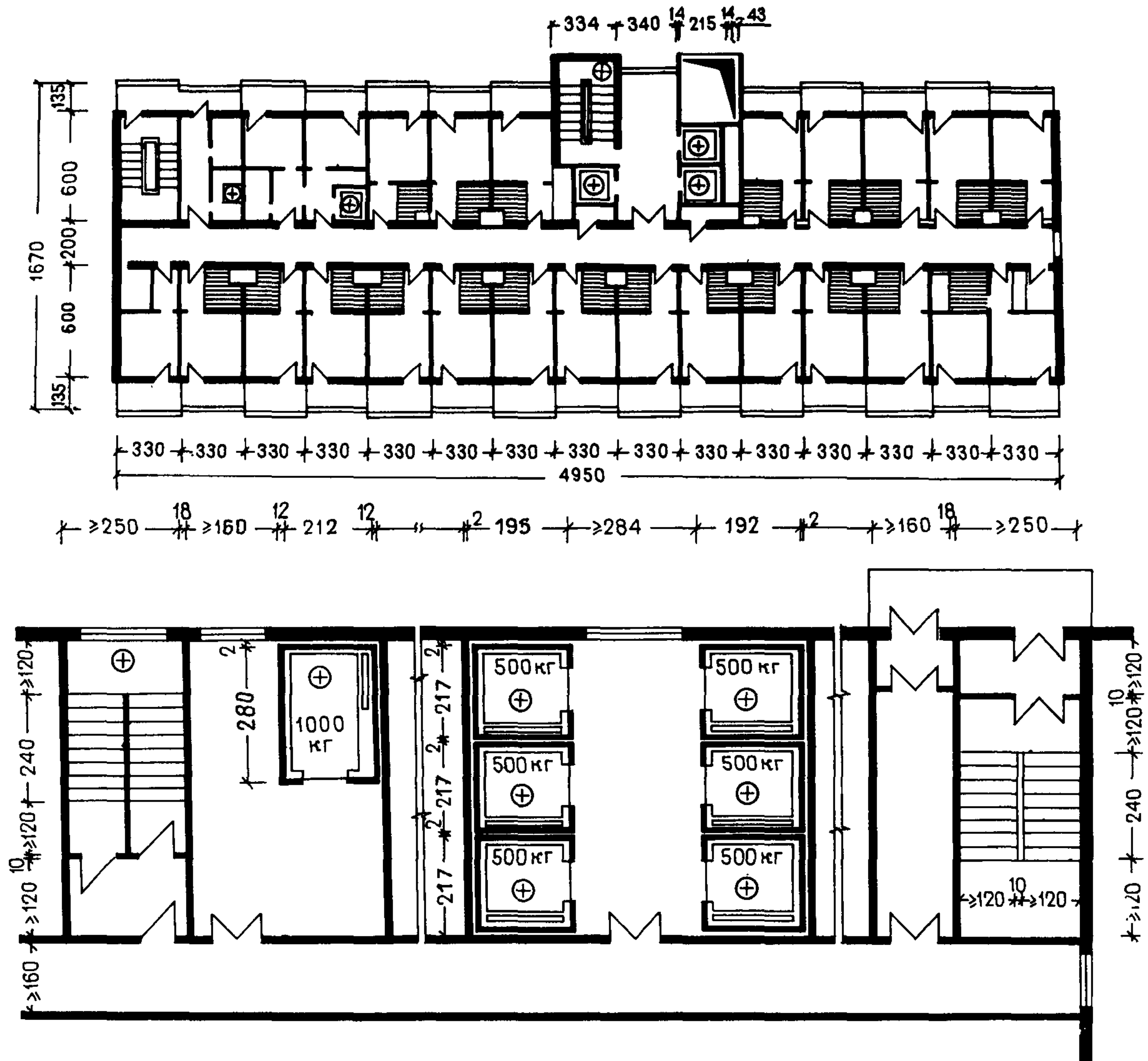
Примеры планировки этажа с двумя незадымляемыми лестницами
