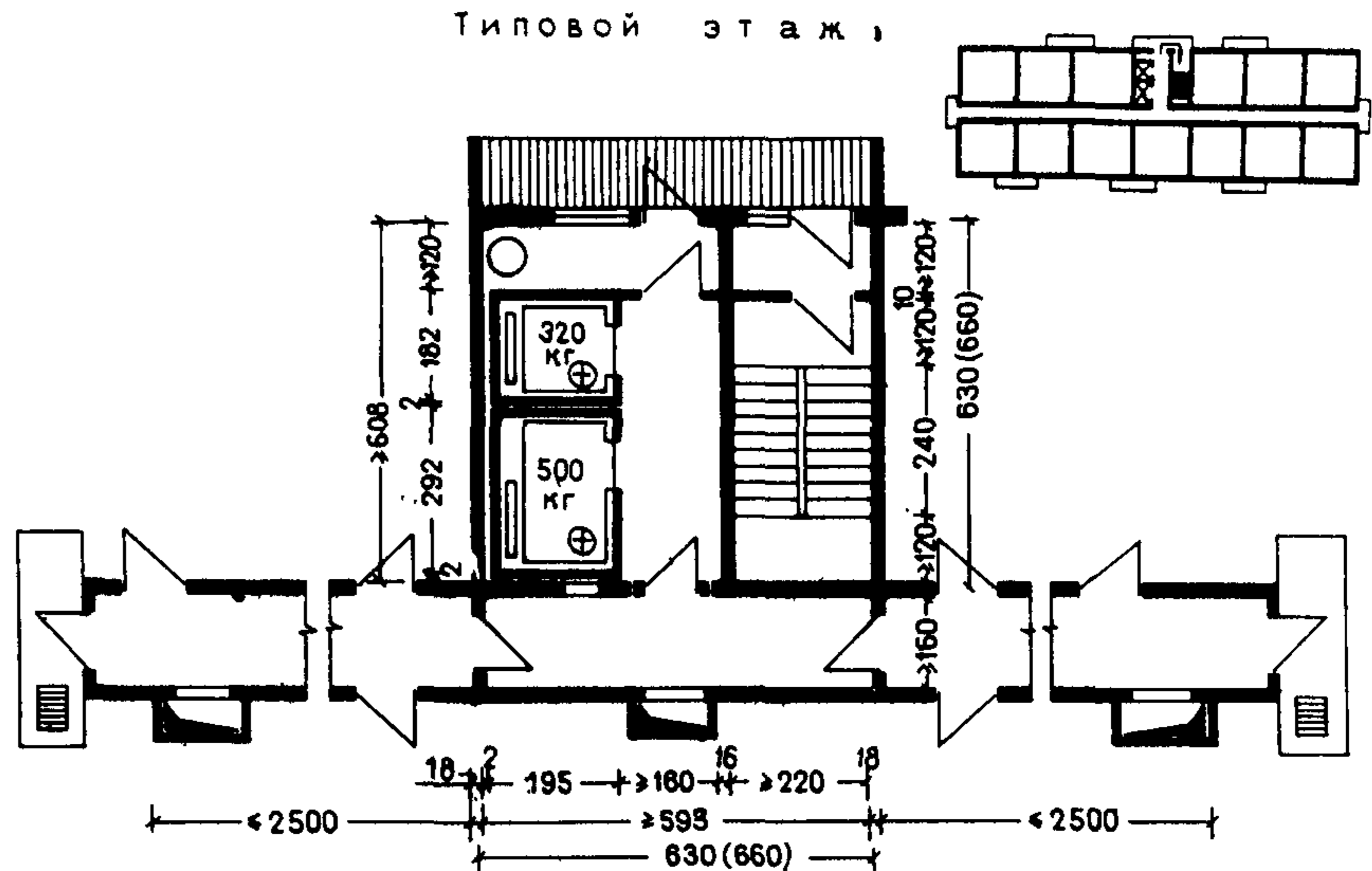
Незадымляемые лестницы с проходом через наружную зону
