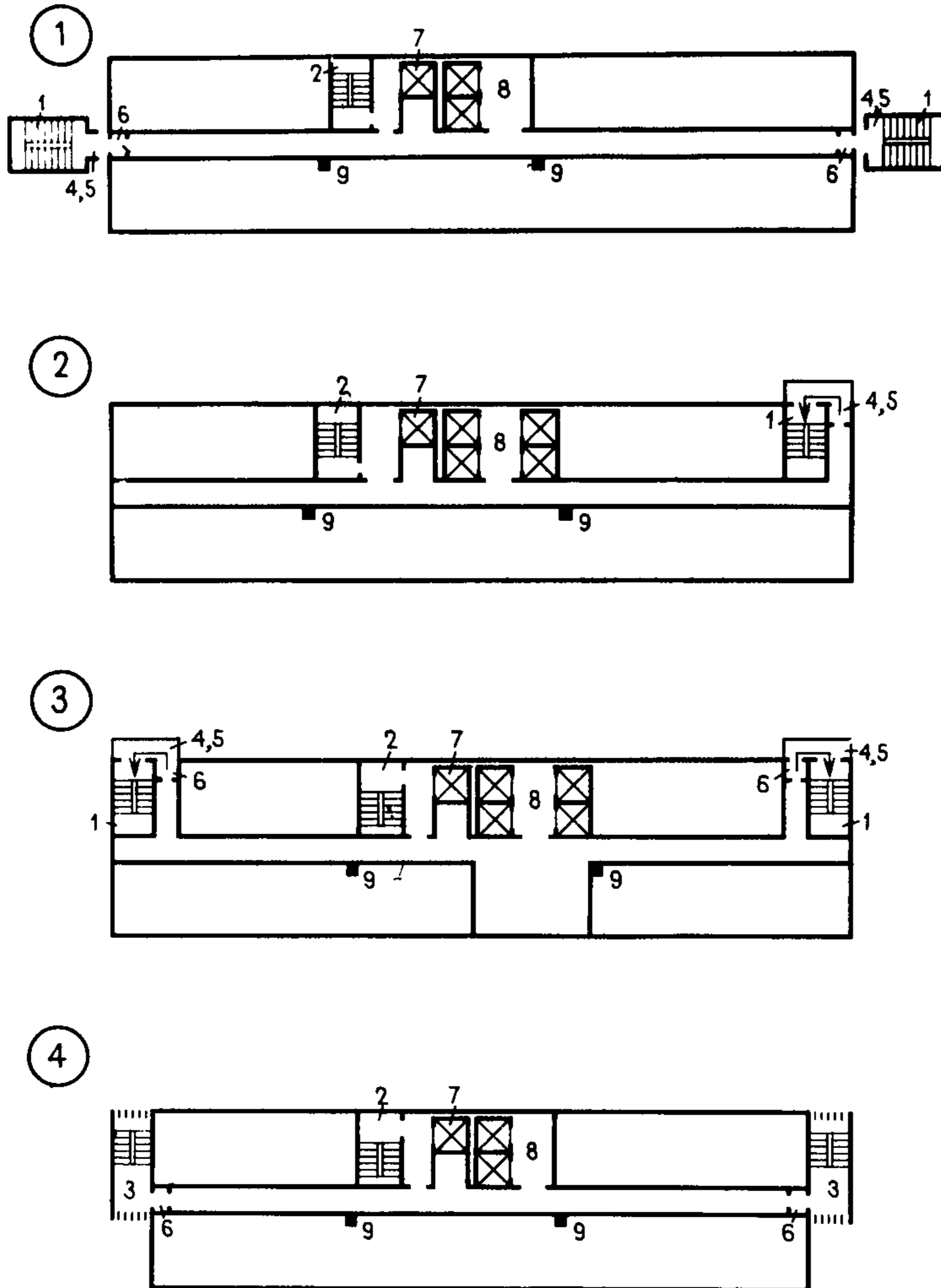
Схемы планировочных решений Пути эвакуации
