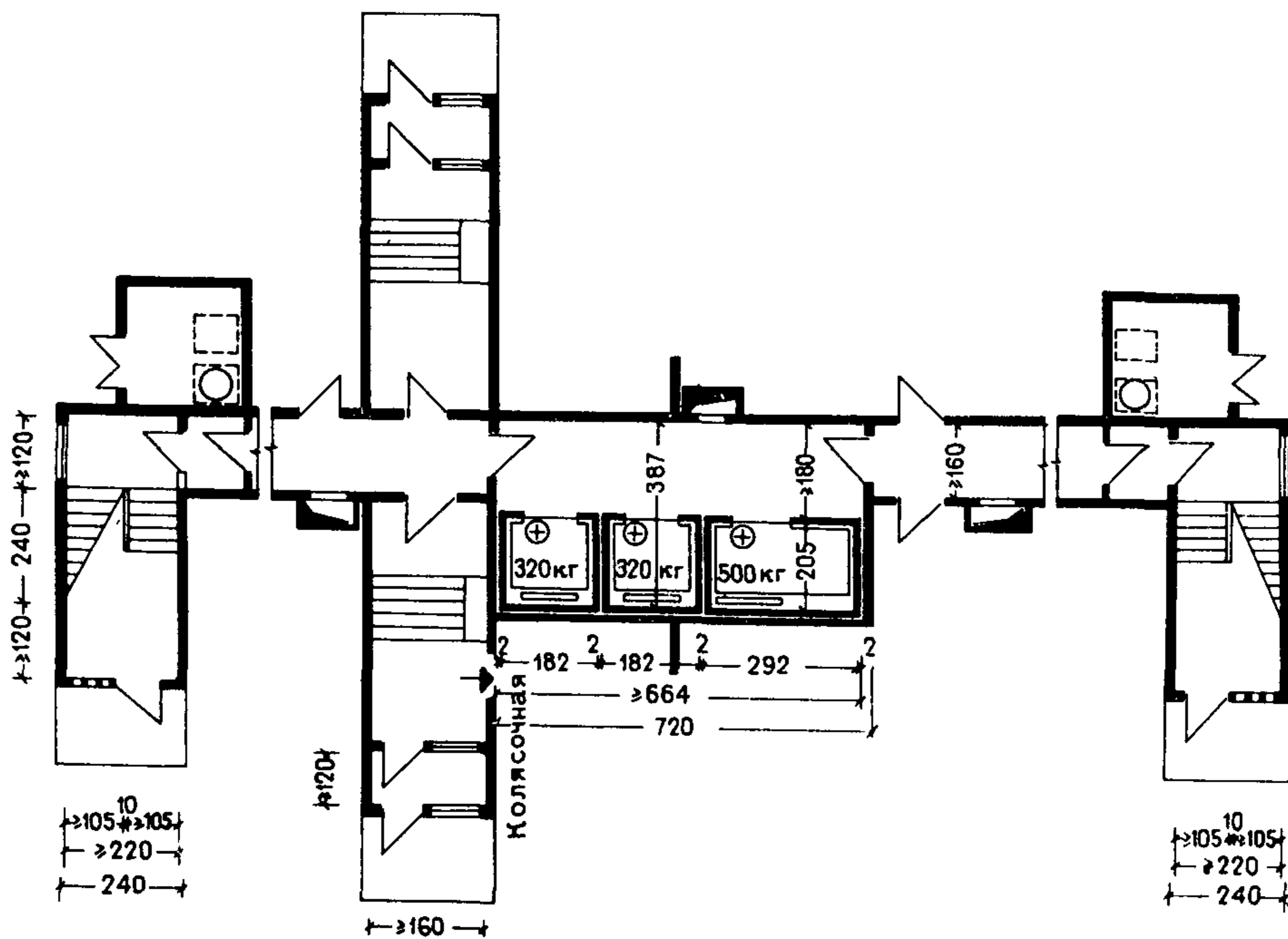
Первый этаж
