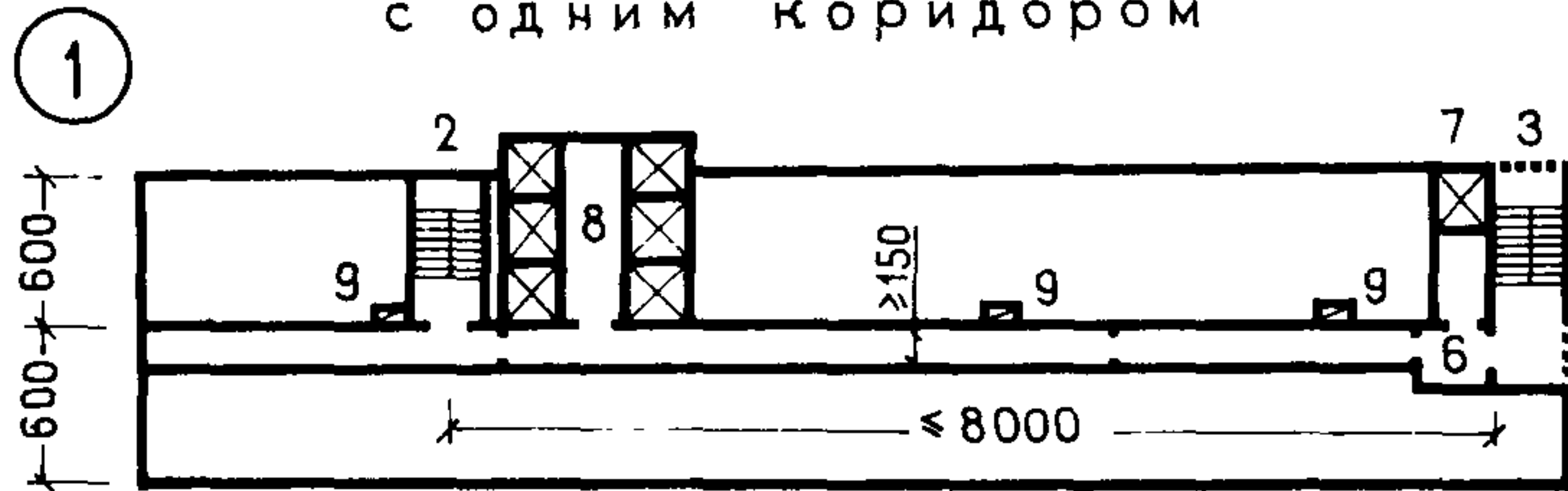
Протяженная двухпролетная схема с одним коридором
