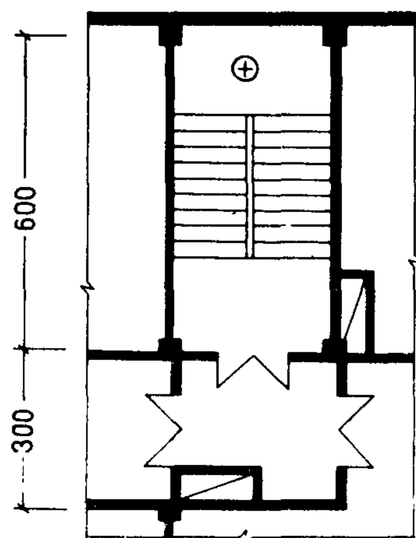
Первый этаж
