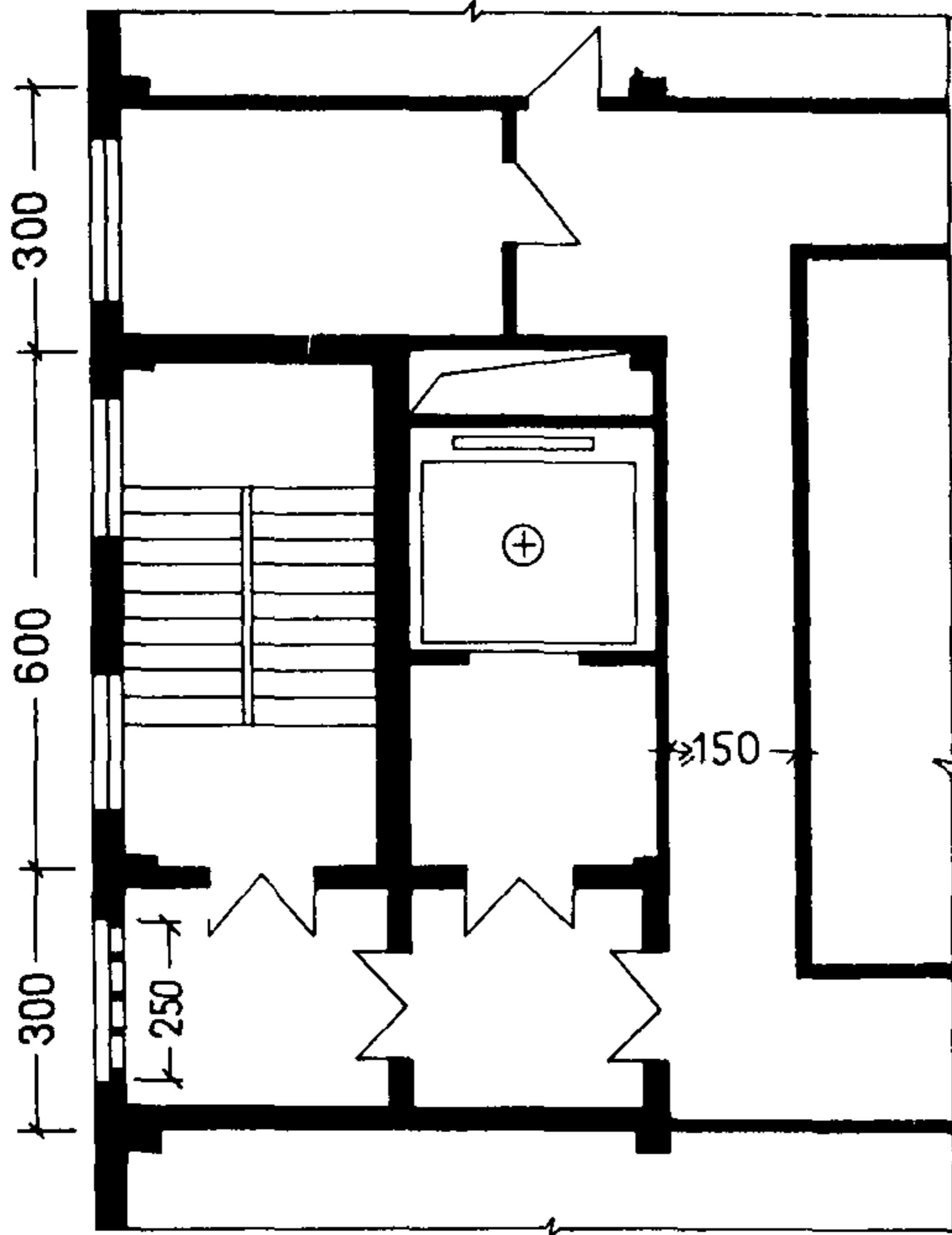
Первый этаж
