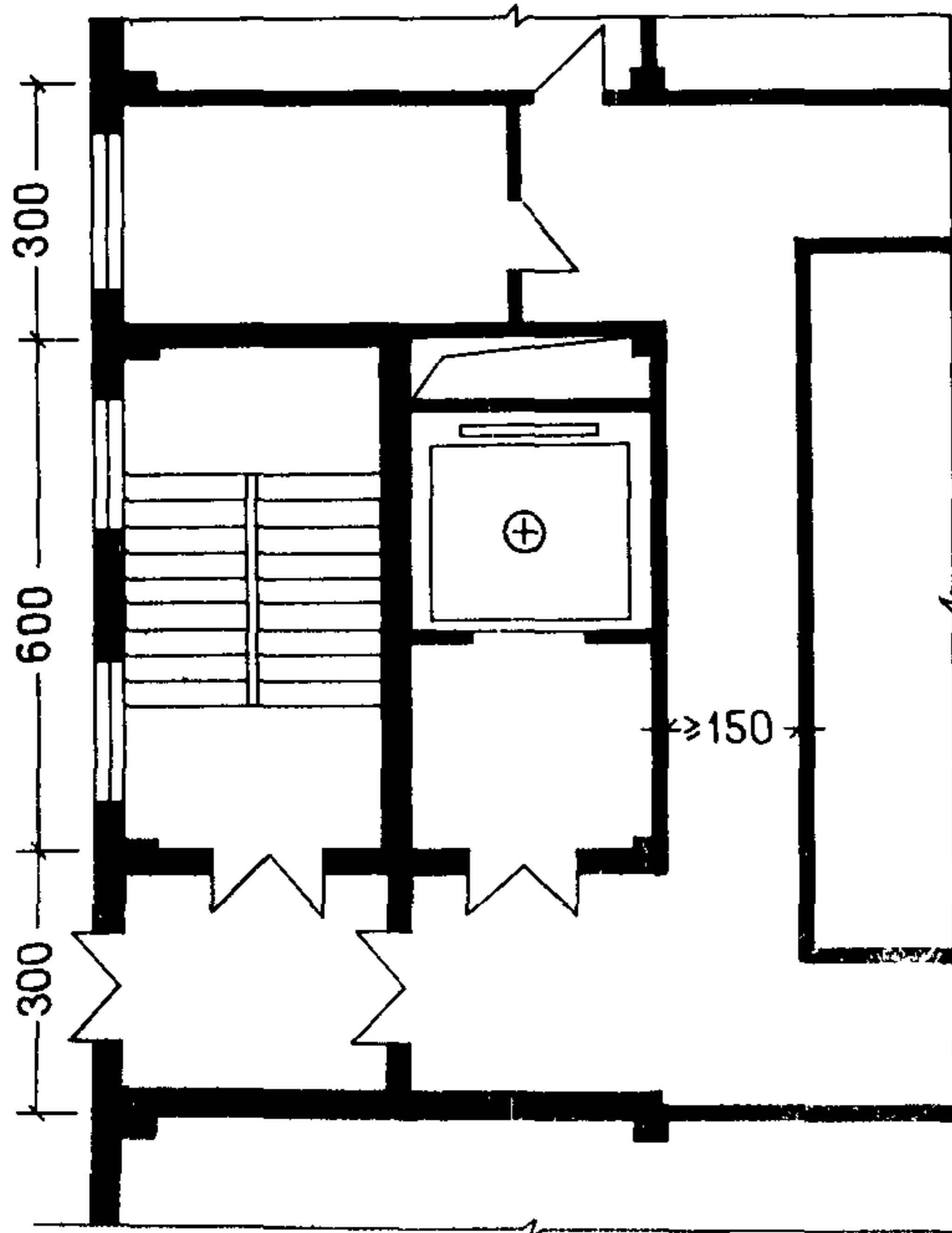
Первый этаж
