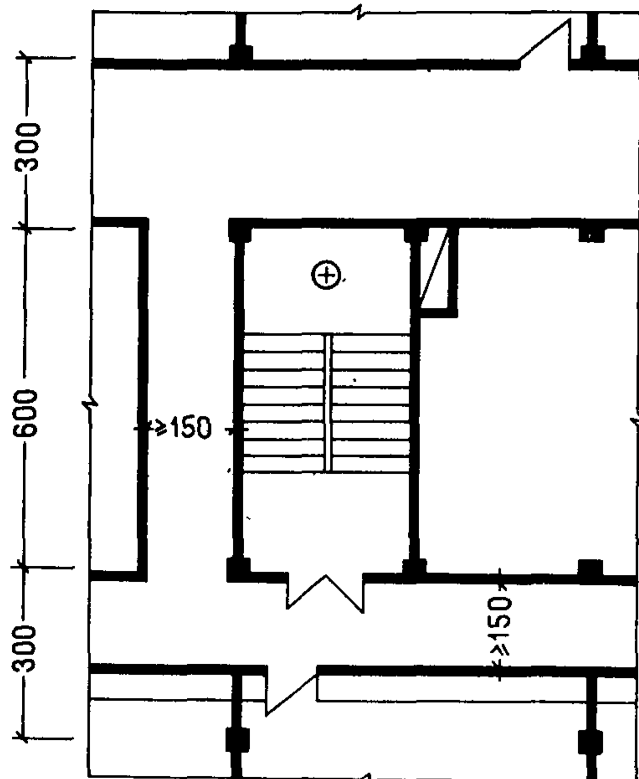
Первый этаж
