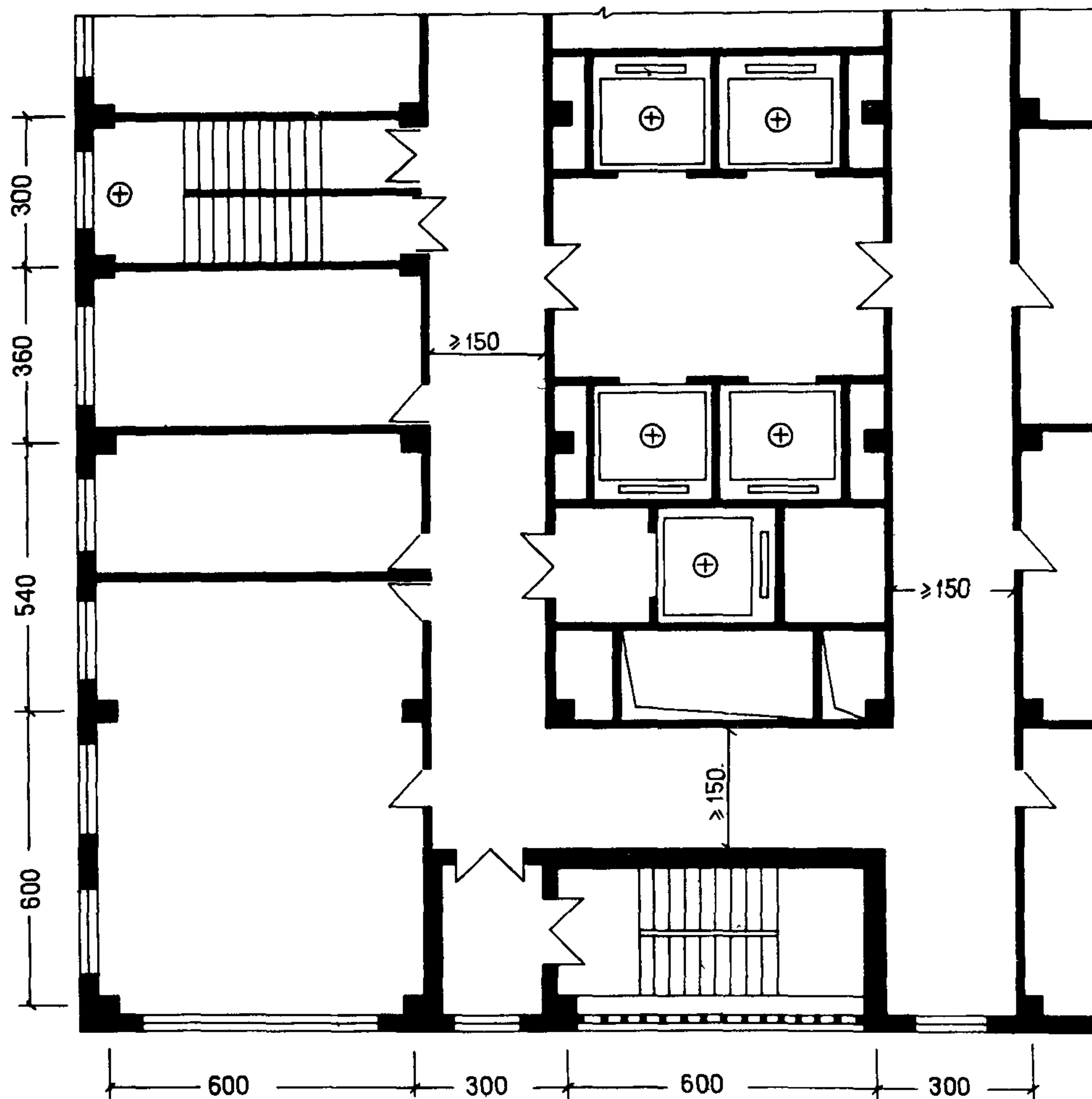
Пример планировки лестнично-лифтового узла
