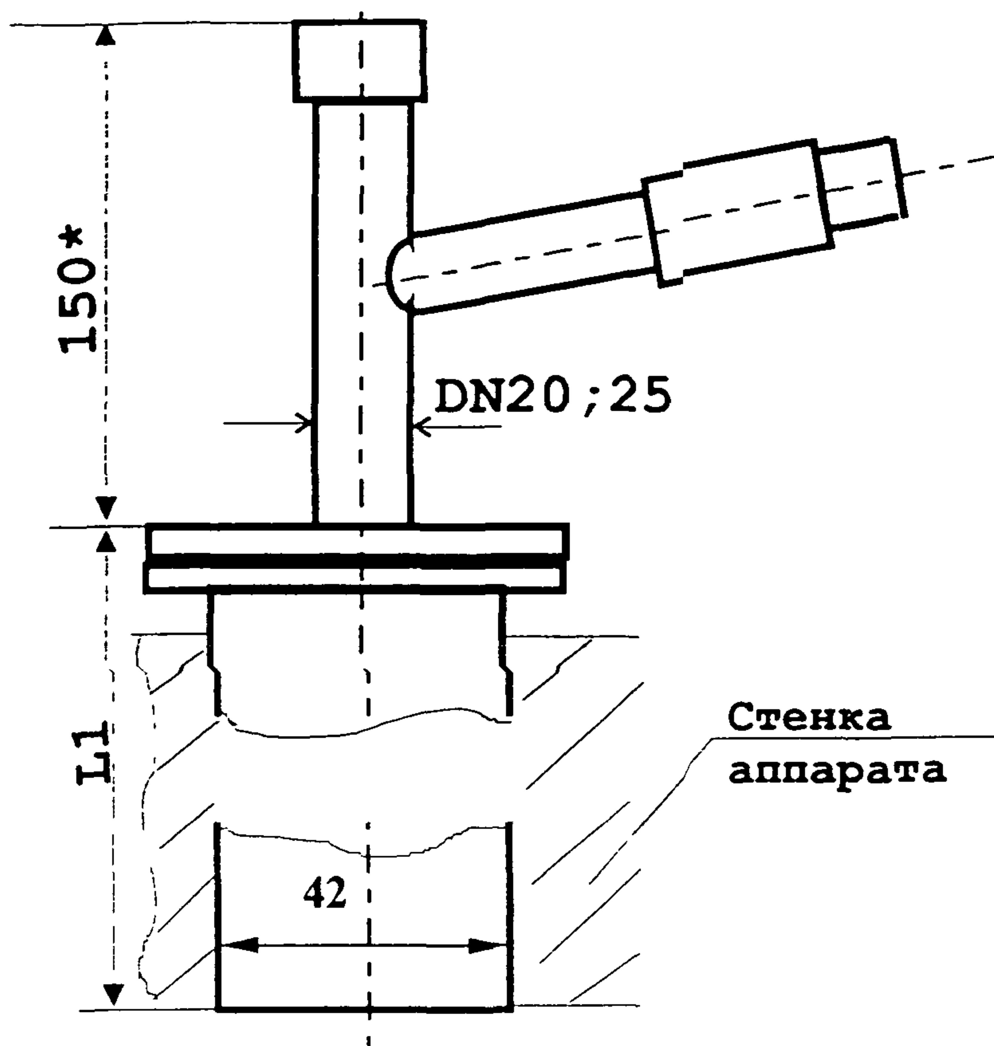
Отборное устройство для запыленных газов с толстостенной обо- лочкой аппарата и не- большими колеба- ниями давления
