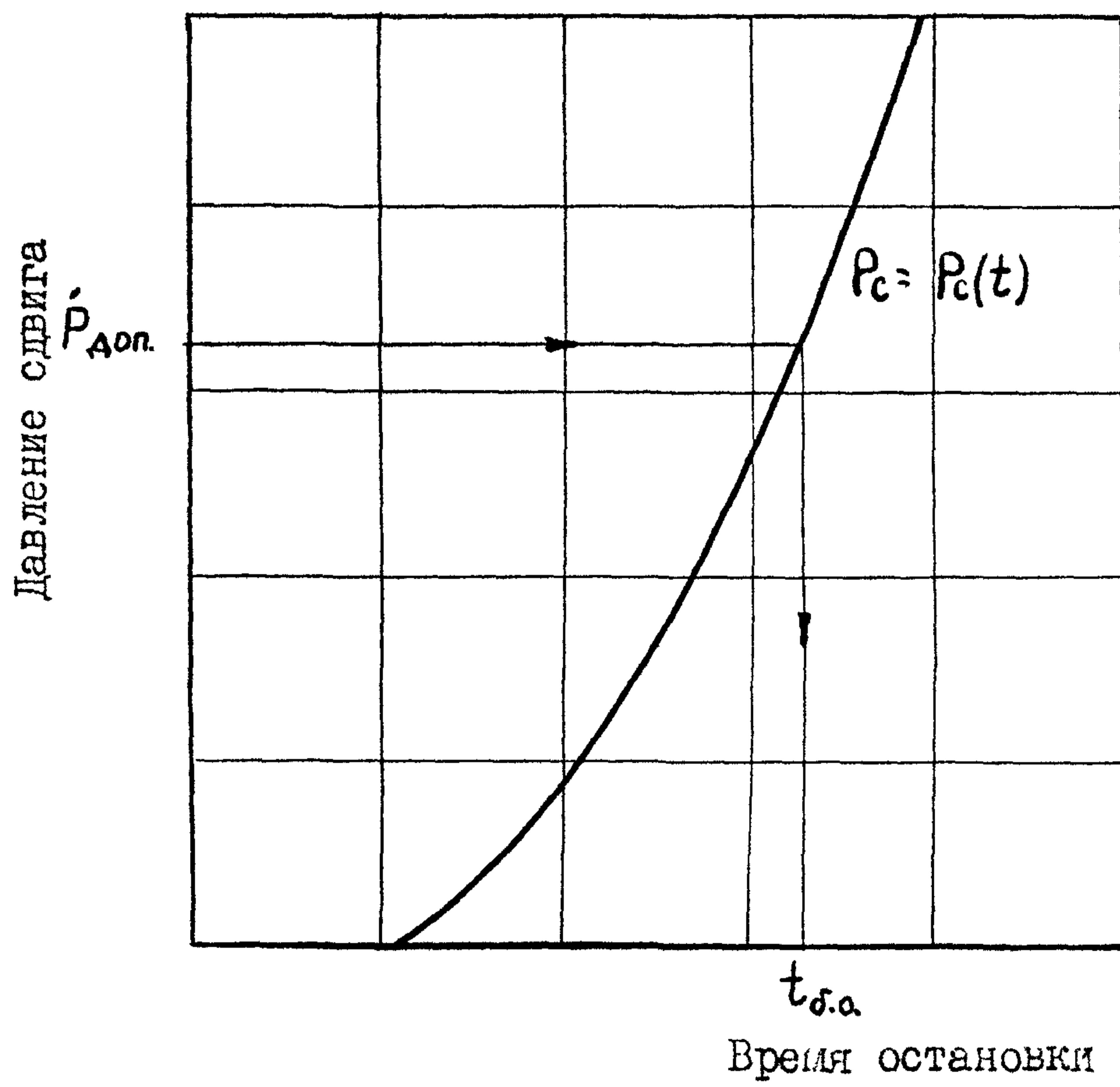
Рис.3. Зависимость давления сдвига от времени остановки перекачки.
