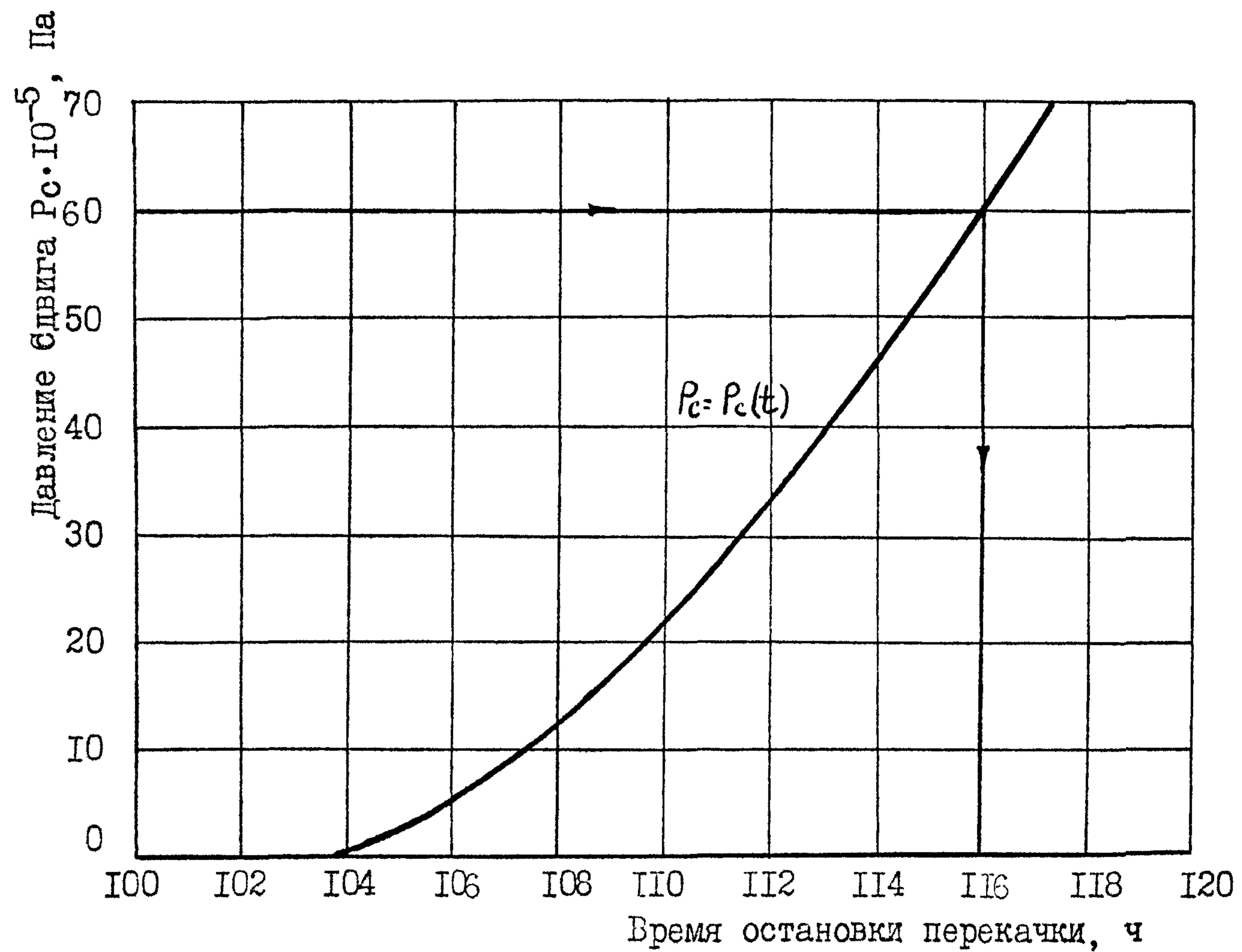
Рис.4. Зависимость давления сдвига от времени остановки перекачки
