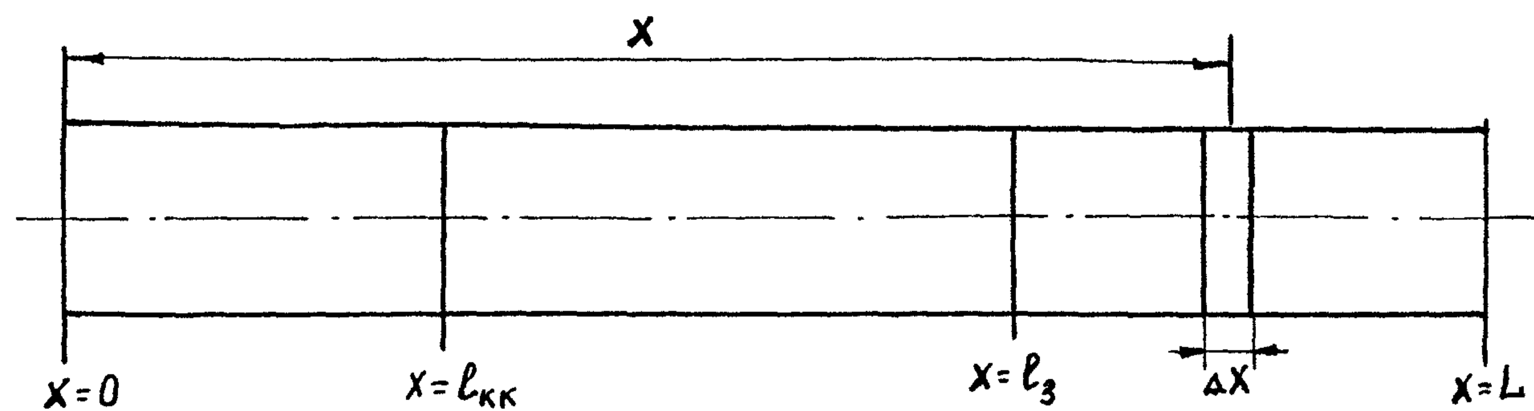
Рис.2. Схема "горячего" трубопровода после его длительной остановки
