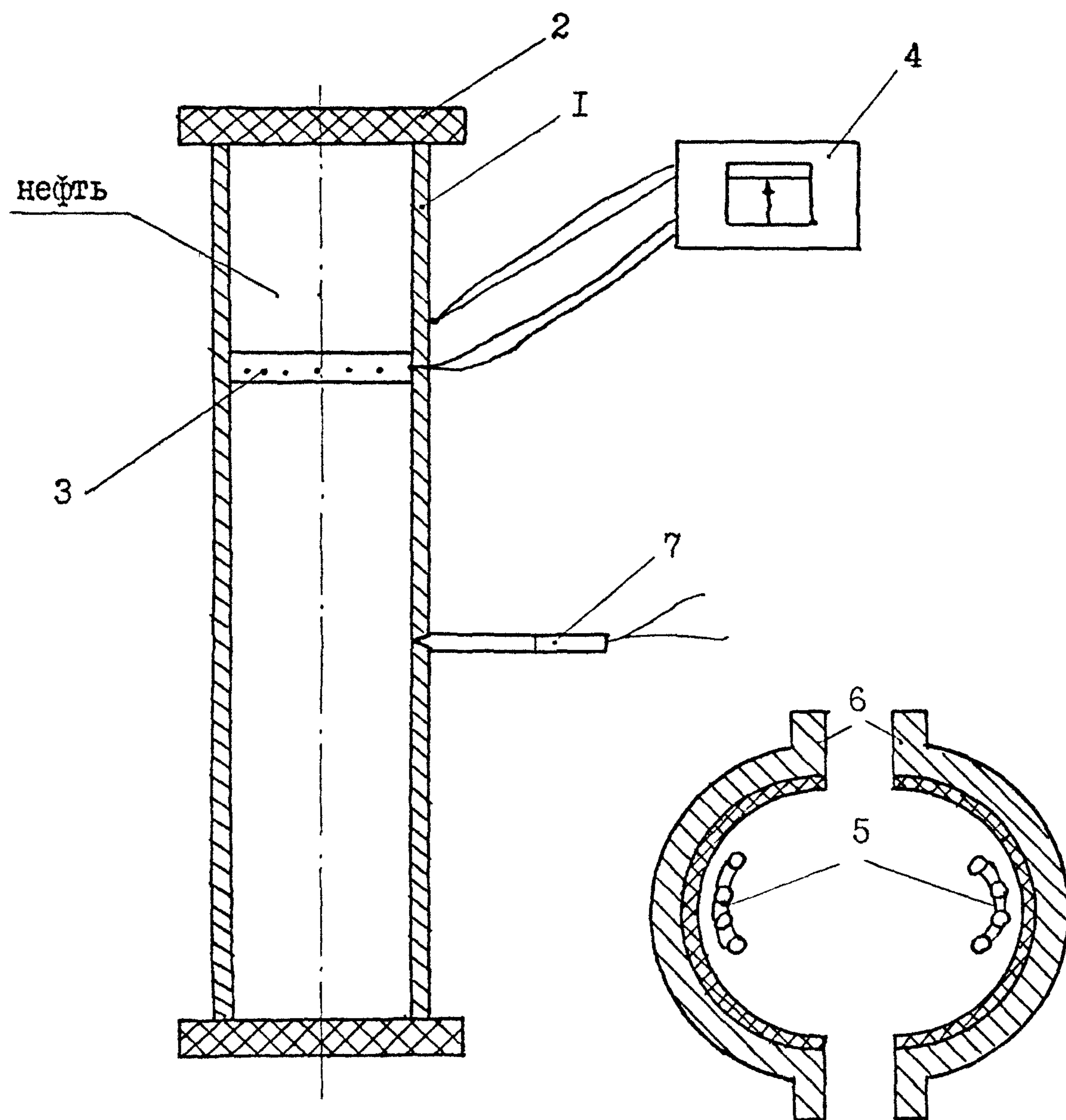
Рис. I. Схема лабораторной установки.
