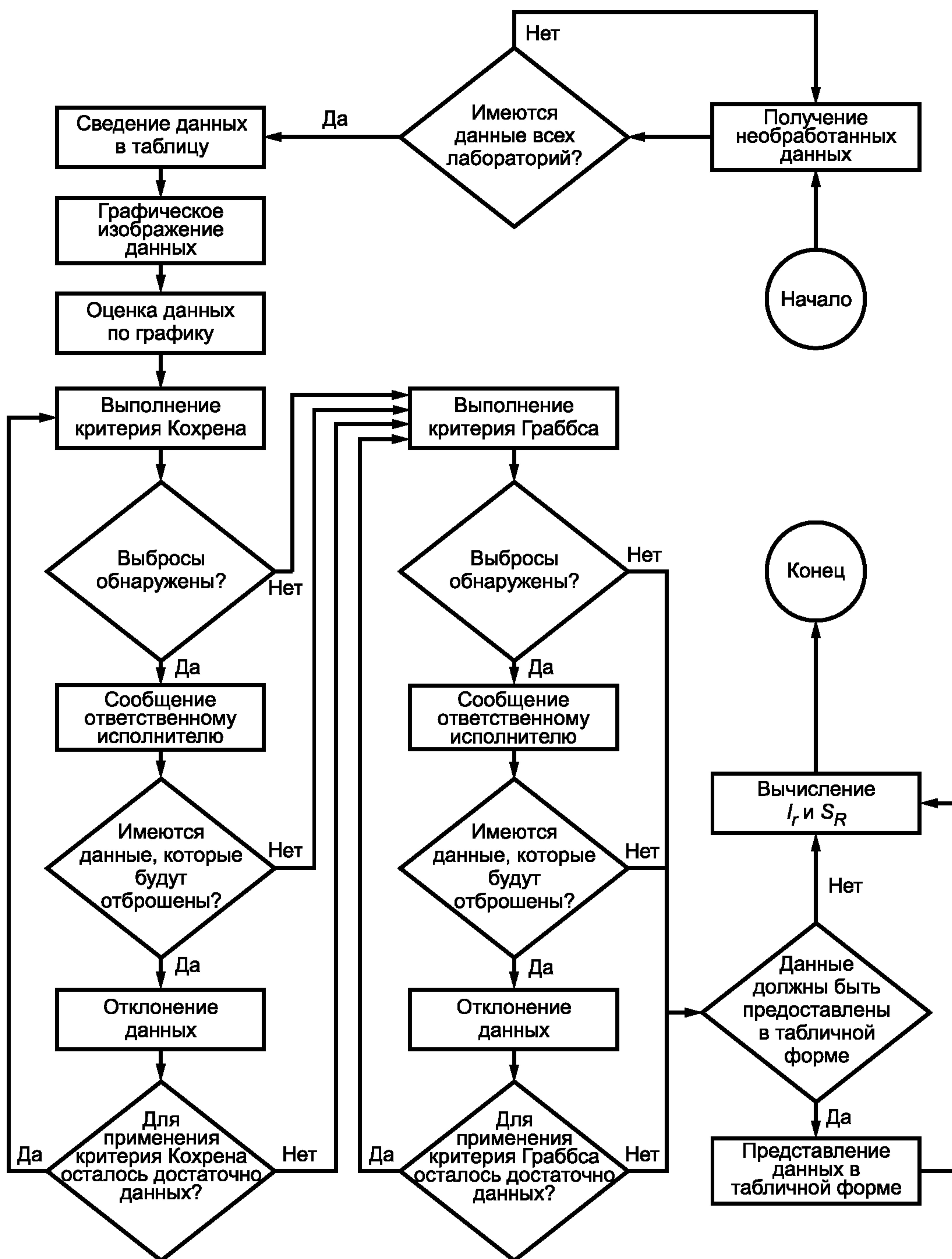
Рисунок 7 — Схема процедуры статистической обработки выбросов
