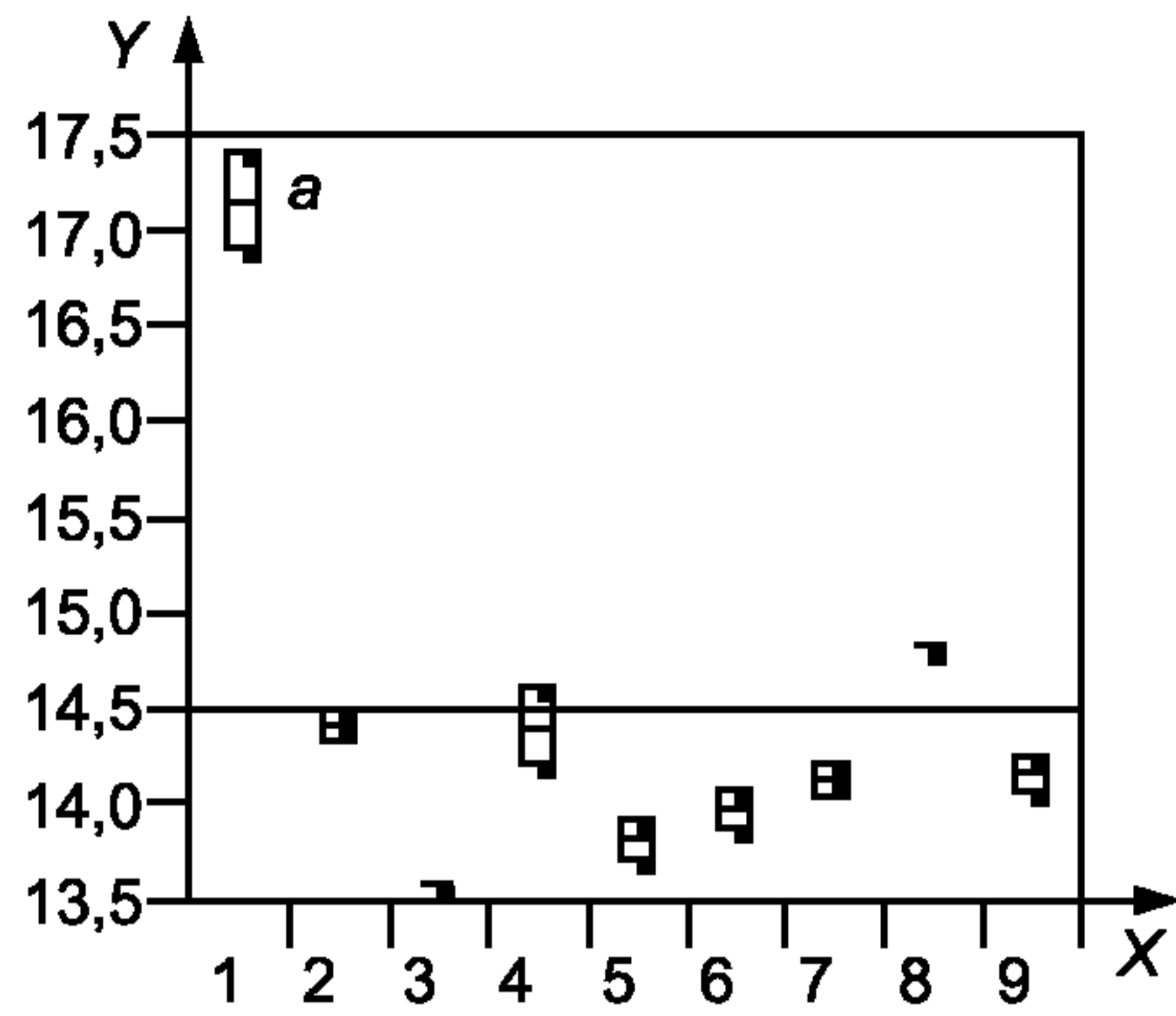
с) Проверка дисперсии уровня 3
