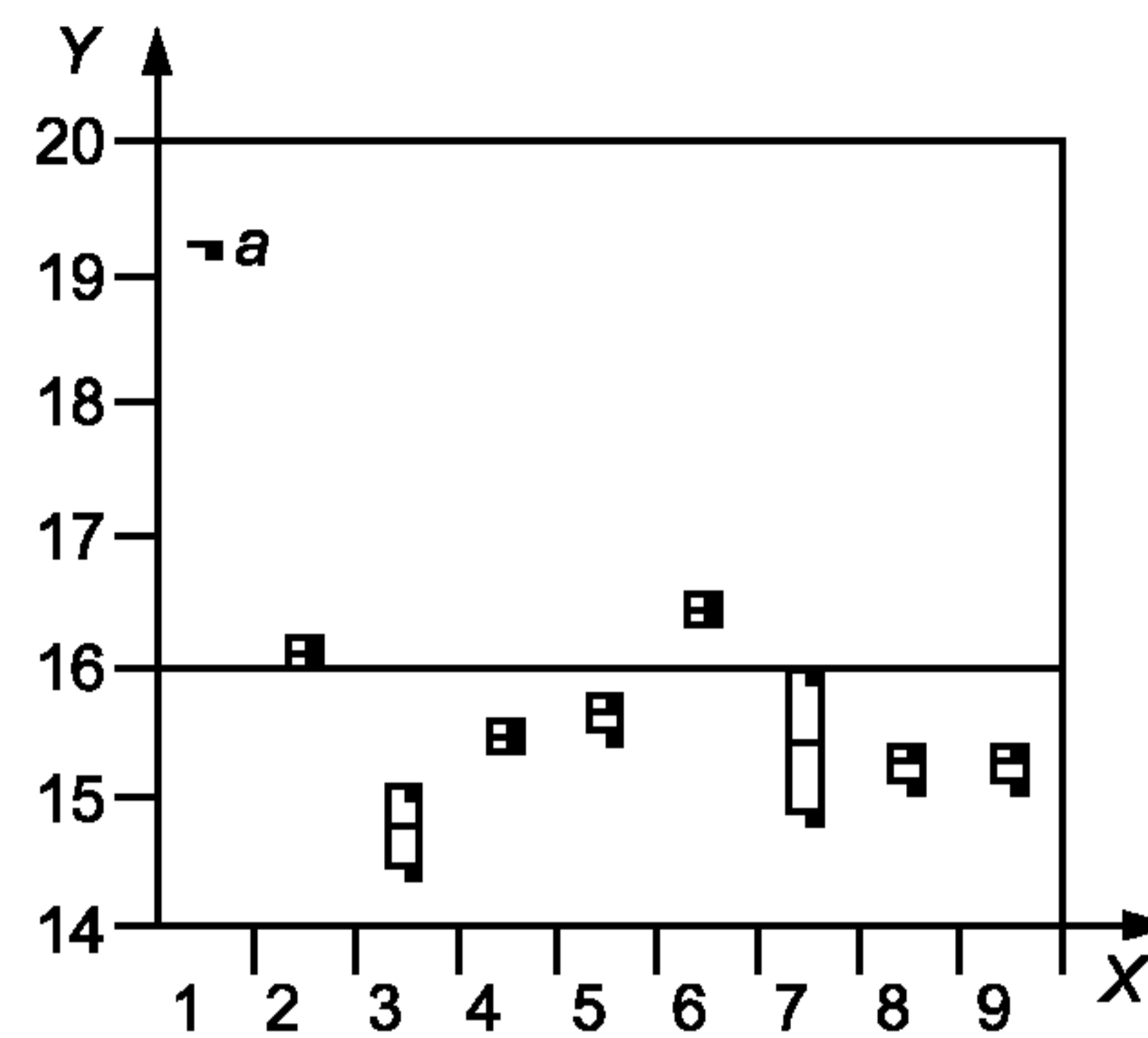
д) Проверка дисперсии уровня 4
