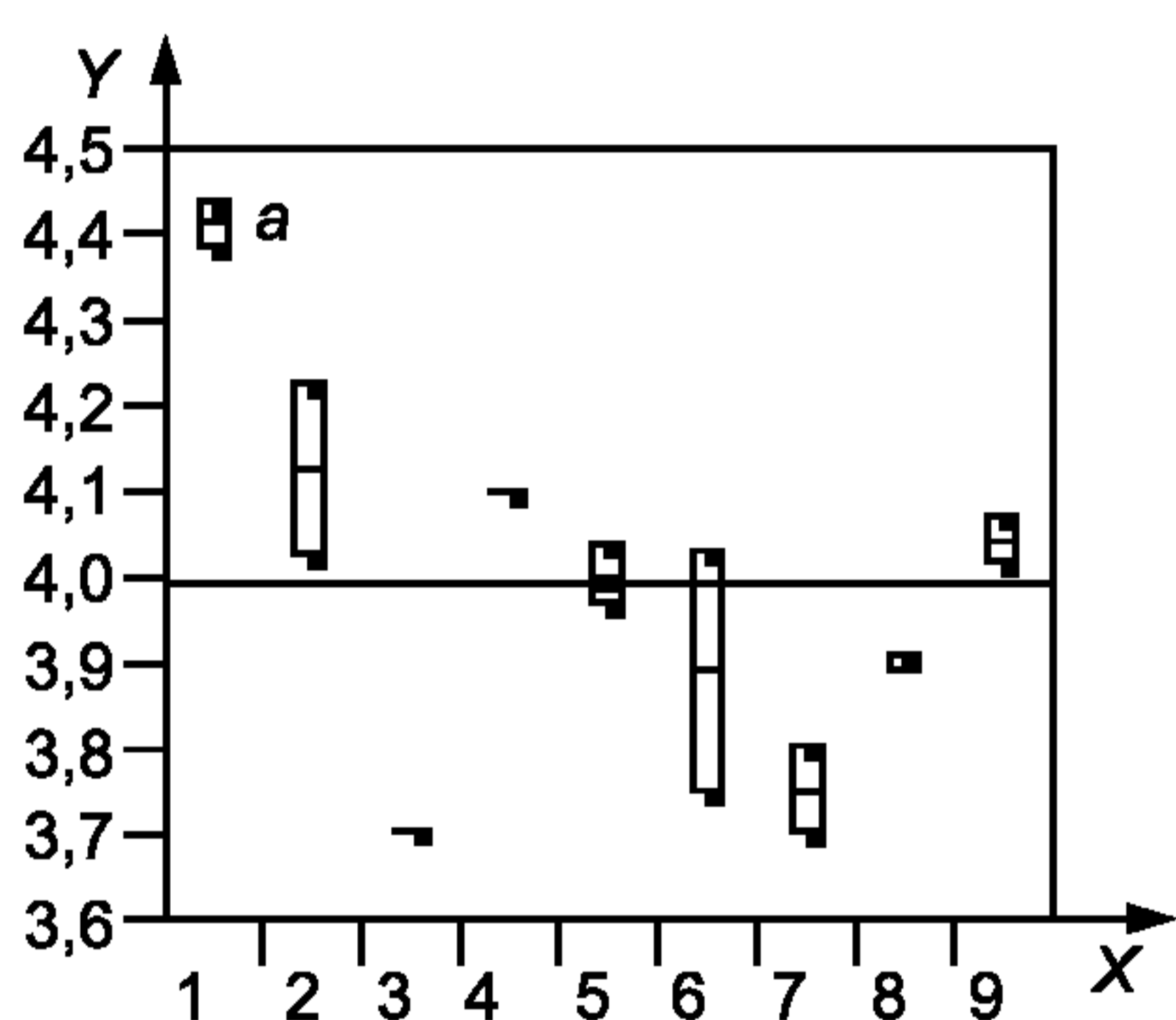
а) Проверка дисперсии уровня 1
