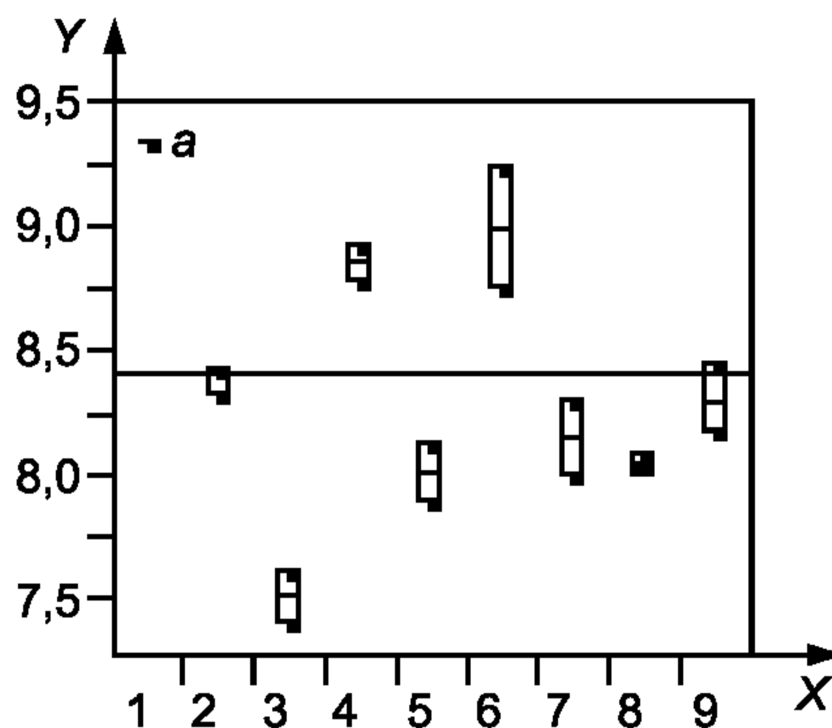
б) Проверка дисперсии уровня 2
