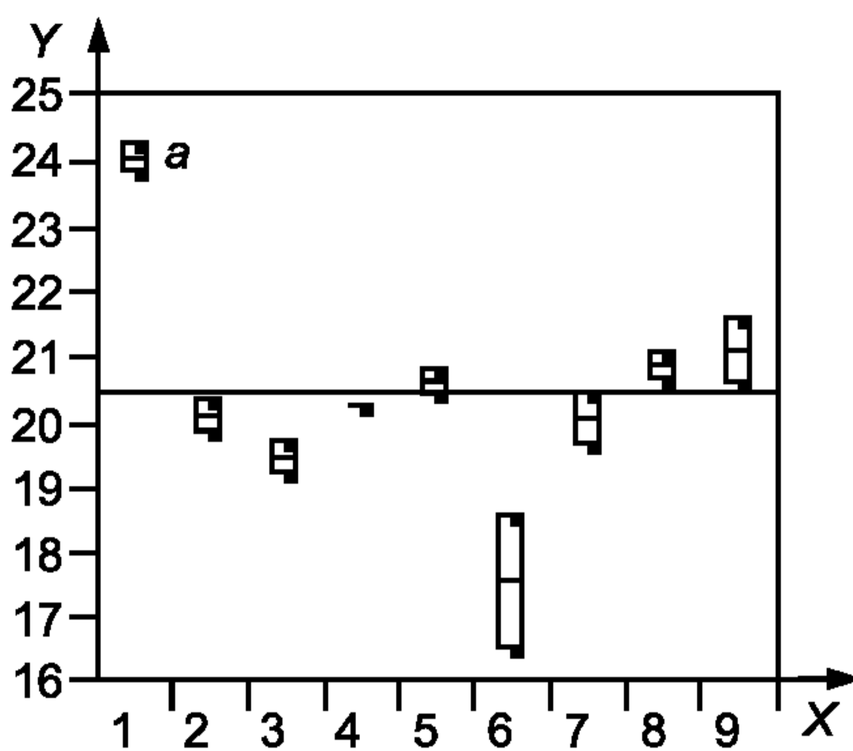
е) Проверка дисперсии уровня 5
