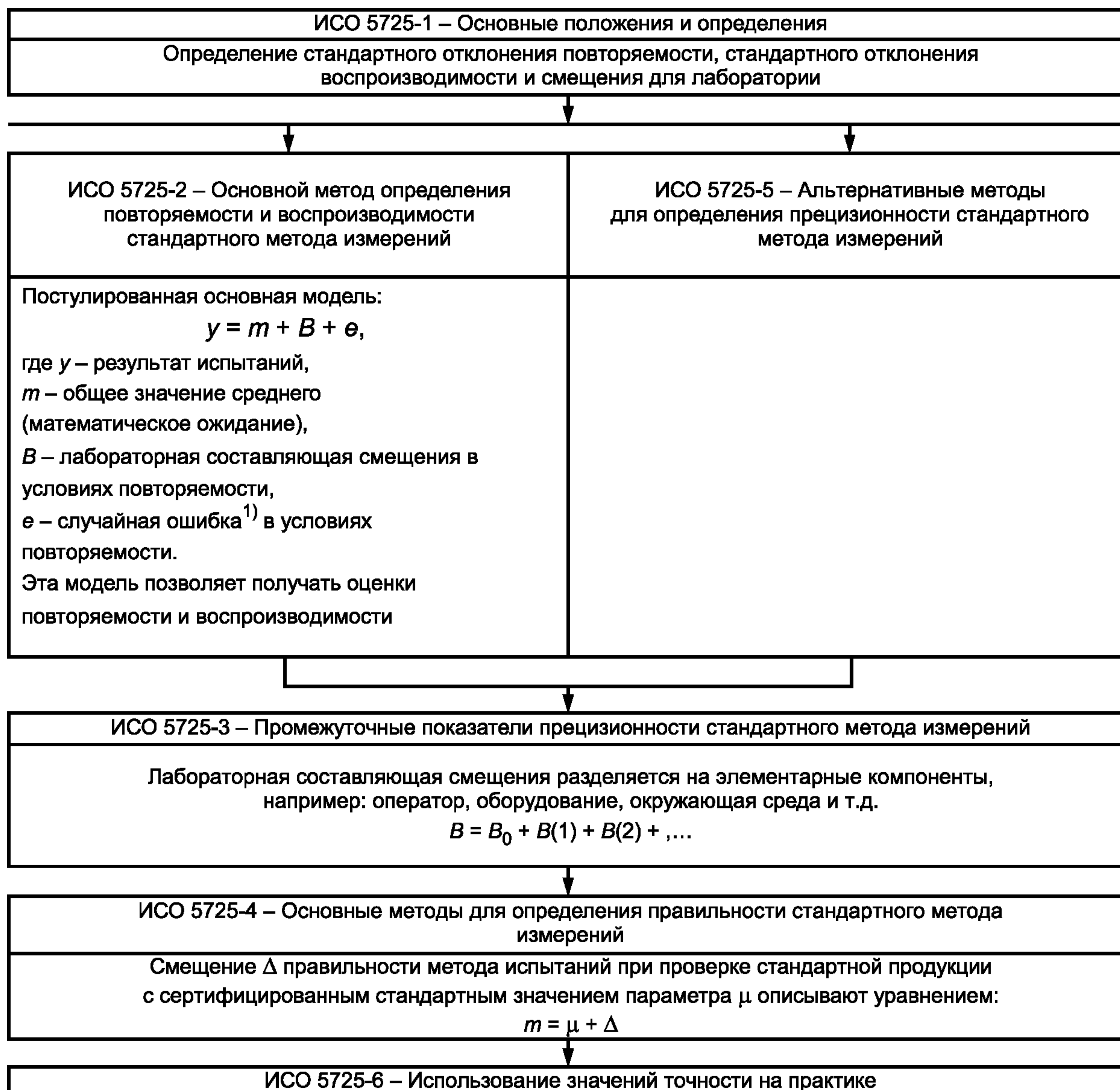
Рисунок 1 — Структура серии стандартов ИСО 5725
