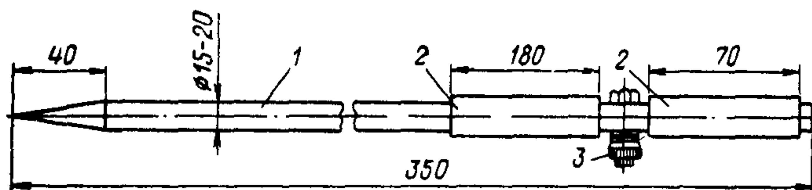
Рис. 5. Стальной электрод
