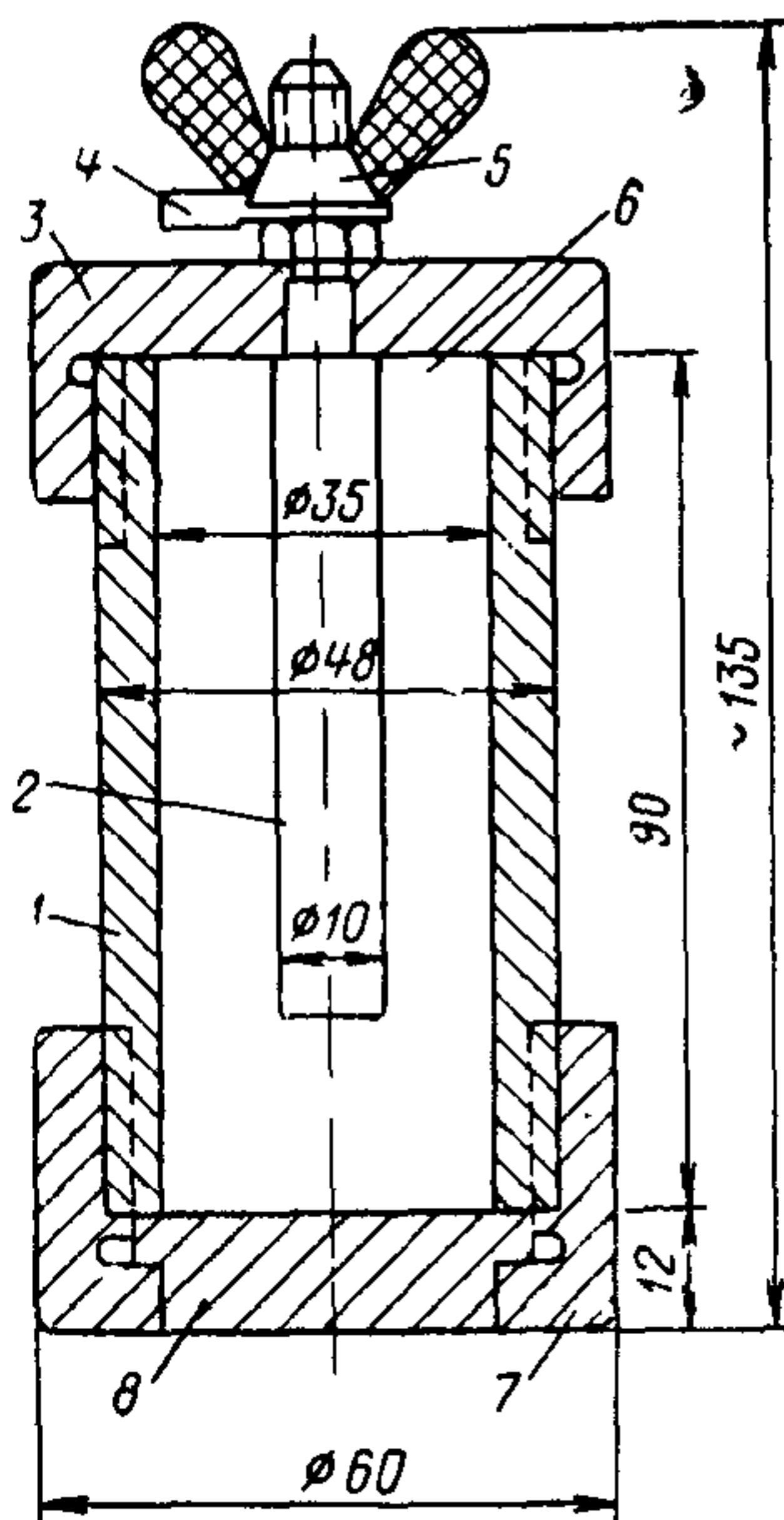
Рис. 6. Неполяризующийся медно-сульфатный электрод
