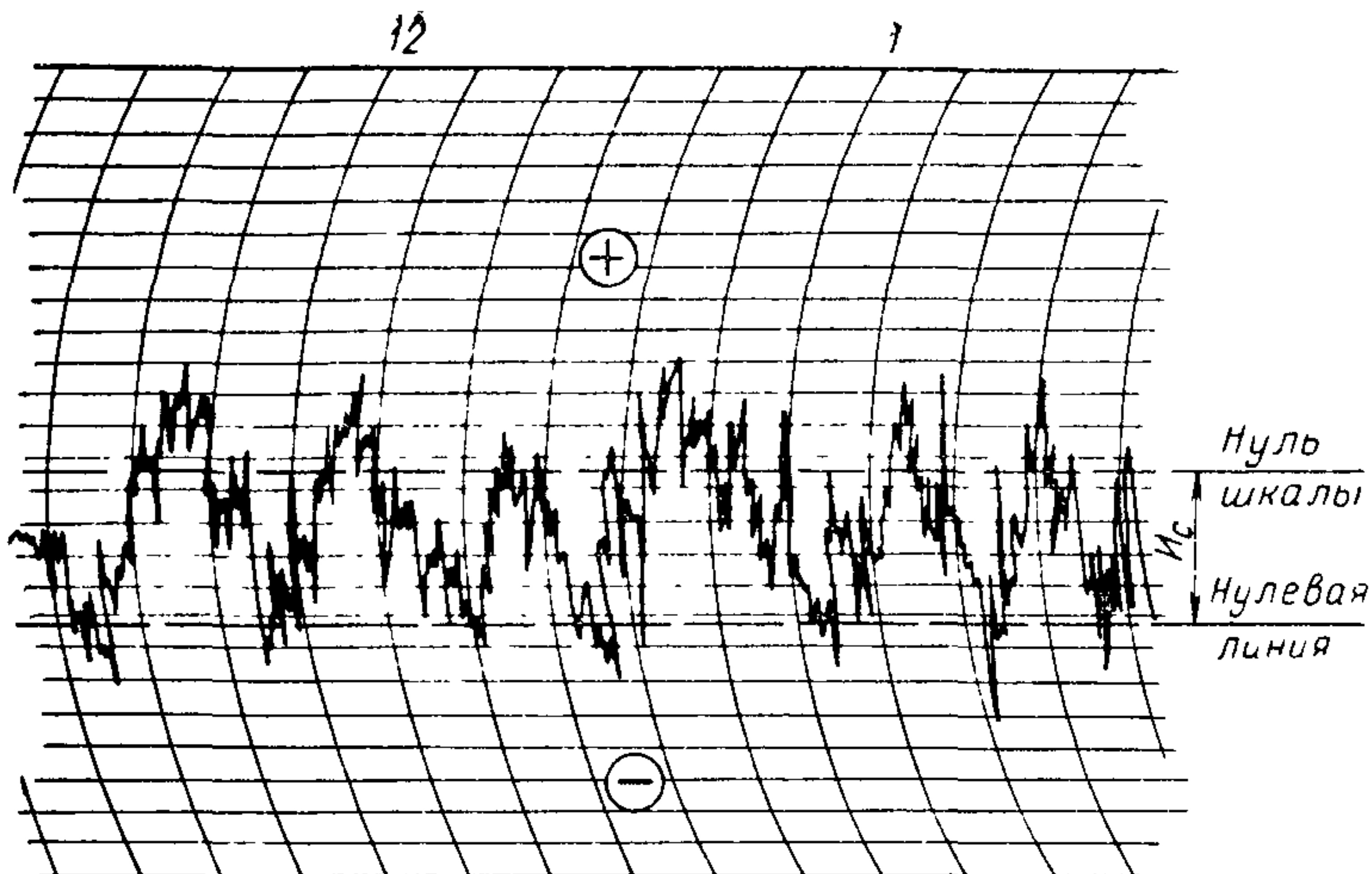
Рис. 2. Образец диаграммы самопишущего прибора
