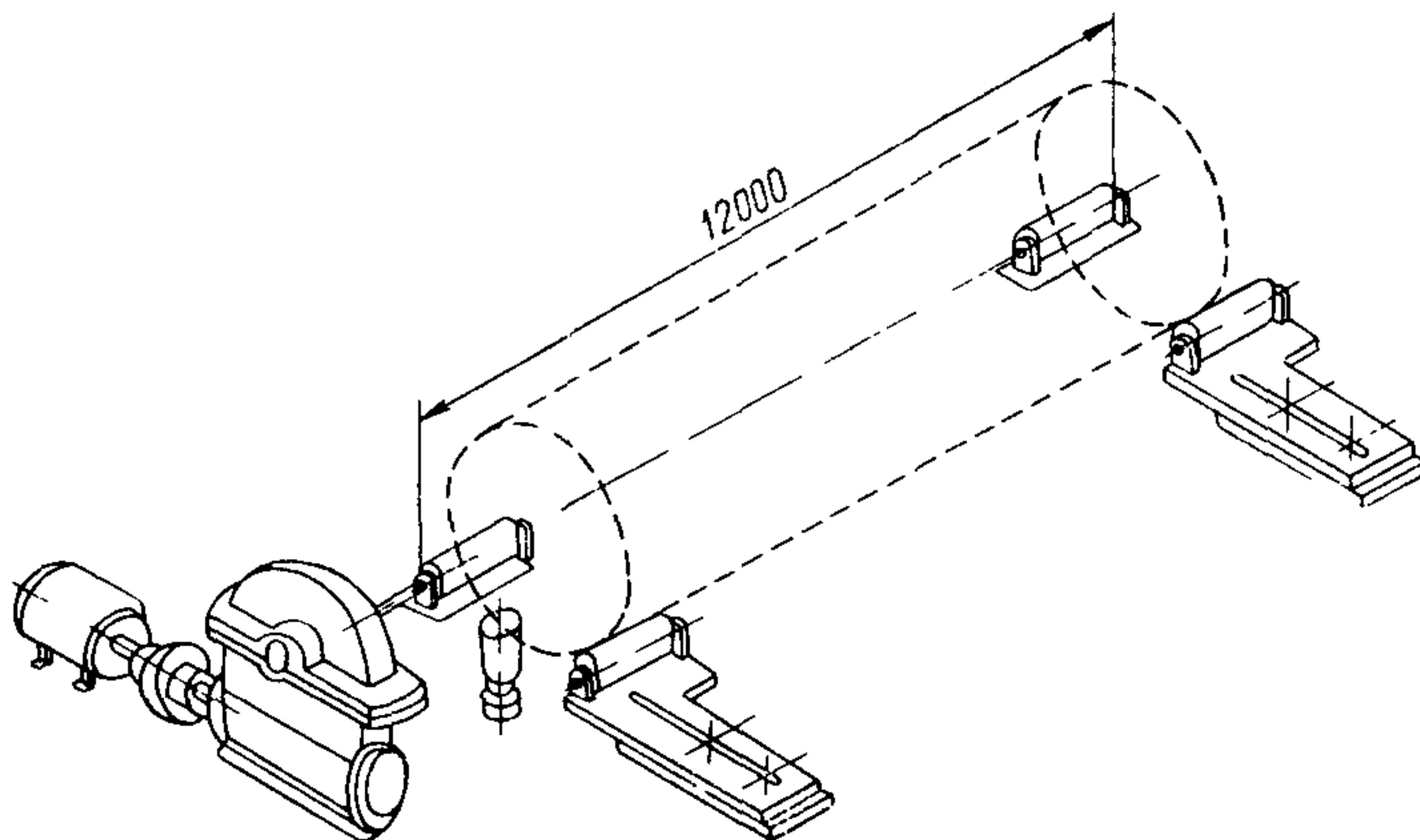
Рис 4. Установка с механическим приводом для вращения труб
