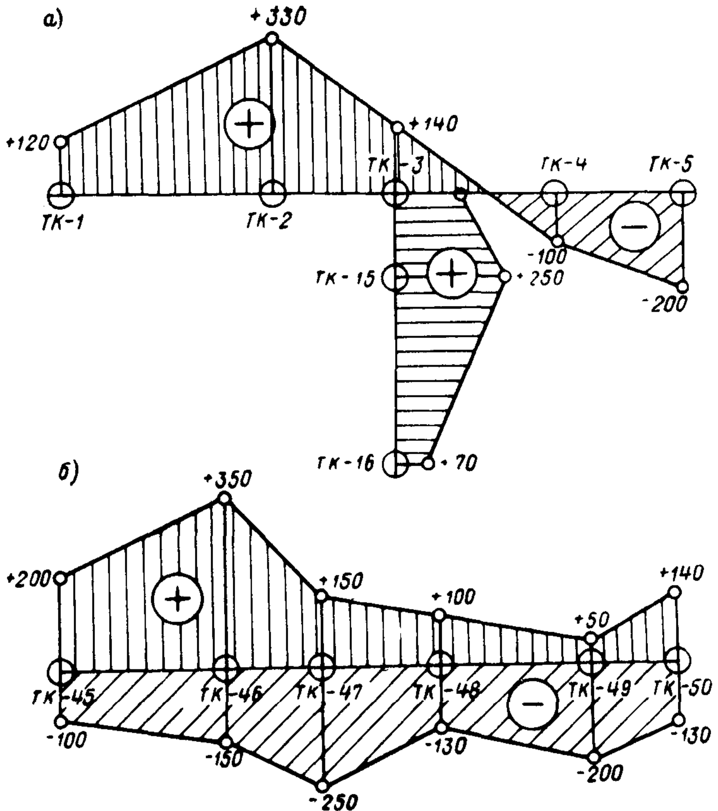
Рис. 3. Построение диаграмм потенциалов на плане сети теплопроводов
