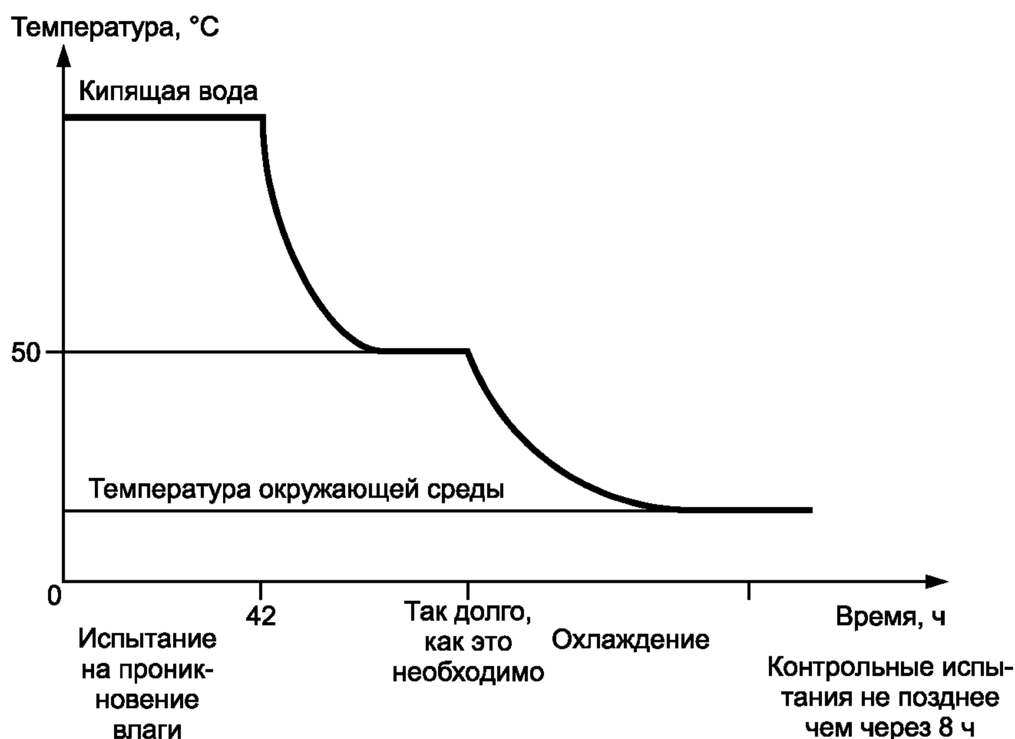
Рисунок 6 — Испытания на проникновение влаги
