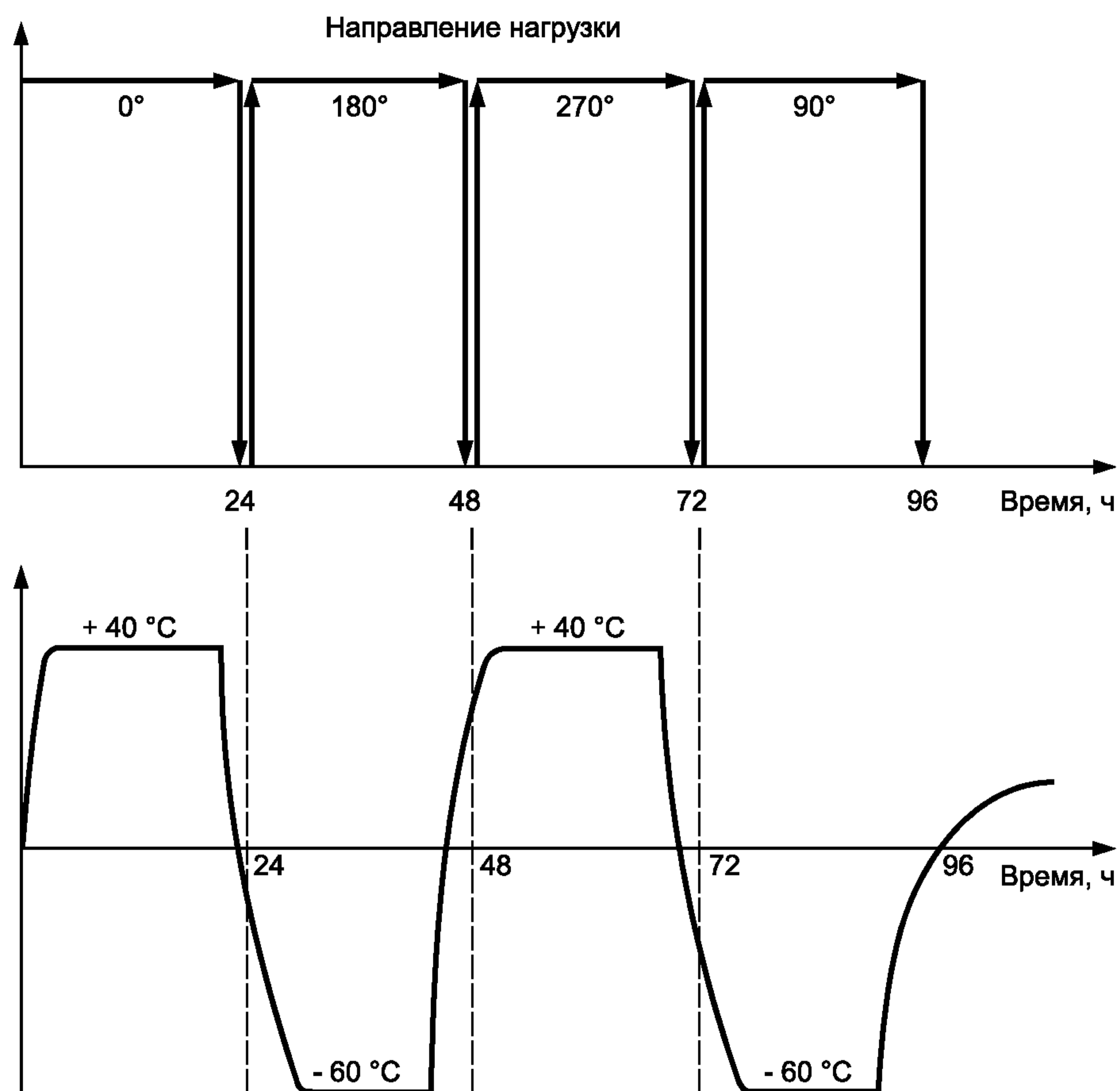
Рисунок 4 — Термомеханические испытания
