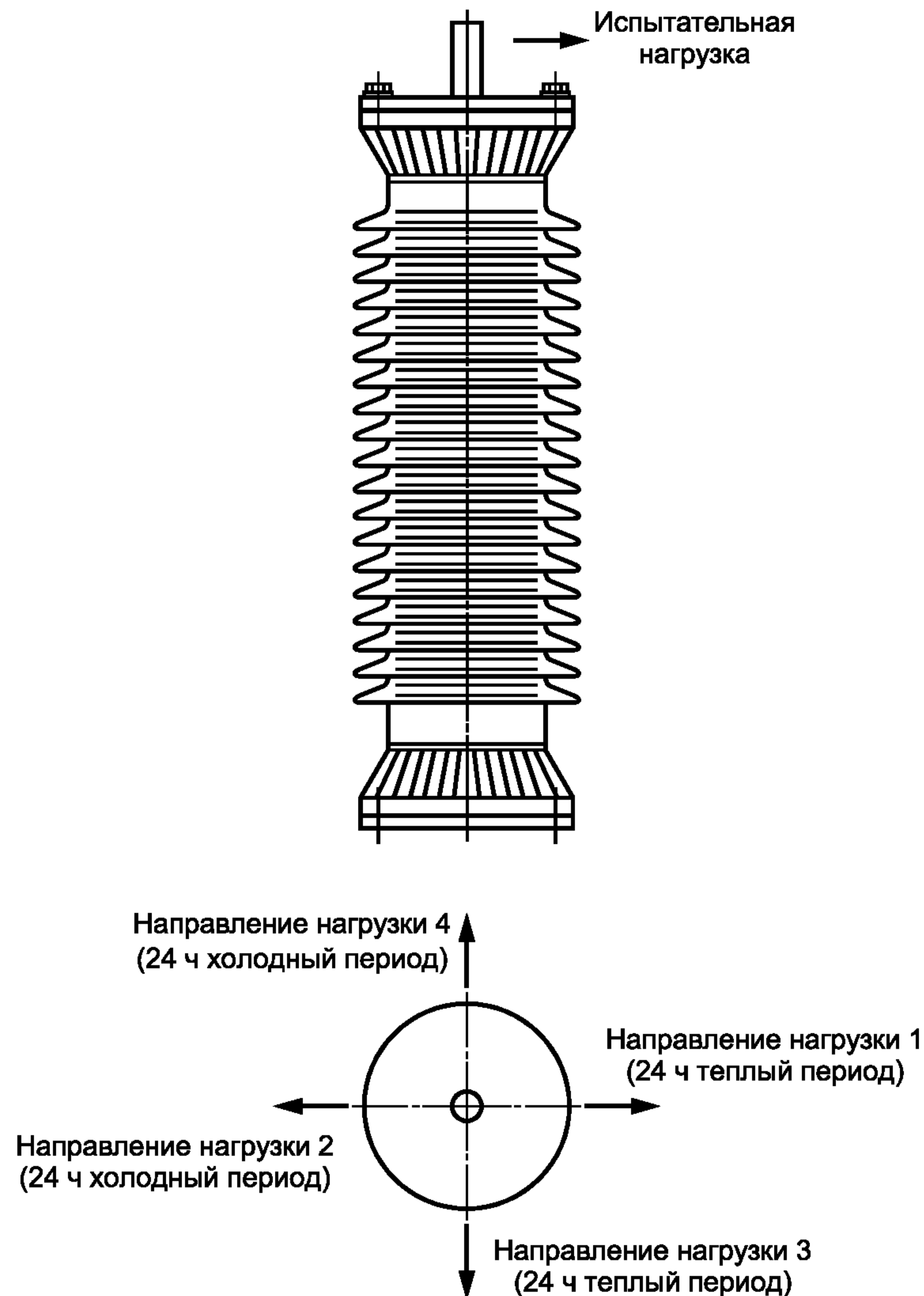
Рисунок 5 — Направления действия изгибающей нагрузки при термомеханических испытаниях
