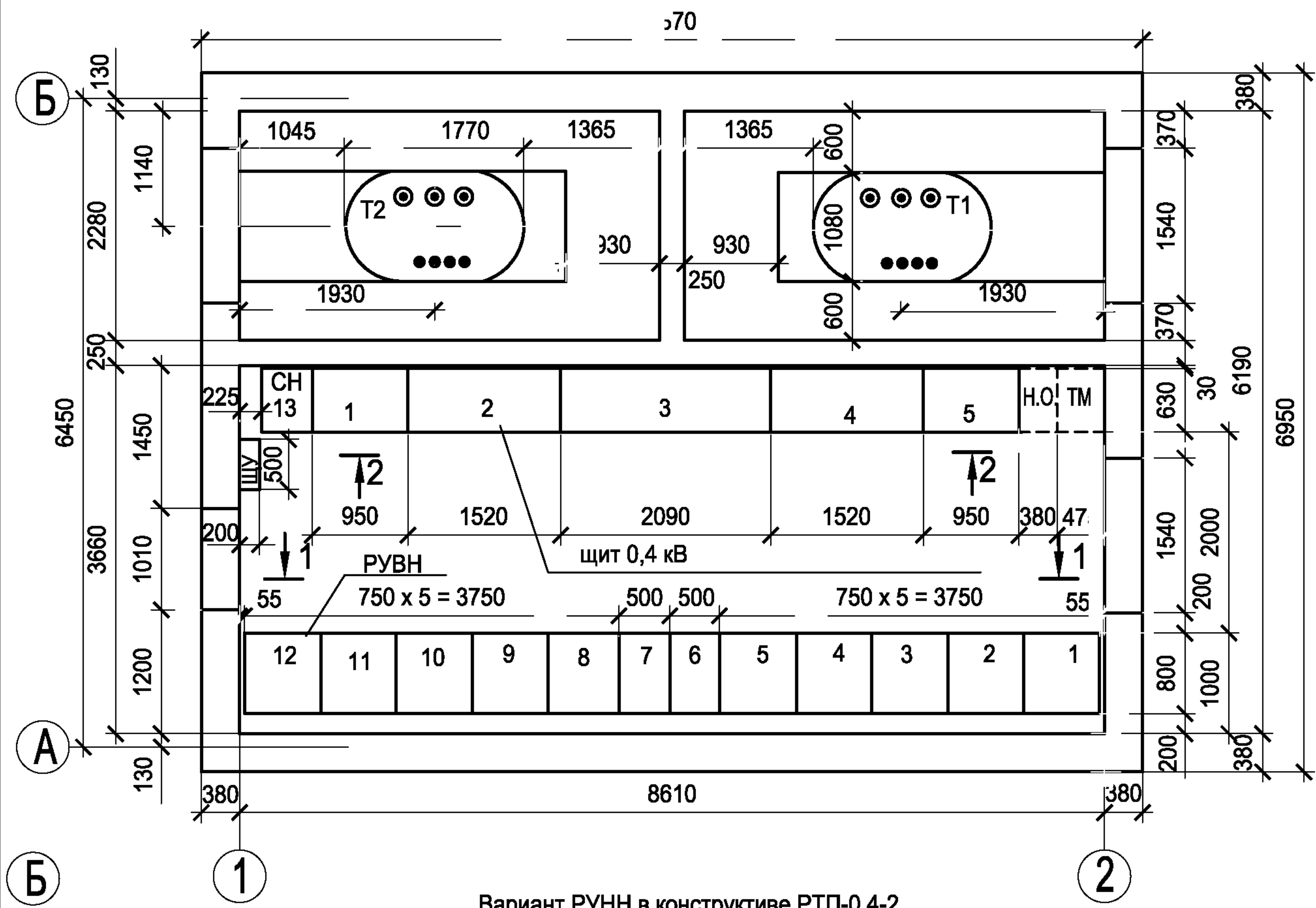
Вариант РУНН в конструктиве РТП-0,4-1
