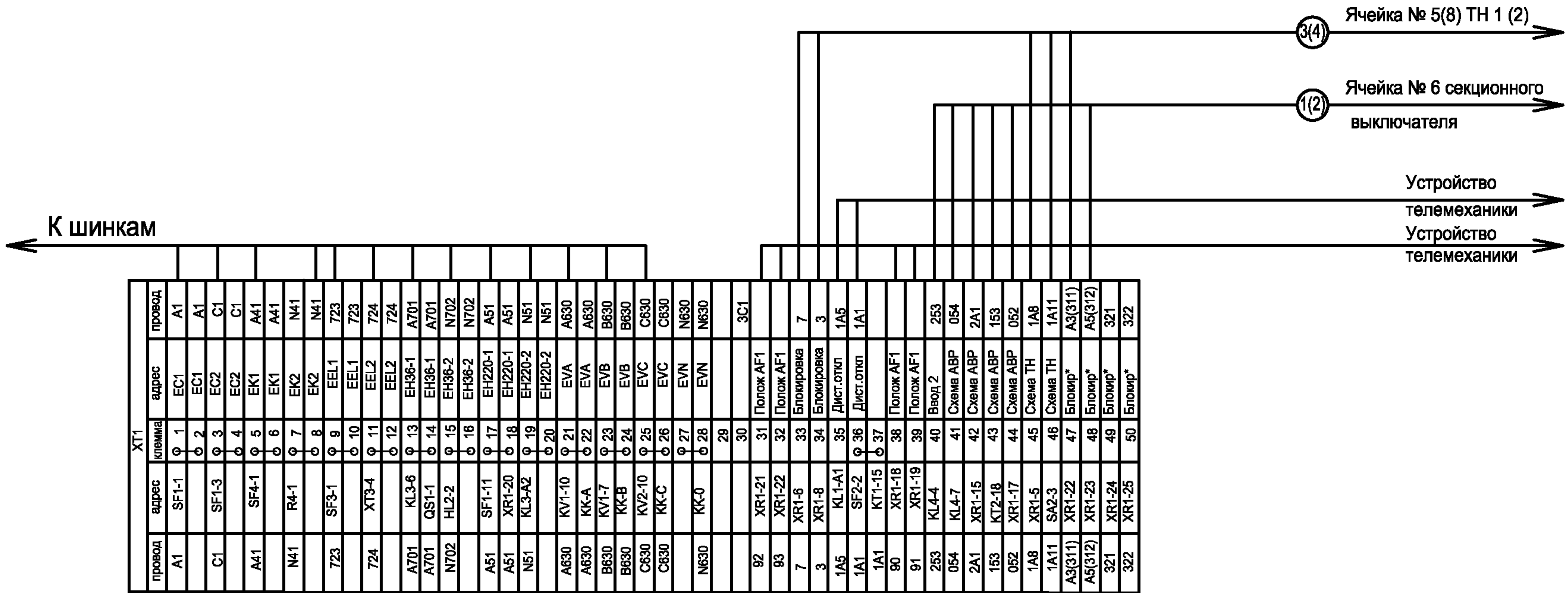
Схему электрическую принципиальную ячейки ввода 10 (6) кВ см. чертеж № 407 - 3 - 660.03 - ЭП листы 11...15.
