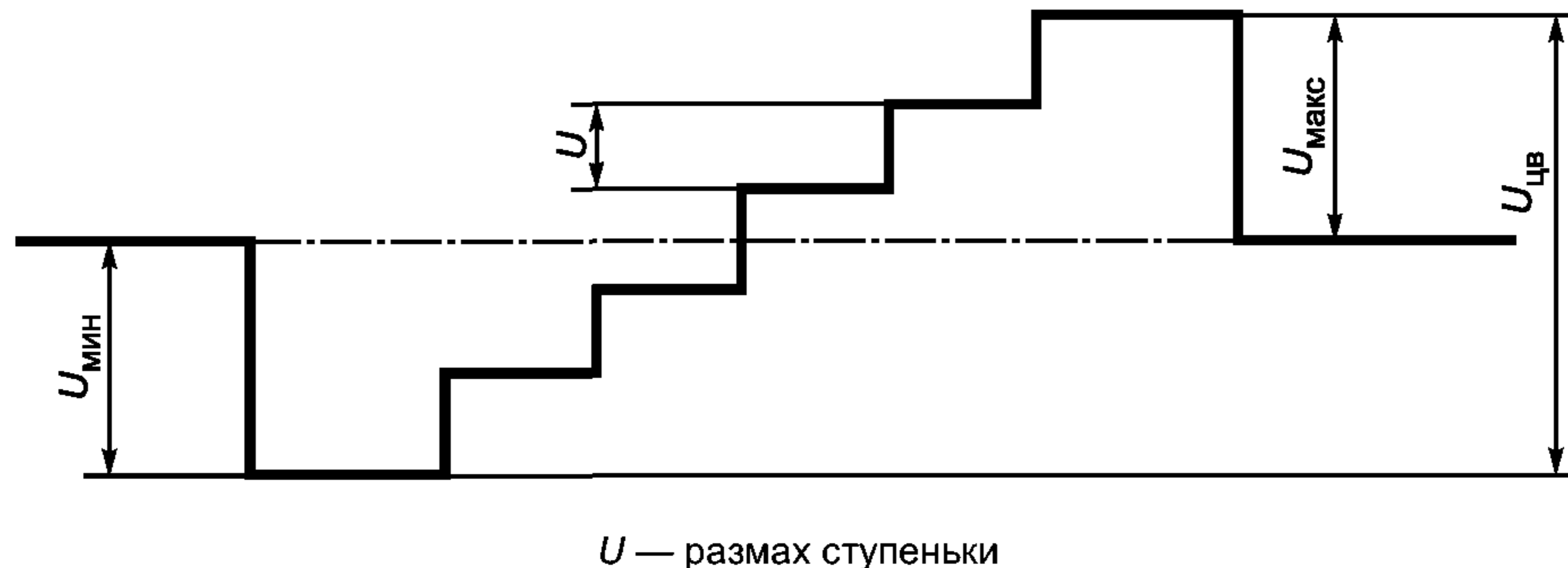
Рисунок 4 — Осциллограмма сигнала для измерения параметров каналов цветности
