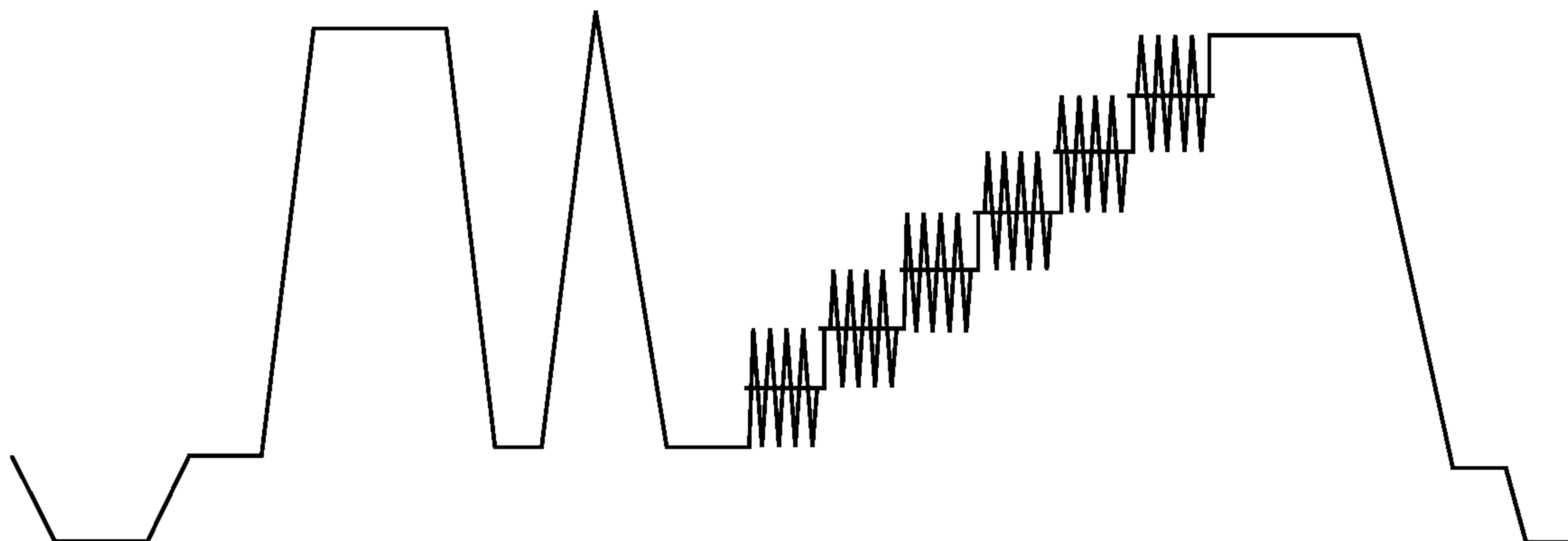
Рисунок 2 — Графическое изображение измерительного сигнала, содержащего сигнал Н1
