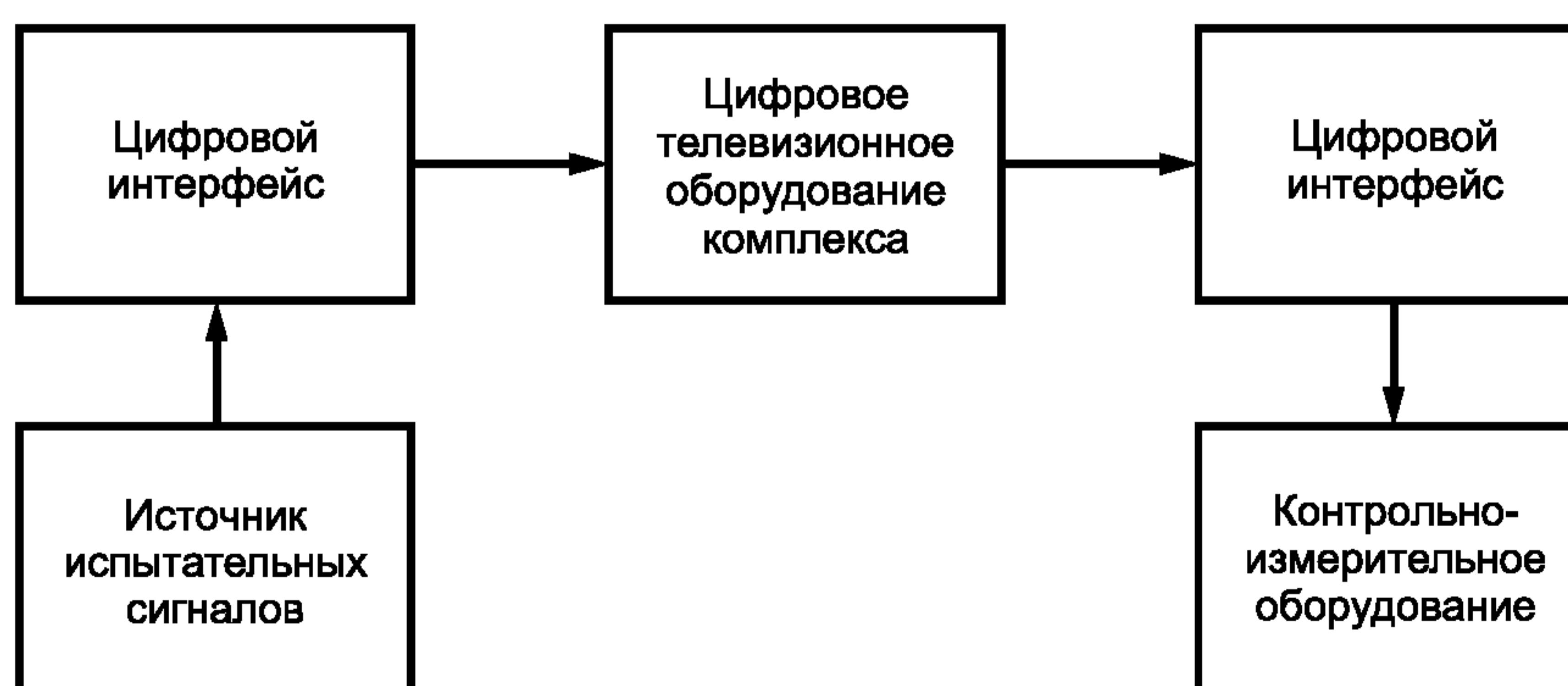
Рисунок 3 — Схема измерения параметров студийного (внестудийного) комплекса
