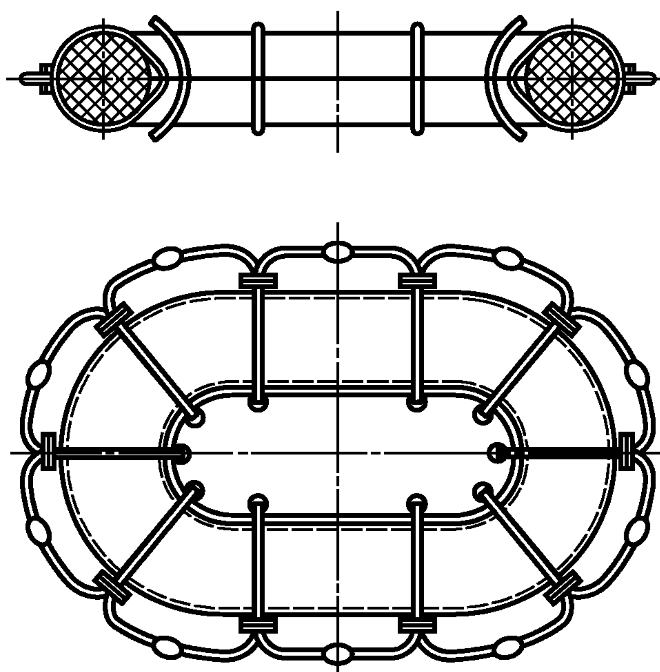
Рисунок 1 — Спасательный прибор
