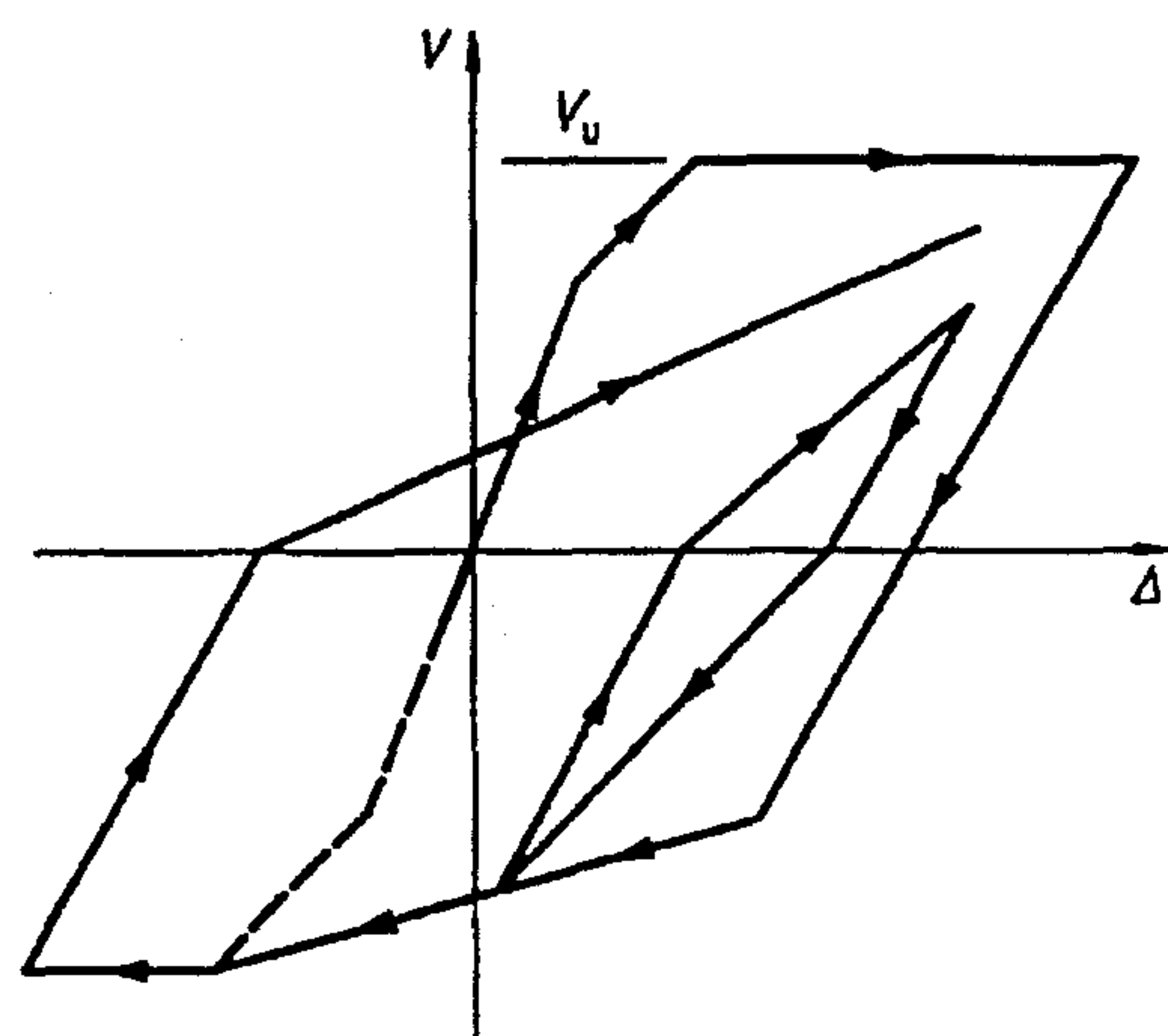
б) модель трехлинейная с пониженными характеристиками
