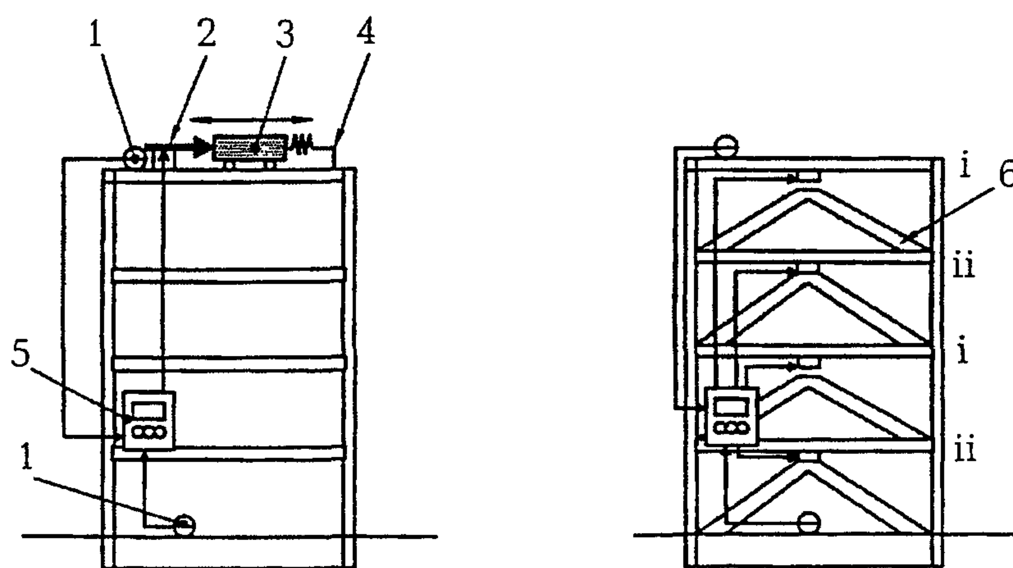
Рисунок I.2 - Пример пассивной системы управления
