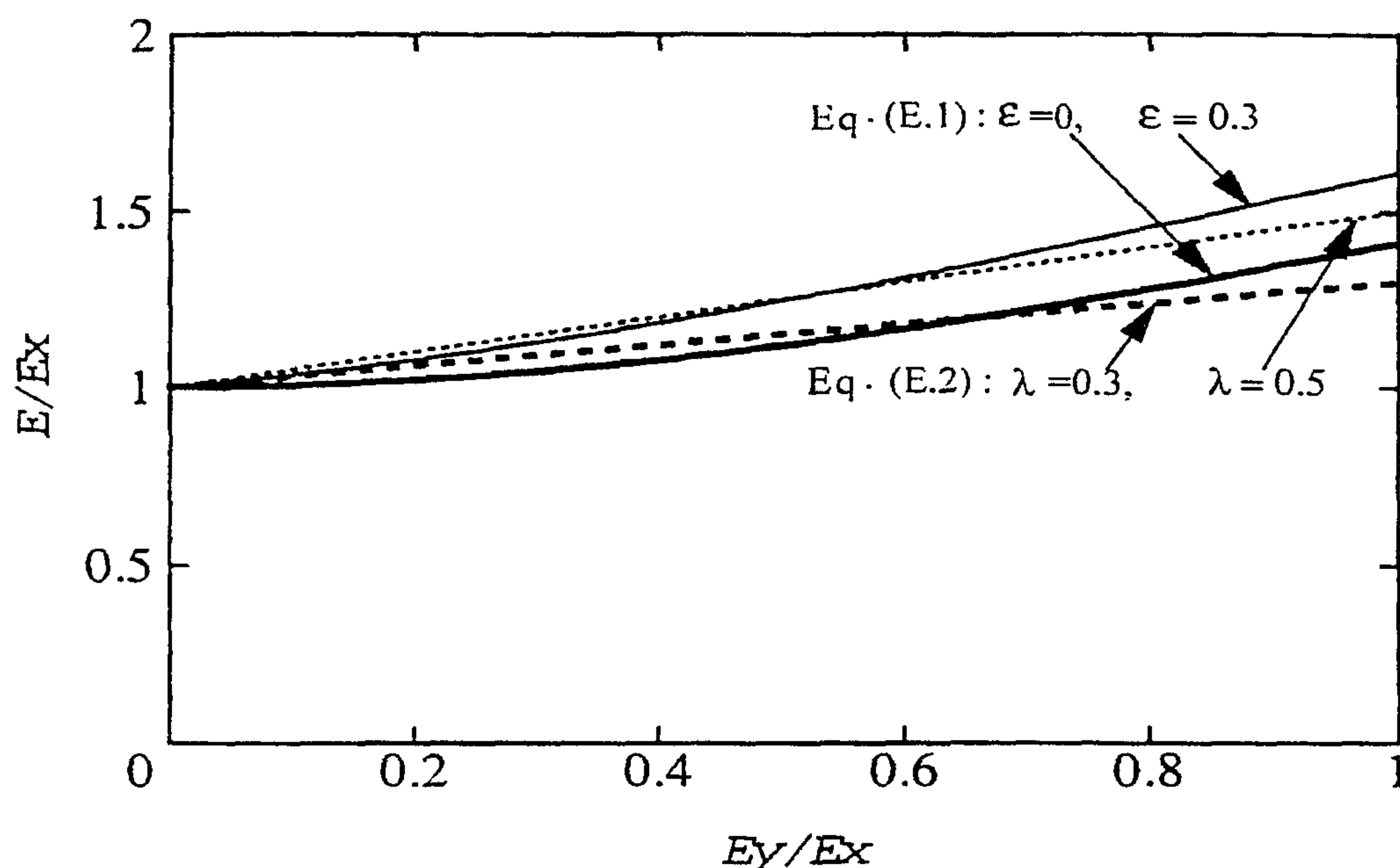
Рисунок Е.1 - Взаимосвязь между \frac{E}{E_x} на основе \frac{E_y}{E_x} согласно уравнениям (Е.1) и (Е.2)
