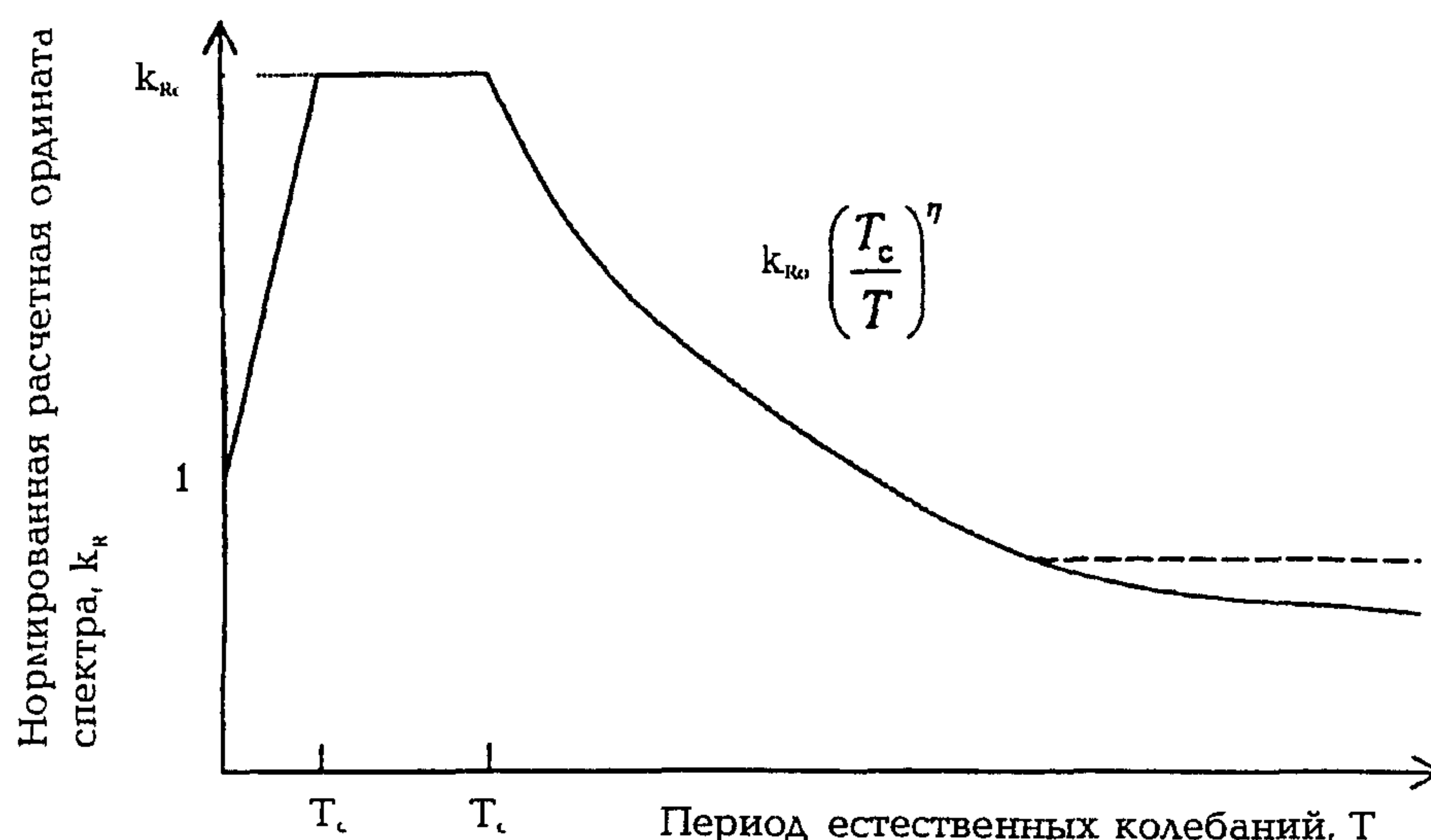
Рисунок С.1 – Нормированный расчетный спектр реакции
