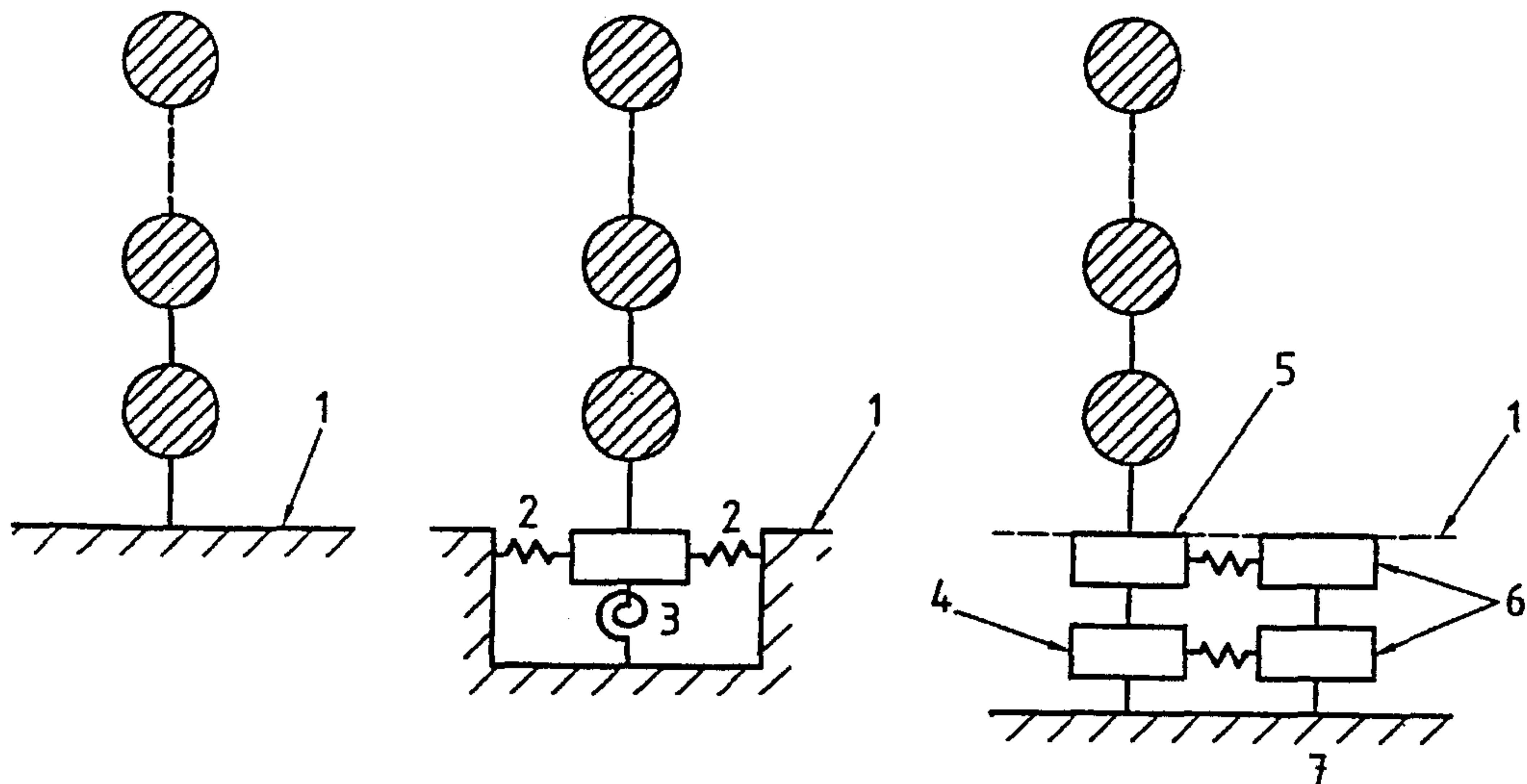
а) модель, укреплен- ная у основания
