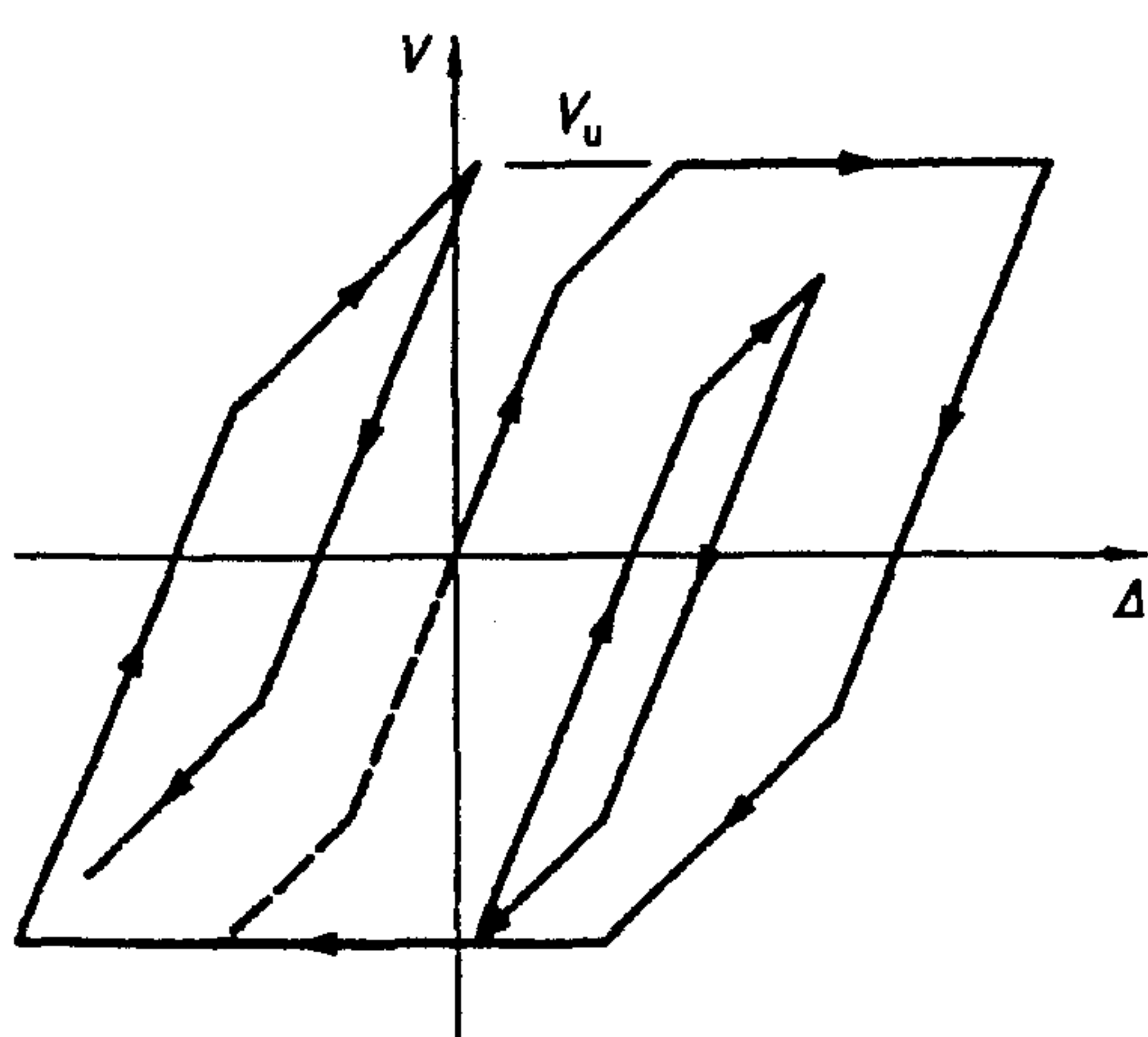
а) трехлинейная модель
