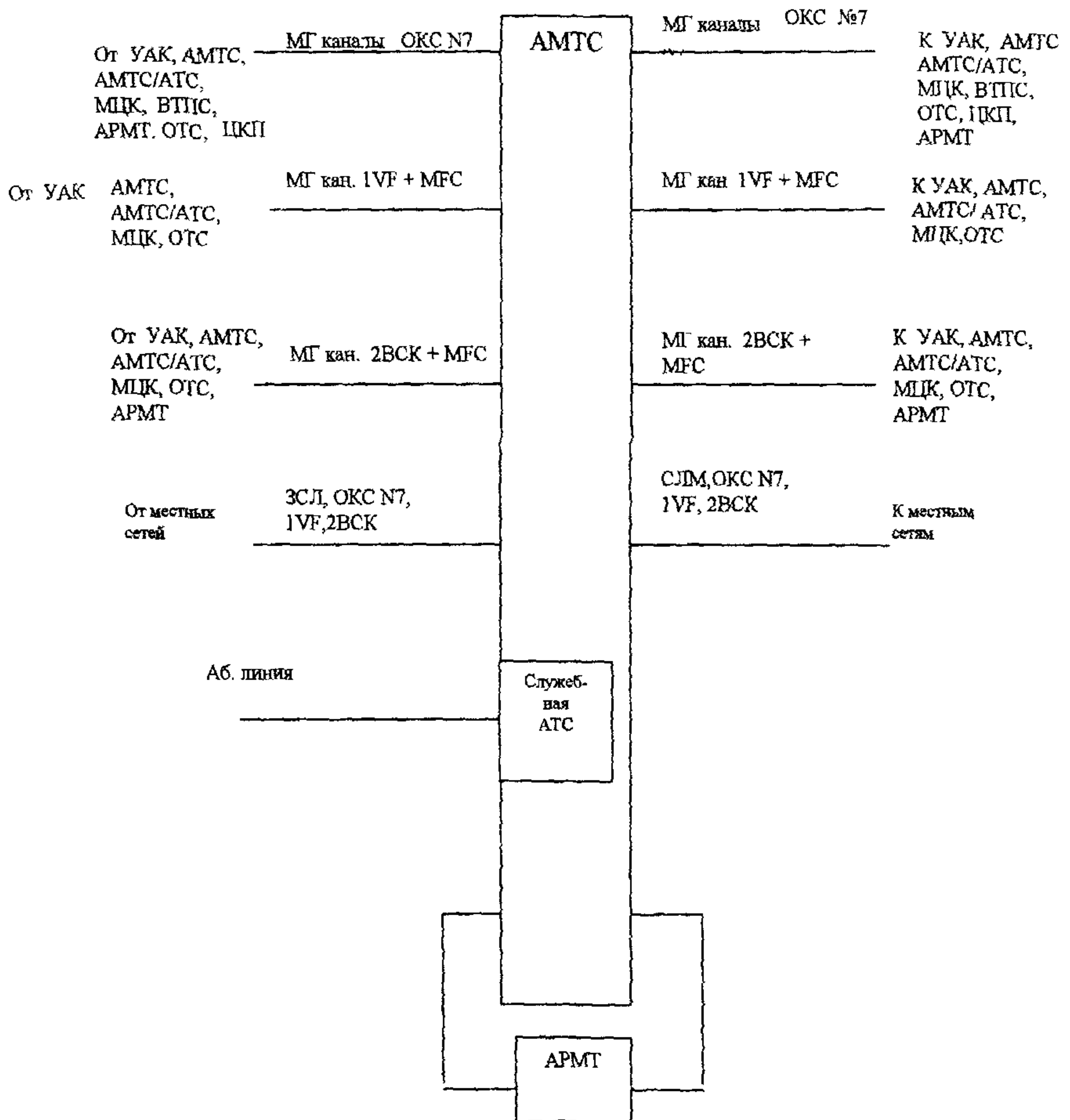
Рисунок 4.1 - Каналы и линии, включаемые в АМТС
