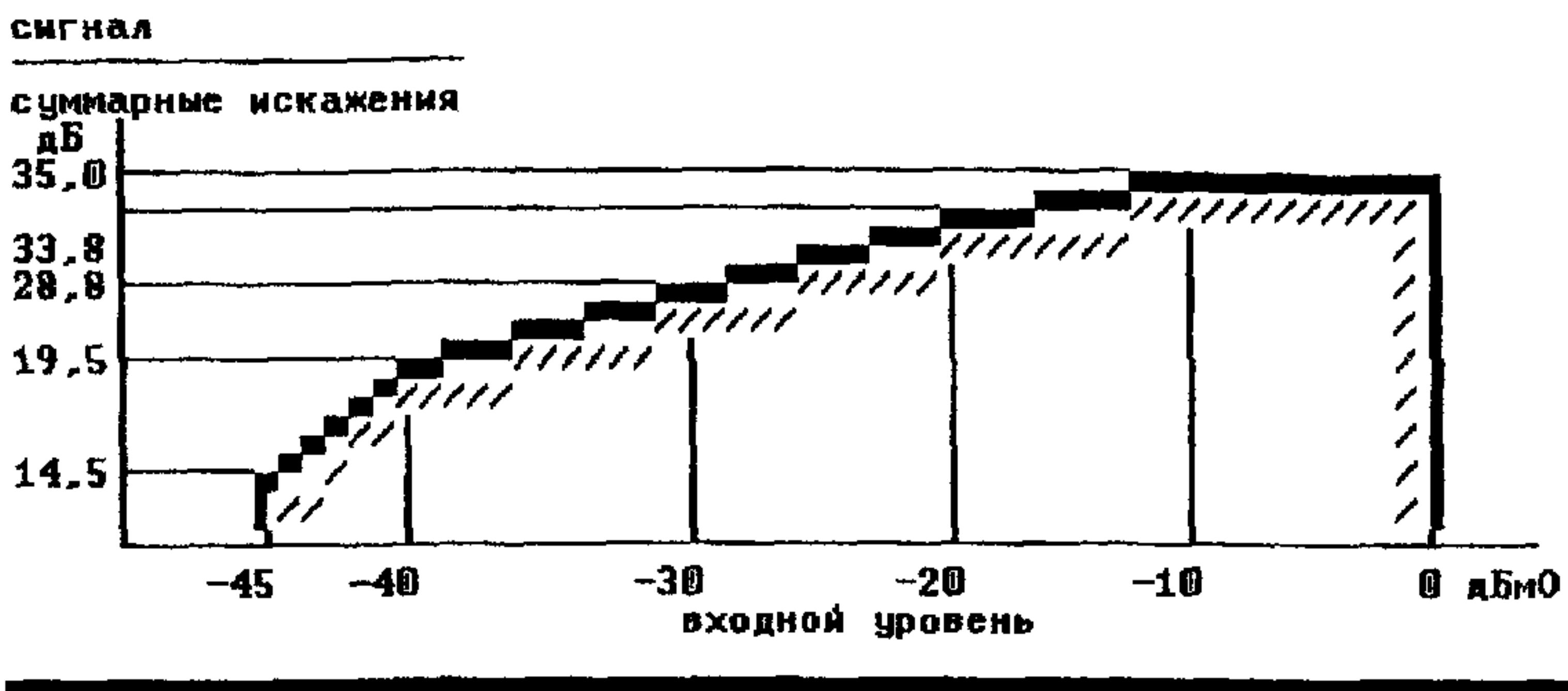
Рисунок 4 8 - Пределы суммарных искажений на входе соединения при L_1 = 0 дБ0 интерфейса Z
