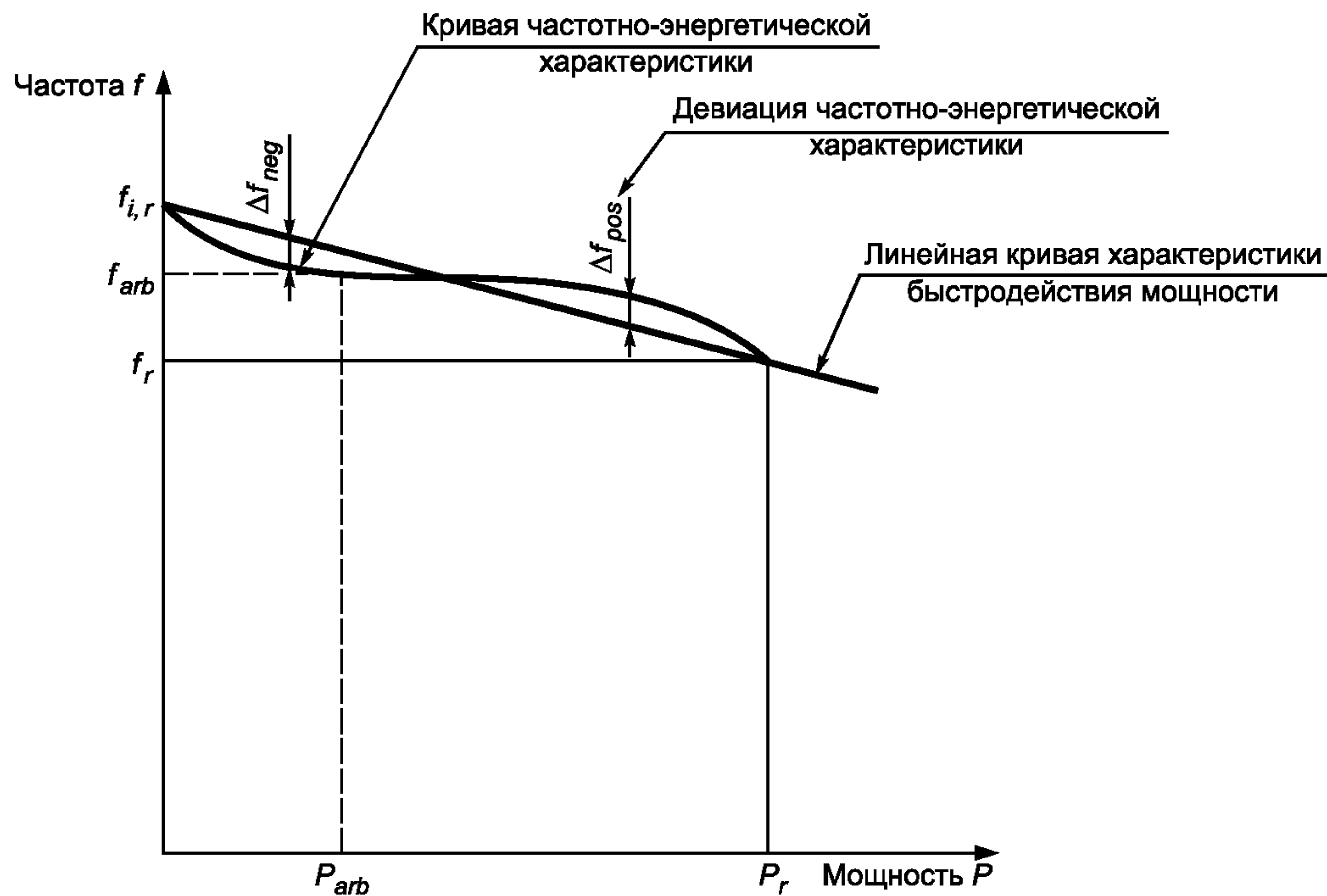
Рисунок 2 — Частотно-энергетическая характеристика отклонения от линейной кривой
