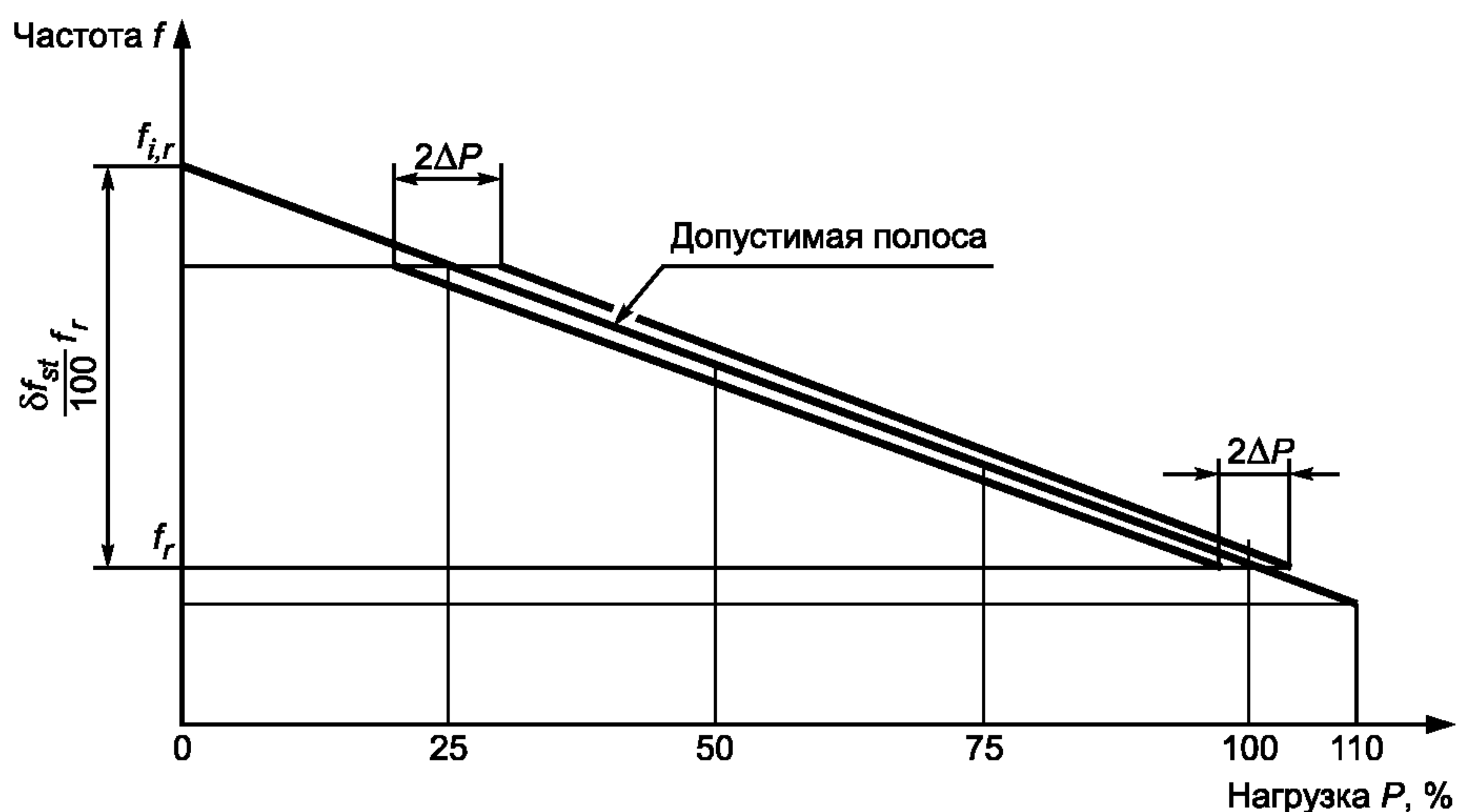
Рисунок 12 — Распределение мощности при параллельной нагрузке
