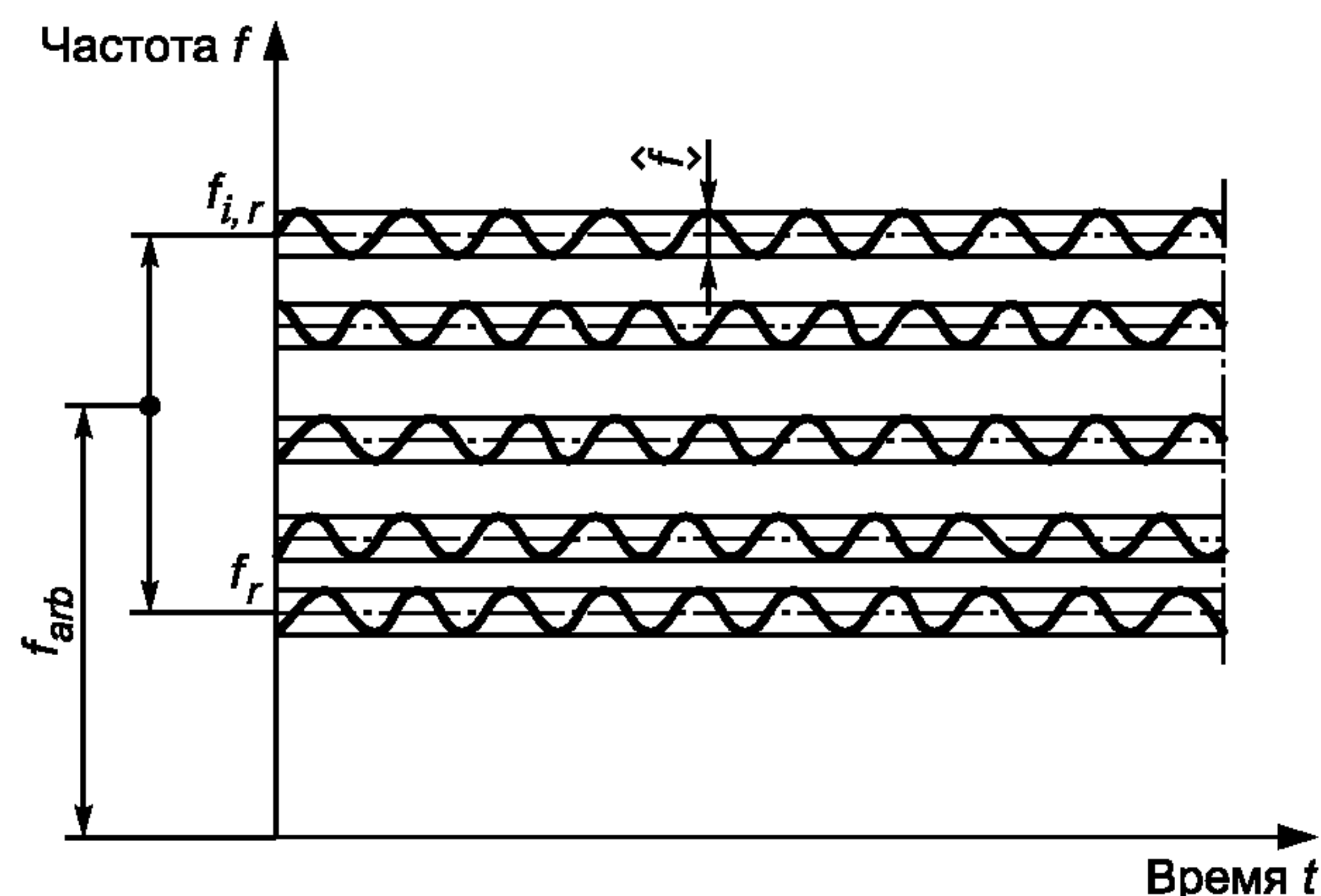
Рисунок 3 — Стабилизированная полоса частот
