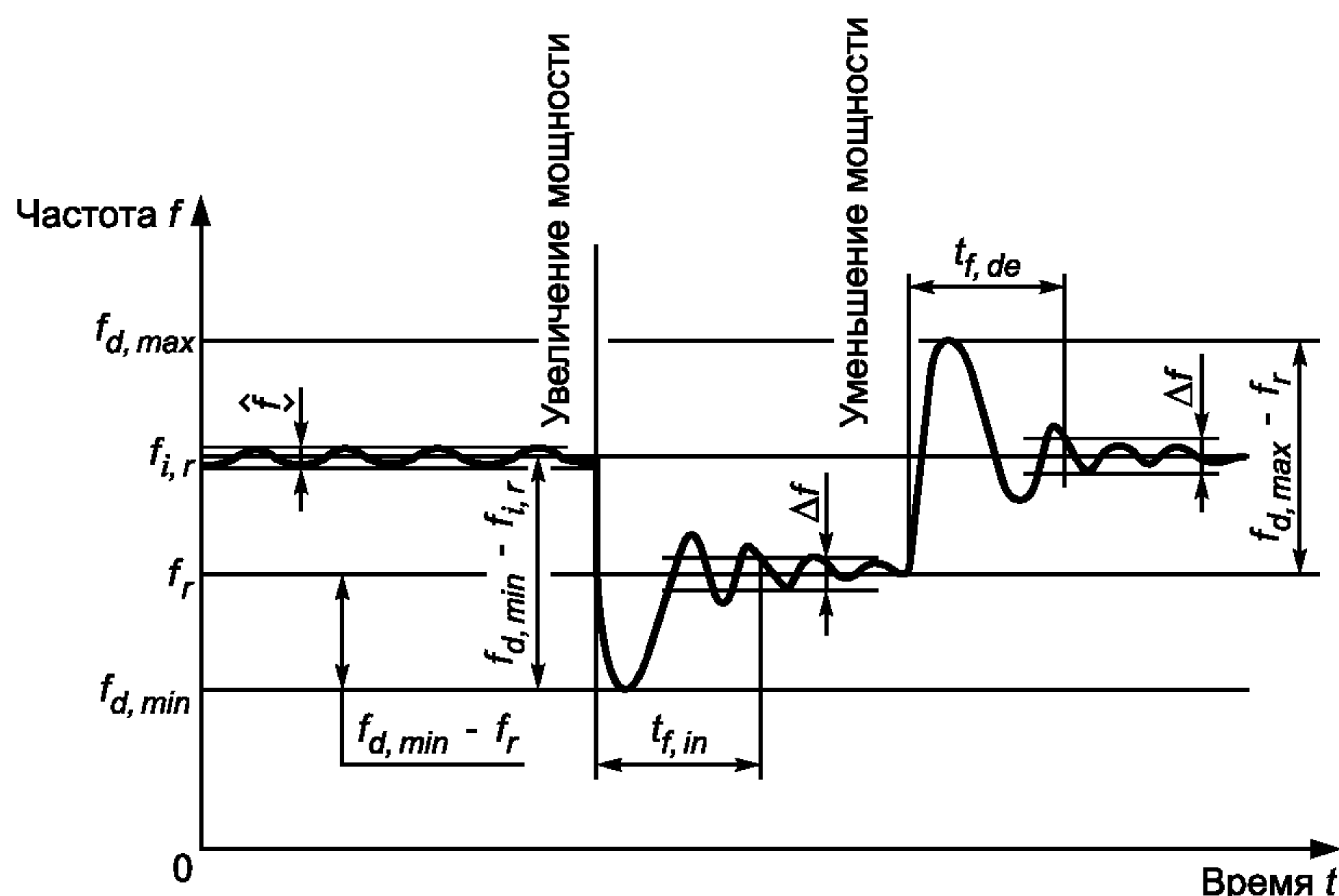
Рисунок 4 — Динамический режим частоты
