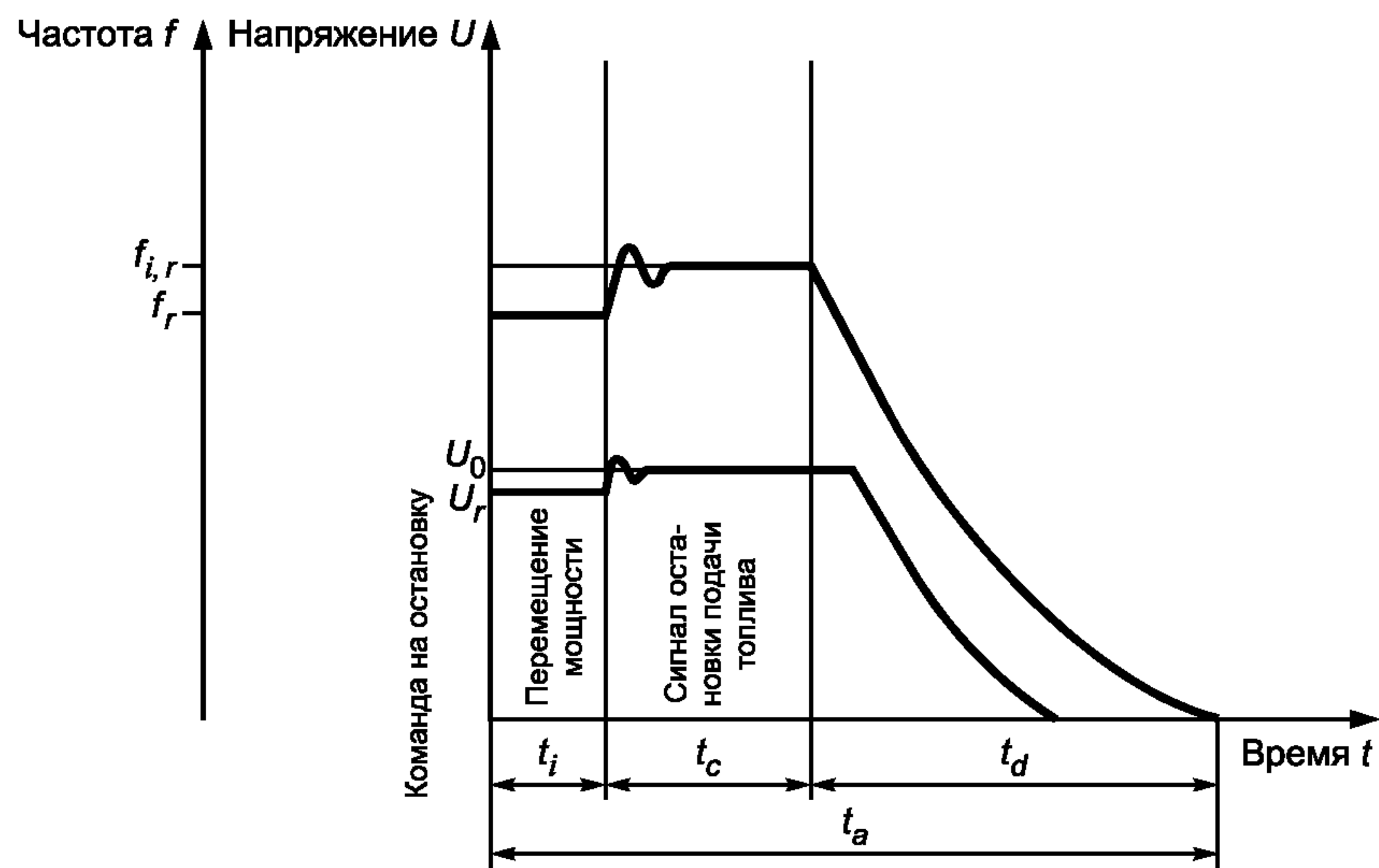
Рисунок 11 — Характеристики остановки
