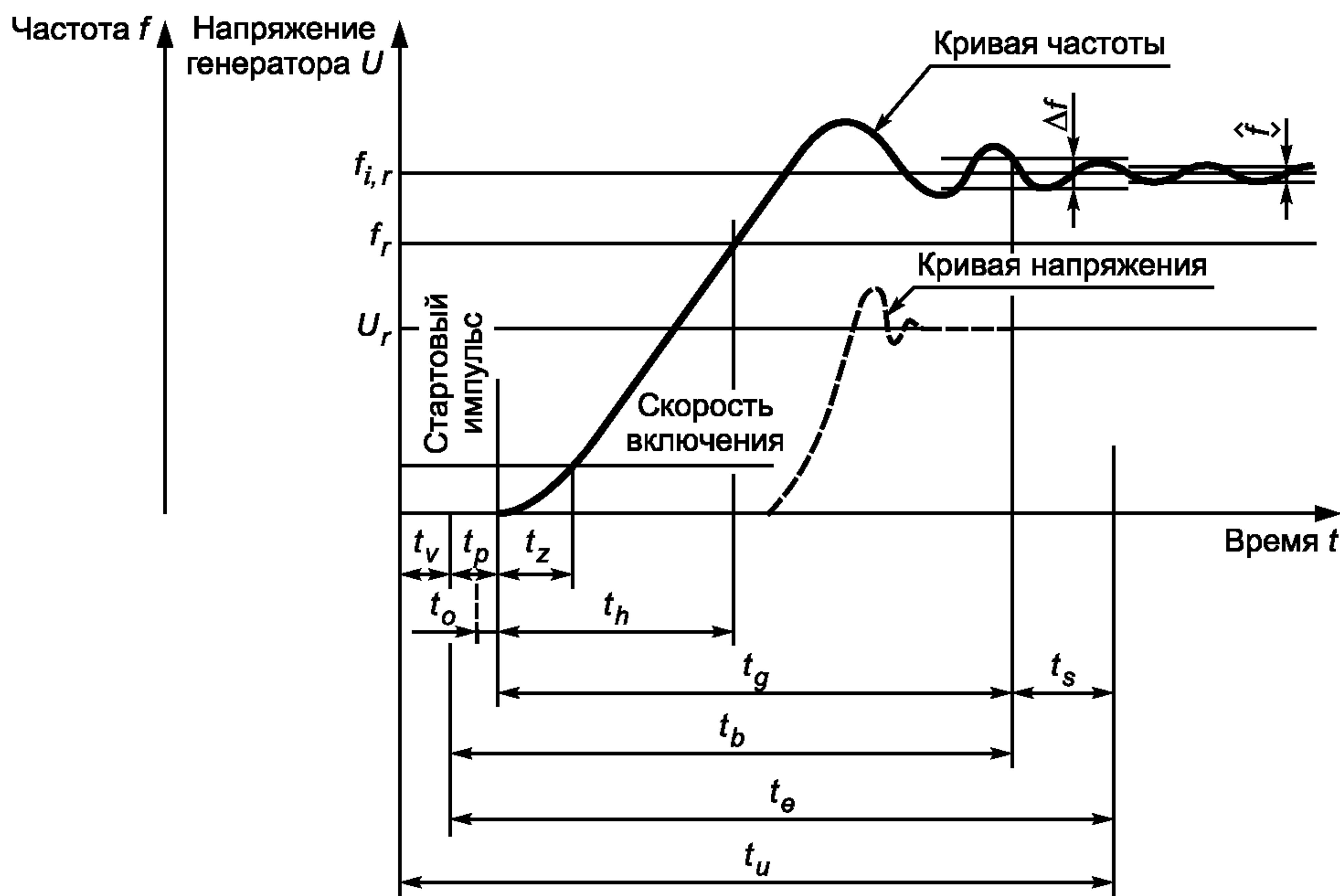
Рисунок 10 — Пусковые характеристики
