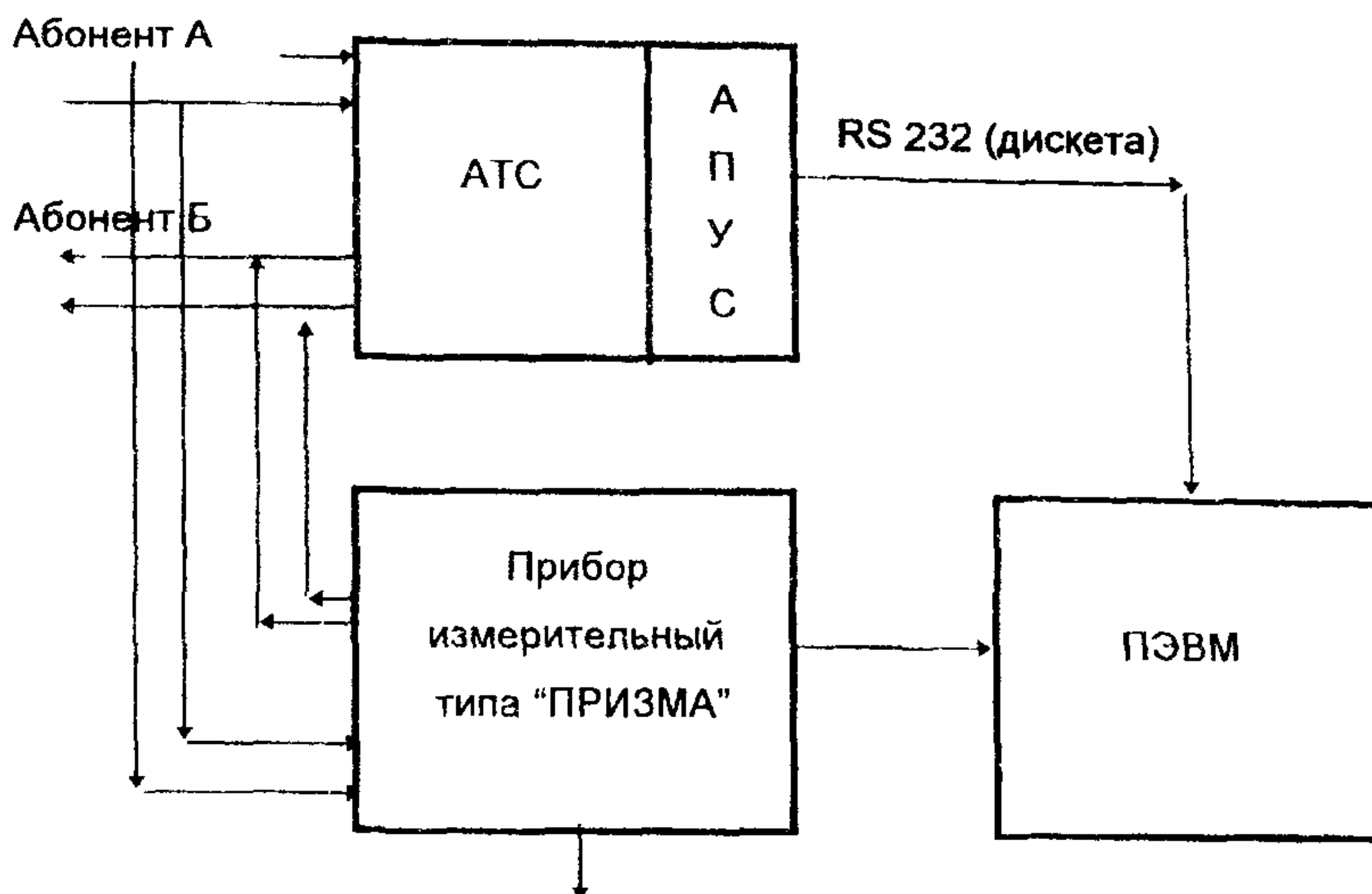
Рисунок 1. Структурная схема для исследований ИИК
