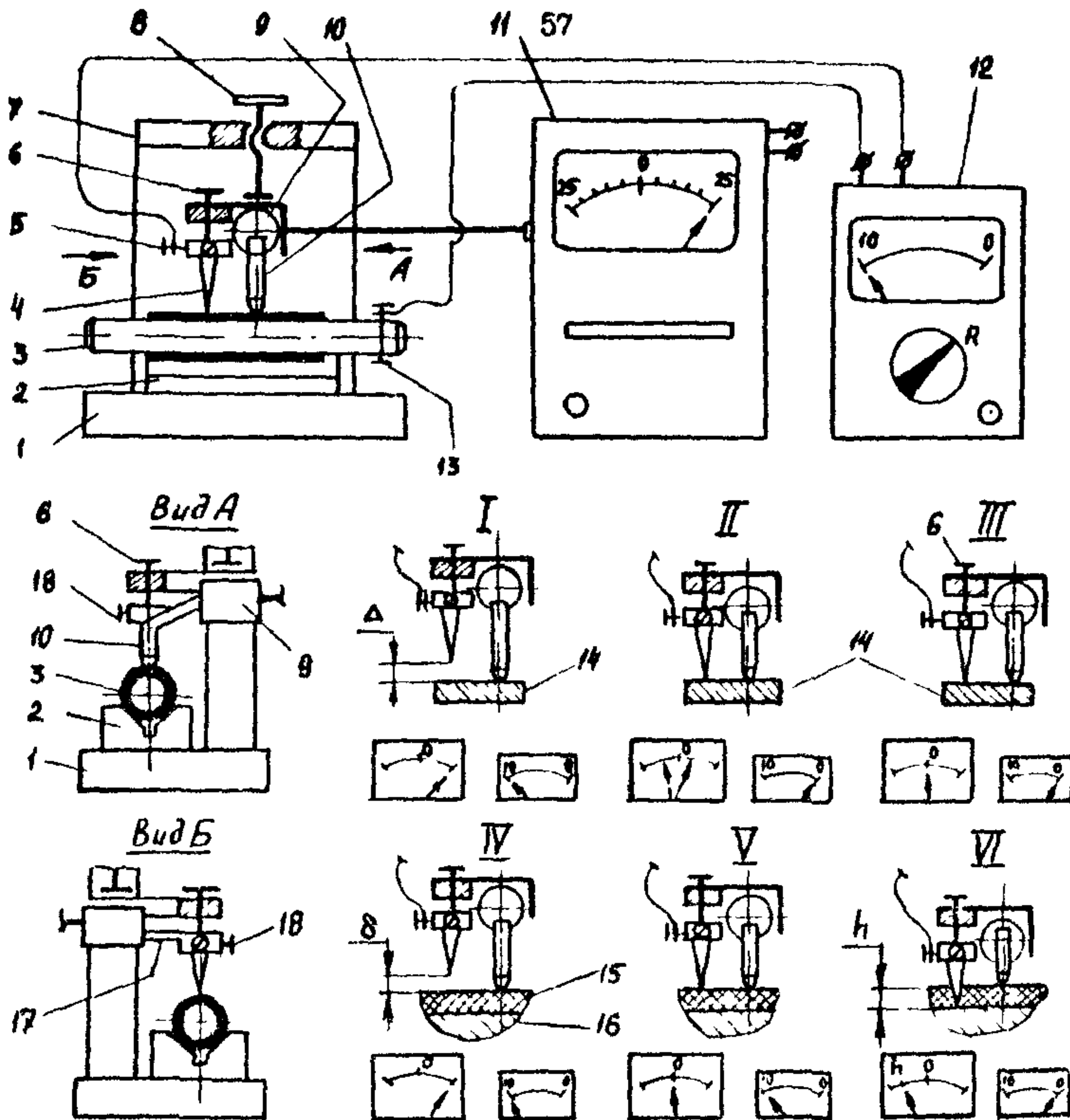
Рис. 14. Схема прибора ИТ-1 для измерения толщины покрытия и принцип его работы:
