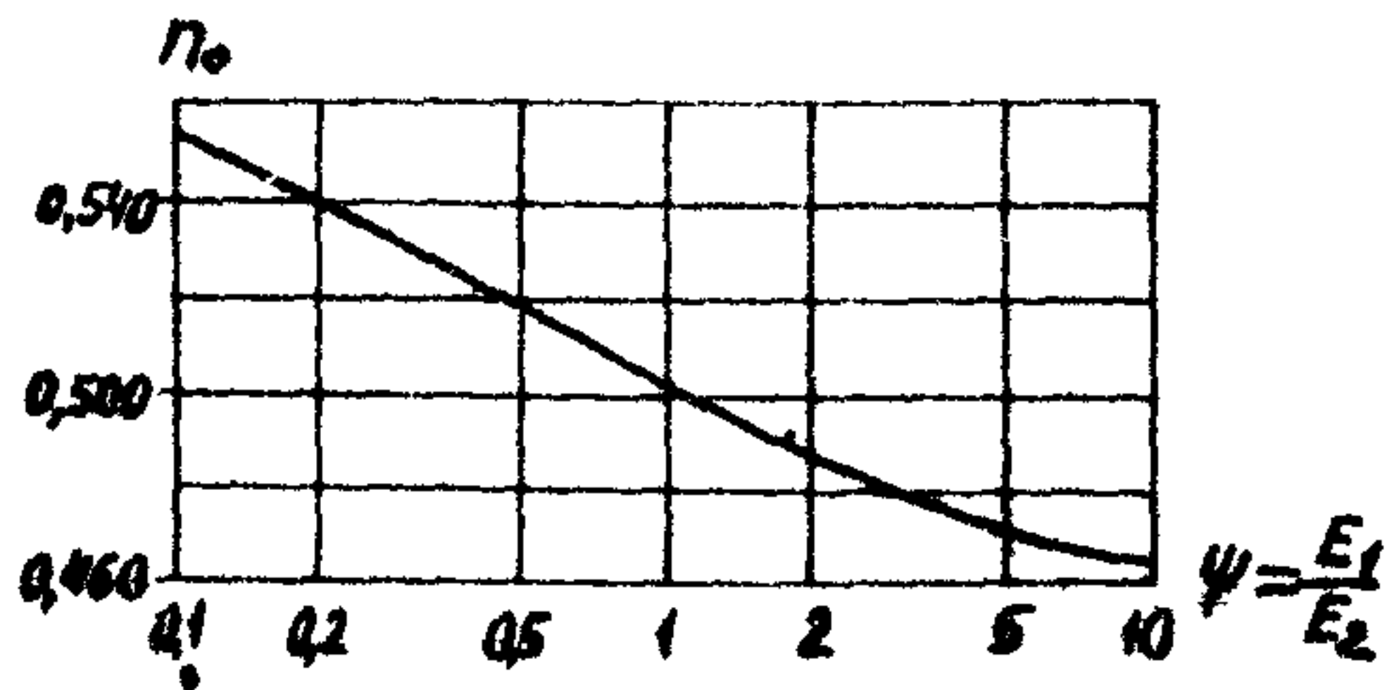
Рис. 9. Зависимость n_0 от \psi
