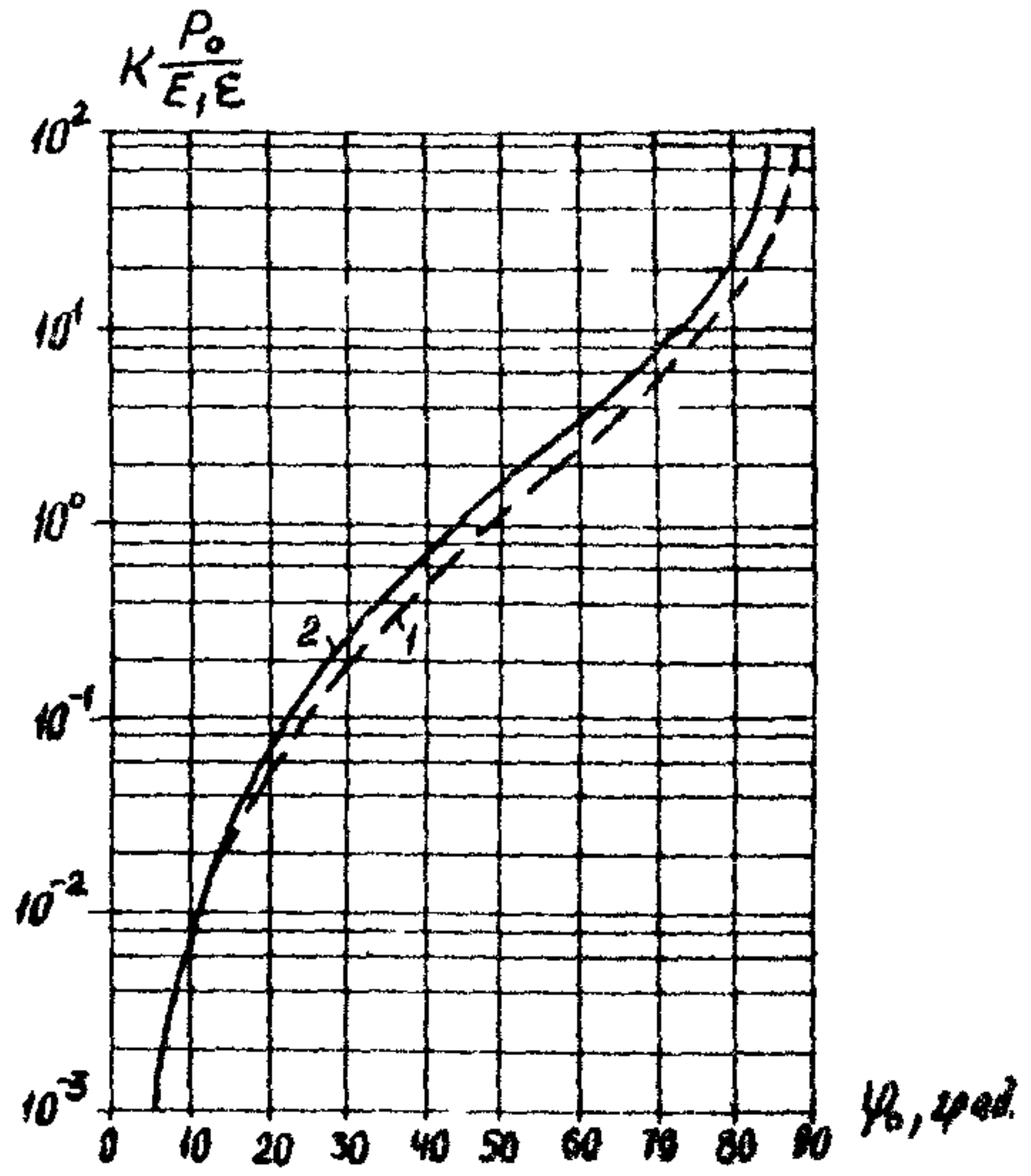
Рис. 8. График функций: \psi(\psi_0) = K \frac{P_0}{E_1 E} - кривая 1 и \psi_1(\psi_0) = K \frac{P_0}{E_1 E} - кривая 2
