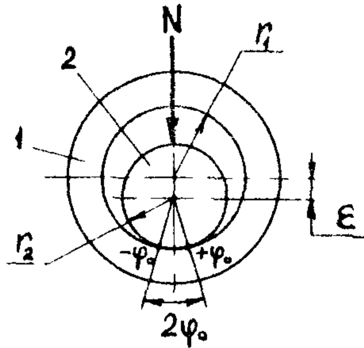
Рис. 7. Схема контакта вала и втулки: 1 – втулка; 2 – вал.
