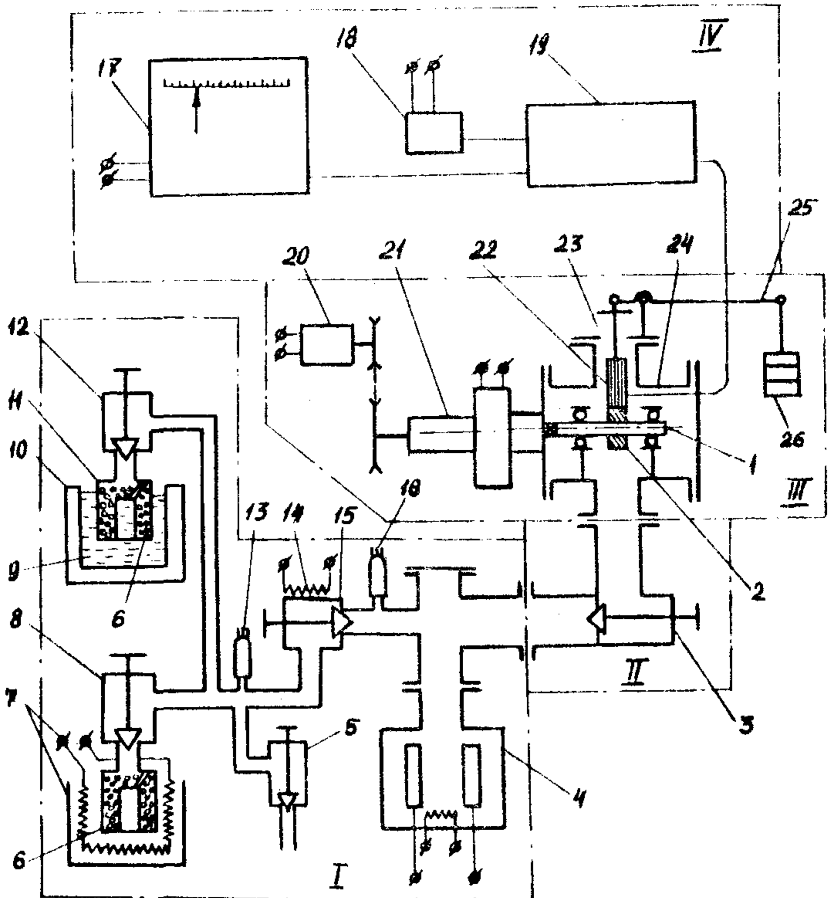
Рис. I Типовая схема установки серия "Трибовак":
