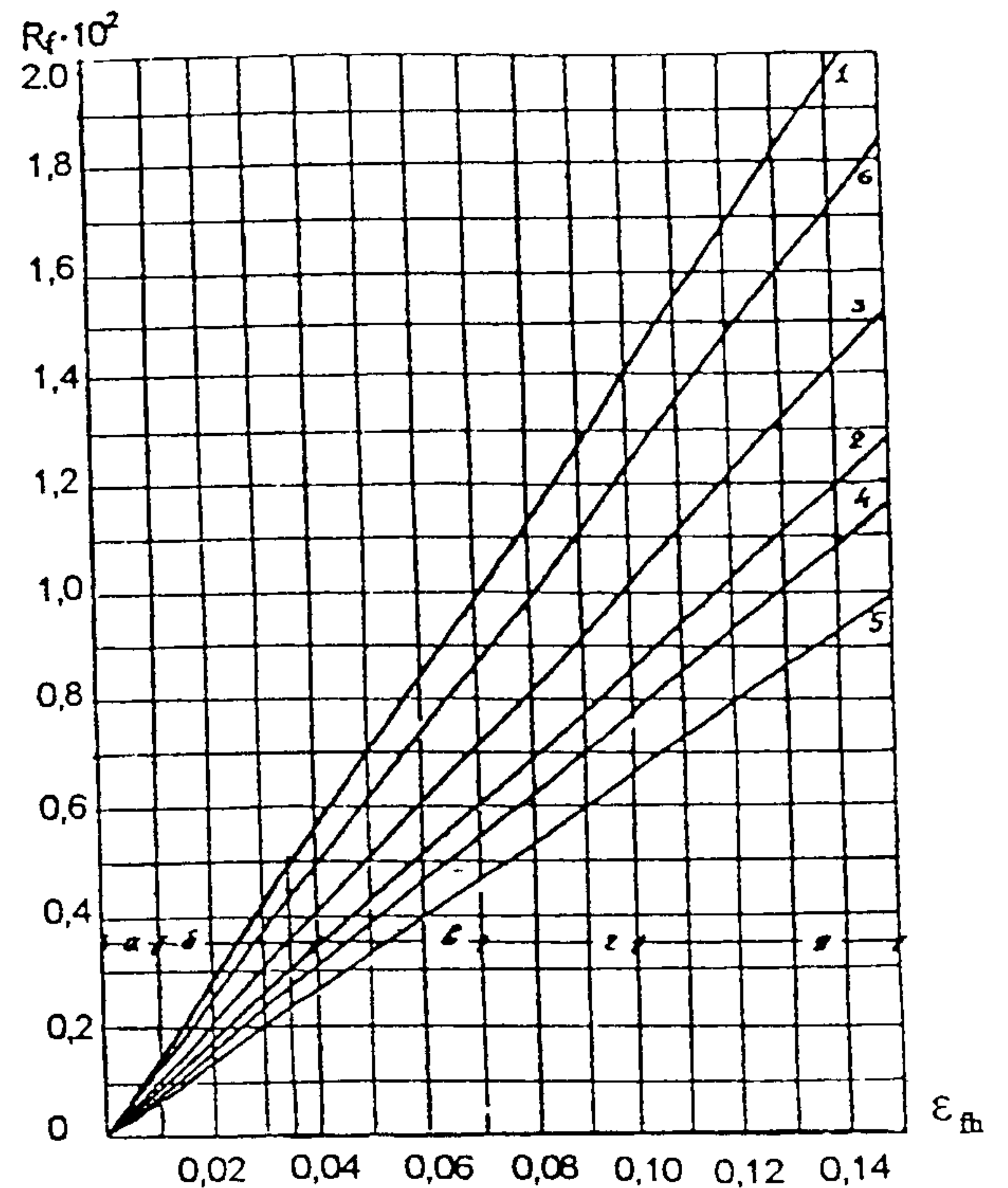
Рис.1. Зависимость относительной деформации пучения \varepsilon_{fb} от параметра R_f :
