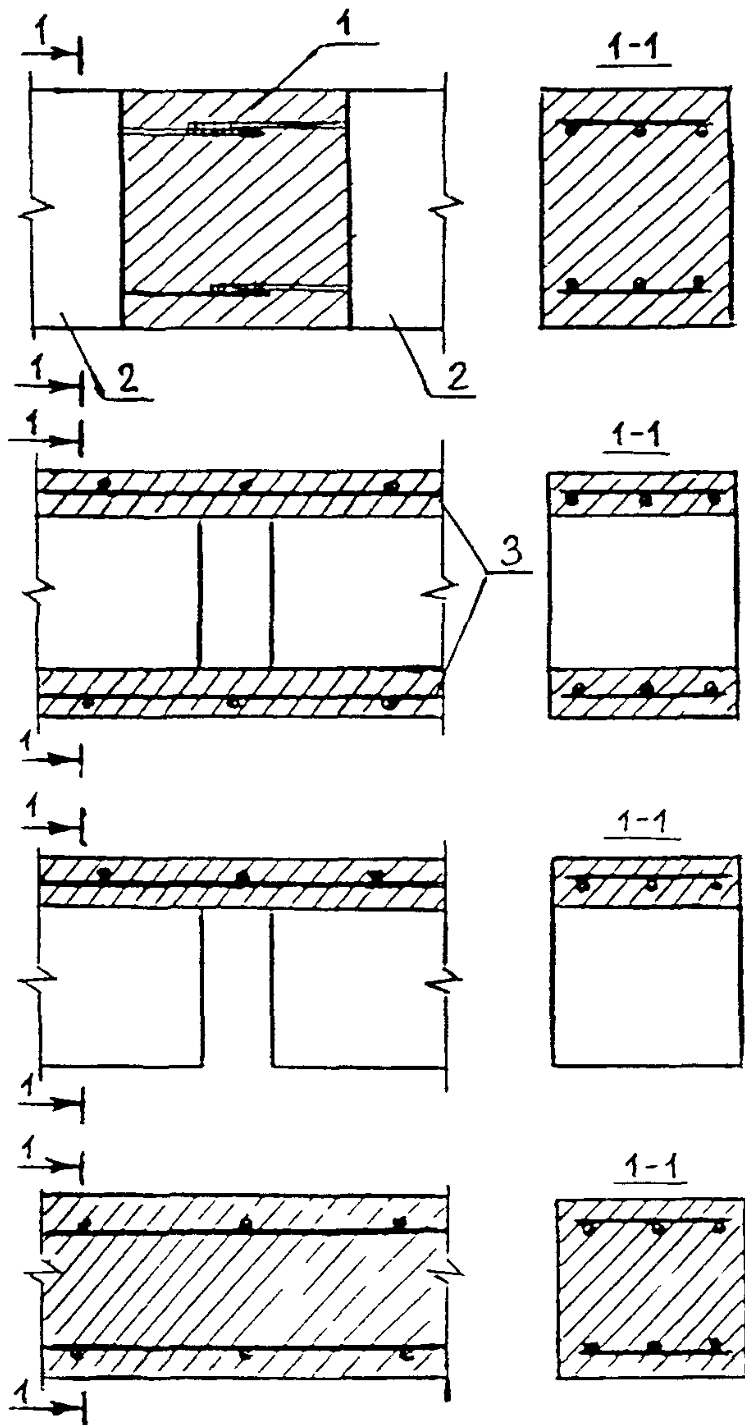
Рис.1 Конструктивные решения соединений элементов мелкозаглубленных ленточных фундаментов
