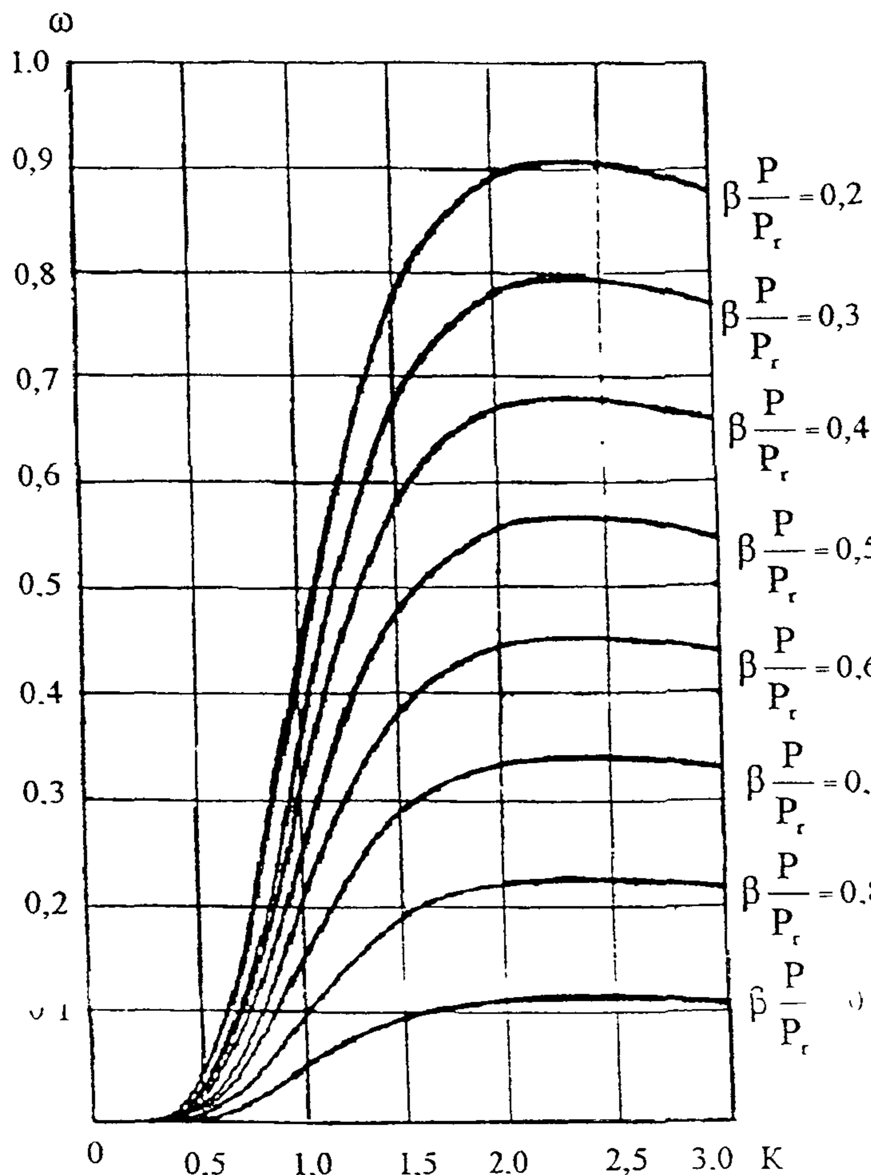
Рис.3. Зависимость \omega от K при разных значениях \frac{\beta P}{P_r} .
