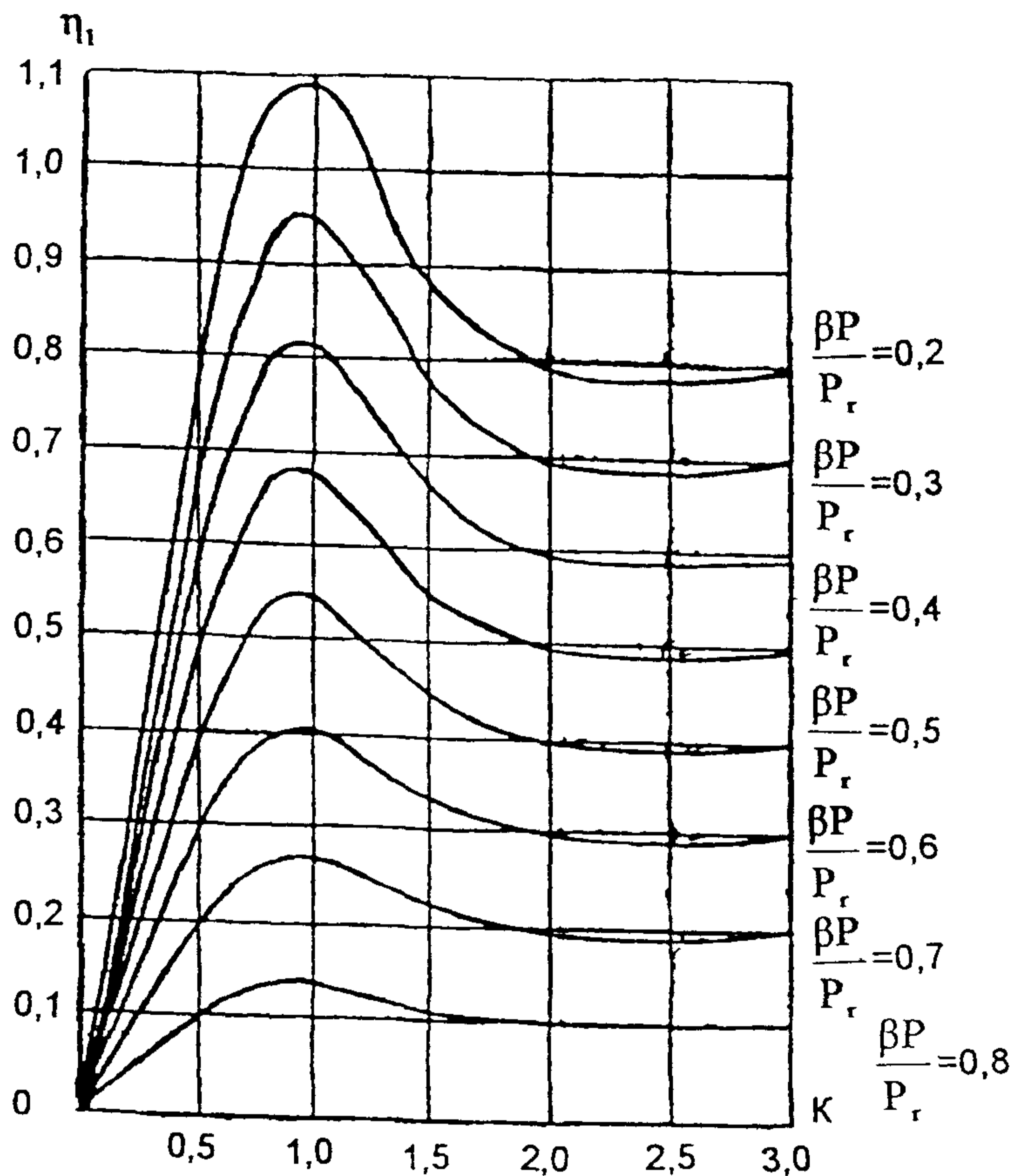
Рис. 5. Зависимость \eta_1 от K при разных значениях \frac{\beta P}{P_r} .
