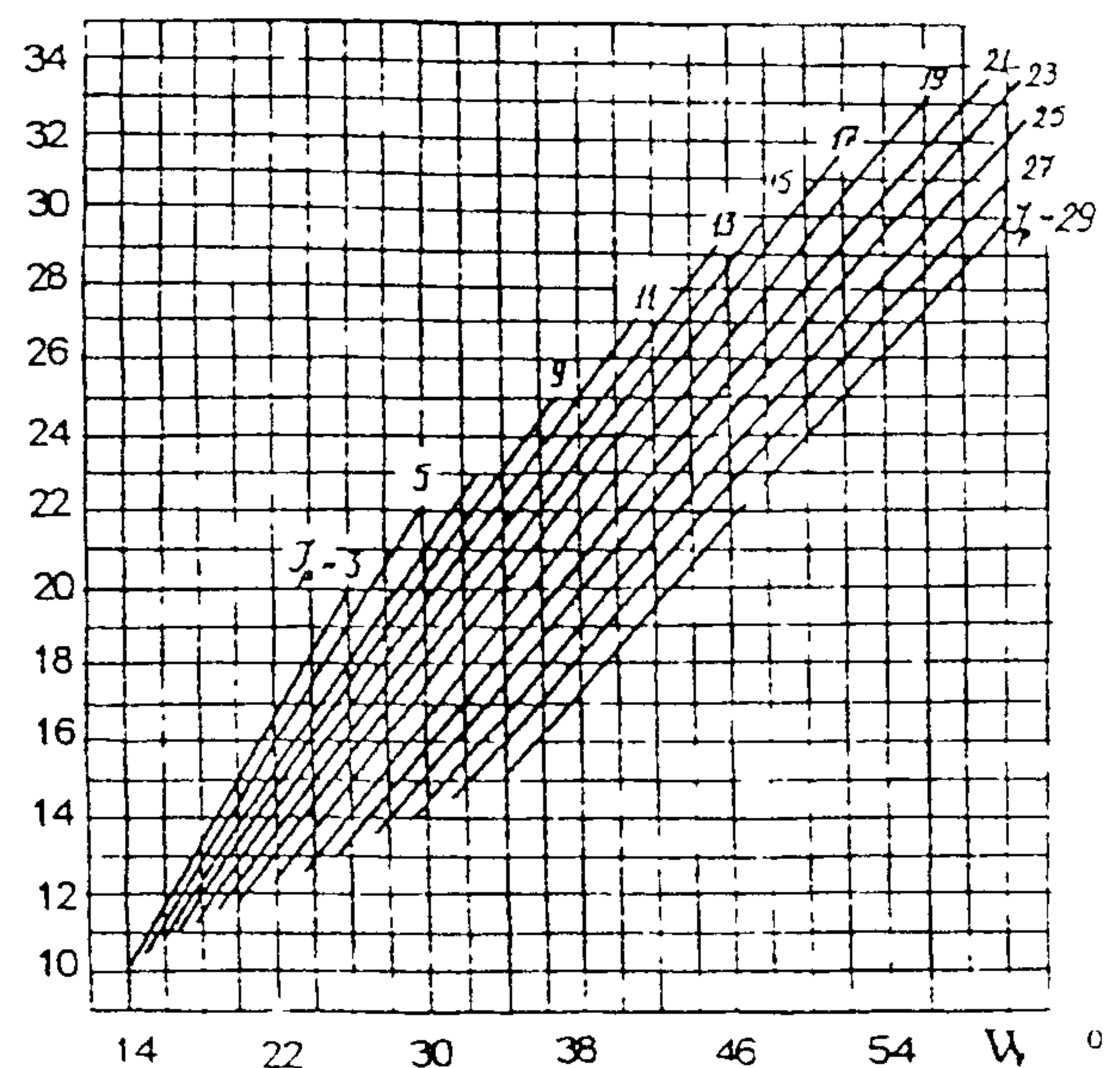
Рис.2. Зависимость критической влажности W_{cr} от числа пластичности J_p и предела текучести грунта W_L
