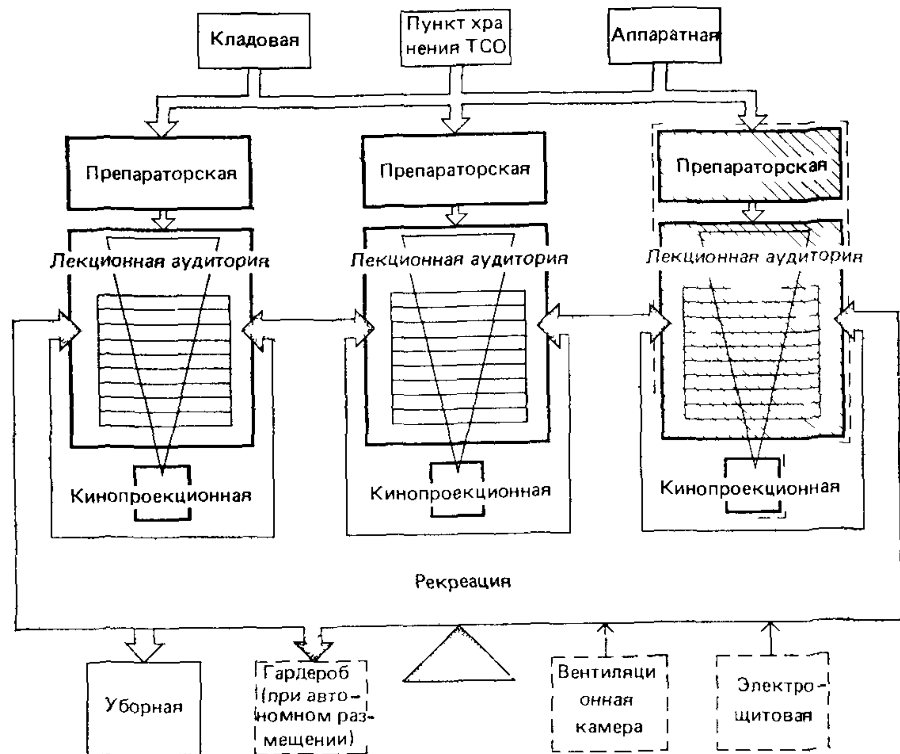
СХЕМА ФУНКЦИОНАЛЬНЫХ ЗОН ЛЕКЦИОННОЙ АУДИТОРИИ
