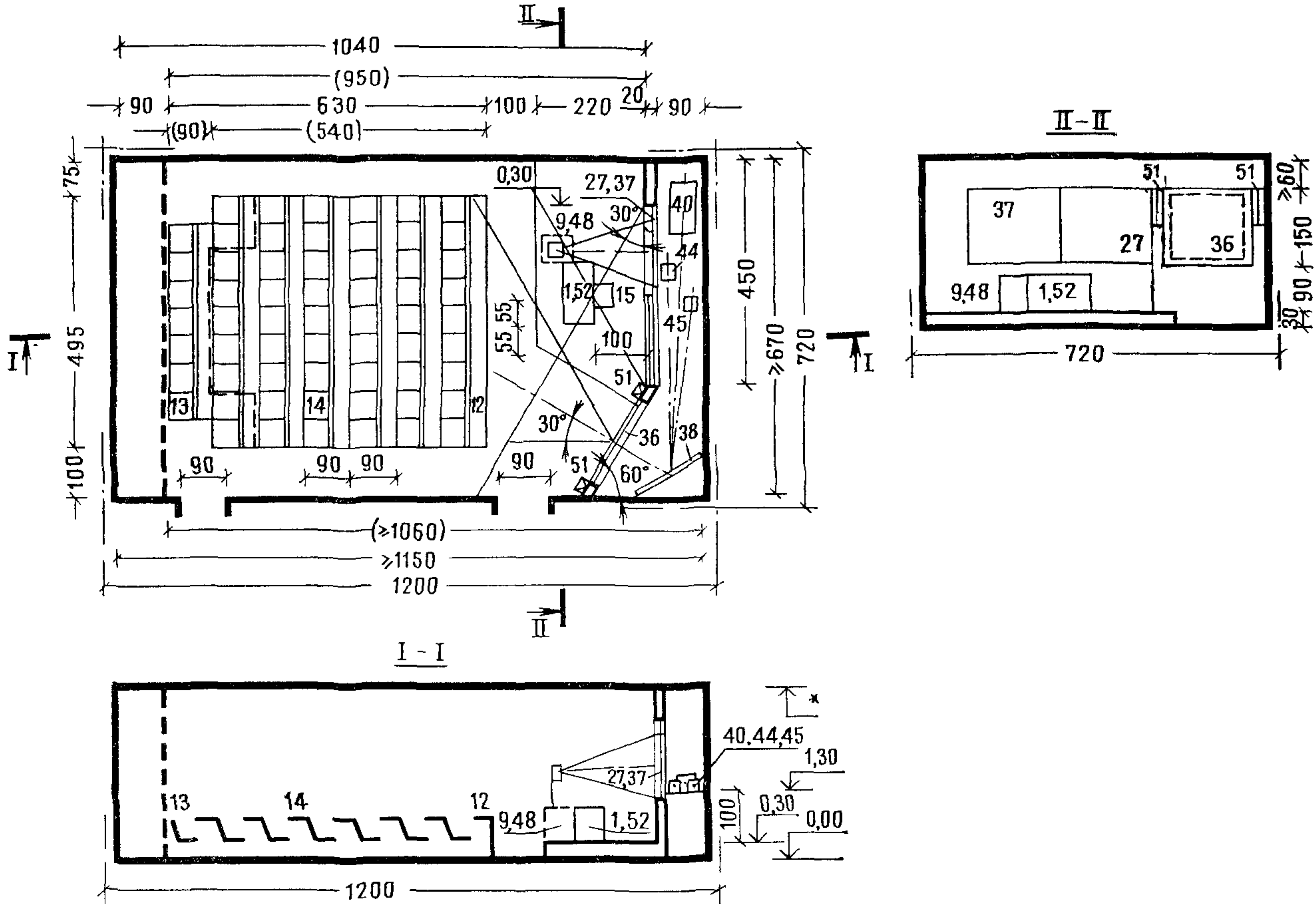
АУДИТОРИЯ НА 60 МЕСТ С ПРОЕКЦИЕЙ НА ПРОСВЕТ
