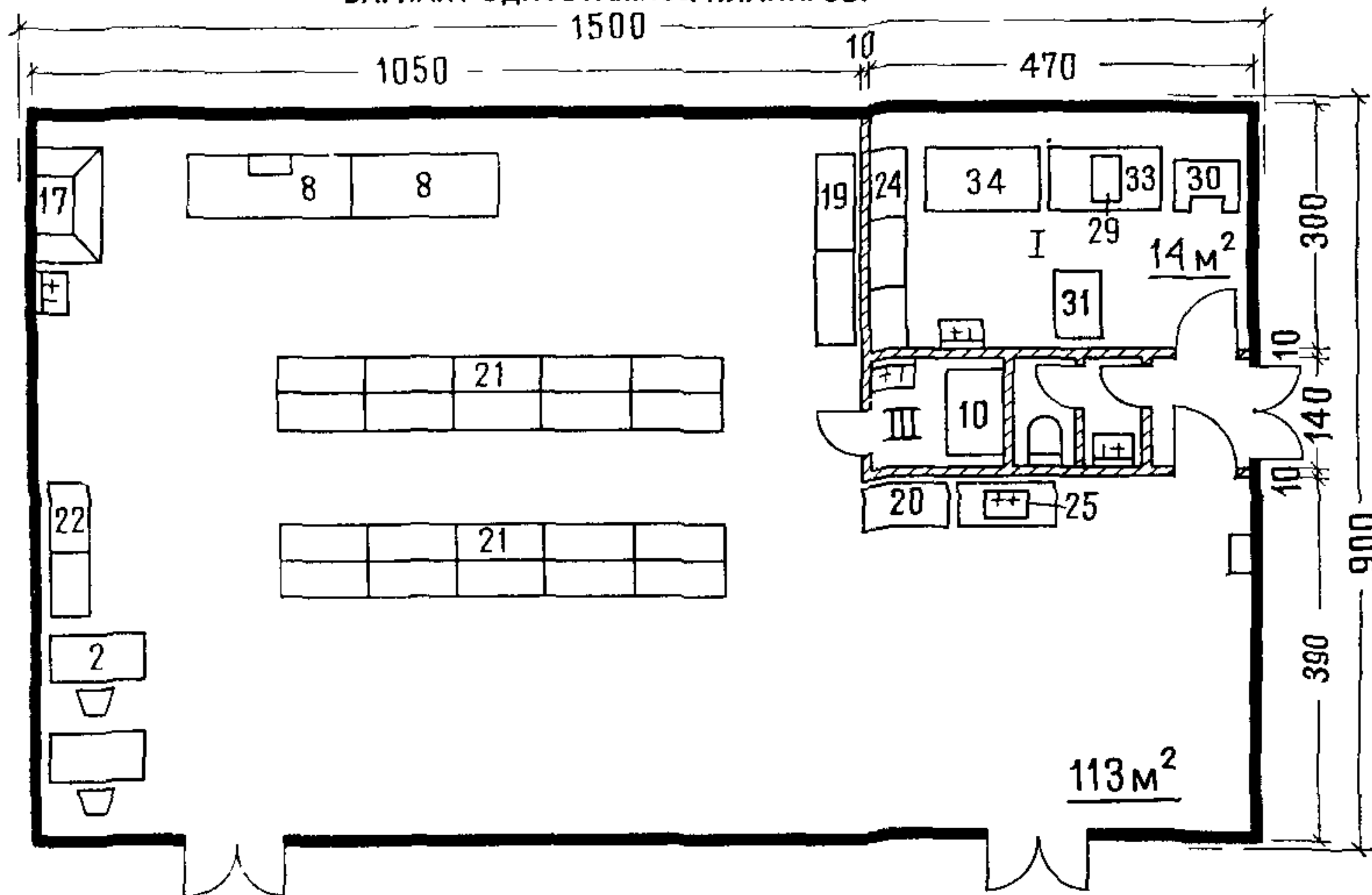
ВАРИАНТ ОДНОЭТАЖНОЙ ПЛАНИРОВКИ
