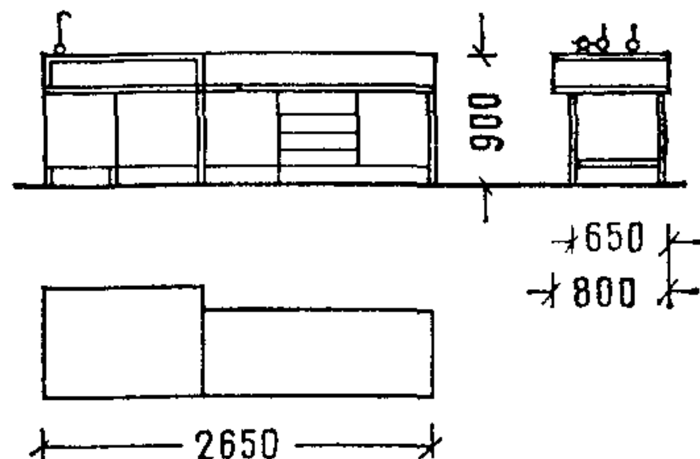
3 СТОЛ ДЕМОСТРАЦИОННЫЙ ДЛЯ ХИМИЧЕСКИХ АУДИТОРИЙ
