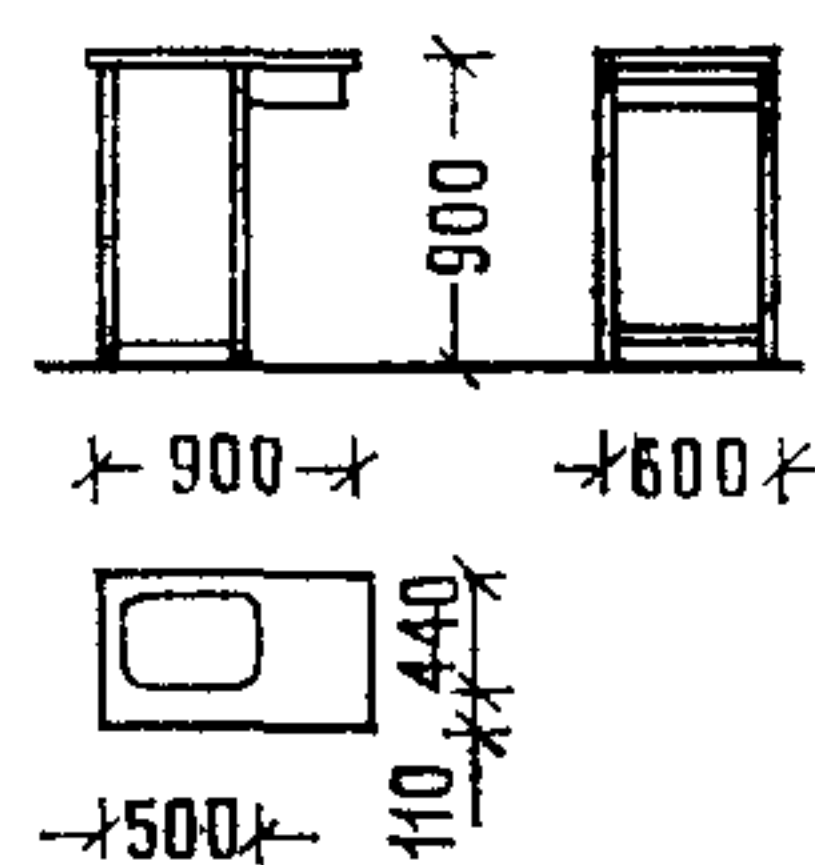
6 СТОЛ ДЛЯ ВЕСОВ
