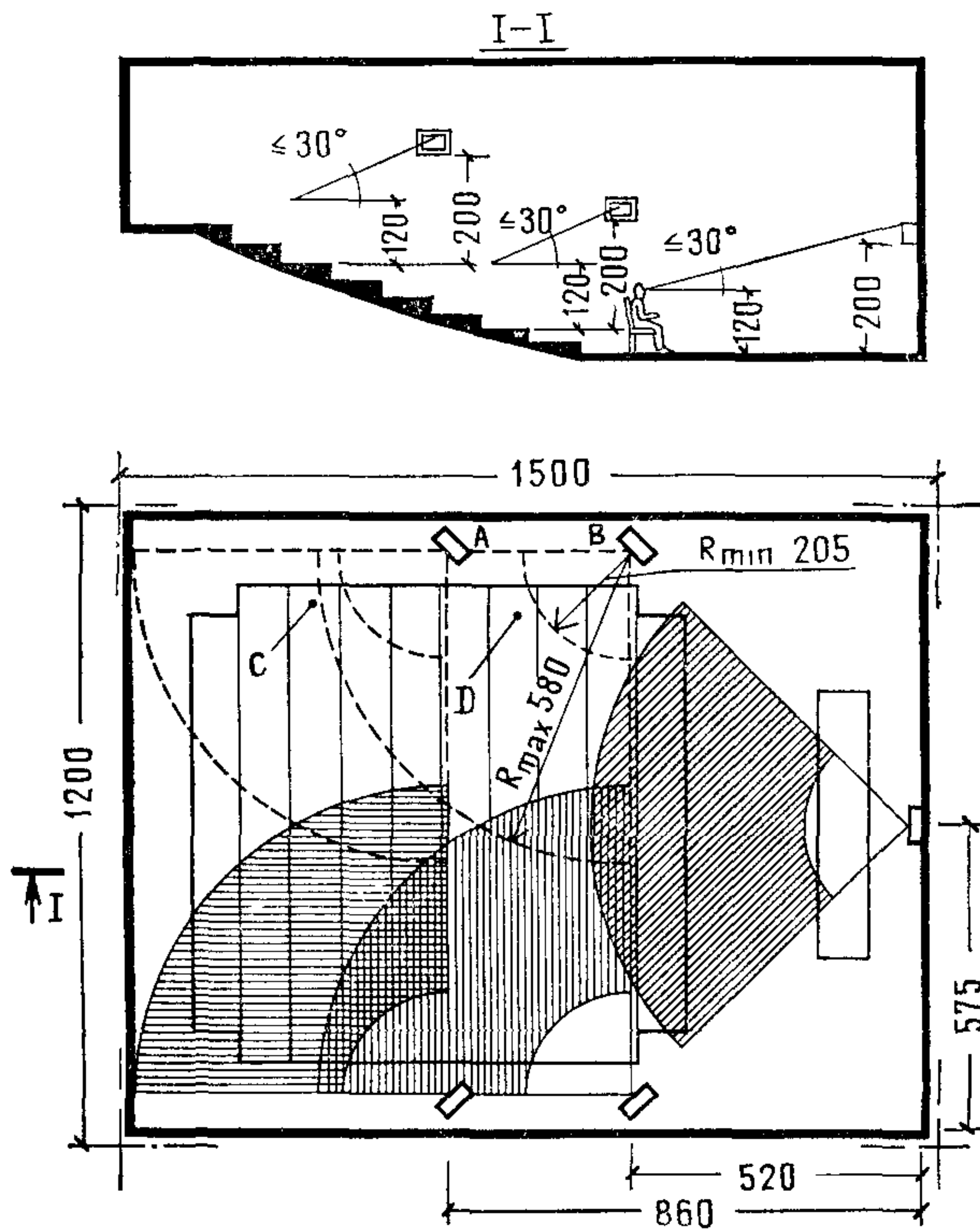
АУДИТОРИЯ РАЗМЕРОМ 12x15 м НА 150 МЕСТ
