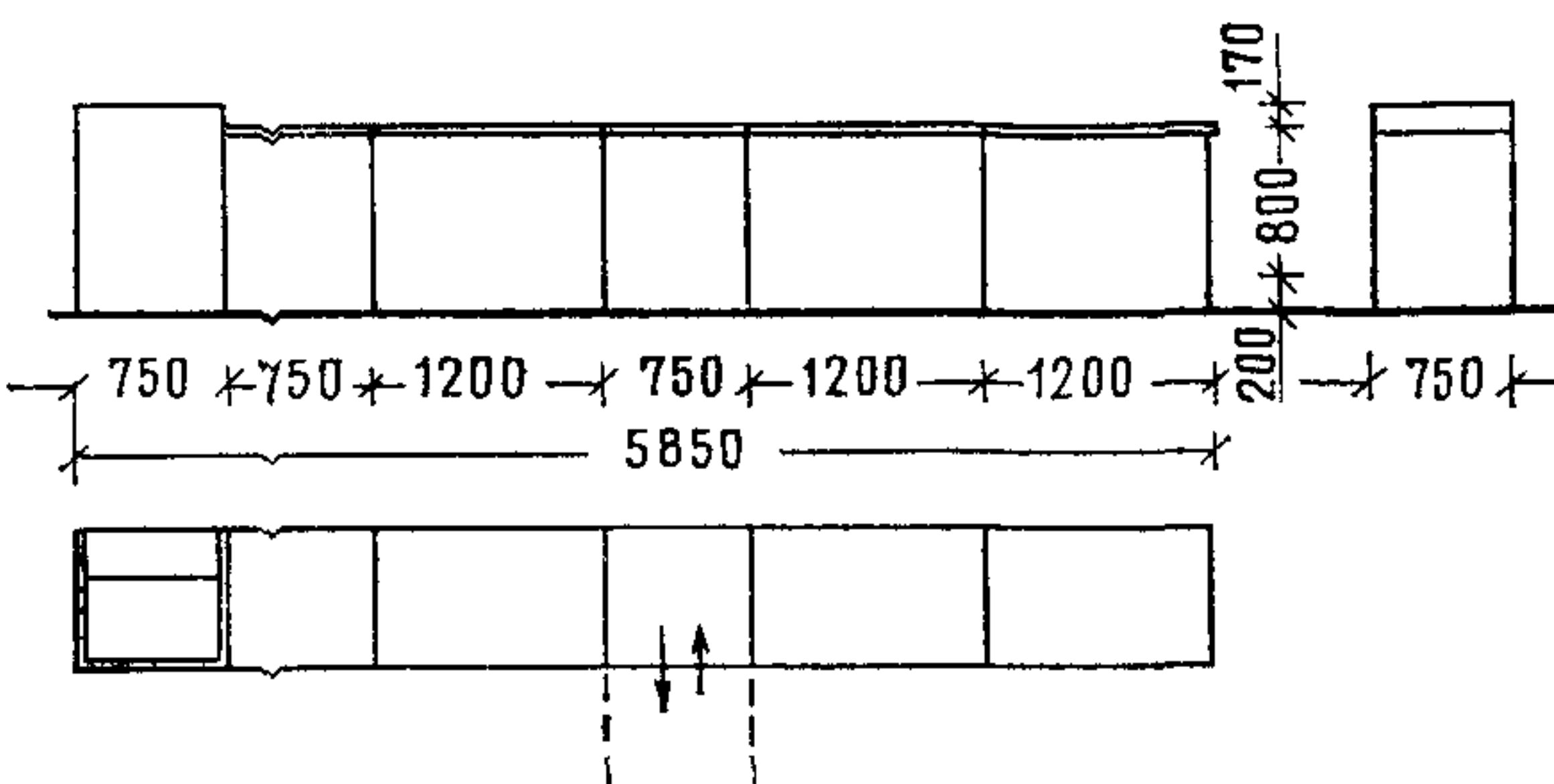
8 СТОЛ ЛАБОРАТОРНЫЙ ФИЗИЧЕСКИЙ
