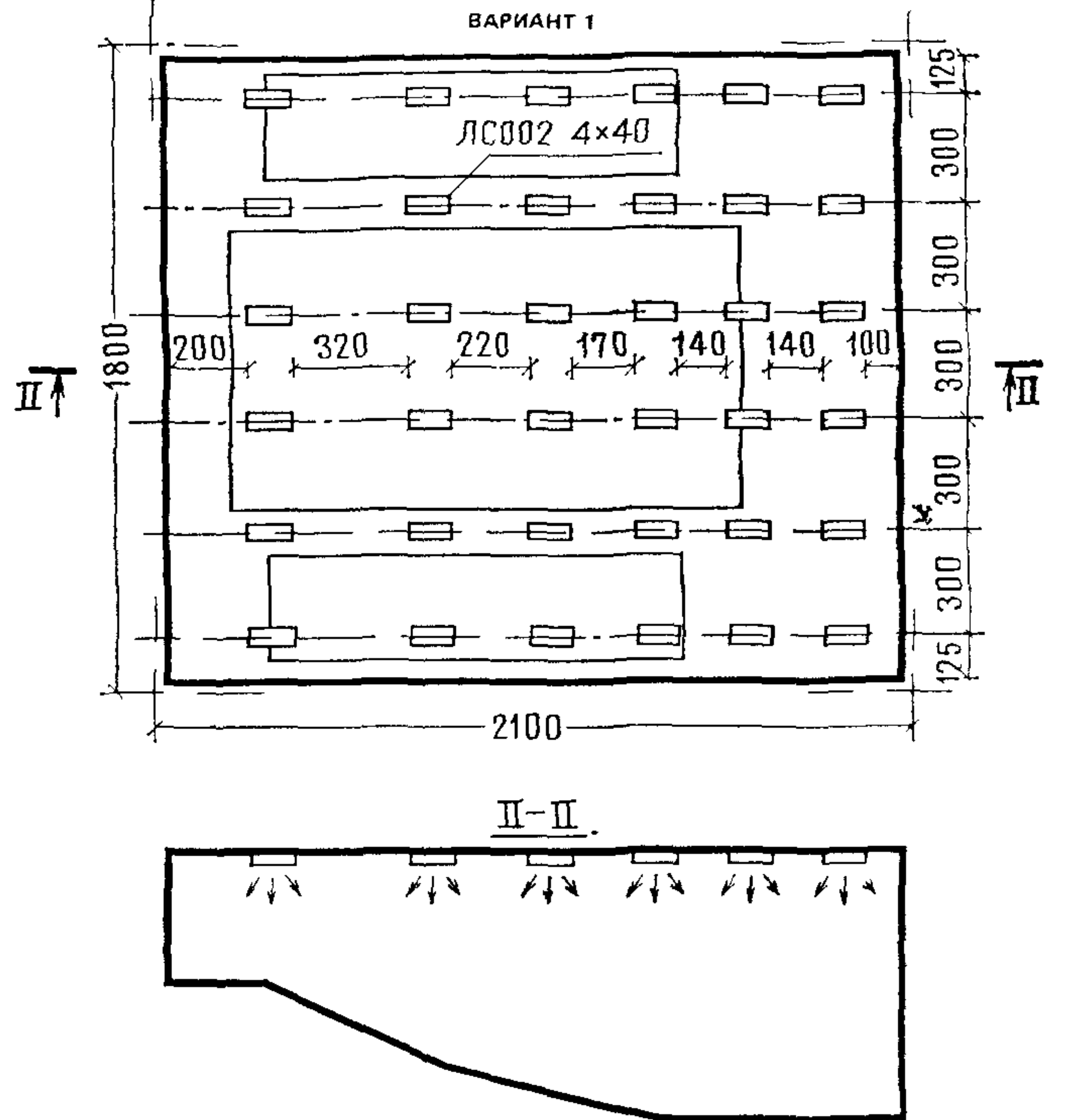
АУДИТОРИЯ РАЗМЕРОМ 18x21 м НА 350 МЕСТ
