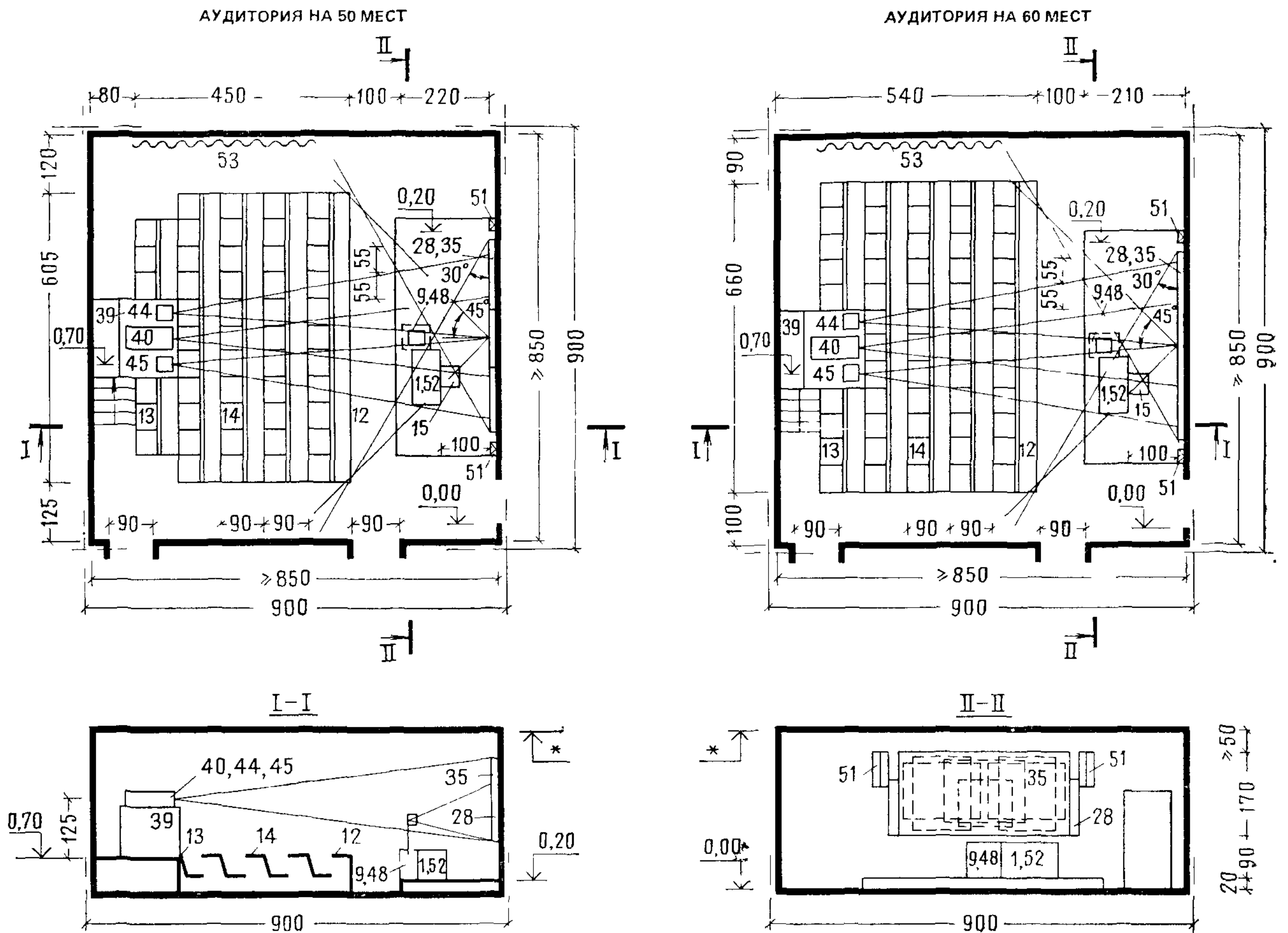
ВАРИАНТЫ РАСПОЛОЖЕНИЯ КИНОЭКРАНОВ НАД МЕЛОВОЙ ДОСКОЙ
