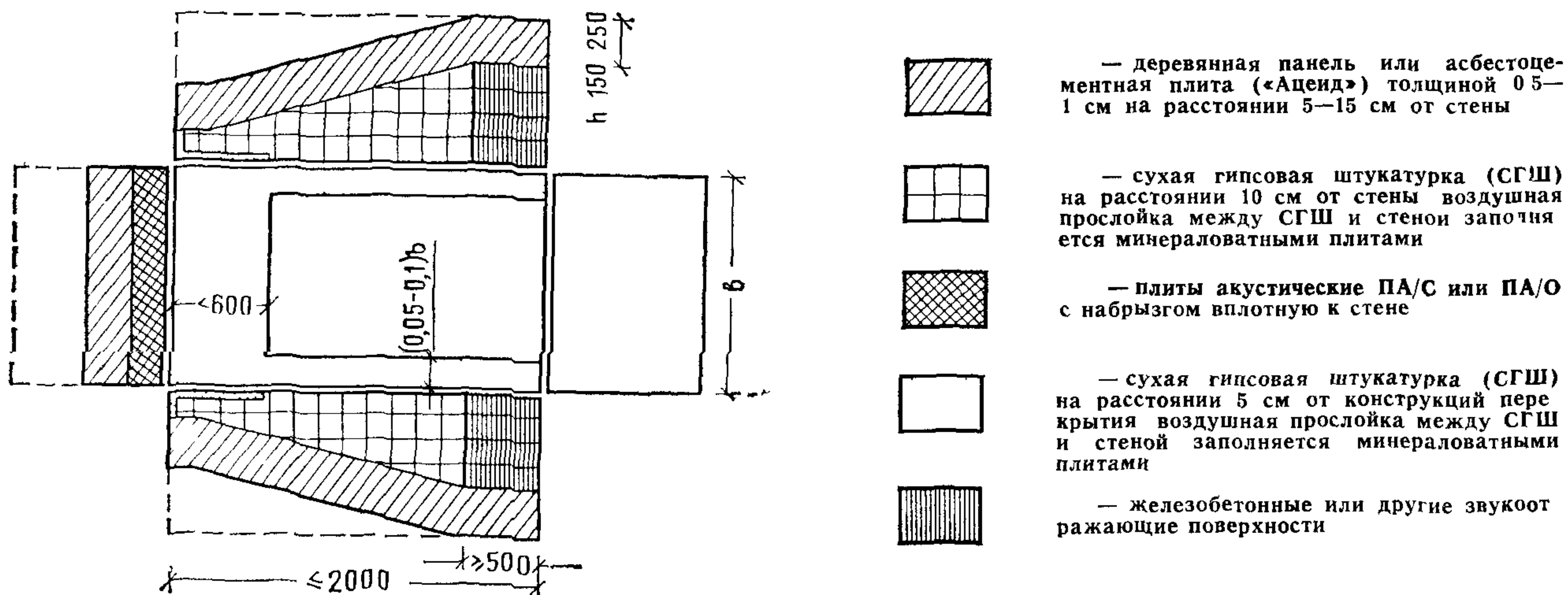
СХЕМА АКУСТИЧЕСКОЙ ОБРАБОТКИ АУДИТОРИИ
