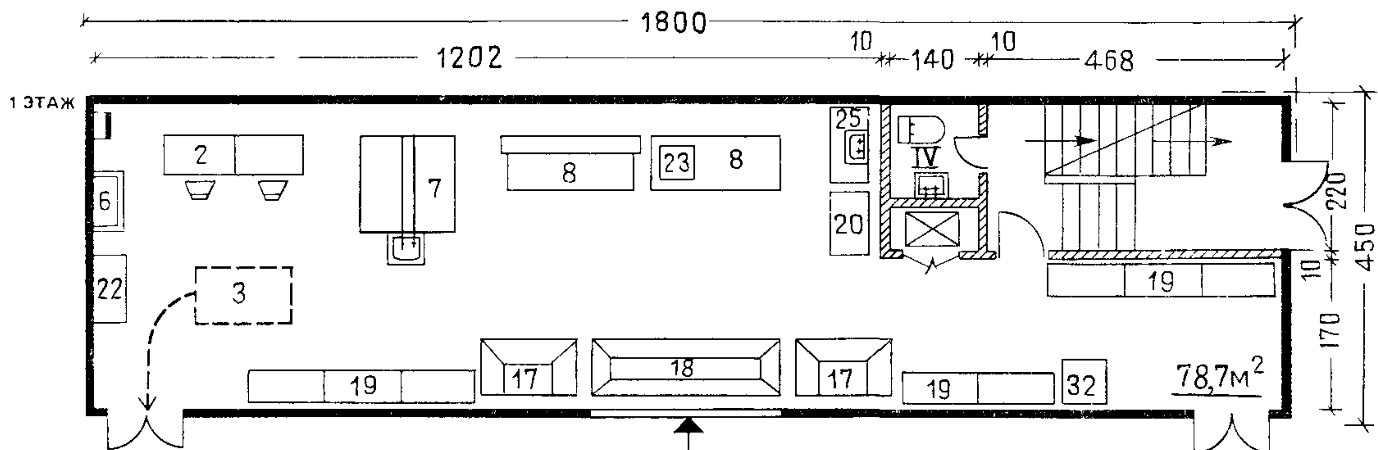
ПРЕПАРАТОРСКАЯ ХИМИИ ПРИ АУДИТОРИЯХ НА 300—350 МЕСТ
