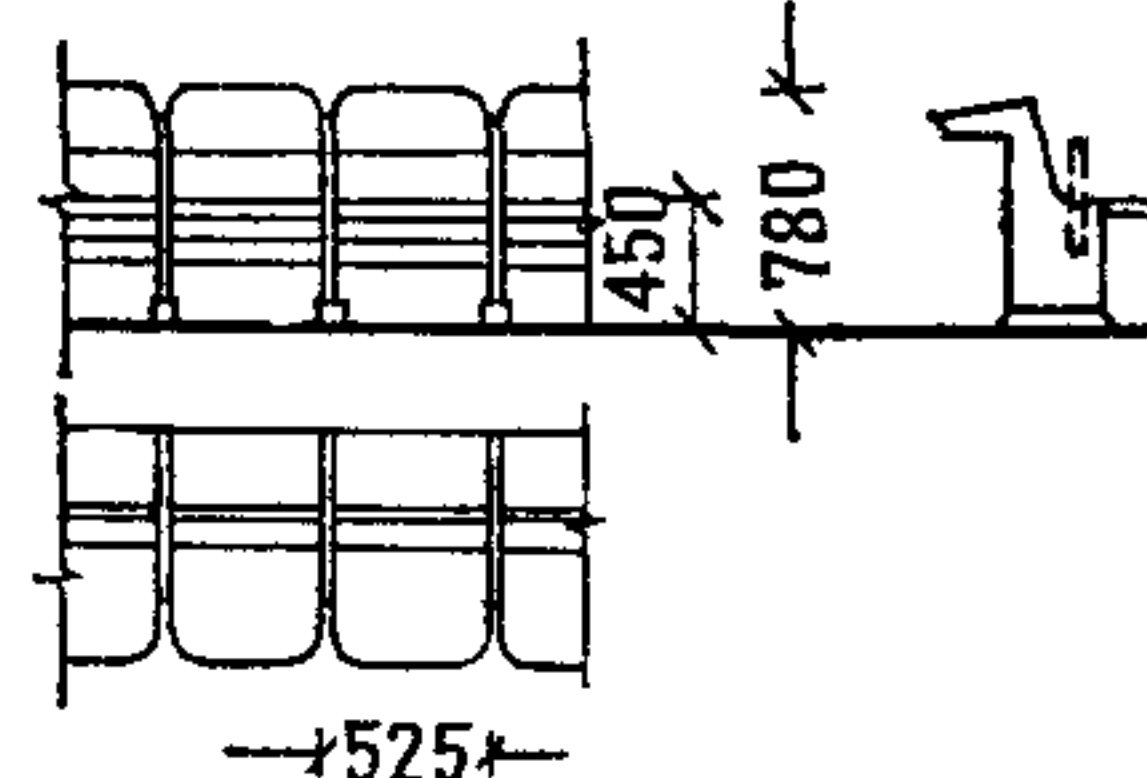
14 КРЕСЛО С ПЮПИТРОМ
