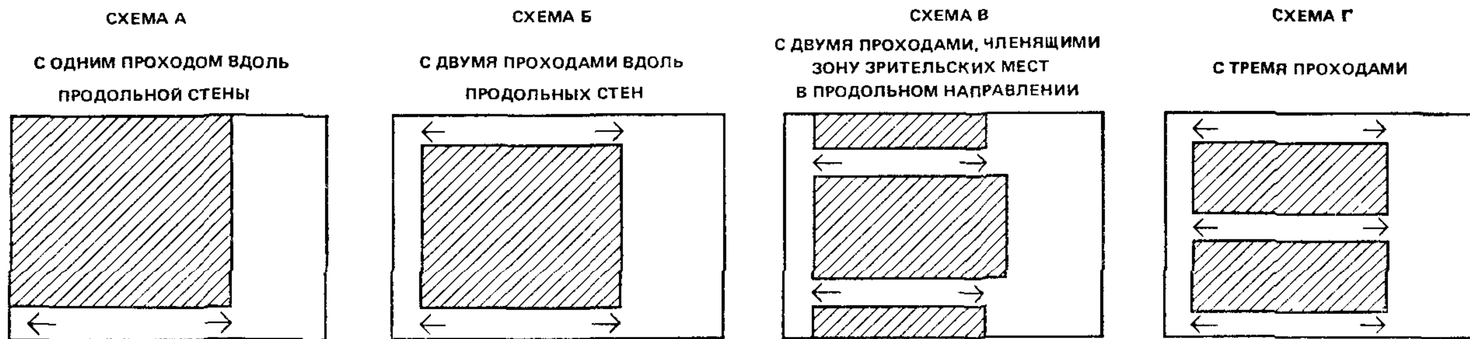
СХЕМЫ РАСПОЛОЖЕНИЯ ЭВАКУАЦИОННЫХ ПРОХОДОВ
