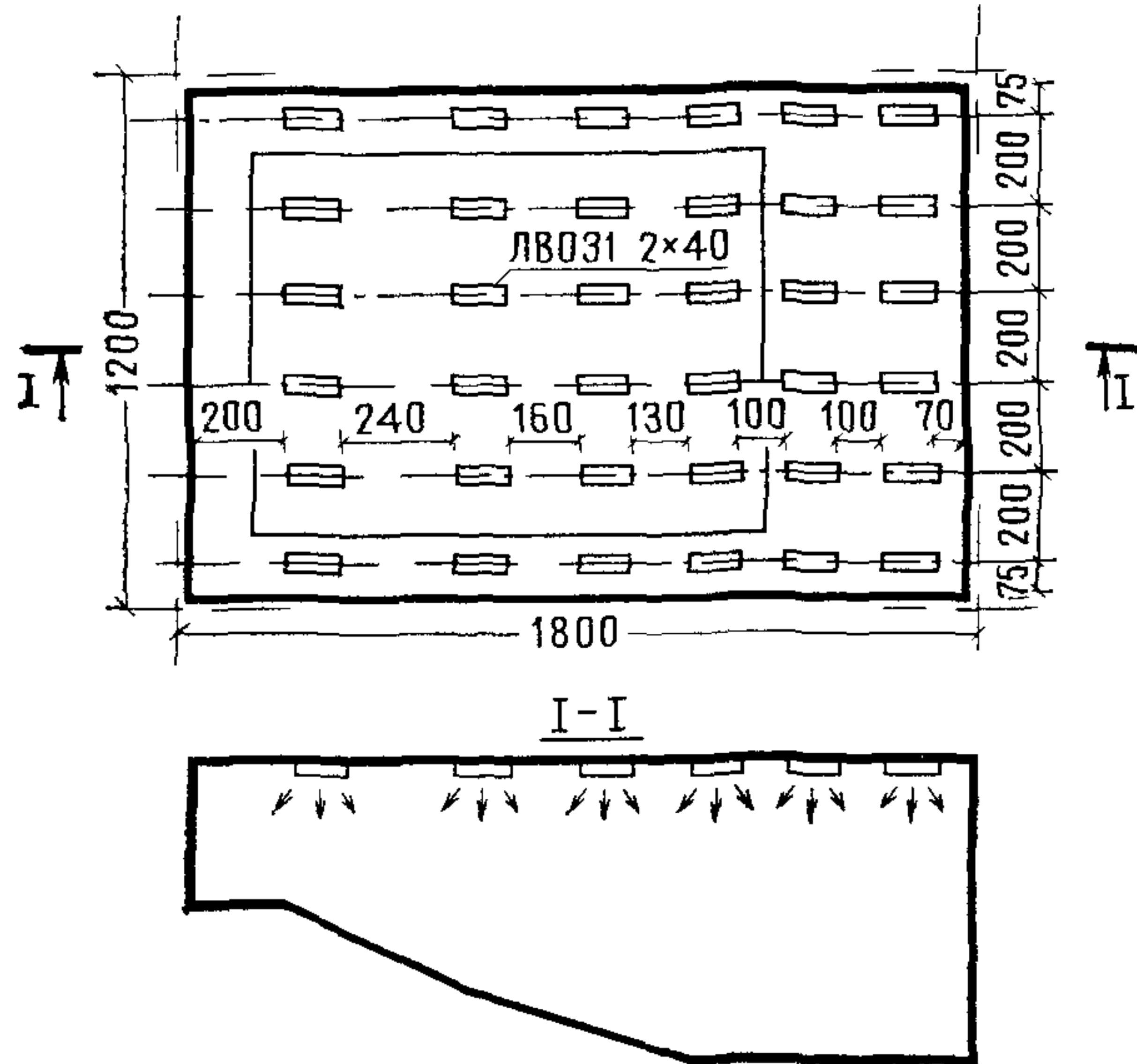
АУДИТОРИЯ РАЗМЕРОМ 12x18 м ЧА 200 МЕСТ
