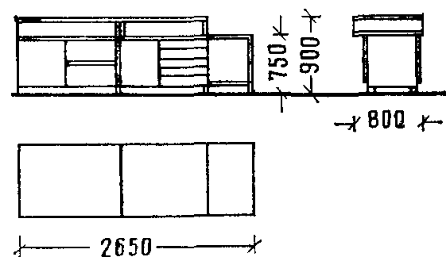
4 СТОЛ ДЕМОСТРАЦИОННЫЙ ДЛЯ ФИЗИЧЕСКИХ АУДИТОРИЙ
