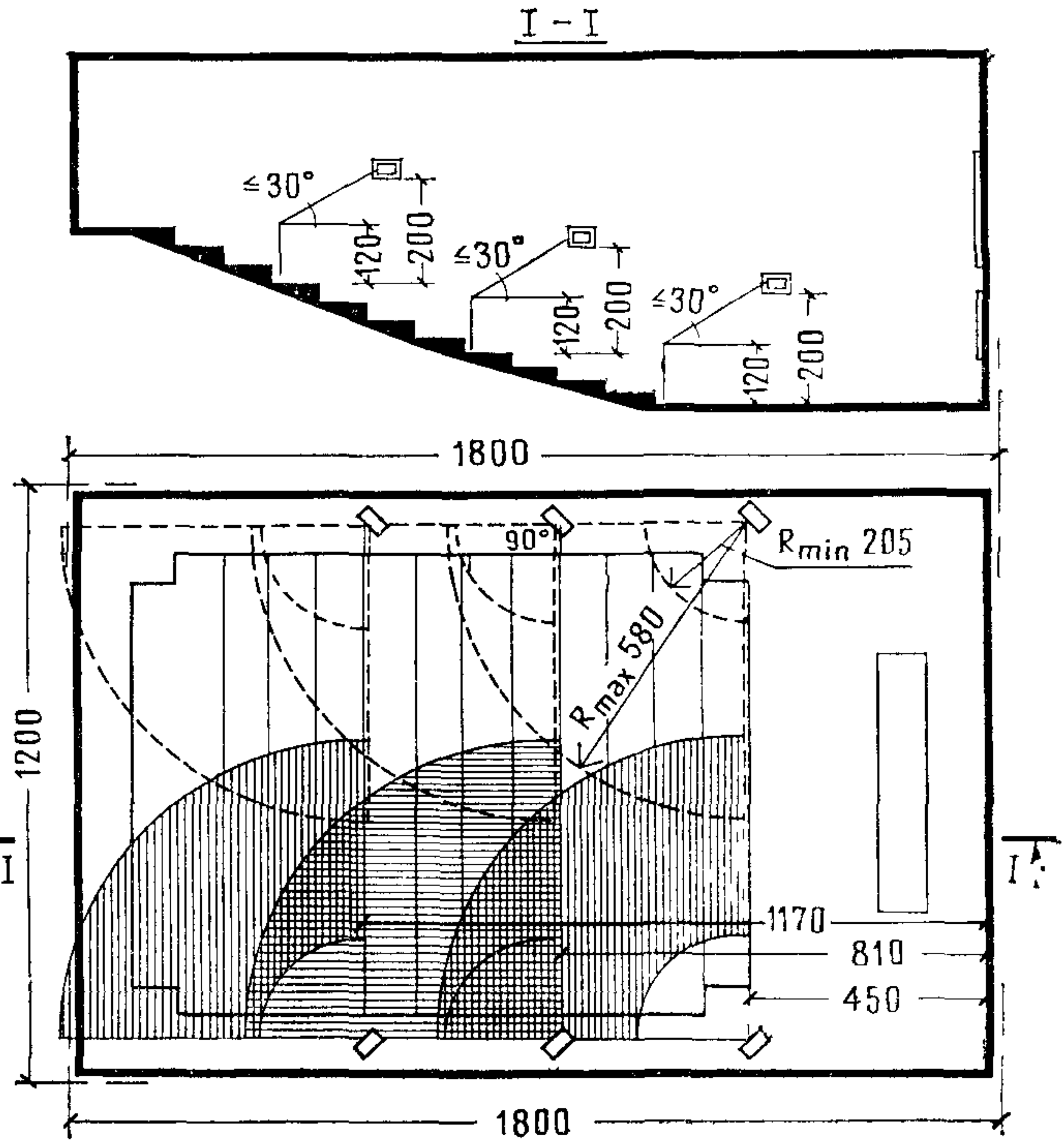
АУДИТОРИЯ РАЗМЕРОМ 12x18 м НА 200 МЕСТ
