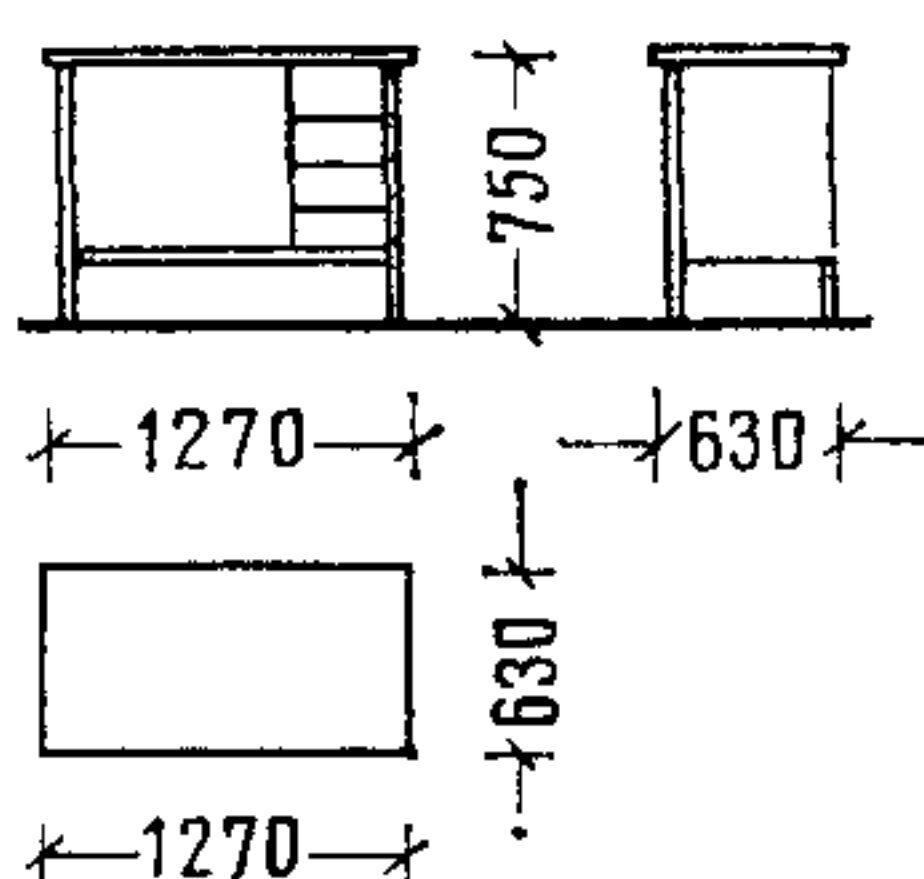
2 СТОЛ ПИСЬМЕННЫЙ ОДНОТУМБОВЫЙ
