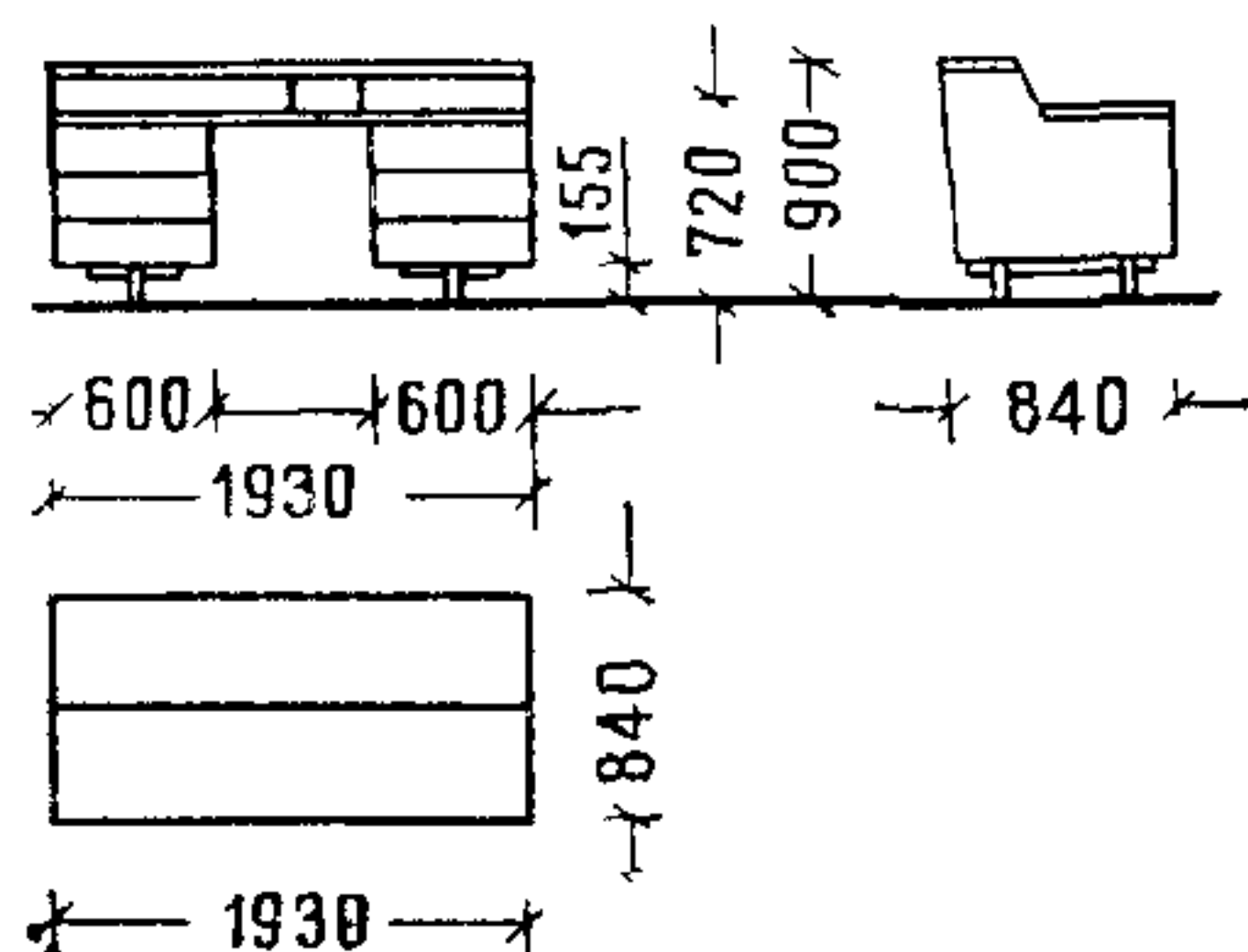
4 СТОЛ ДЕМОСТРАЦИОННЫЙ ДЛЯ ФИЗИЧЕСКИХ АУДИТОРИЙ
