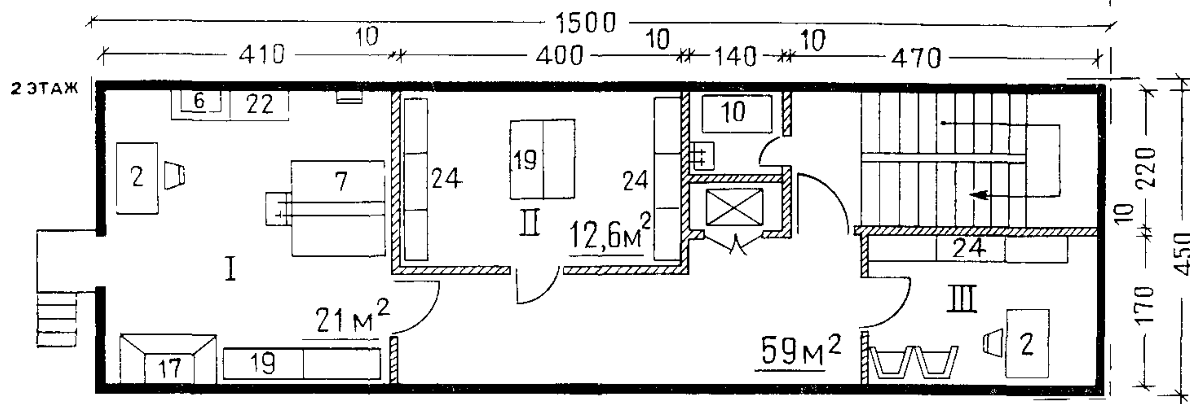
ПРЕПАРАТОРСКАЯ ХИМИИ ПРИ АУДИТОРИЯХ НА 300—350 МЕСТ
