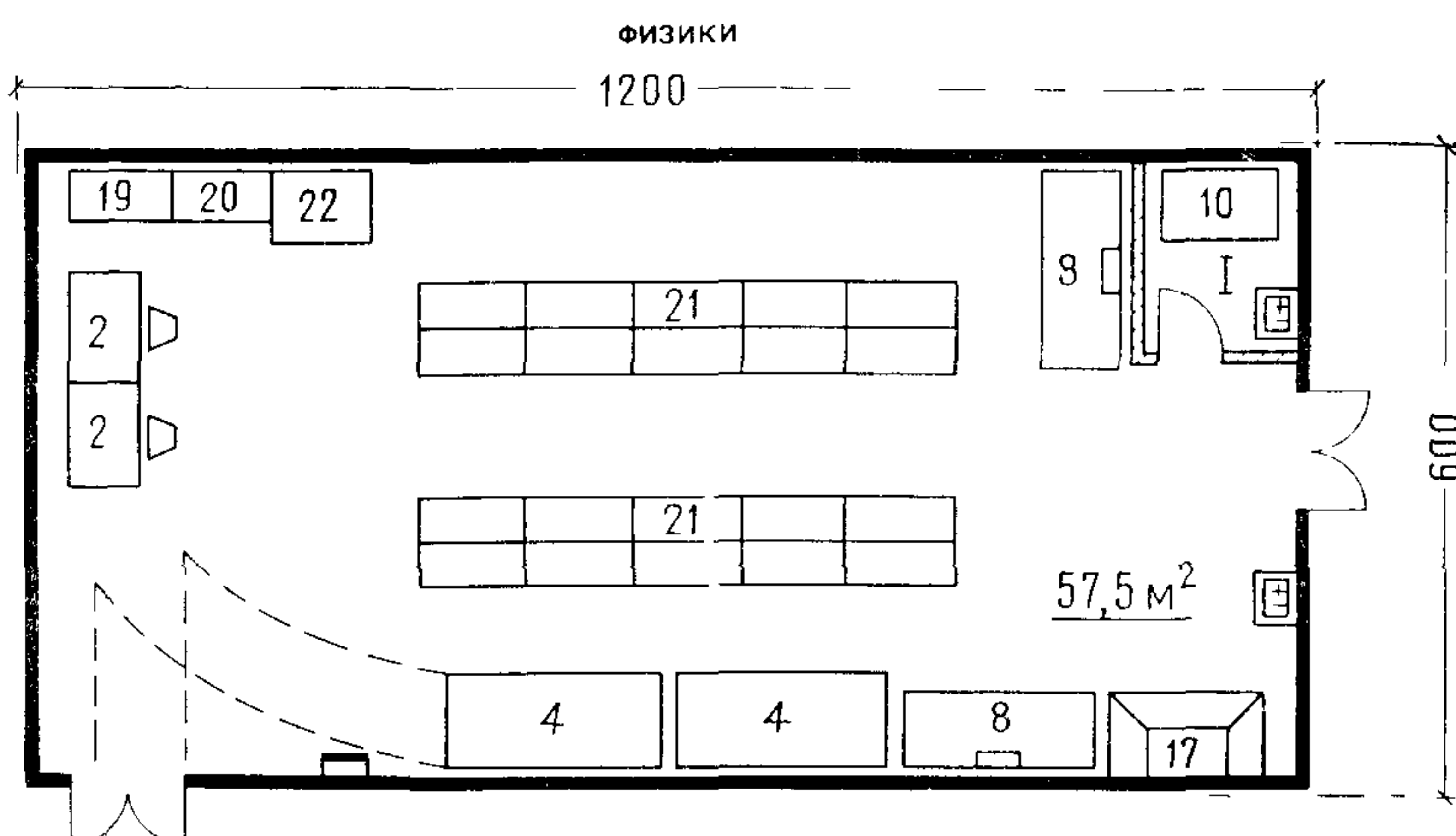
ПРЕПАРАТОРСКАЯ ПРИ АУДИТОРИИ НА 100—200 МЕСТ
