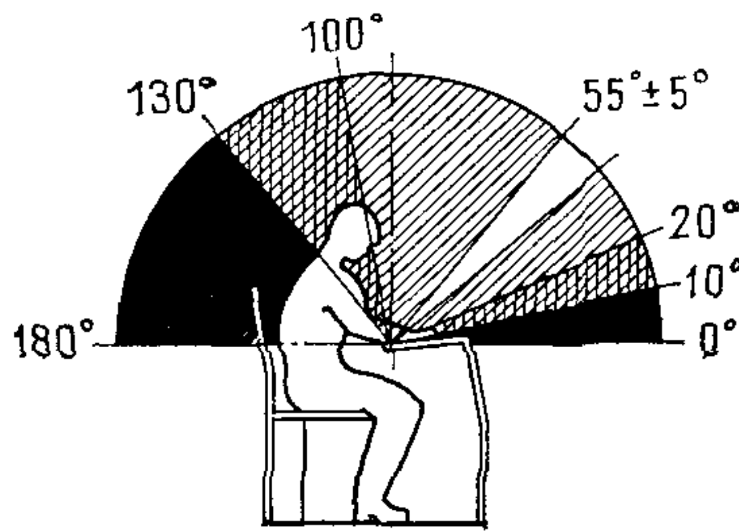
РЕКОМЕНДУЕМЫЕ НАПРАВЛЕНИЯ СВЕТА НА АУДИТОРНОМ МЕСТЕ
