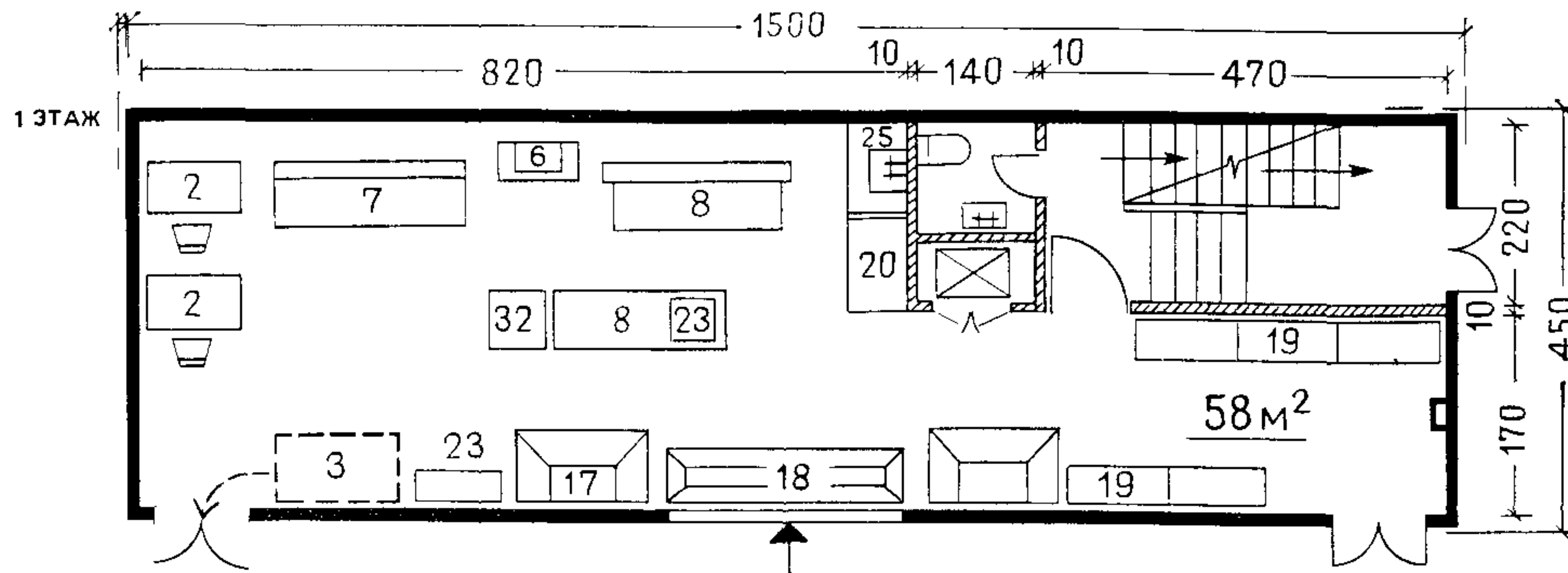
ПРЕПАРАТОРСКАЯ ХИМИИ ПРИ АУДИТОРИЯХ НА 200—300 МЕСТ
