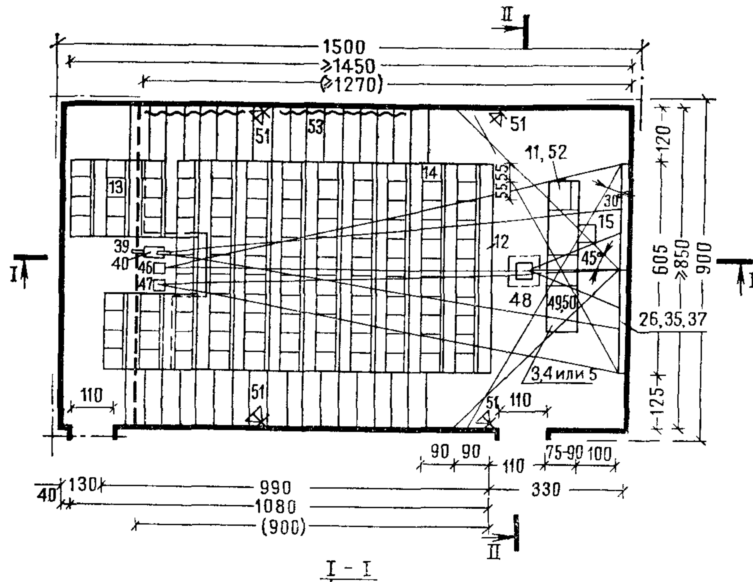
АУДИТОРИЯ НА 120 МЕСТ
