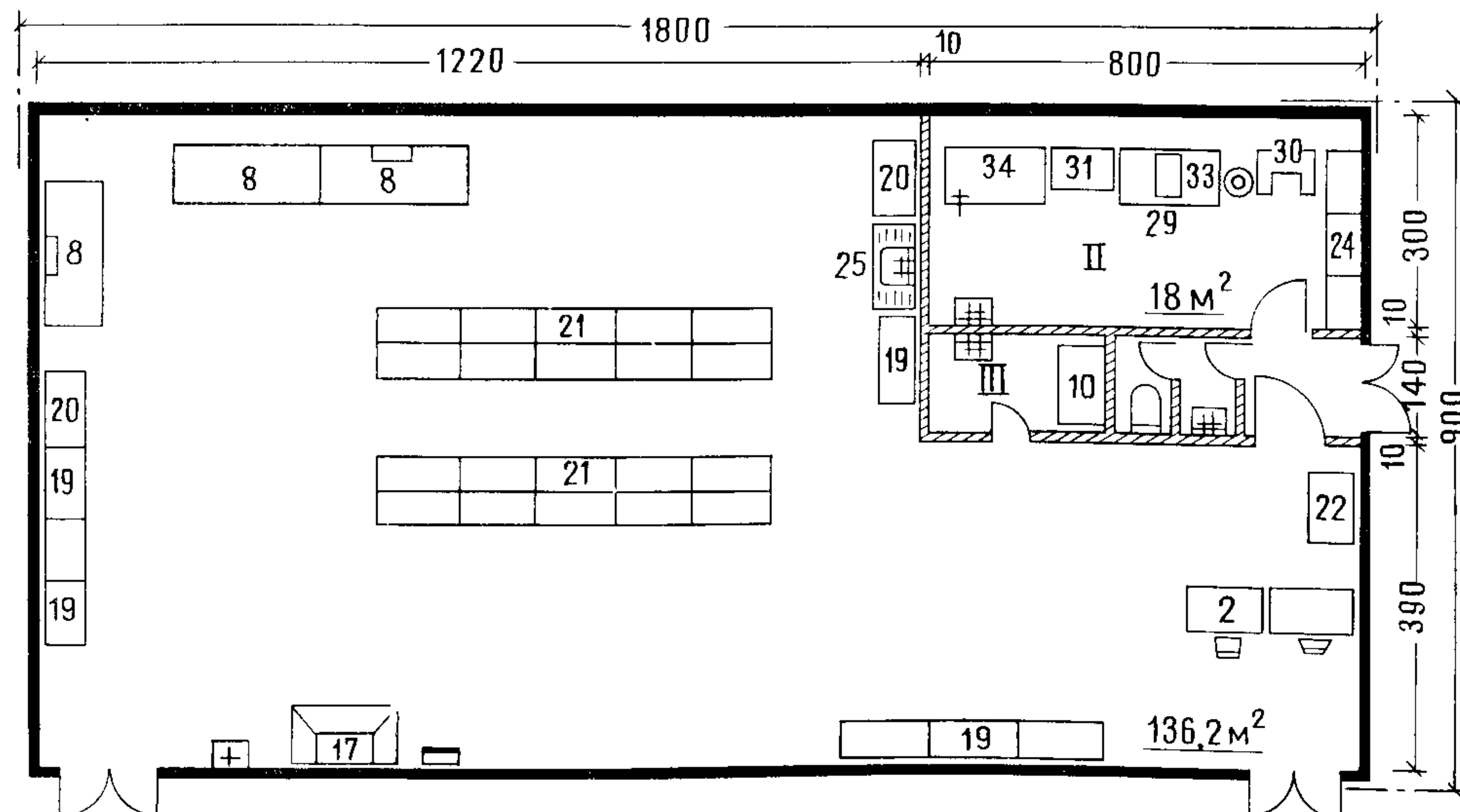
ВАРИАНТ ОДНОЭТАЖНОЙ ПЛАНИРОВКИ
