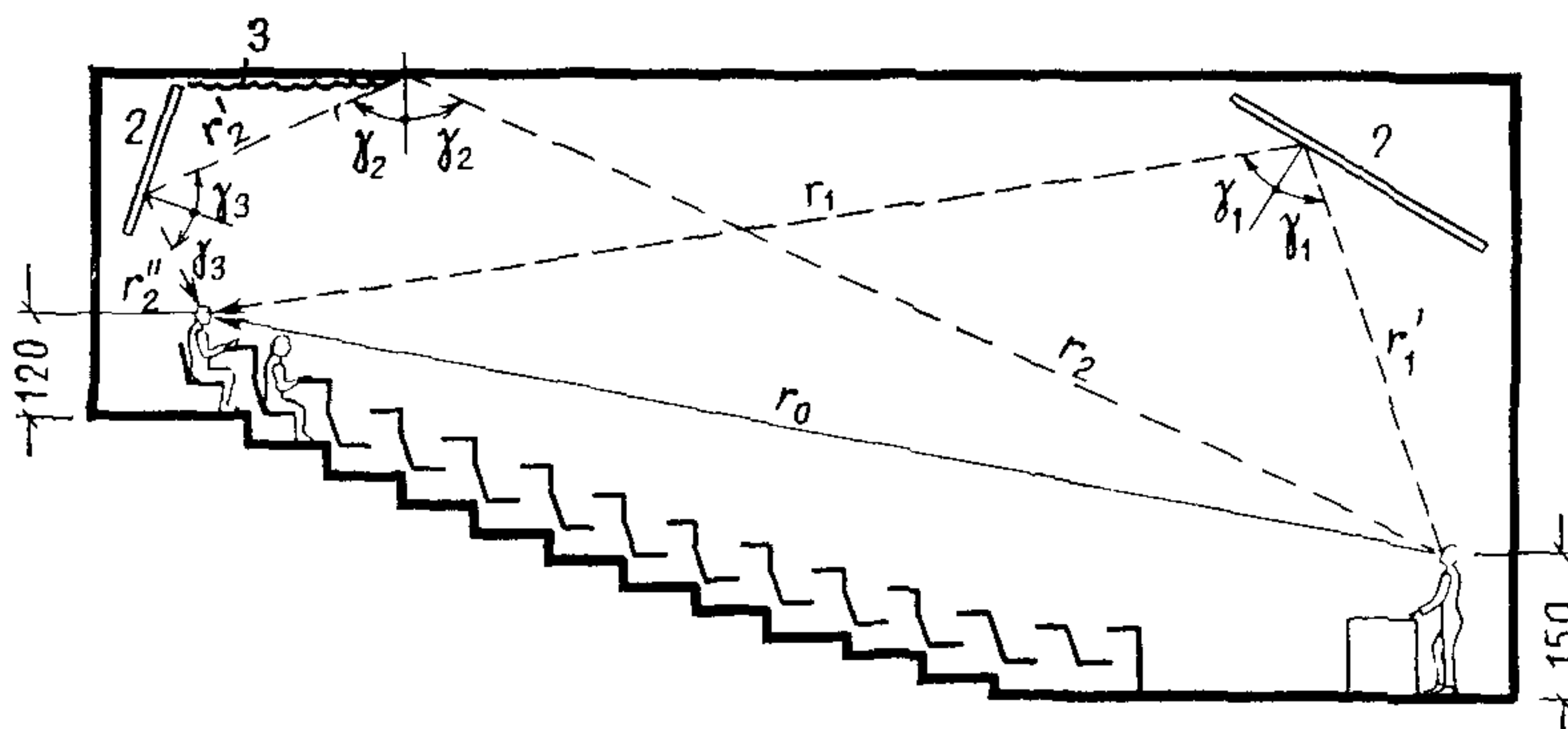
РАЦИОНАЛЬНОЕ РАСПРЕДЕЛЕНИЕ ОТРАЖЕНИЙ ОТ ПОТОЛКА ДЛЯ АУДИТОРИИ ВМЕСТИМОСТЬЮ 300 МЕСТ И БОЛЕЕ
