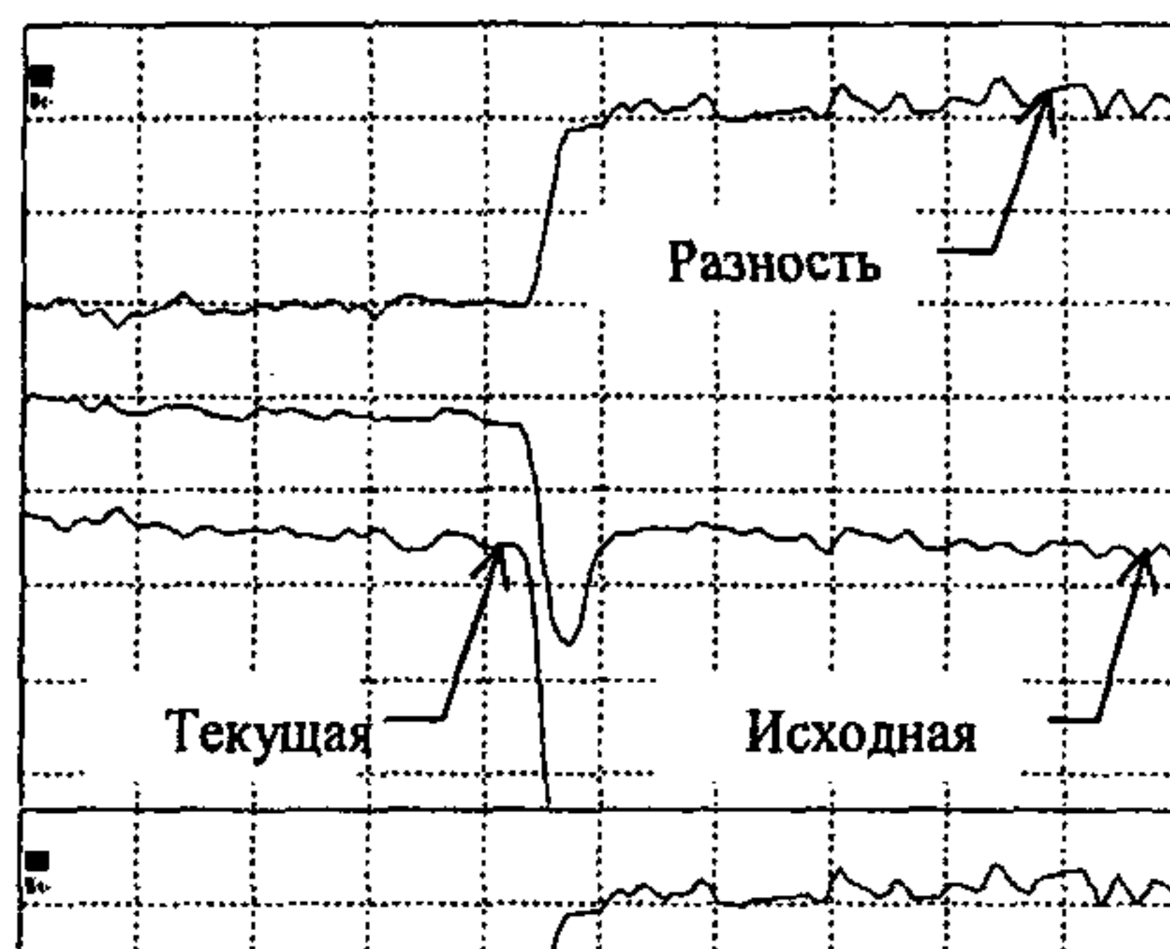
Рисунок 9 - Пример отображения разности исходной и текущей рефлектограмм
