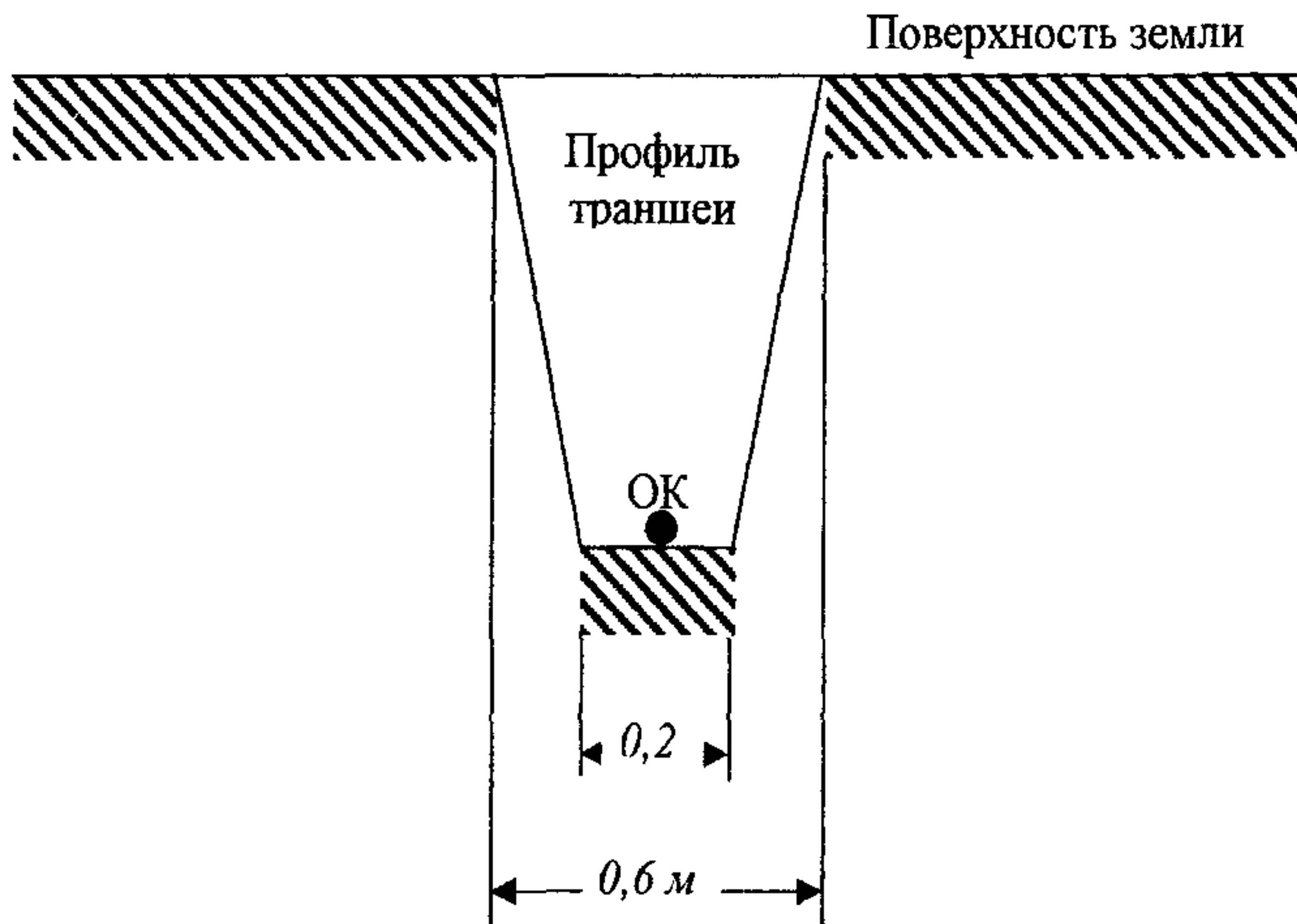
Рисунок 8 - Профиль траншеи.
