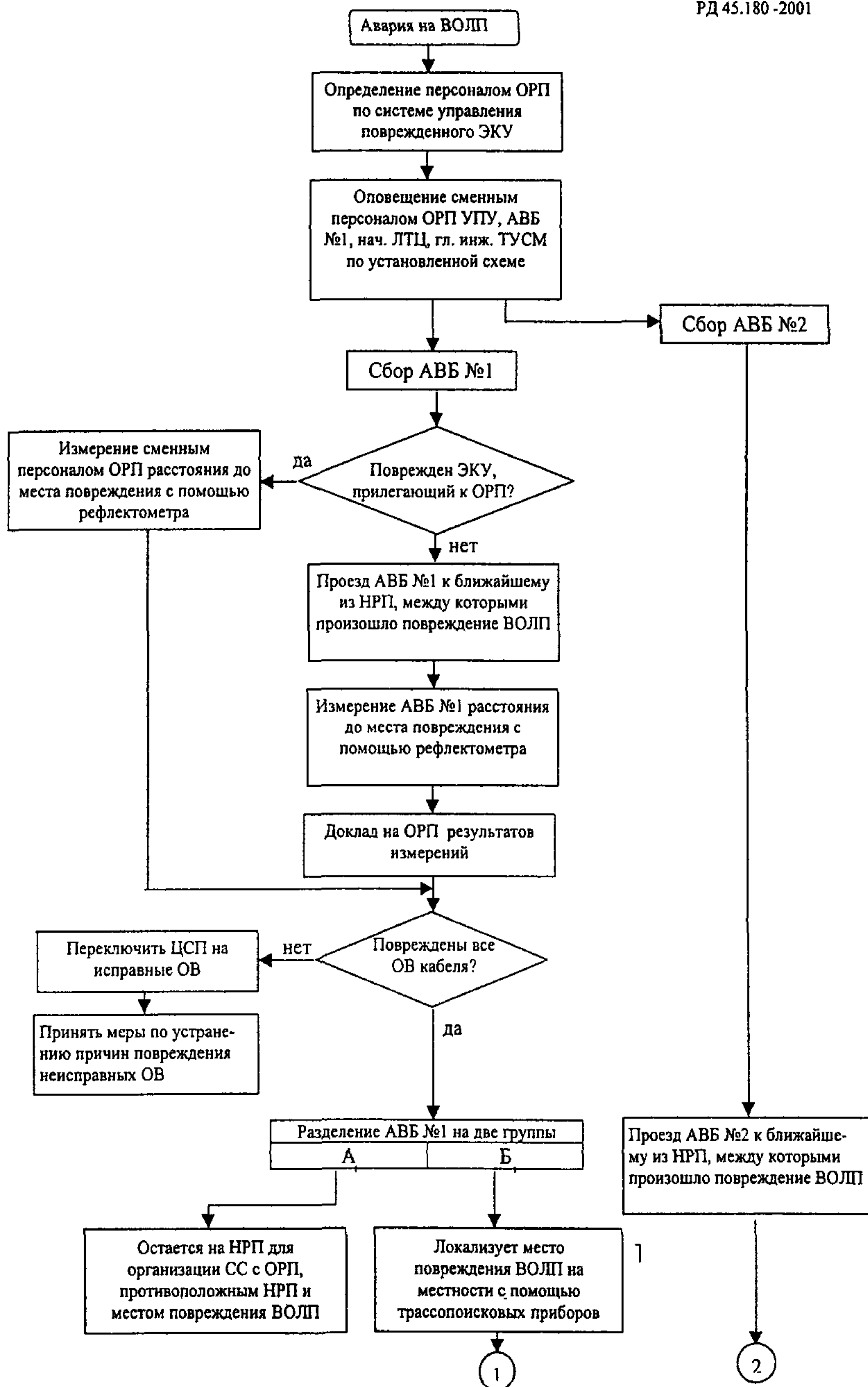
Рисунок 1, лист 1 – Структура типовой технологической карты по АВР
