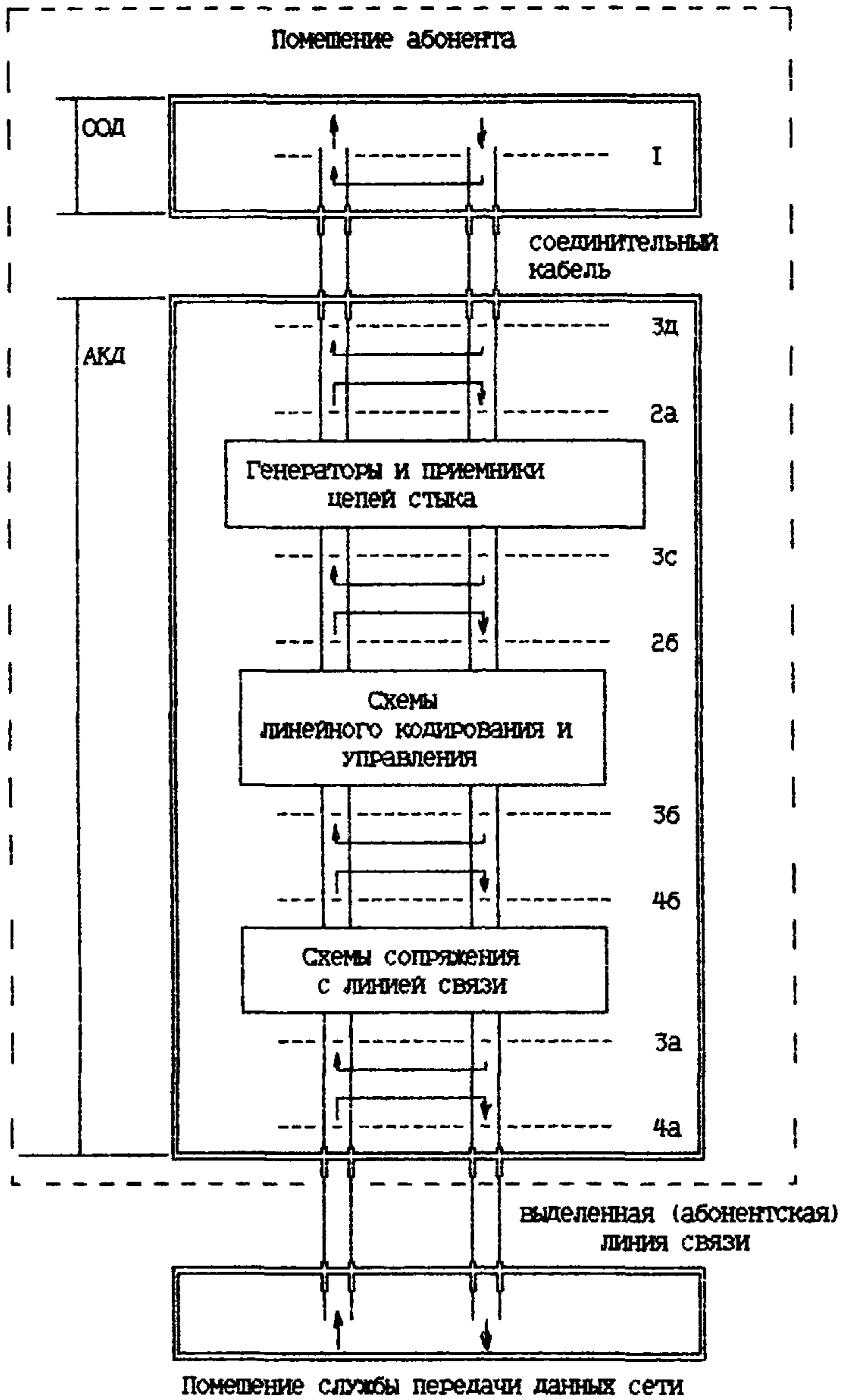
Рисунок 1. Структурная схема оборудования с расположением шлейфов
