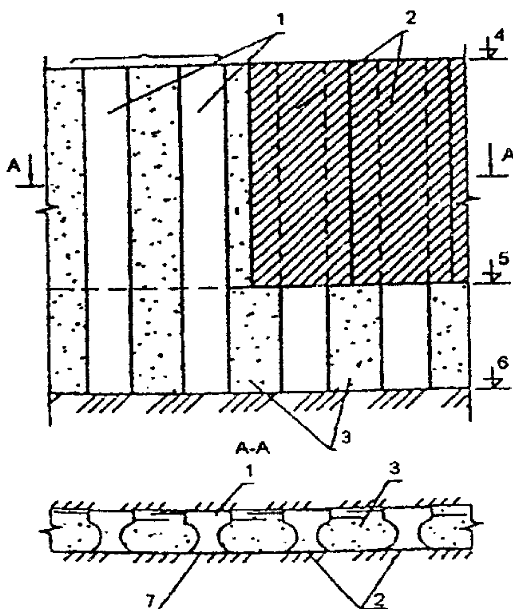
Рис. 4.1. Принципиальная схема сборно-монолитной «стены в грунте»: 1-стеновой блок; 2-листовая арматура; 3-бетонное заполнение; 4-отметка верха блока; 5-отметка дна котлована; 6-отметка низа стены; 7-контур траншеи
