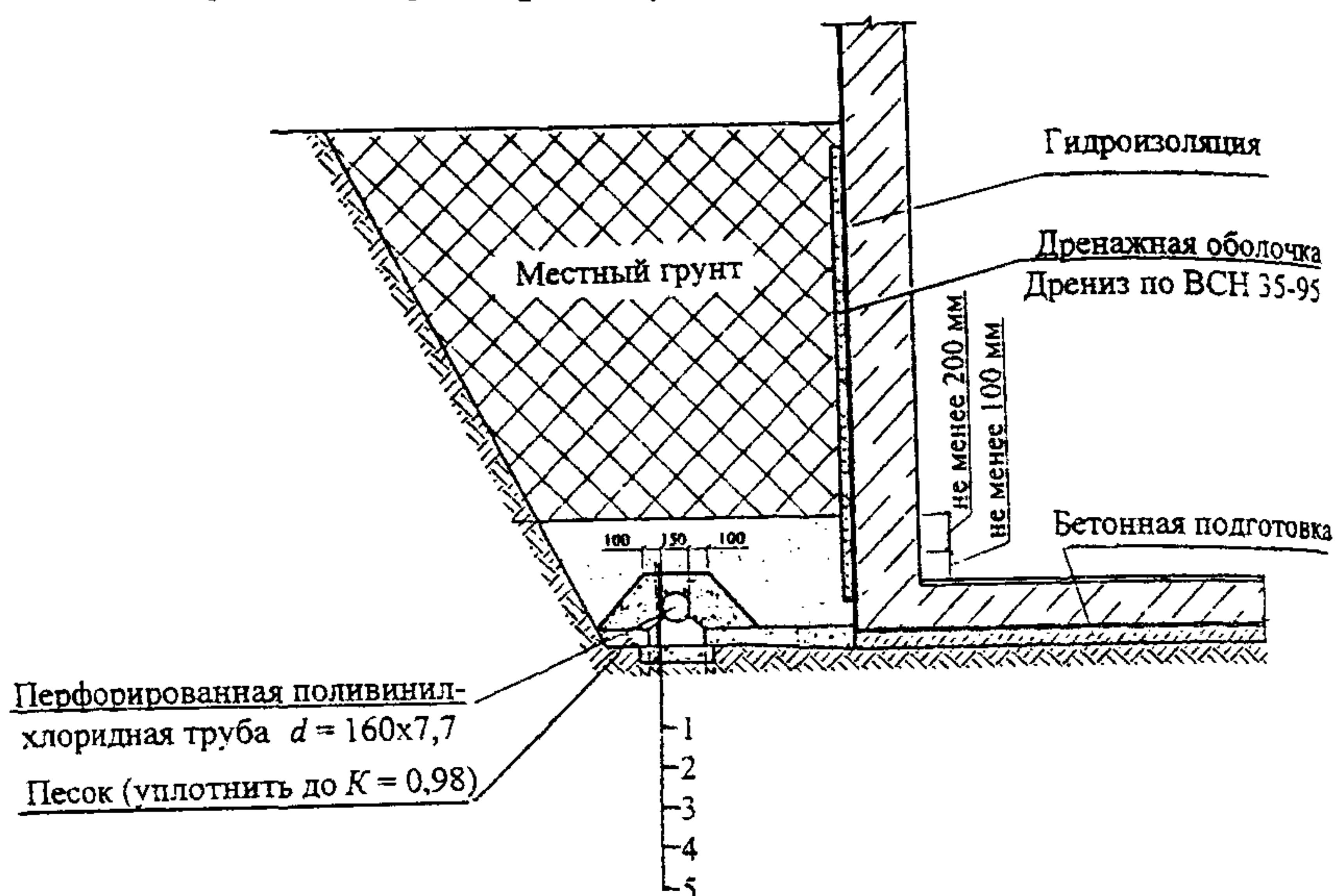
Рис. 6.3. Схема пристенного дренажа с применением поливинилхлоридных труб и дренажной оболочки «Дрениз»
