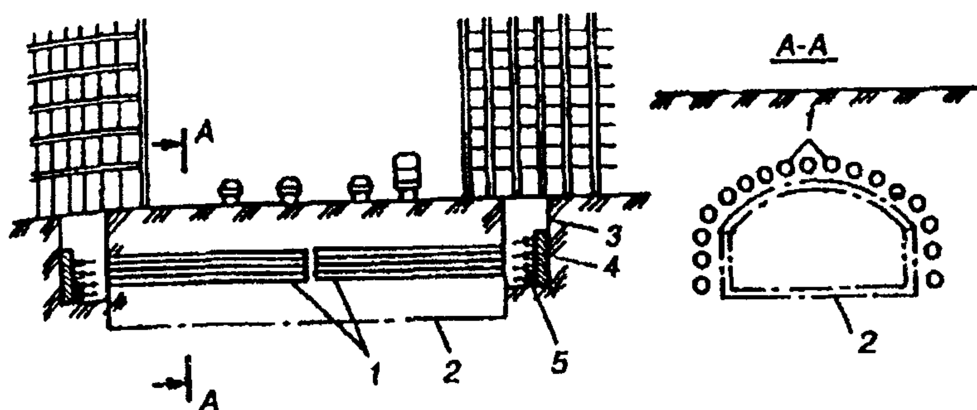
Рис. 5.4. Схема экрана из труб
