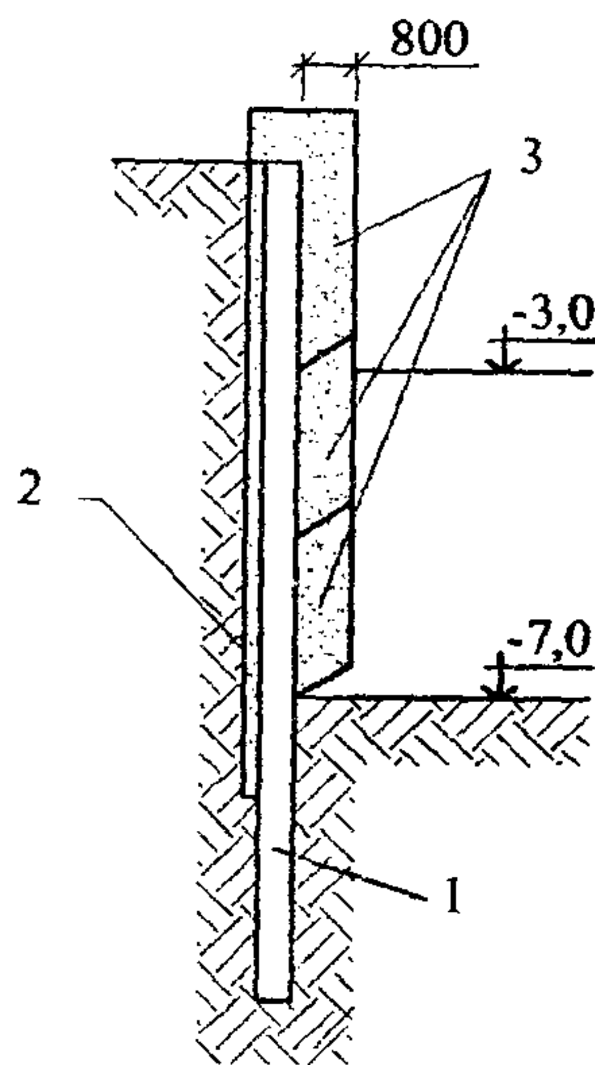
Рис. 4.4. Конструкция стены подземного сооружения из 2-х рядов свай
