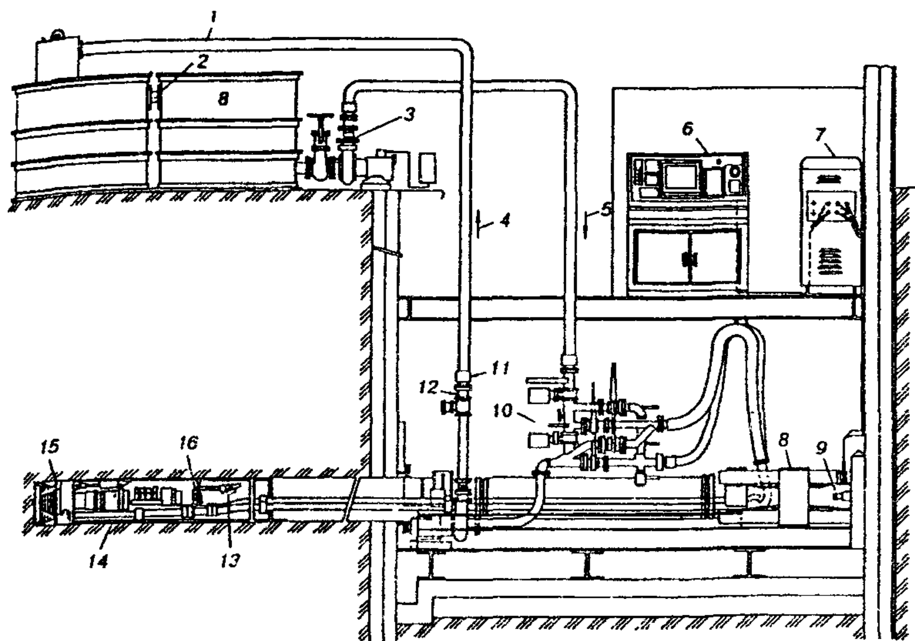
Рис. 5.10. Схема установки для прокладки коммуникаций способом микротоннелирования
