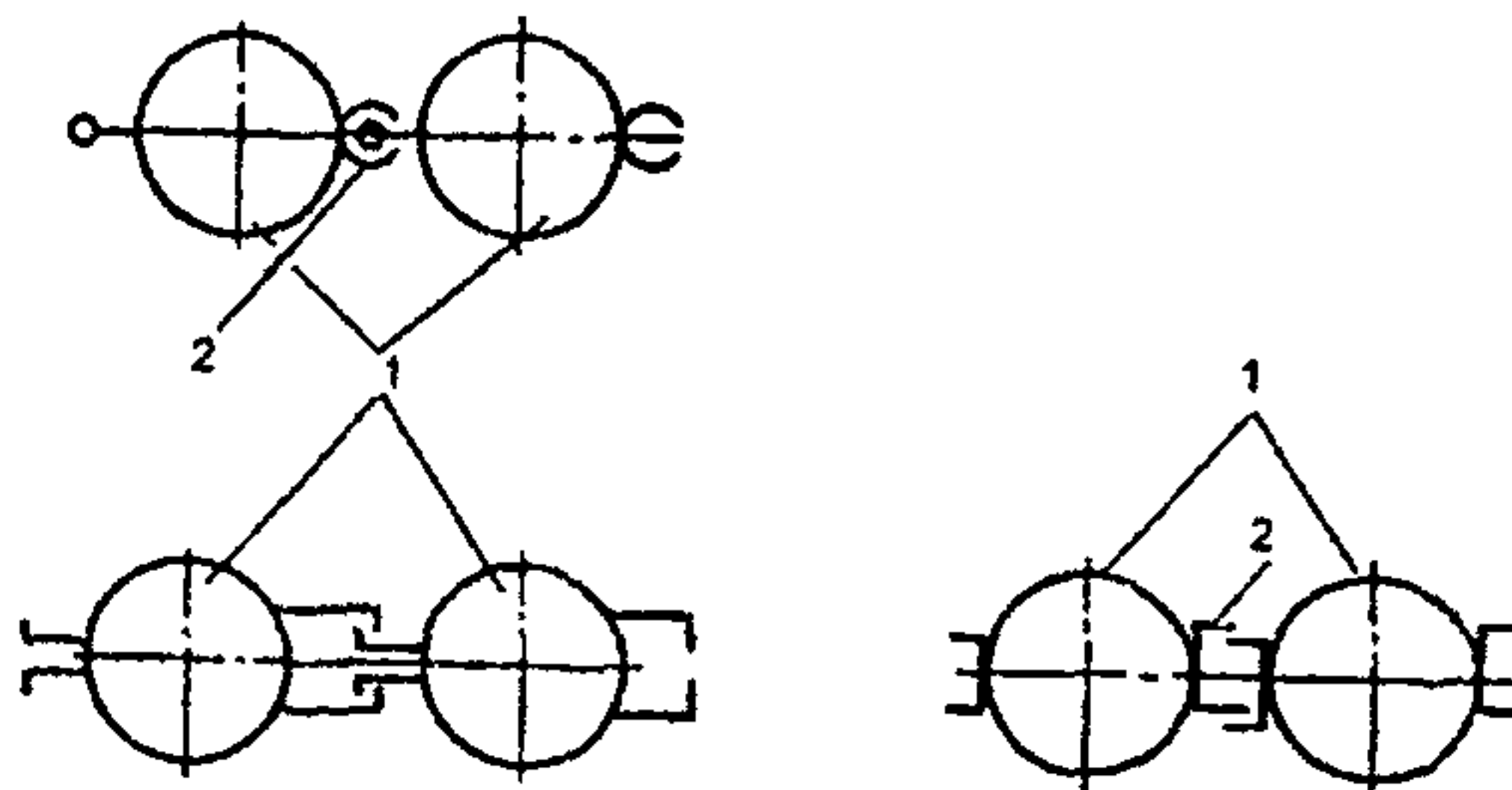
Рис. 5.5. Способ соединения труб 1- трубы; 2- замковые соединения
