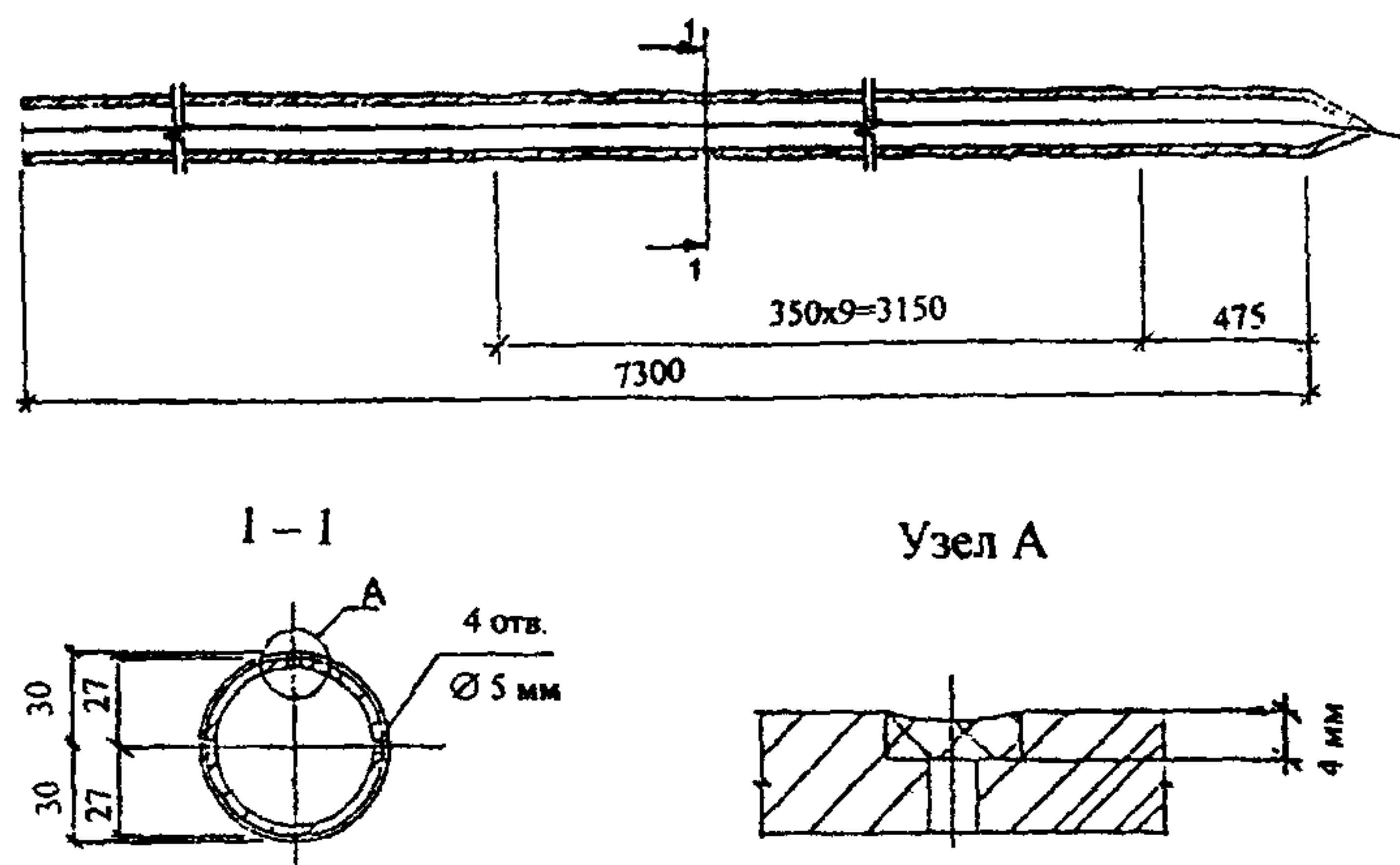
Рис. 7.1. Конструкция трубы-инъектора
