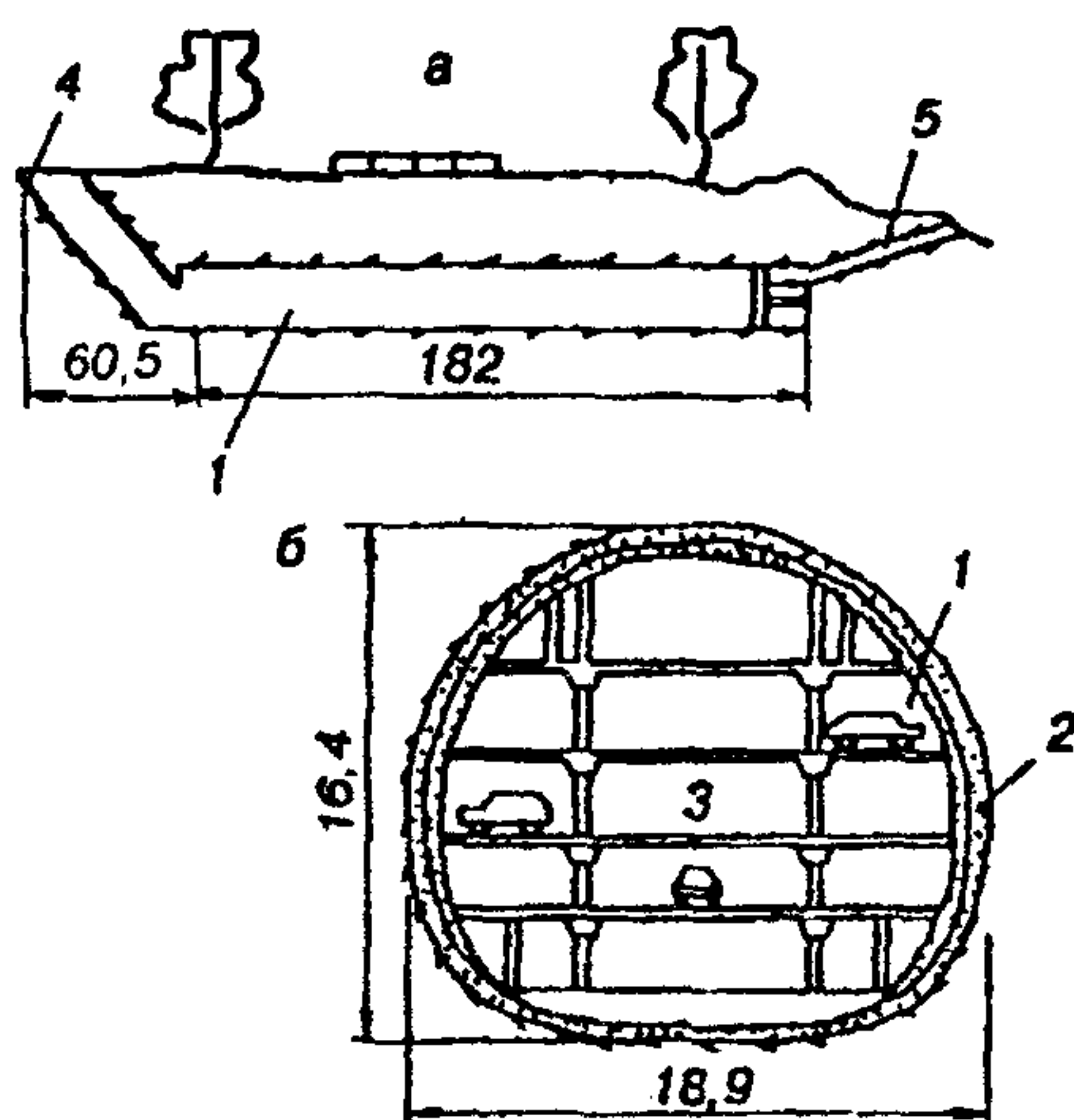
рис. 5.3. Продольный разрез (а) и поперечный разрез (б) подземной авто- стоянки в г. Ландесберге (Германия) 1- стояночные места; 2- обделка; 3- проезд; 4- въезд-выезд; 5- аварийный выезд; (рас- стояние в метрах)
