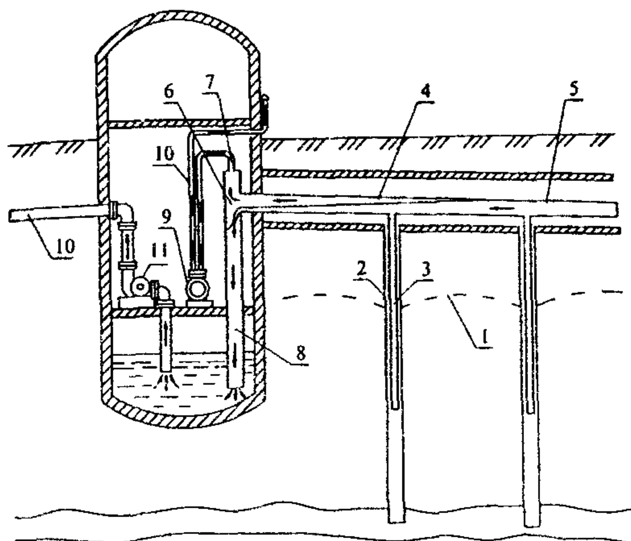
Рис. 6.8. Схема вертикального дренажа с системой сифонного водоотвода
