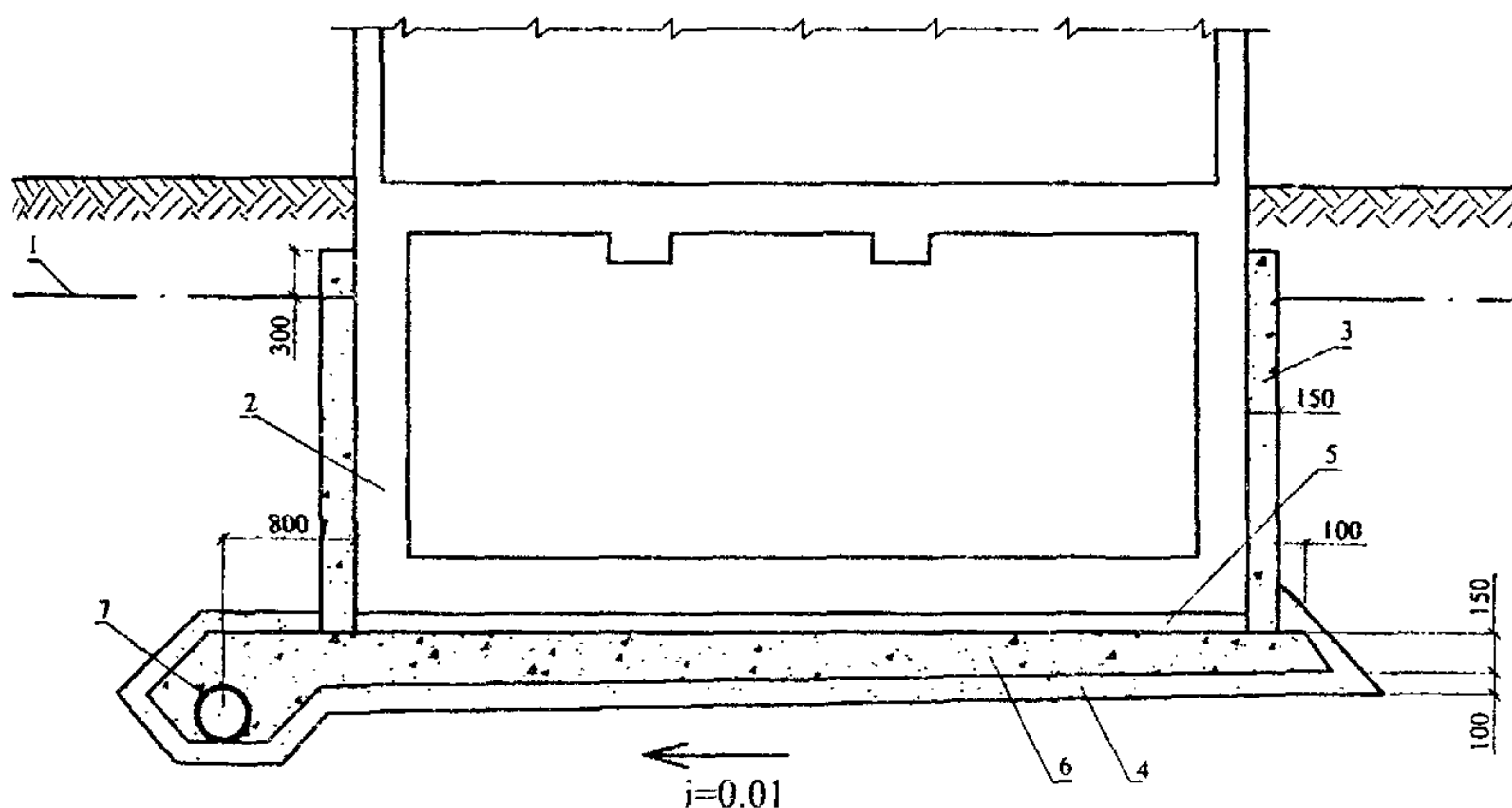
Рис. 6.2. Схема пластового дренажа
