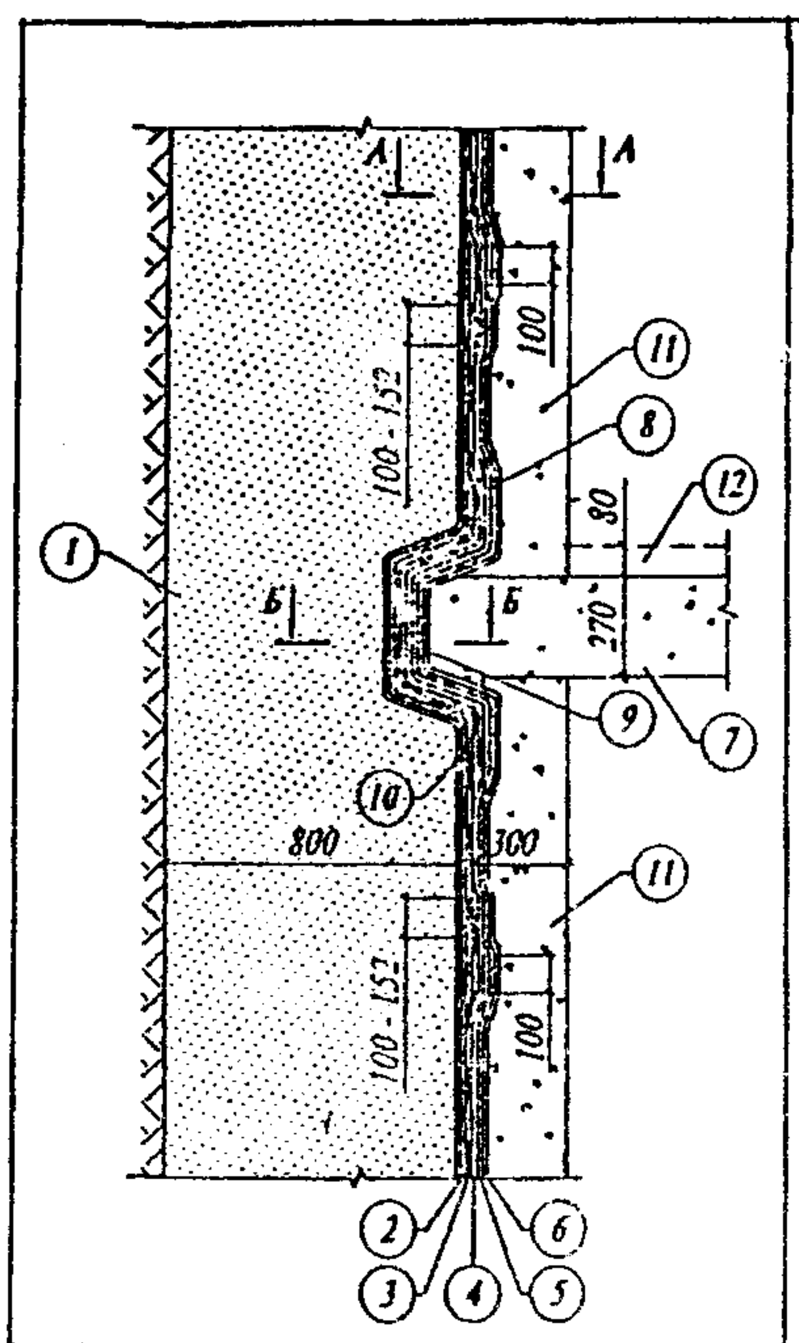
Рис. 6.9. Узел сопряжения гидроизоляции траншейной стены с промежуточным перекрытием, возводимым по схеме «сверху-вниз» (Многофункциональный комплекс «Царев сад», г. Москва)
