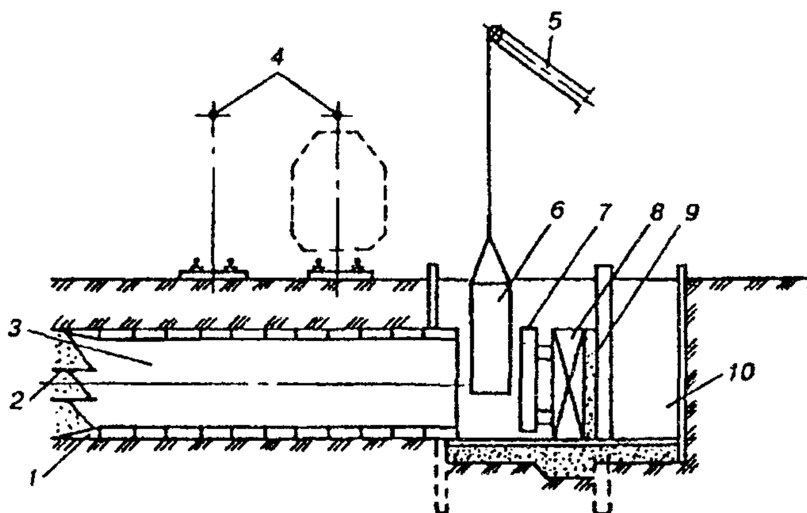
Рис. 5.8. Схема продавливания пешеходного тоннеля
