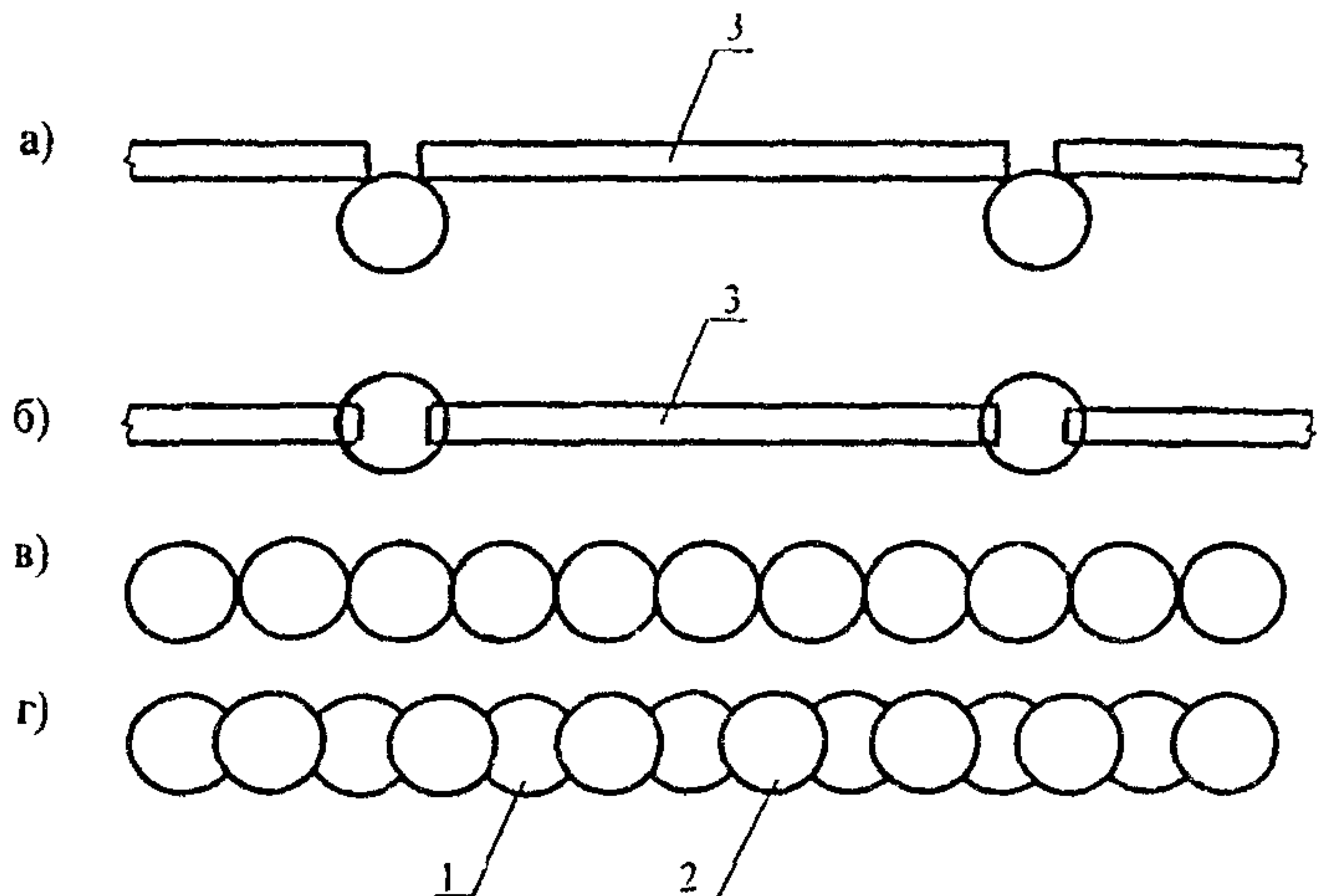
Рис. 4.2. Типы ограждений котлована из буронабивных свай
