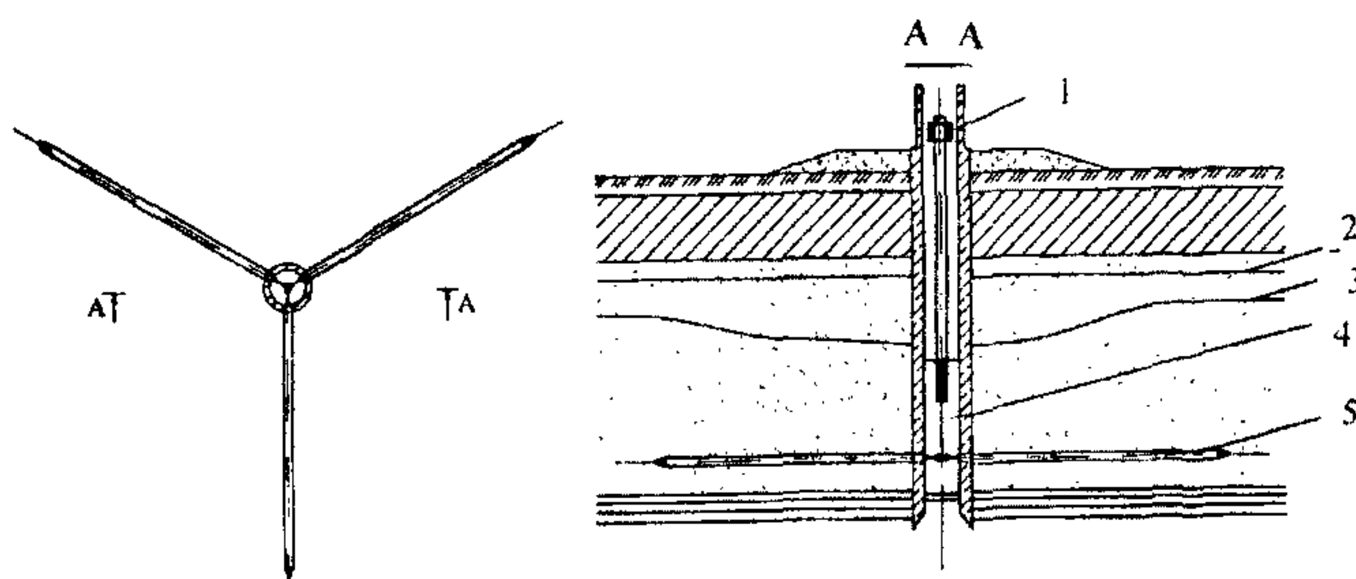
Рис.6.6. Лучевой дренаж.
