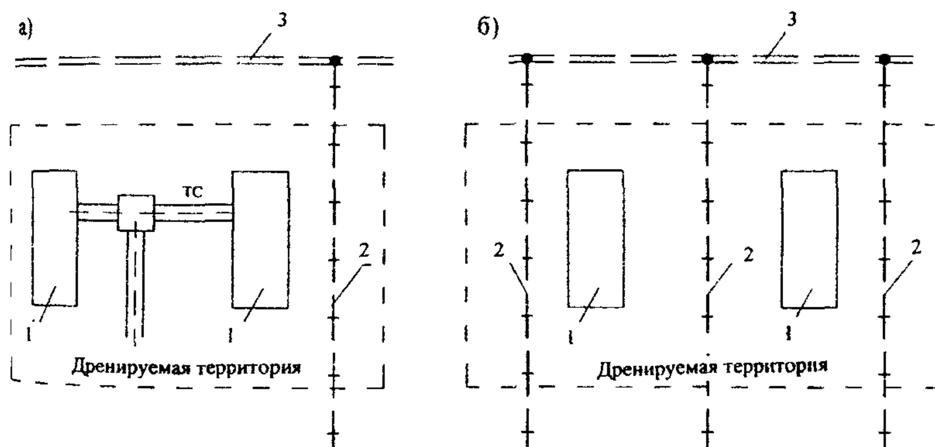
Рис. 6.1. Схемы дренажа: а) головного; б) систематического 1 – подземные сооружения; 2 – дренаж; 3 – водосточный коллектор
