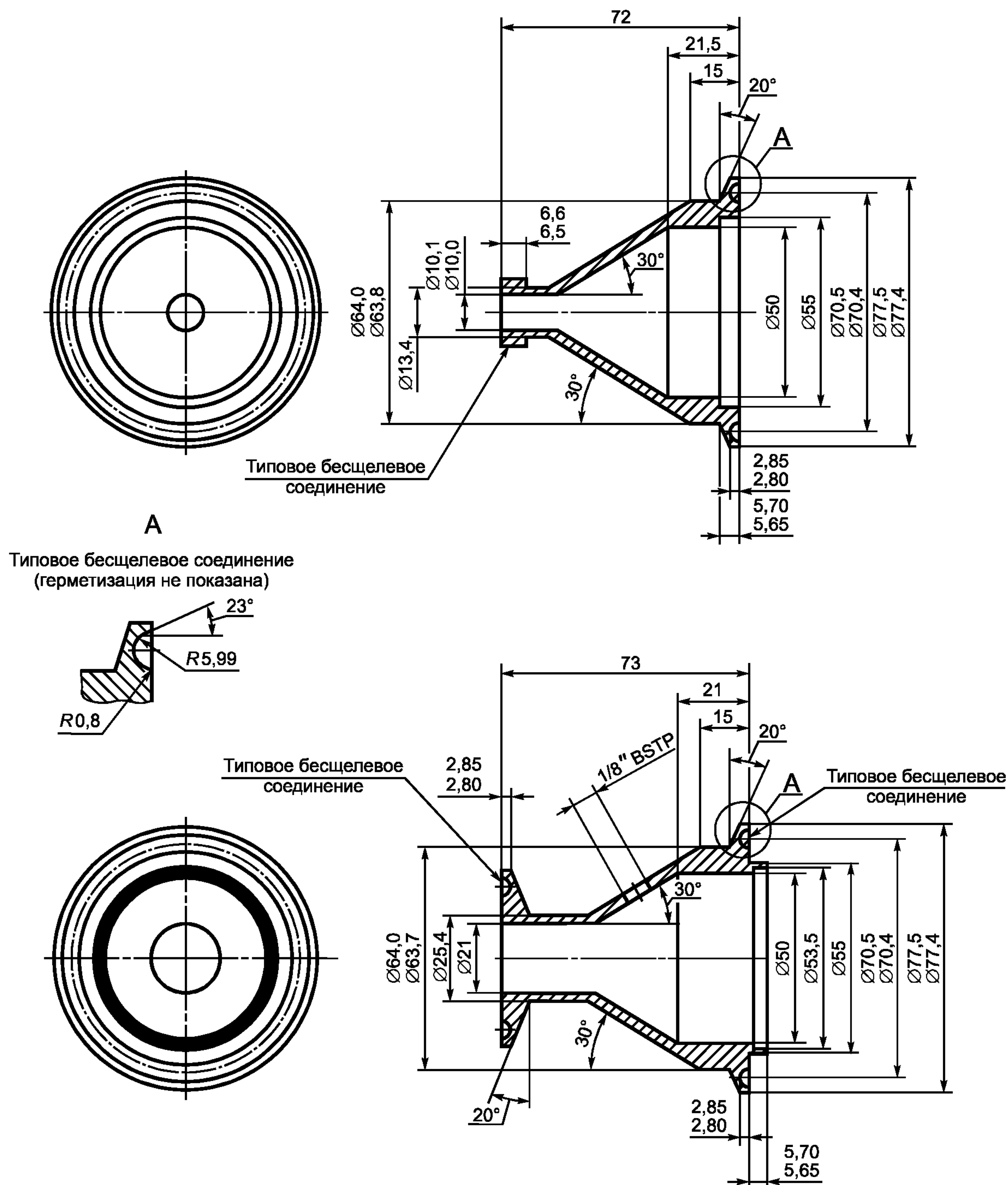
Рисунок 4 — Пример типового патрона мембраны
