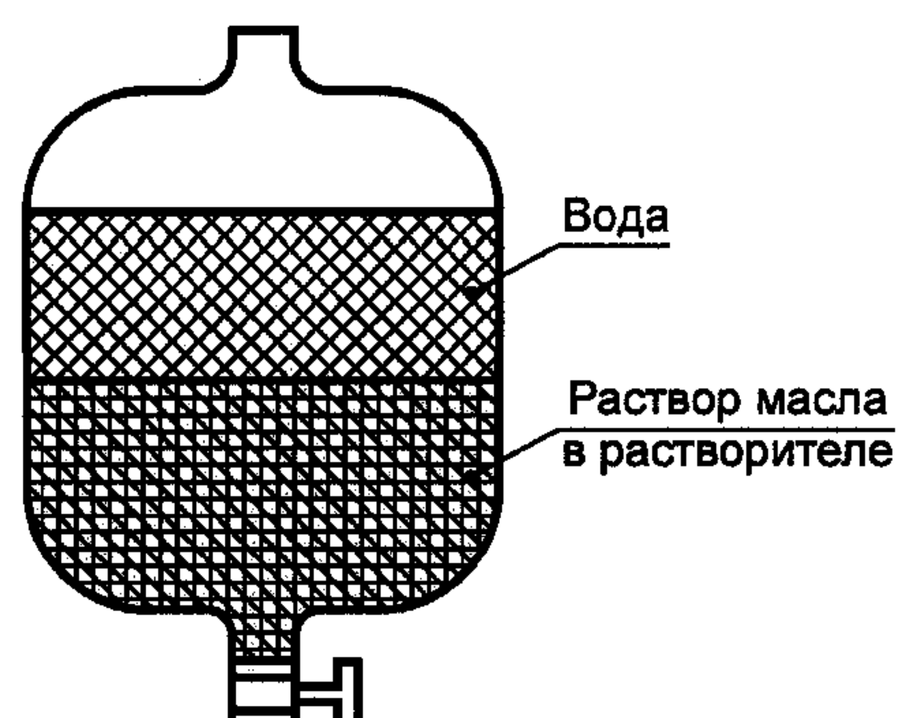
Рисунок 9 — Сепаратор для извлечения масла растворителем
