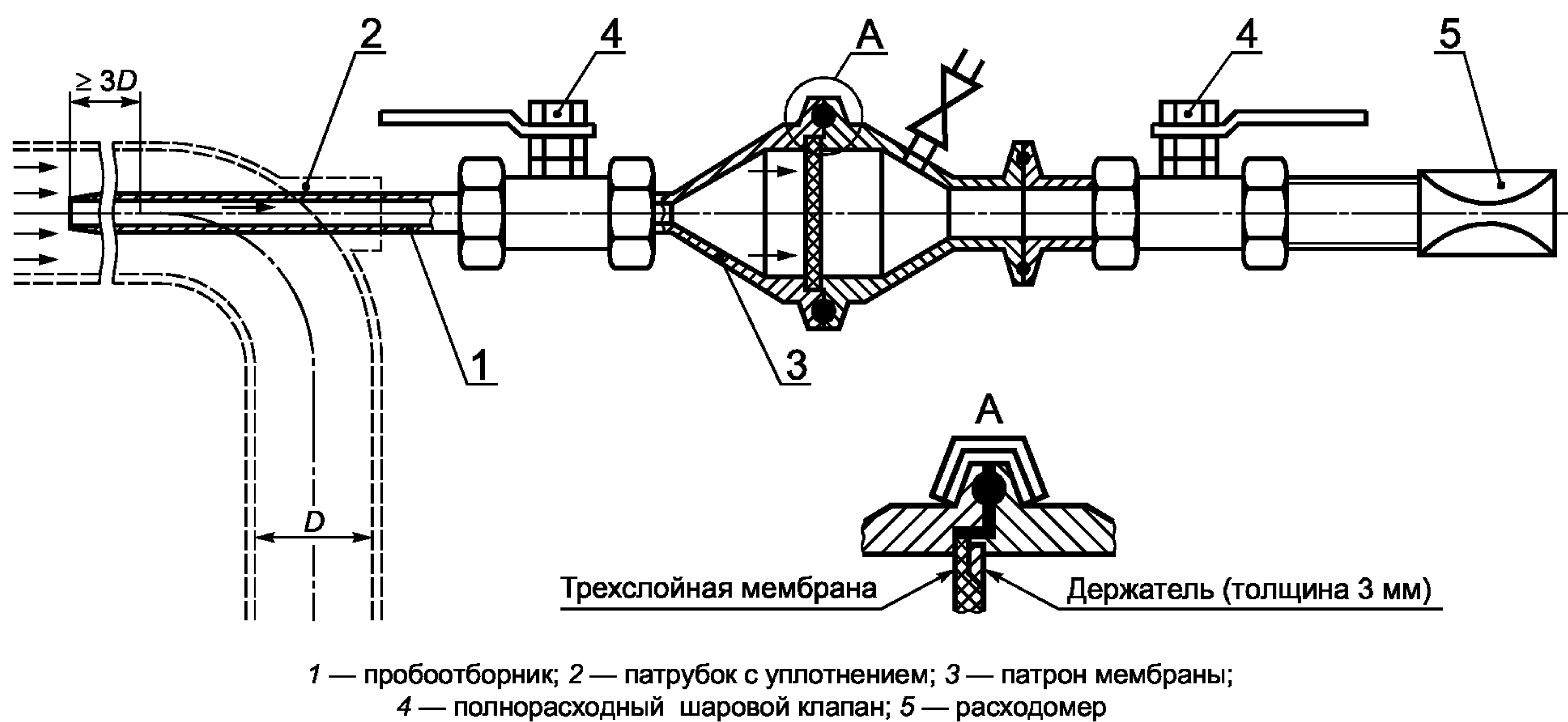
Рисунок 5 — Оборудование для изокINETического отбора проб в месте изгиба трубы по методу B2
