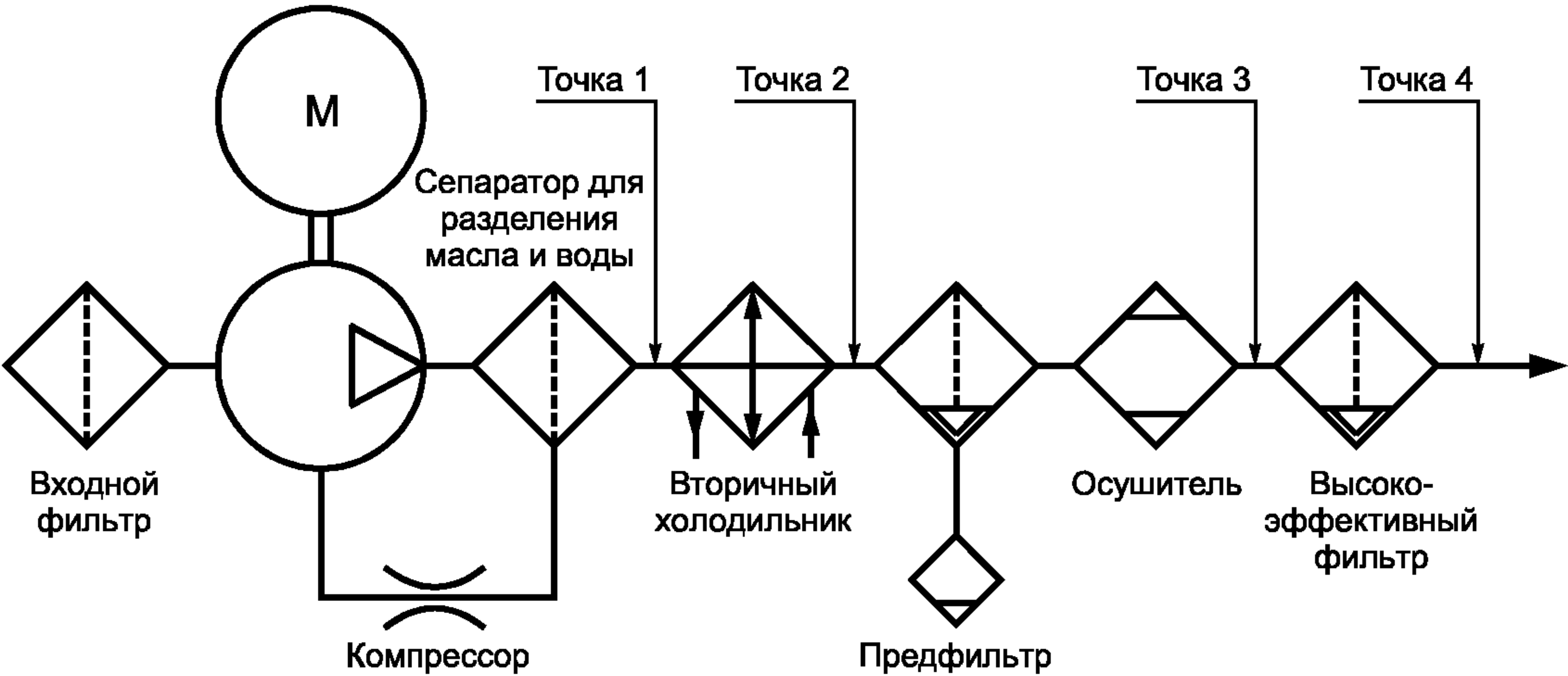
Рисунок 1 — Рекомендуемые точки отбора проб в системе сжатого воздуха
