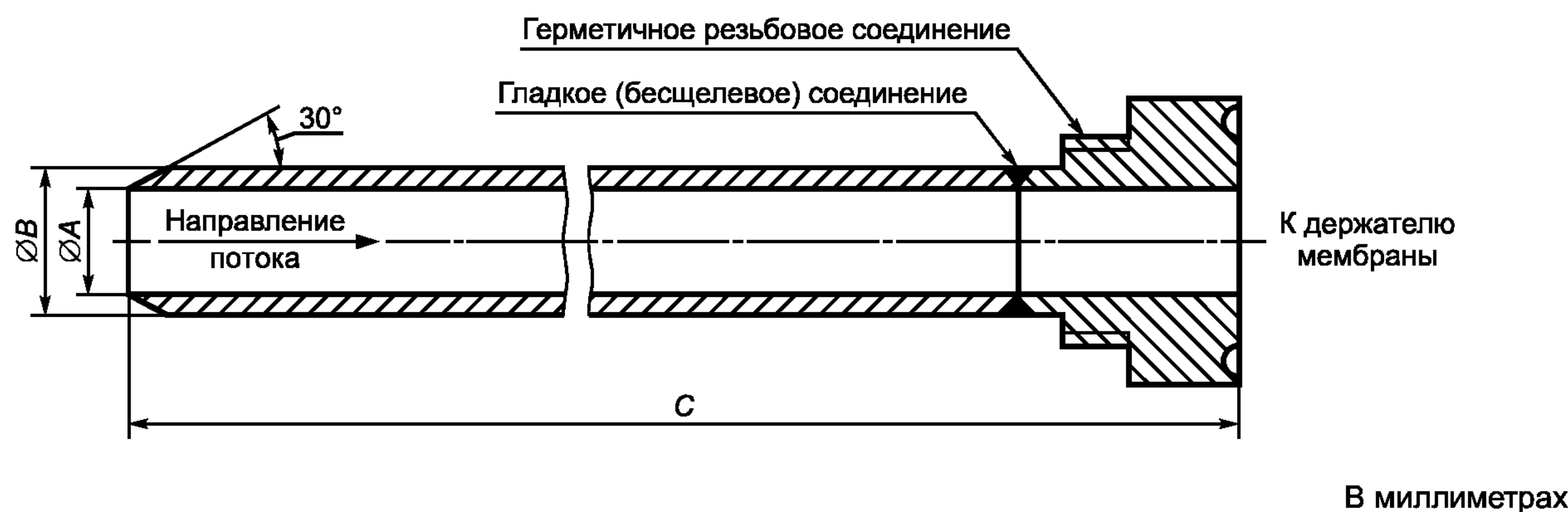
Рисунок 5 — Оборудование для изокINETического отбора проб в месте изгиба трубы по методу B2
