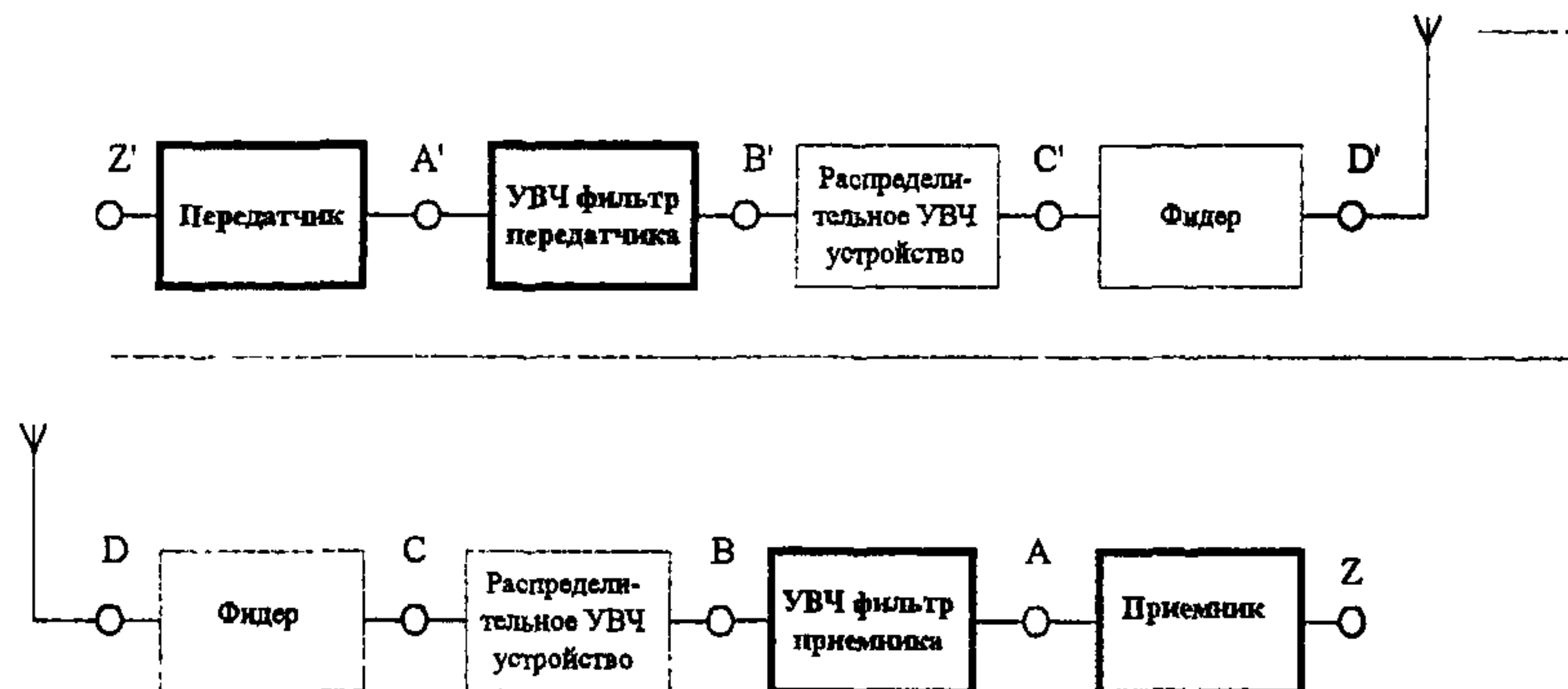
Рисунок 5.2 - Структурная схема радиооборудования АРД FH-CDMA 1-3 ГГц
