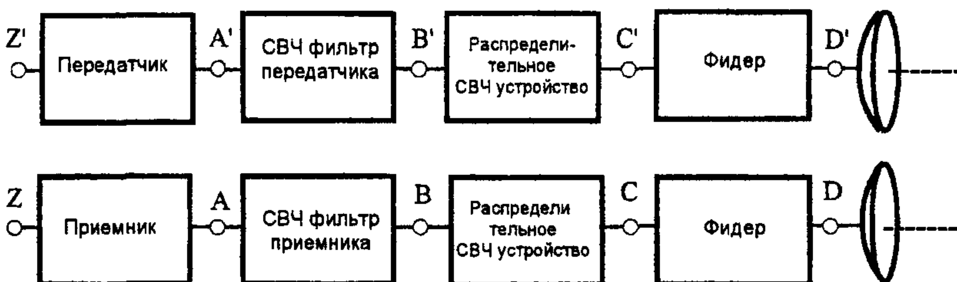
Рисунок 5.2 - Структурная схема радиооборудования АРД TDMA 3-11 ГГц
