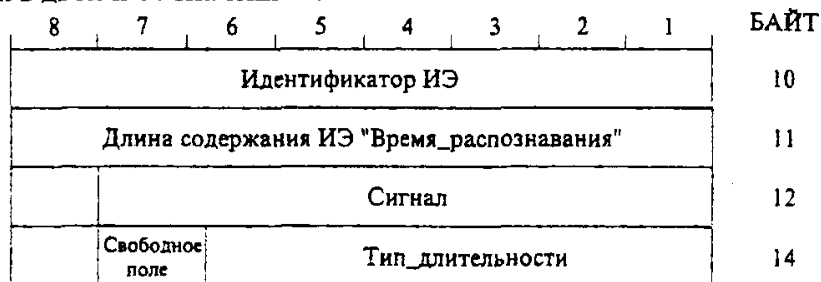
Рисунок 27- Структура ИЭ "Время_распознавания"
