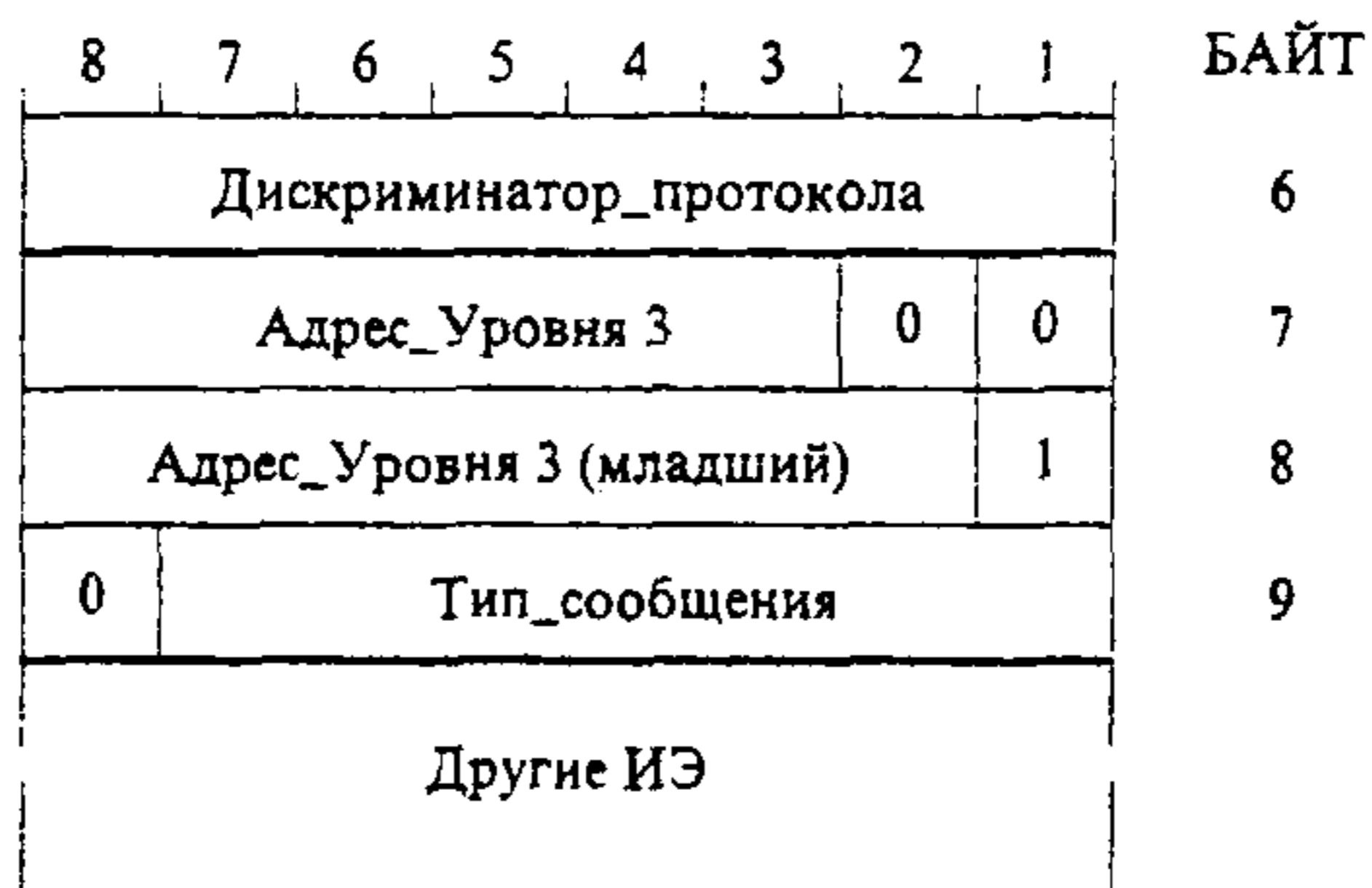
Рисунок 15- Структура кадра сообщения протокола управления
