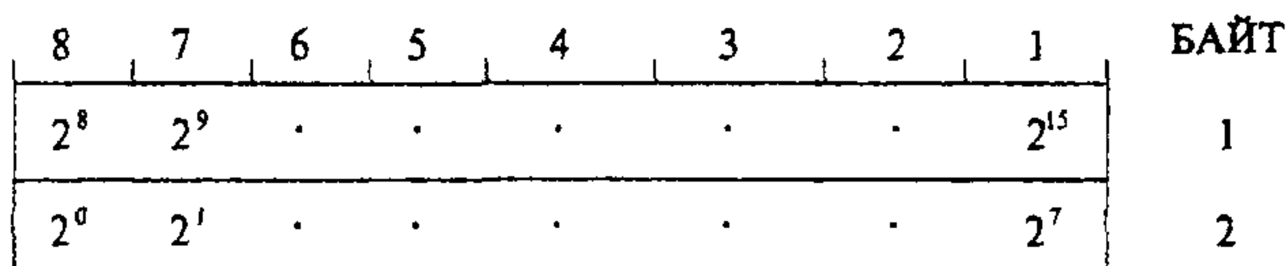
Рисунок 21- Способ размещения битов ППК
