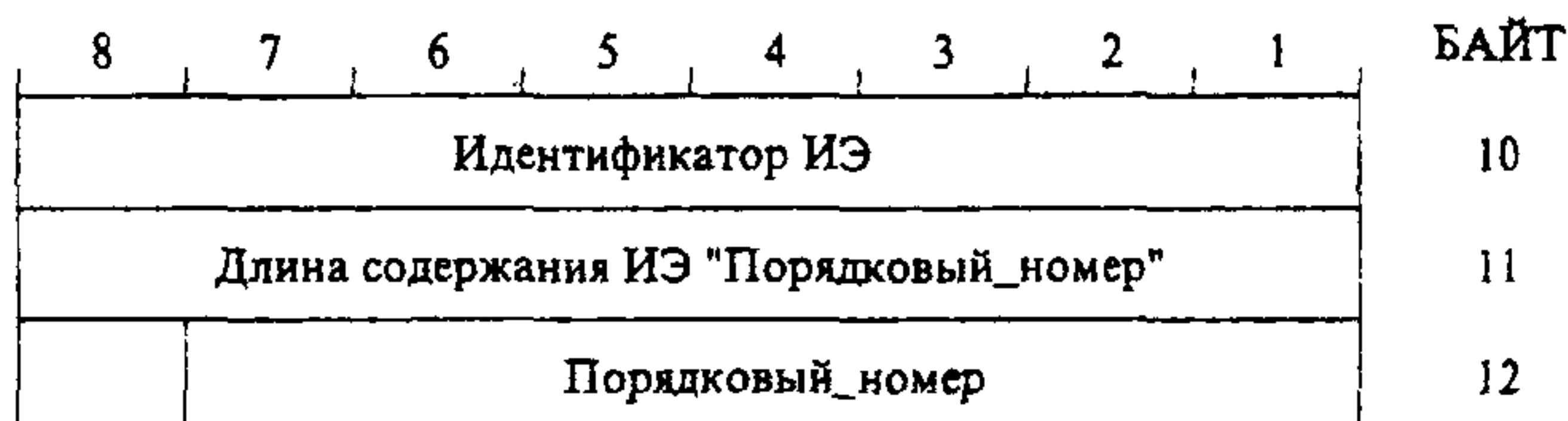
Рисунок 22- Структура ИЭ "Порядковый_номер"
