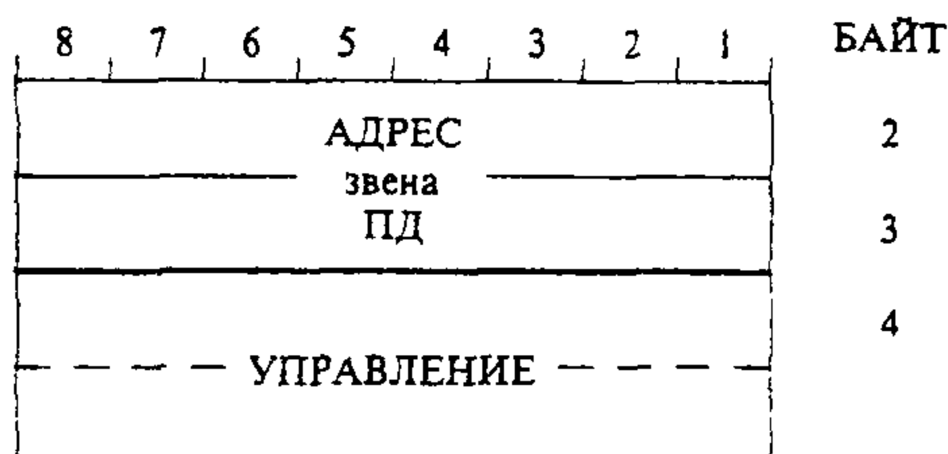
Рисунок 6- Структура А кадра звена ПД с полем “УПРАВЛЕНИЕ”; поле “Информация звена ПД” - отсутствует
