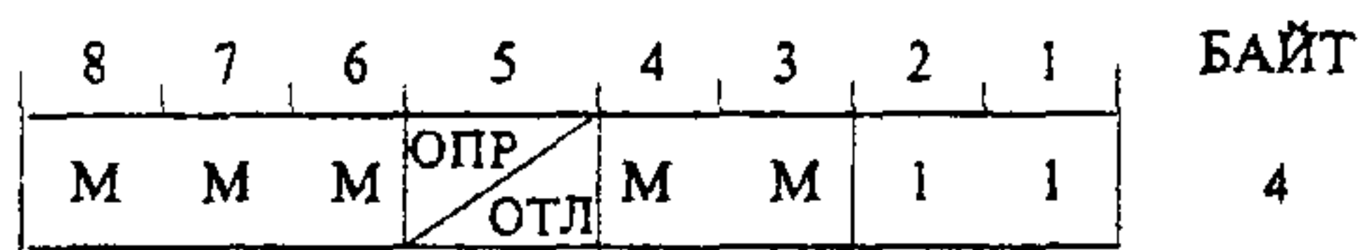
Рисунок 13- Структура “Н-формата”
