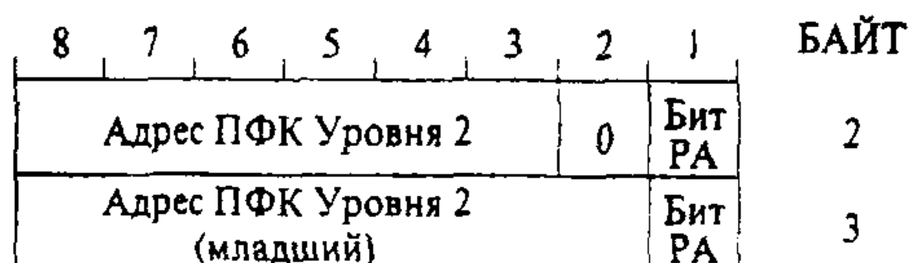
Рисунок 5- Поле адреса ПФК Уровня 2
