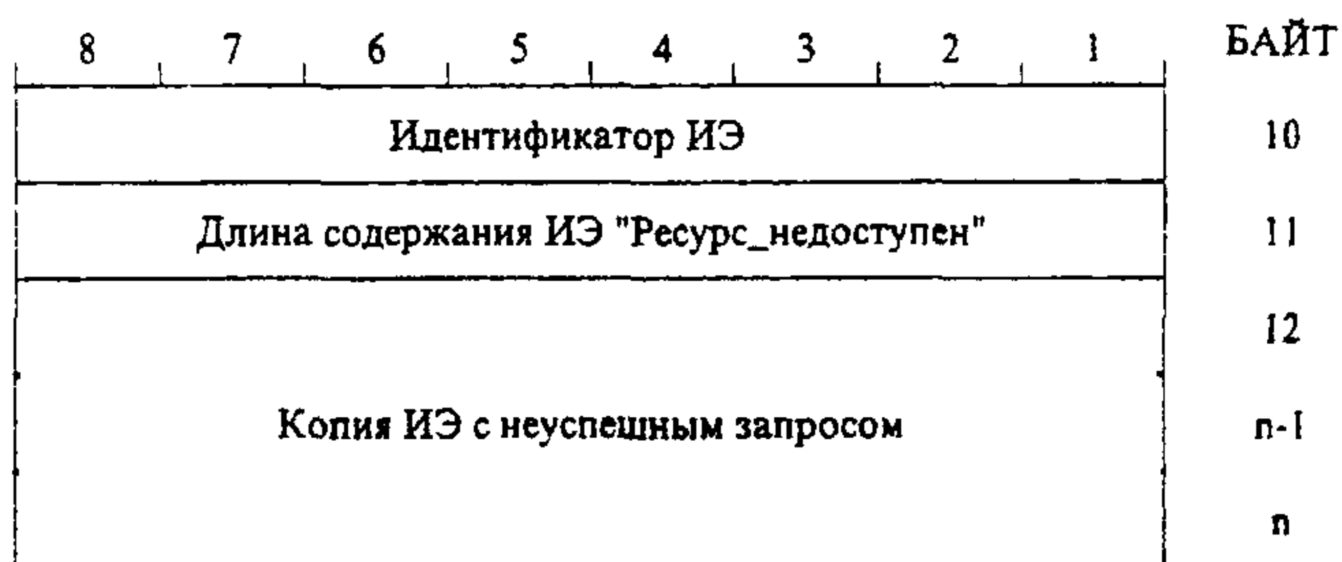
Рисунок 32- Структура ИЭ "Ресурс_недоступен"
