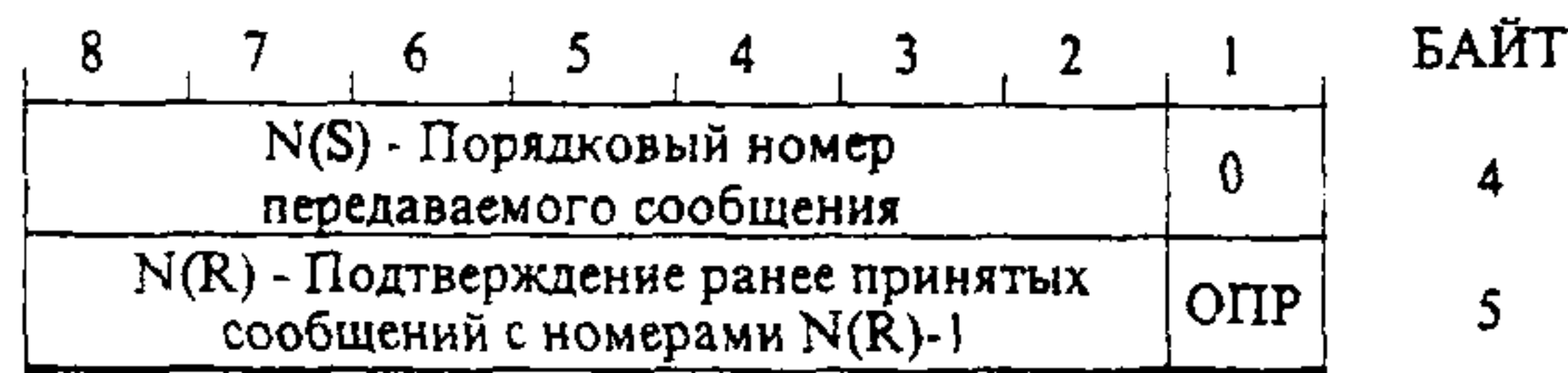
Рисунок 11- Структура “И-формата”
