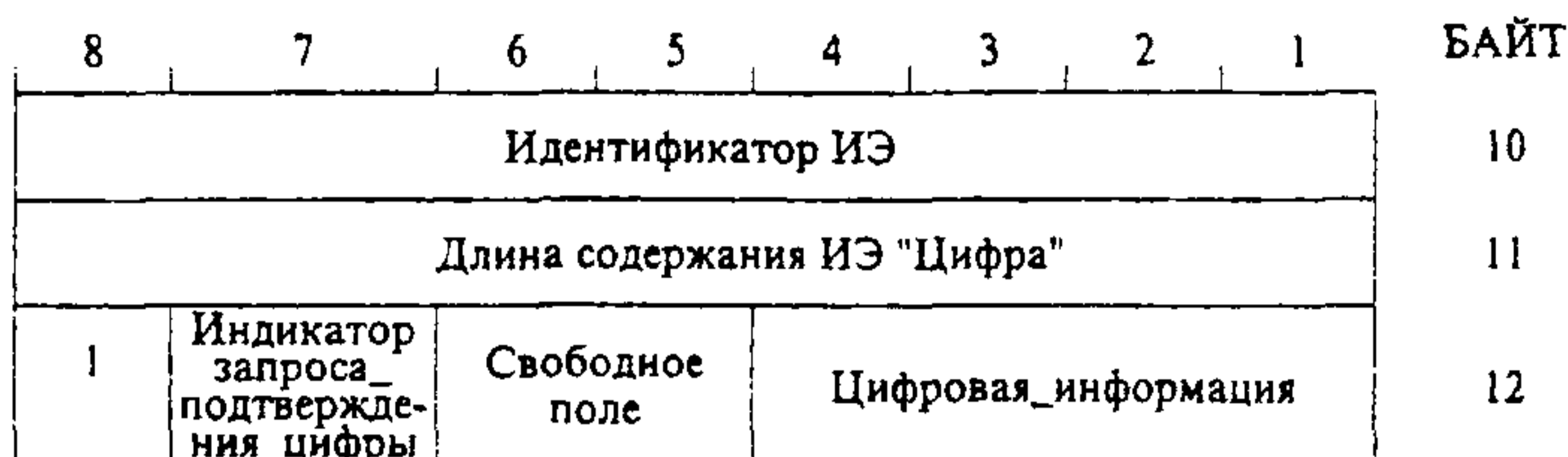
Рисунок 26- Структура ИЭ "Цифра"
