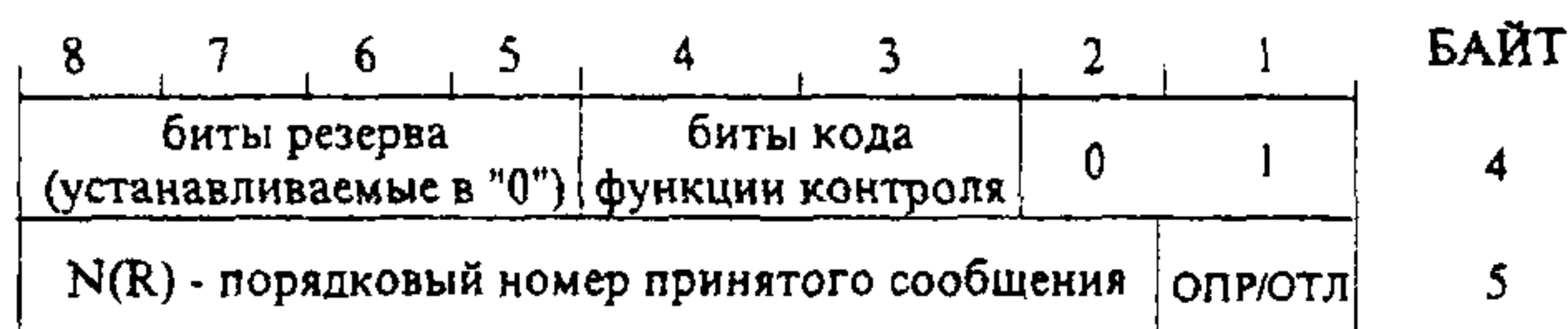
Рисунок 12- Структура “К-формата”
