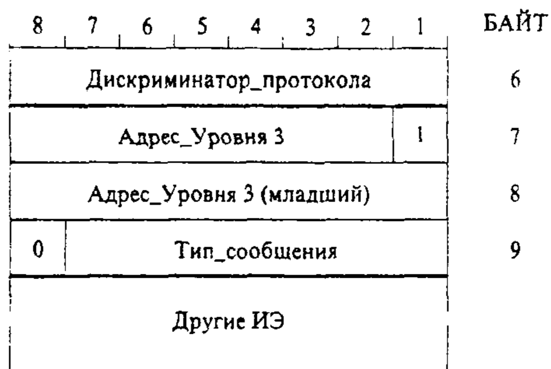
Рисунок 14- Структура кадра сообщения для передачи сигнализации ТФОП
