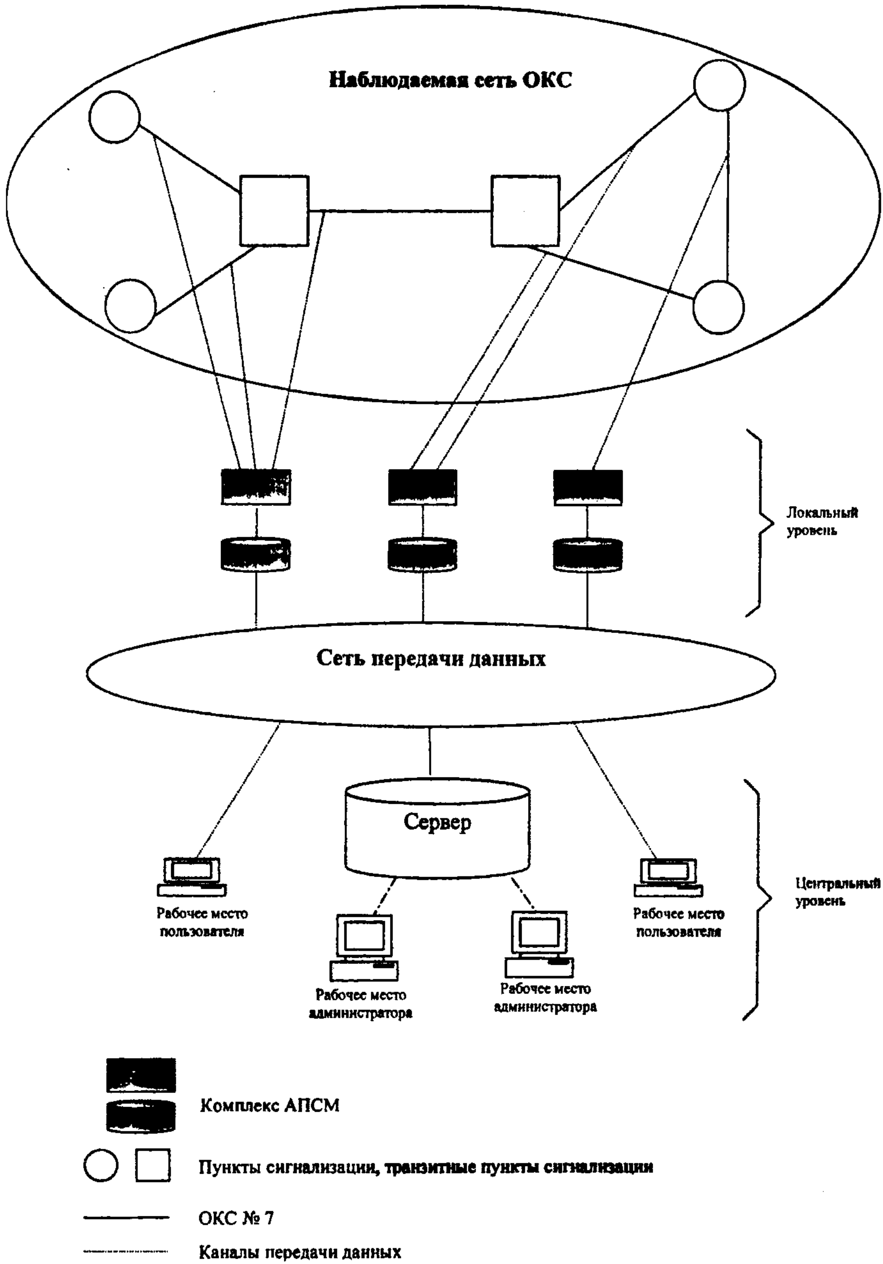
Рис.1. Архитектура комплекса АПСМ сети ОКС 7
