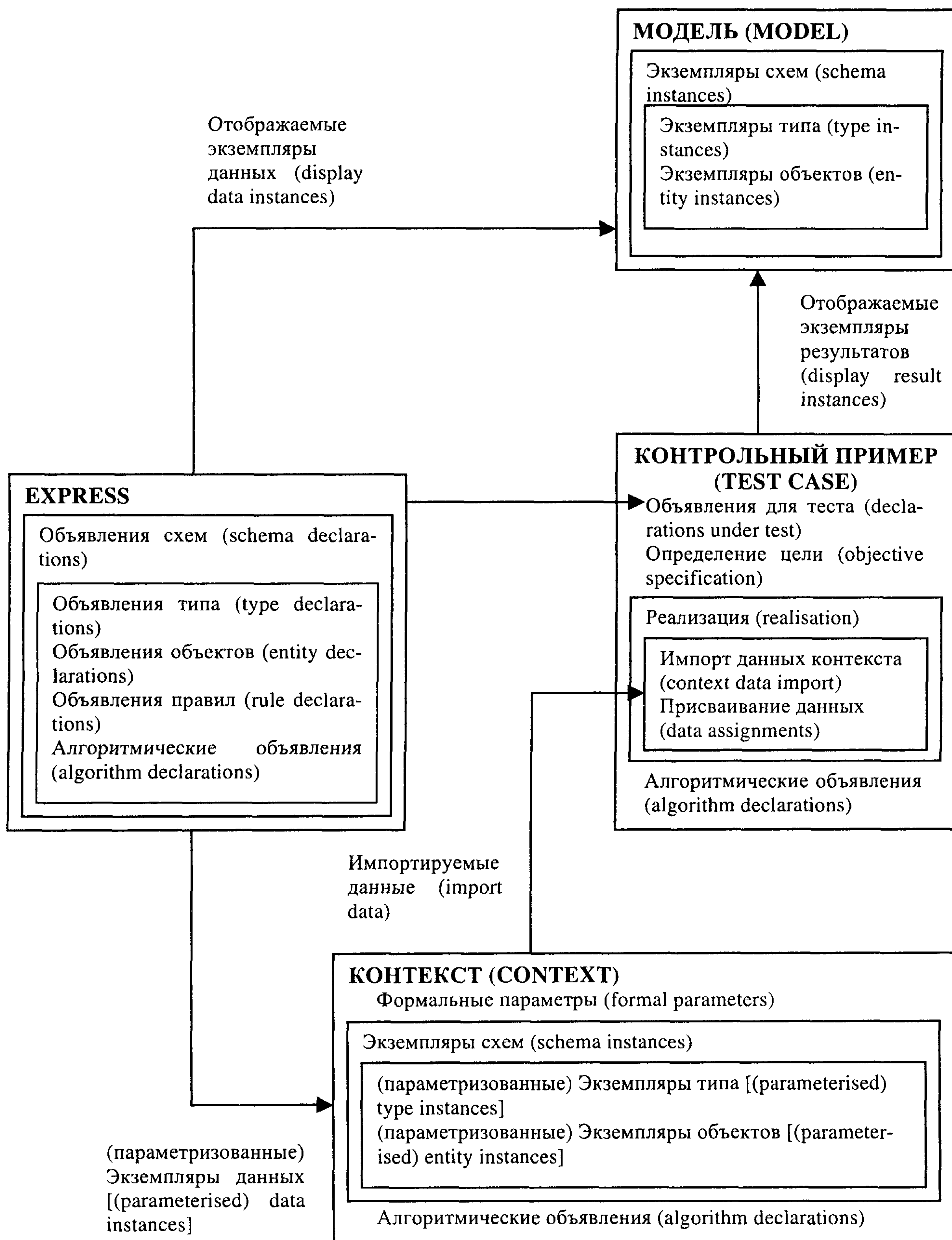
Рисунок 1 – Главные элементы языка EXPRESS-I
