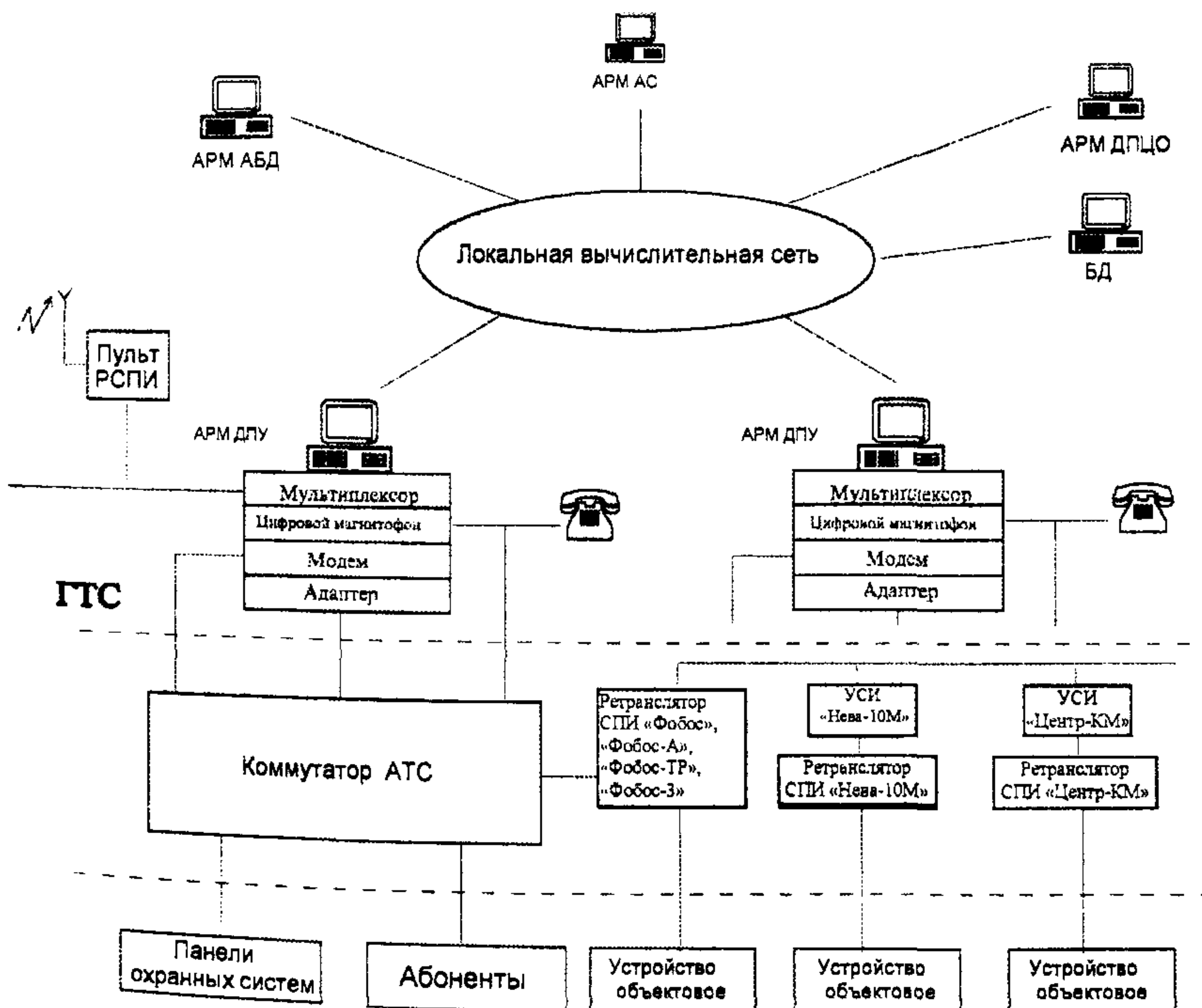
Рисунок 7 - Структурная схема КСА ПЦО
