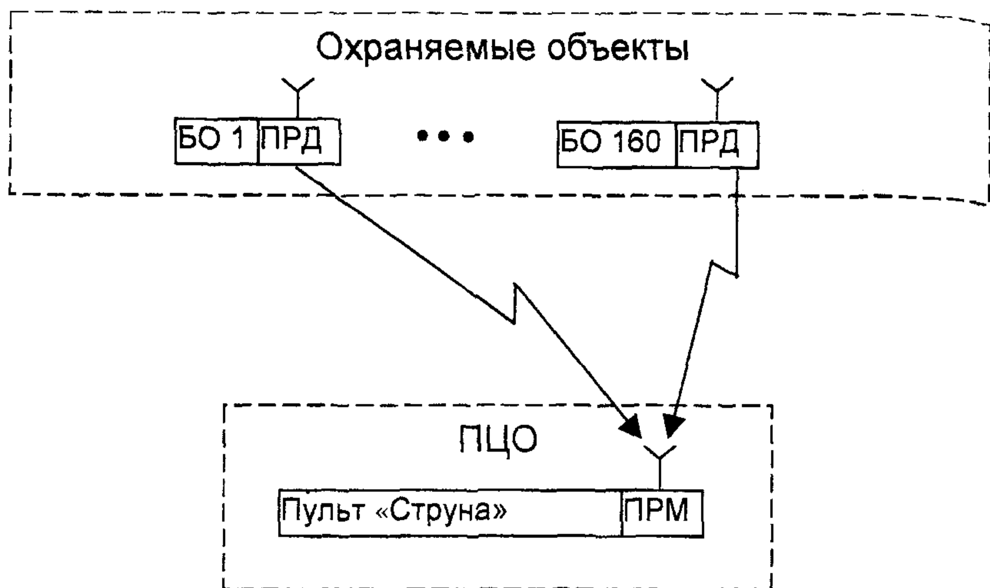
Рисунок 5 – Структурная схема РСПИ «Струна-3»
