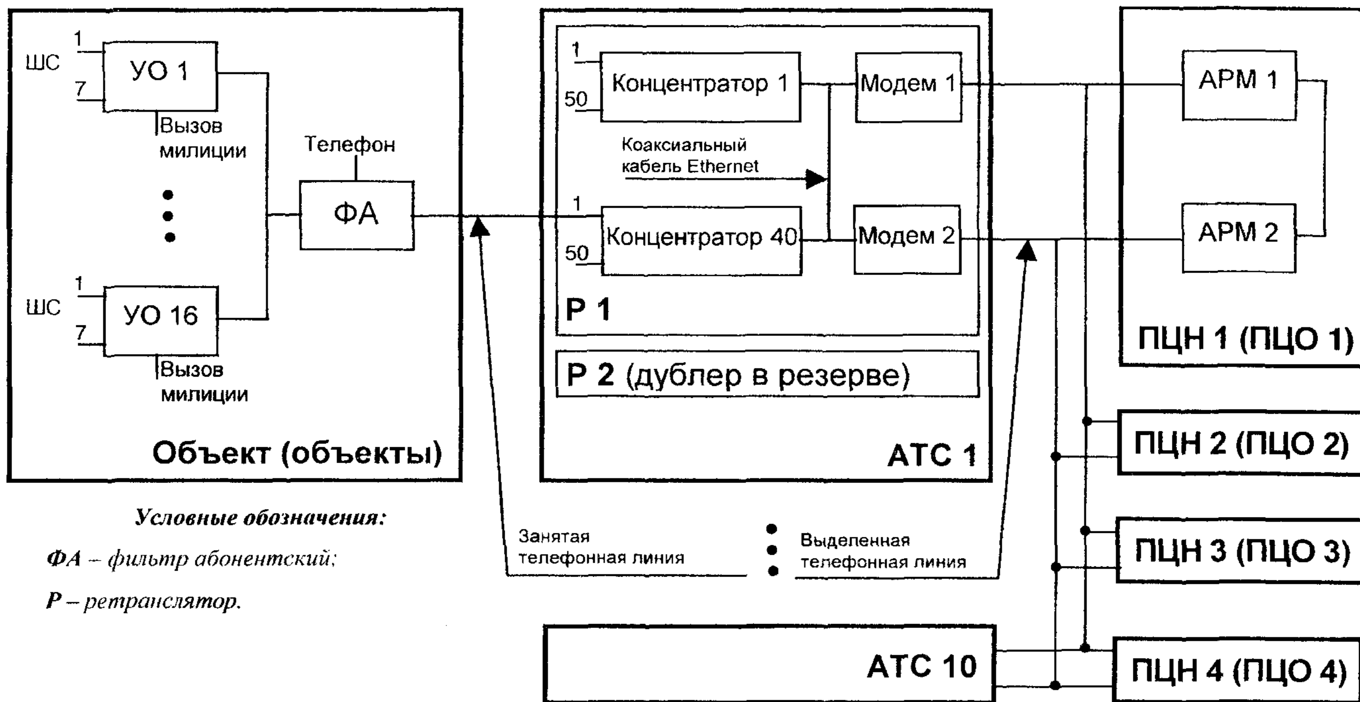
Рисунок 3 - Структурная схема АСПИ «Ахтуба»
