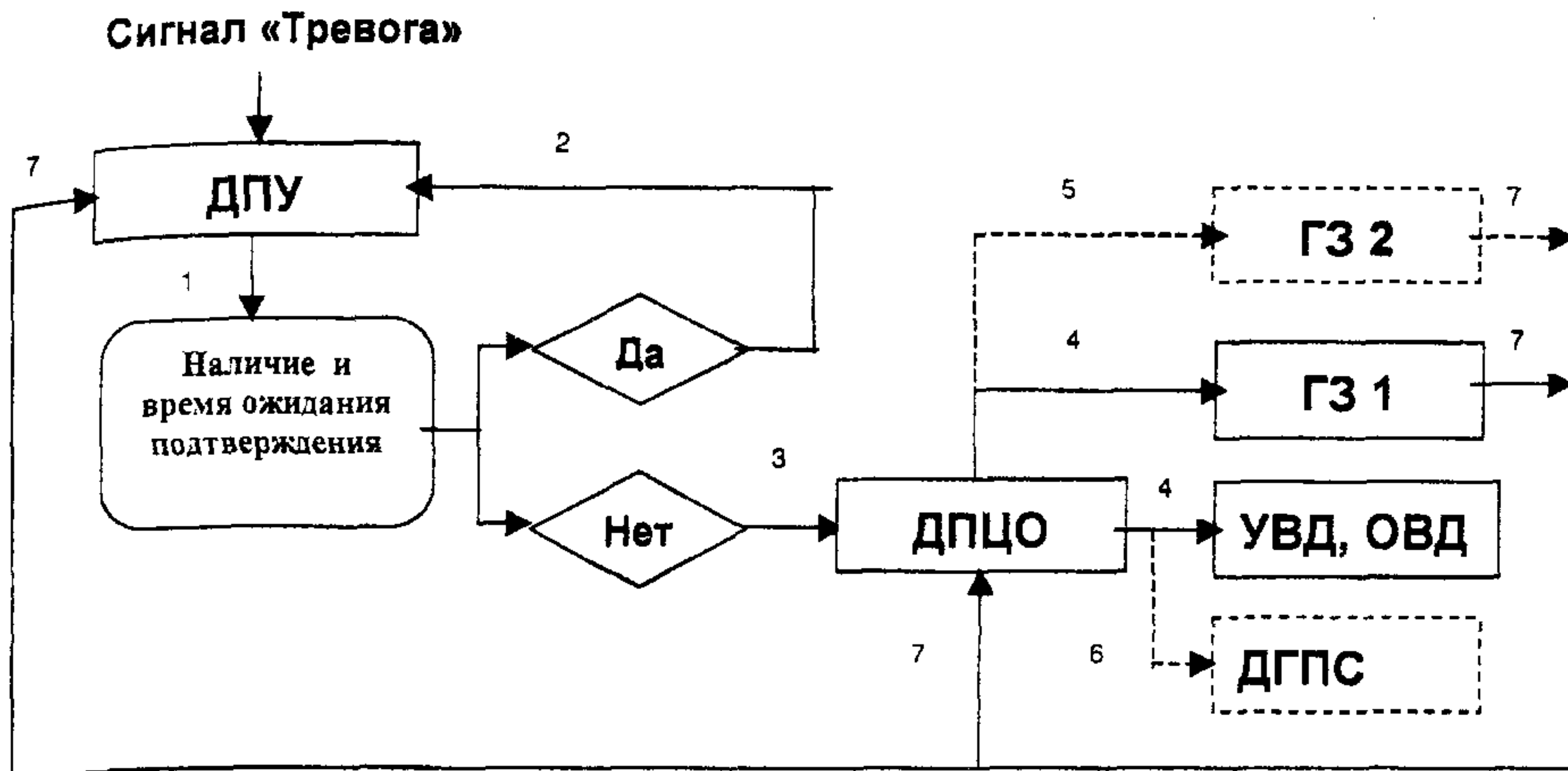
Рисунок 9 – Алгоритм действий
