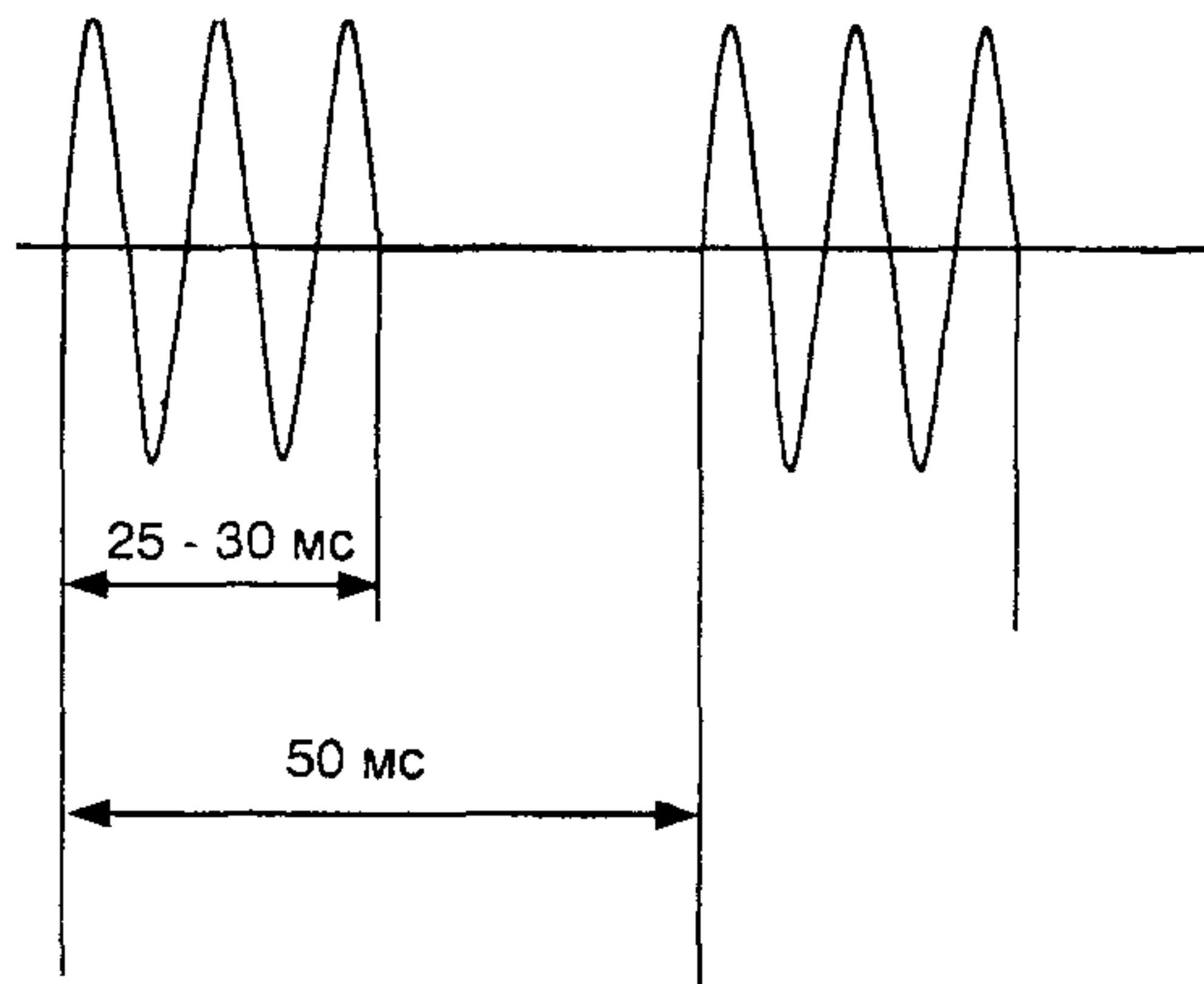
Рисунок А.1 - Радиопульсы движения распределителя ДП
