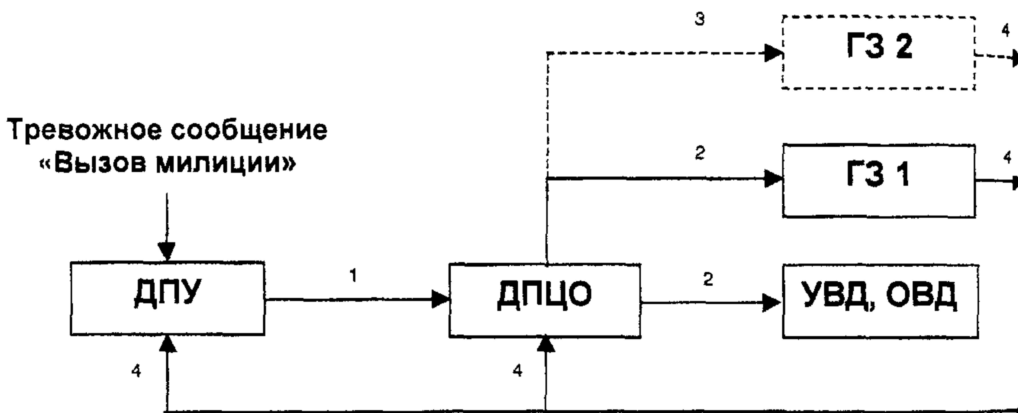
Рисунок 10 – Алгоритм действий
