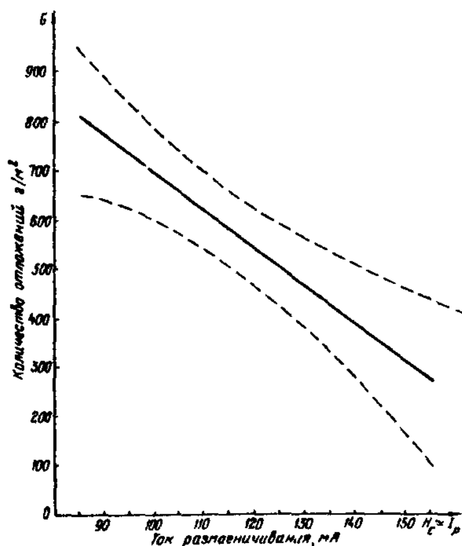
Рис.4. Зависимость количества внутренних эксплуатационных отложений от коэрцитивной силы труб для котлов ТГМ-84 на отметке 6 м
