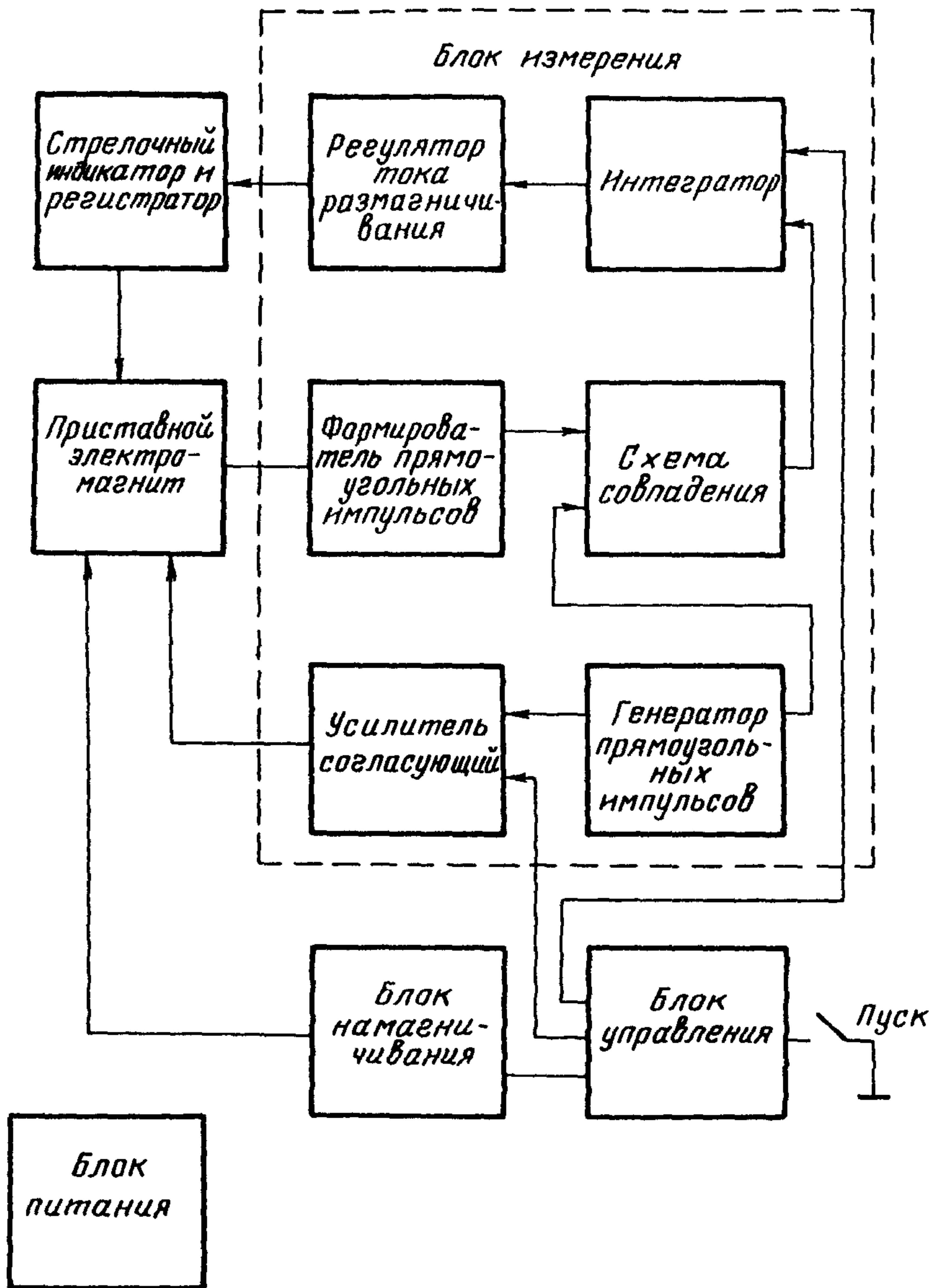
Рис.3. Структурная электрическая схема коэрцитиметра
