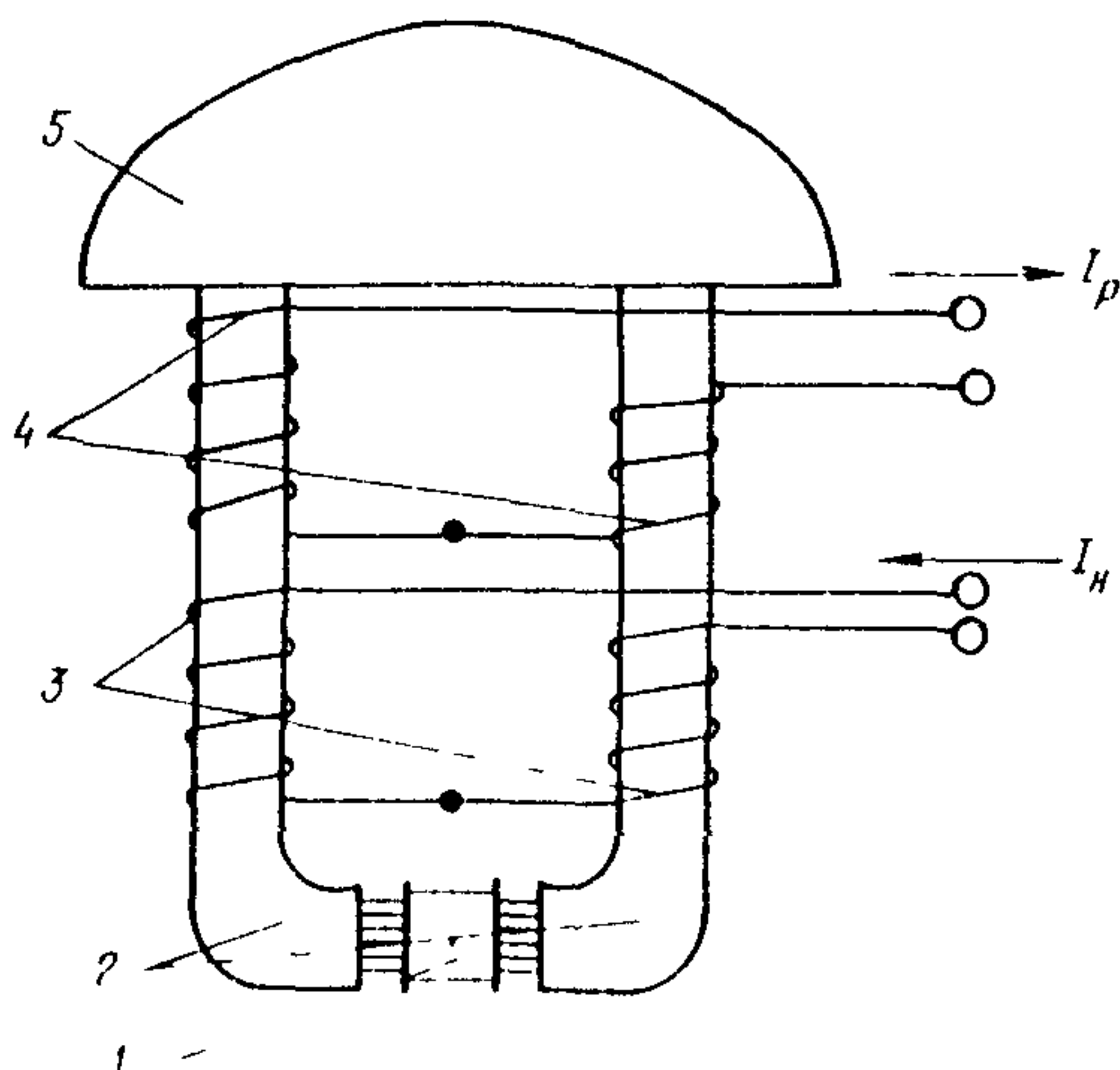
Рис. I. Общая схема приставного электромагнита:
