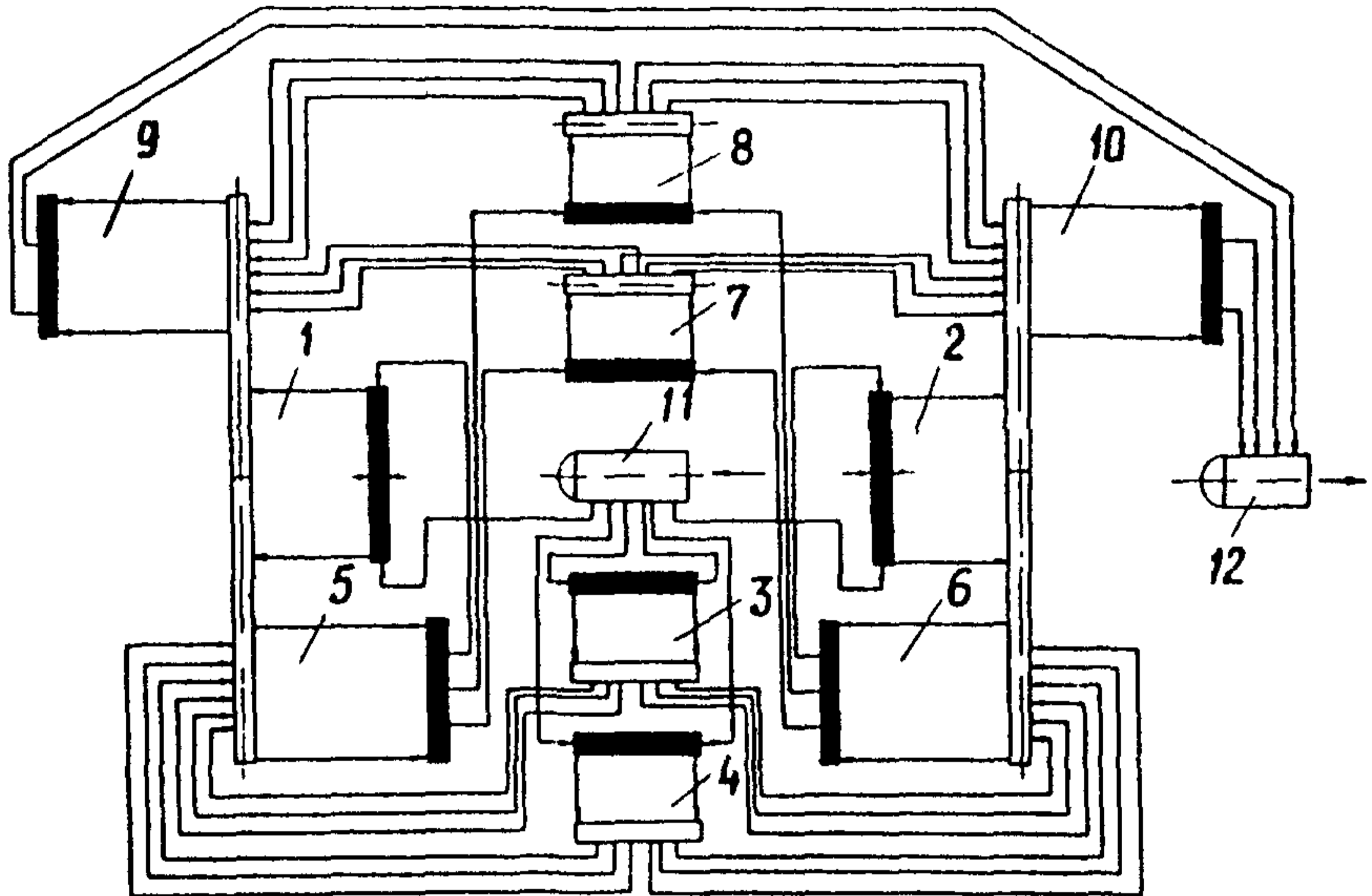
Рис. П1.1. Гидравлическая схема водогрейного котла КВГМ-180-150 (основной режим):
