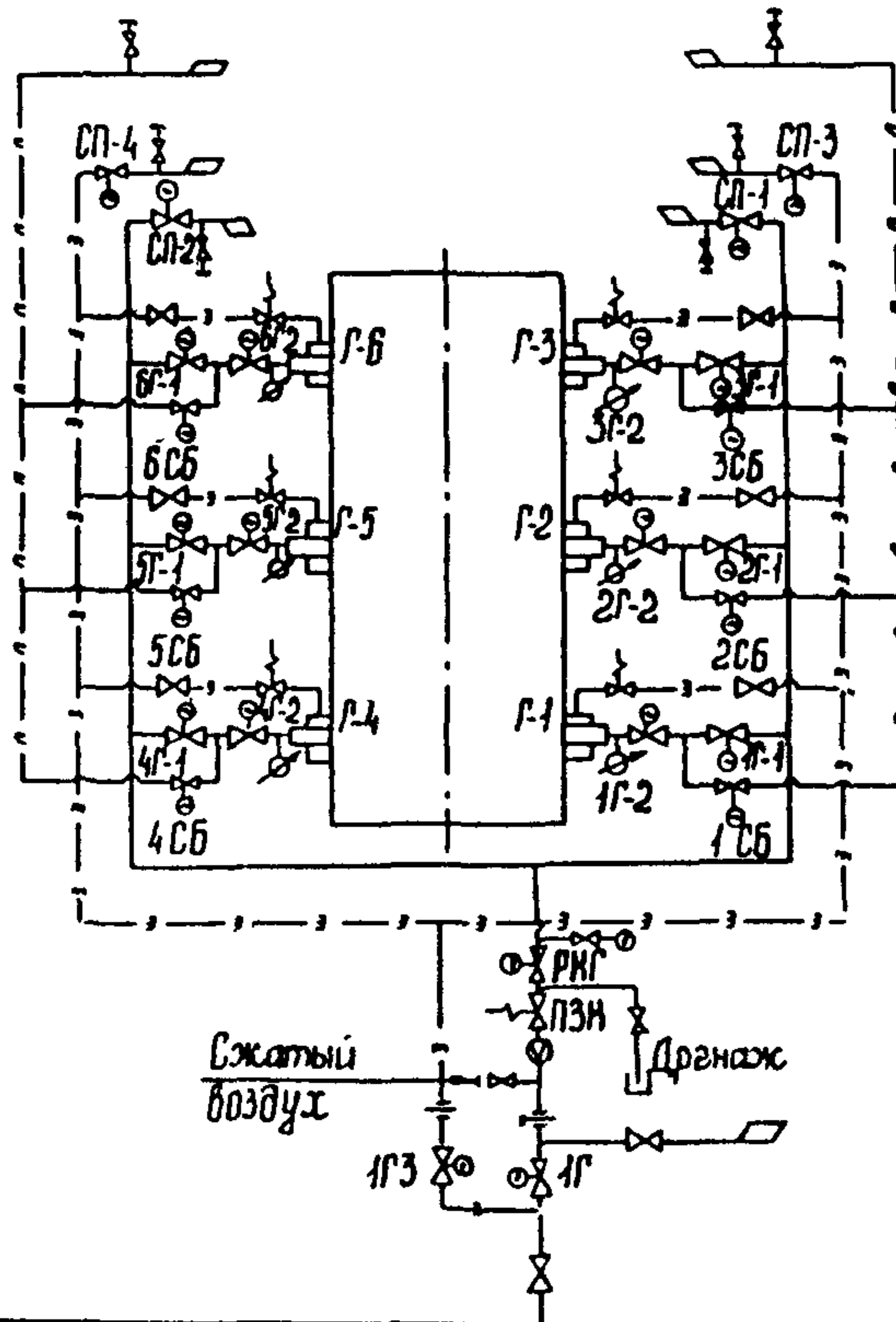
Рис. 3. Схема газопроводов котла КВГМ-180:
