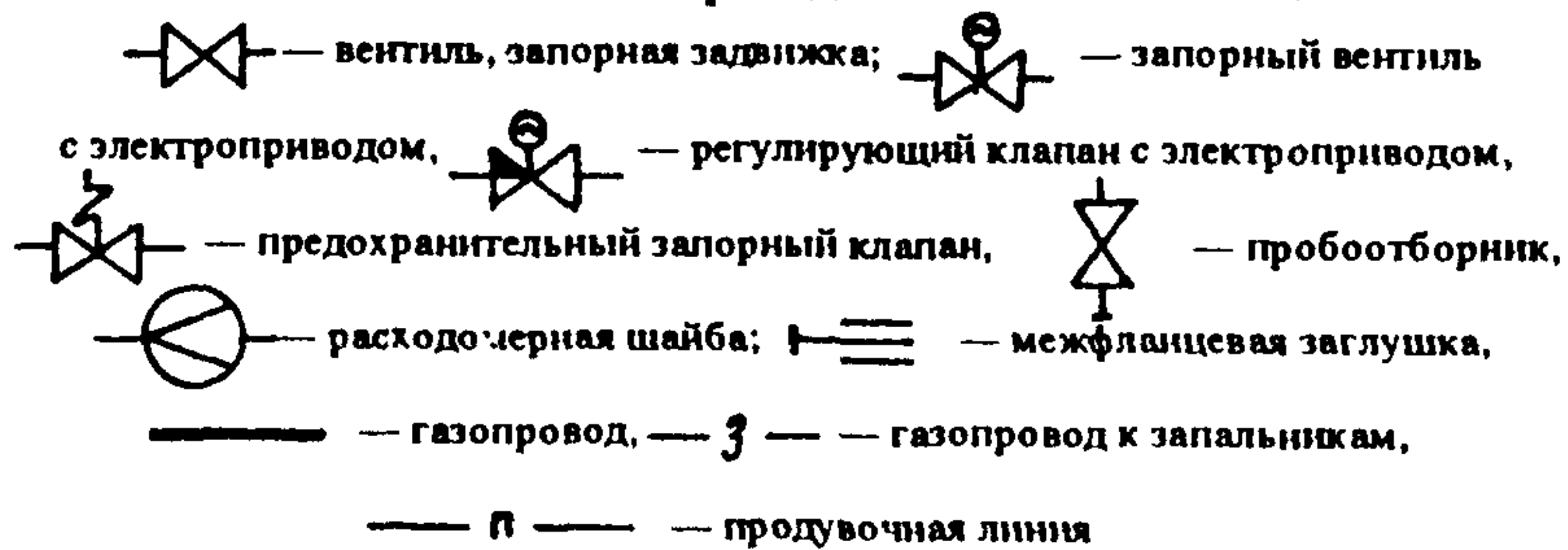
Рис. 3. Схема газопроводов котла КВГМ-180:
