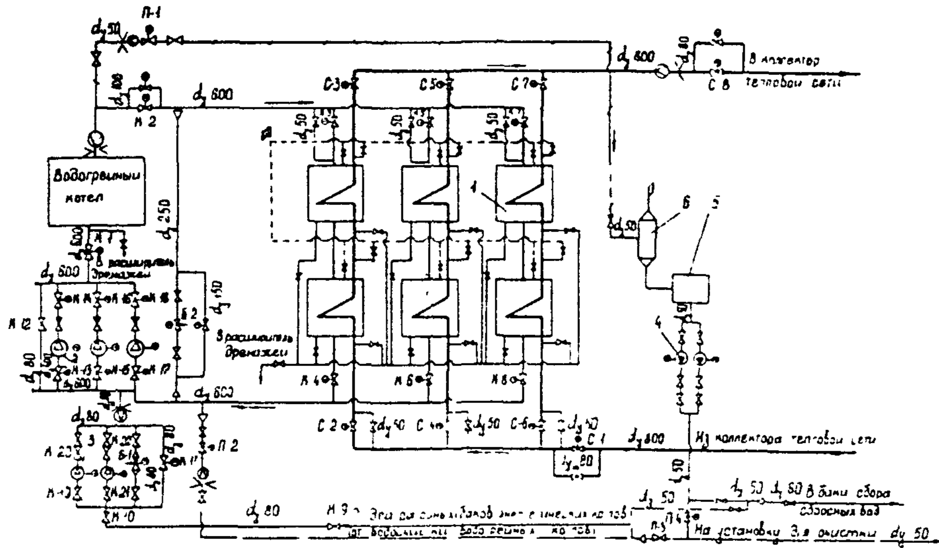
Рис. 1. Тепловая схема котла с внешним теплообменником:
