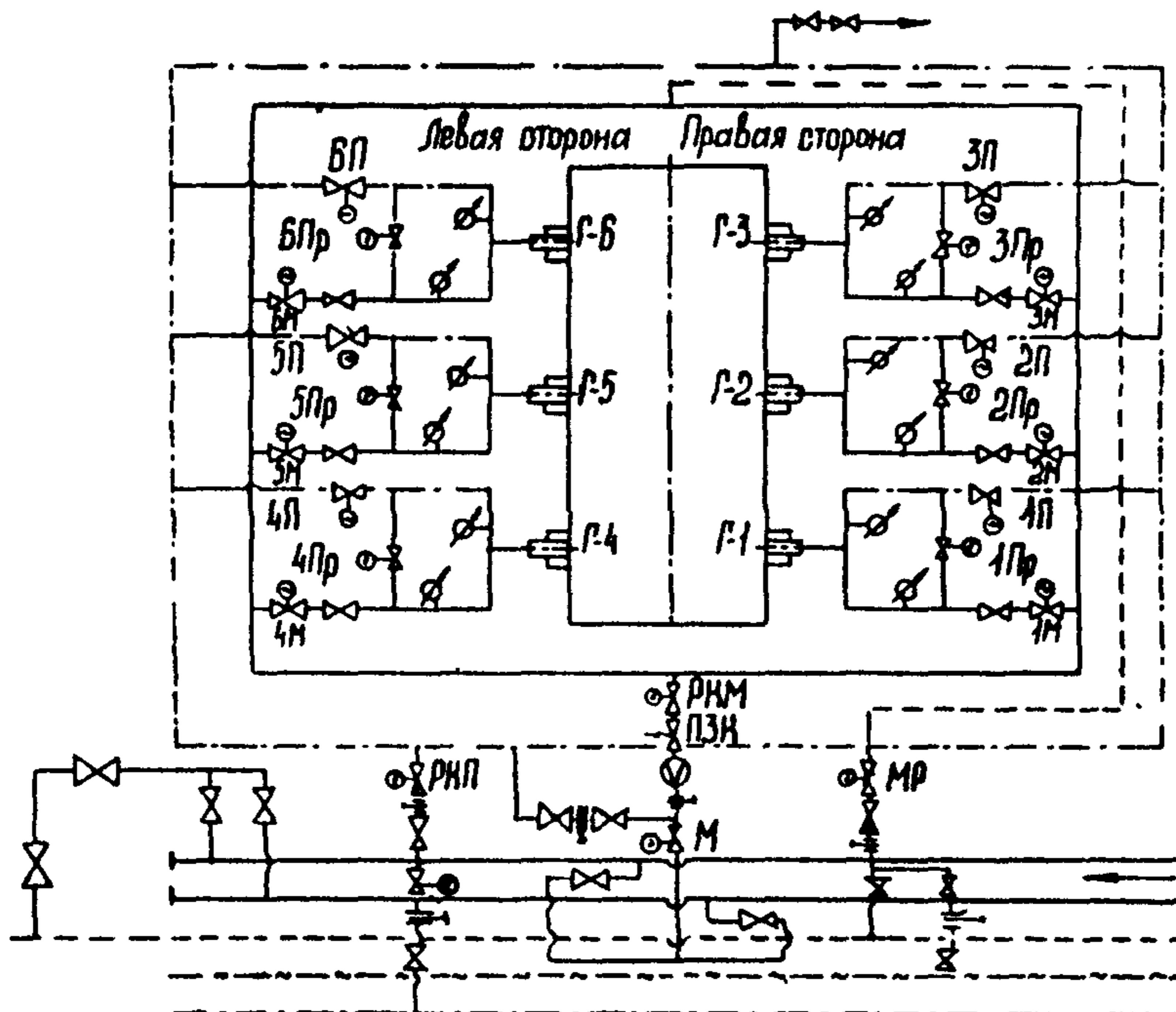
Рис. 2. Схема паромазутопроводов котла КВГМ-180:
