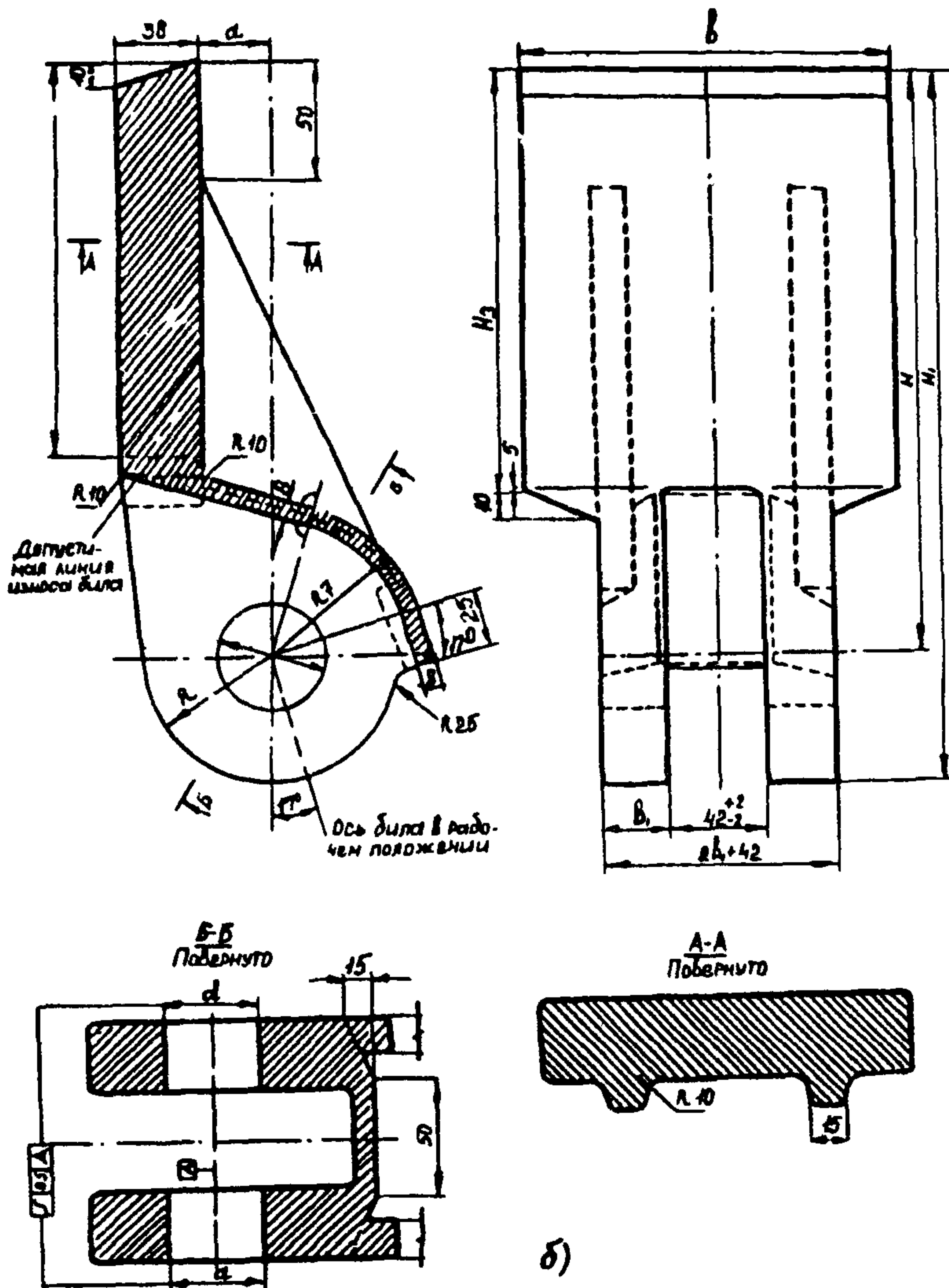
Рис. П2.3. Унифицированное било:
