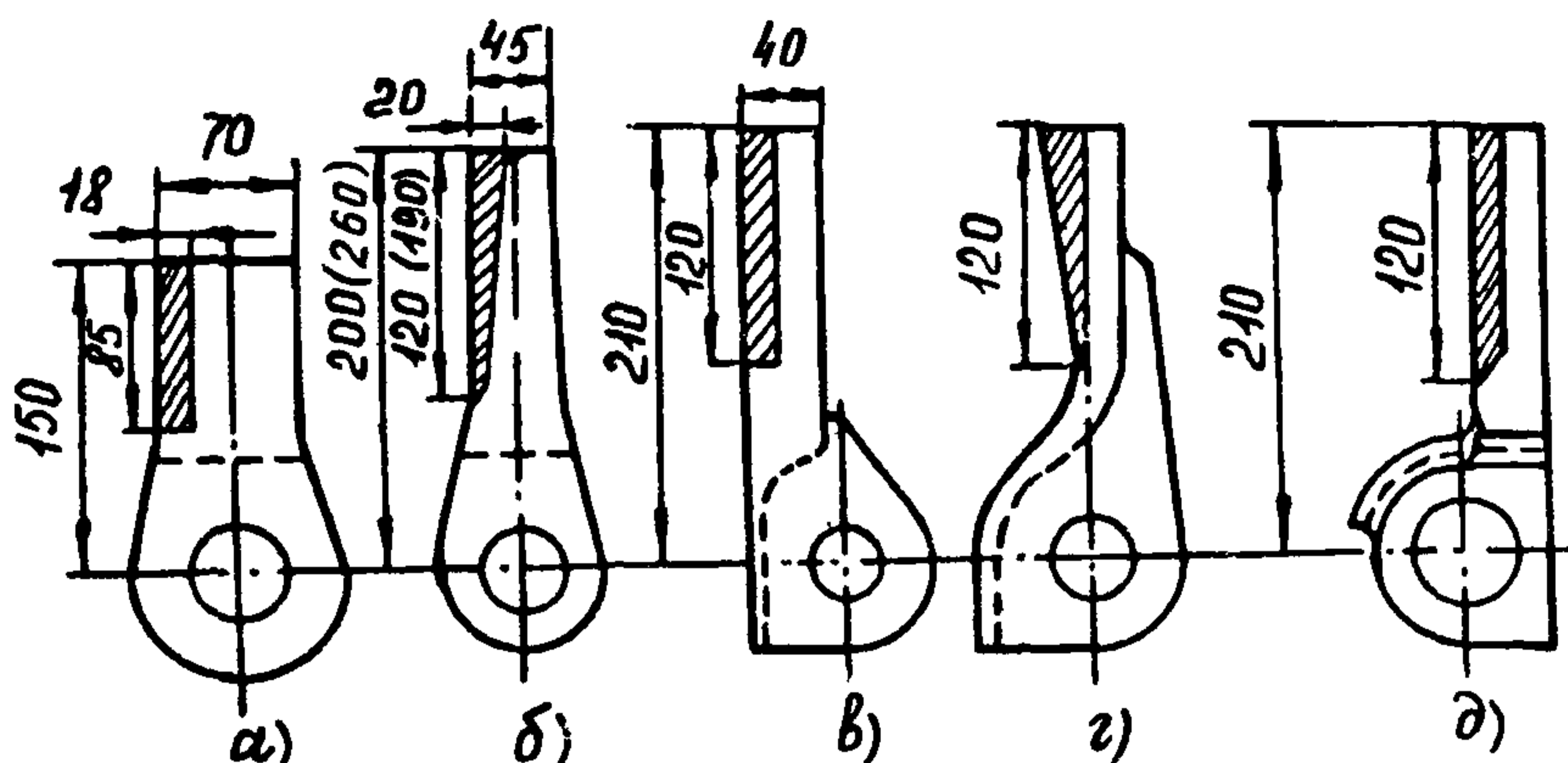
Рис. П2.2. Конструкции бил, применяемых для оснащения молотковых мельниц:
