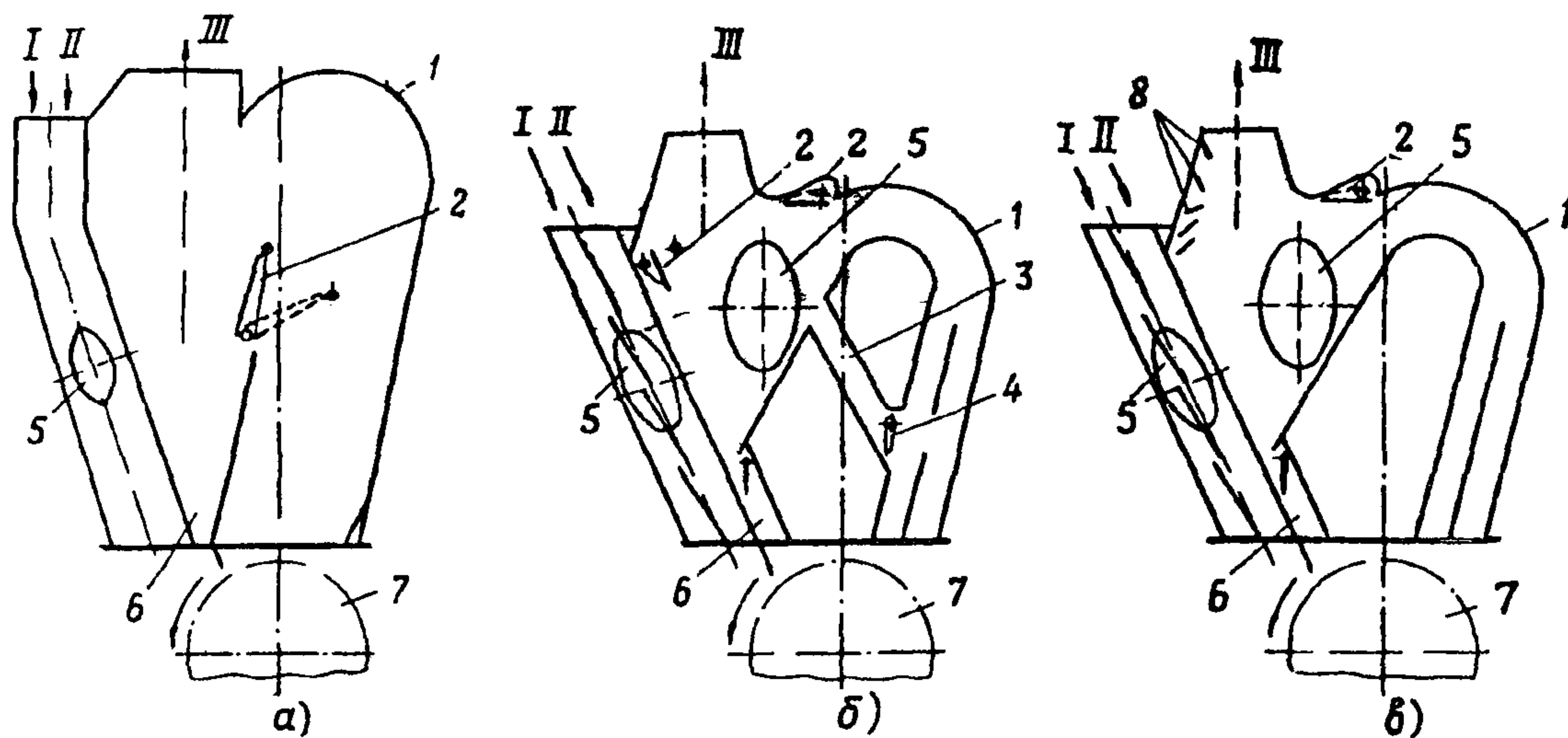
Рис. П2.4. Инерционный сепаратор пыли:
