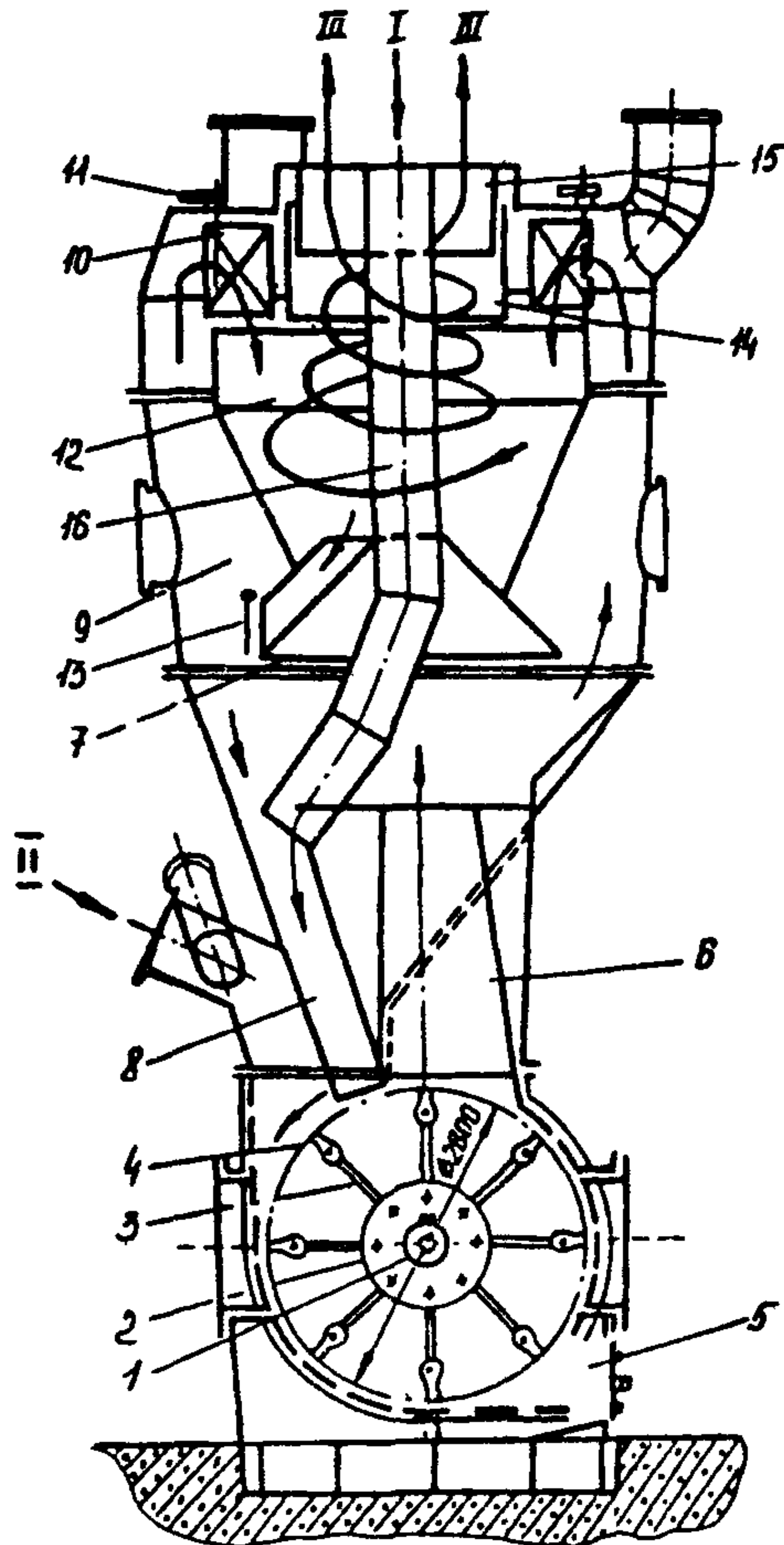
Рис. П2.1. Схема молотковой мельницы ММТ 2600/2550/590К:
