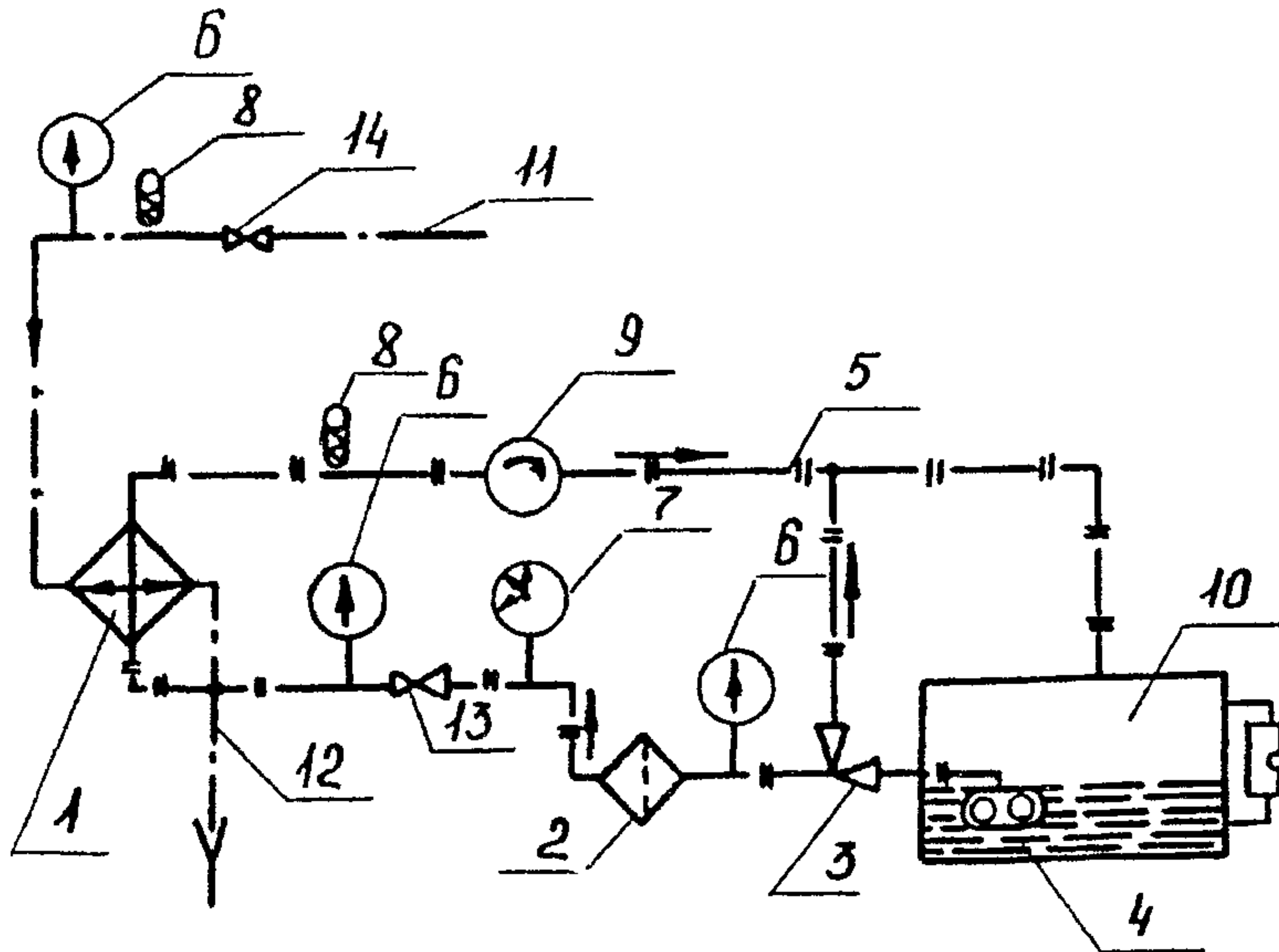
Рис. 4. Принципиальная схема жидкой смазки редуктора:
