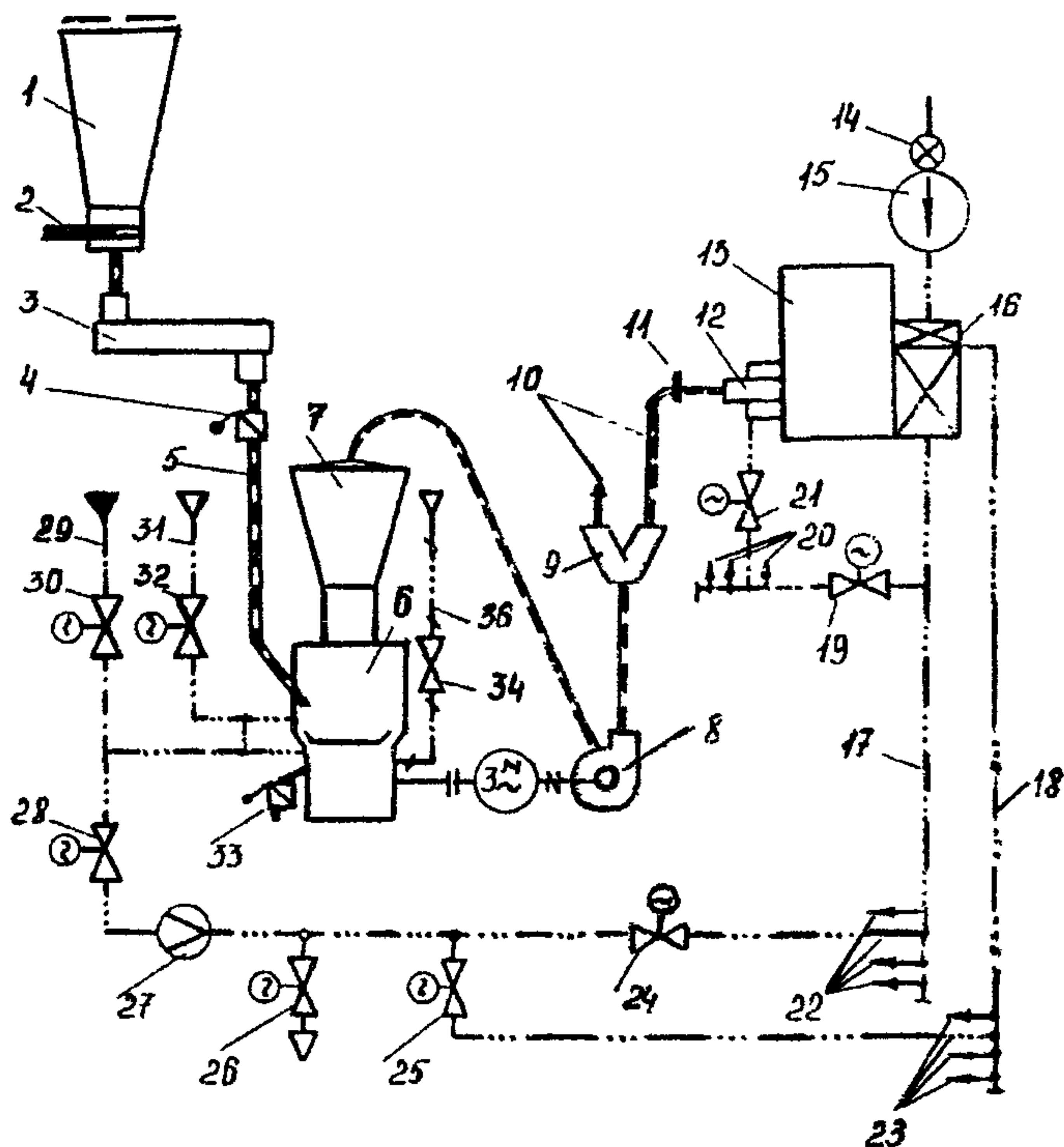
Рис. 1. Схема системы пылеприготовления с мельницей типа МВС для работы под разрежением:
