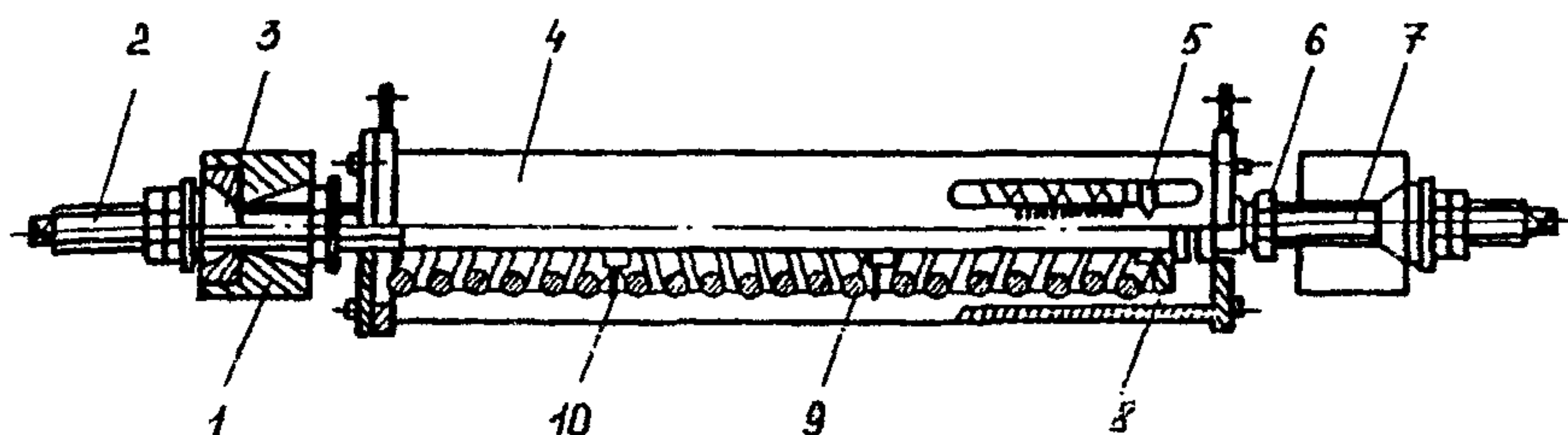
Рис. П1.5. Нажимное устройство — пружинный блок:
