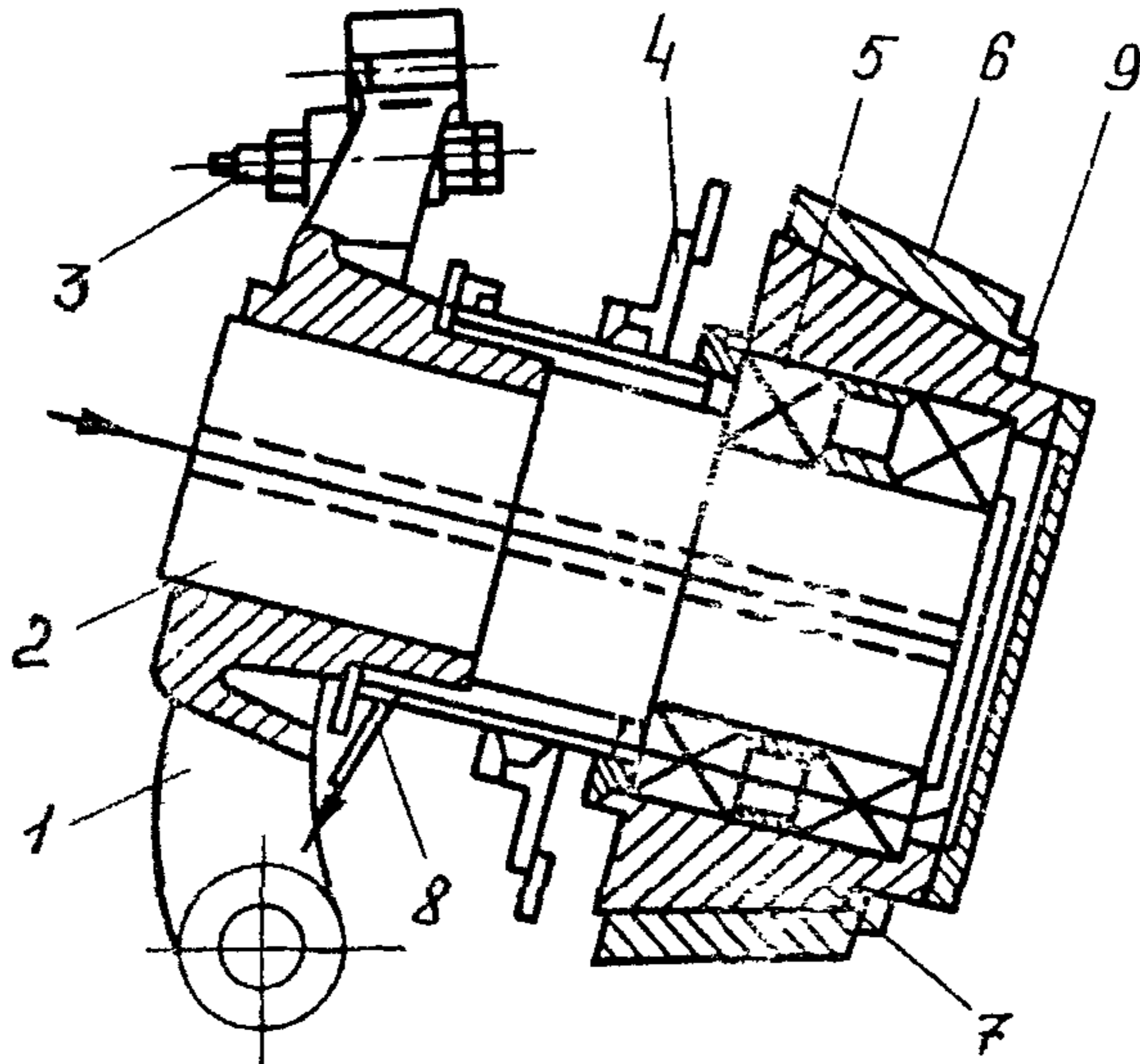
Рис. П1.2. Размольный валок:
