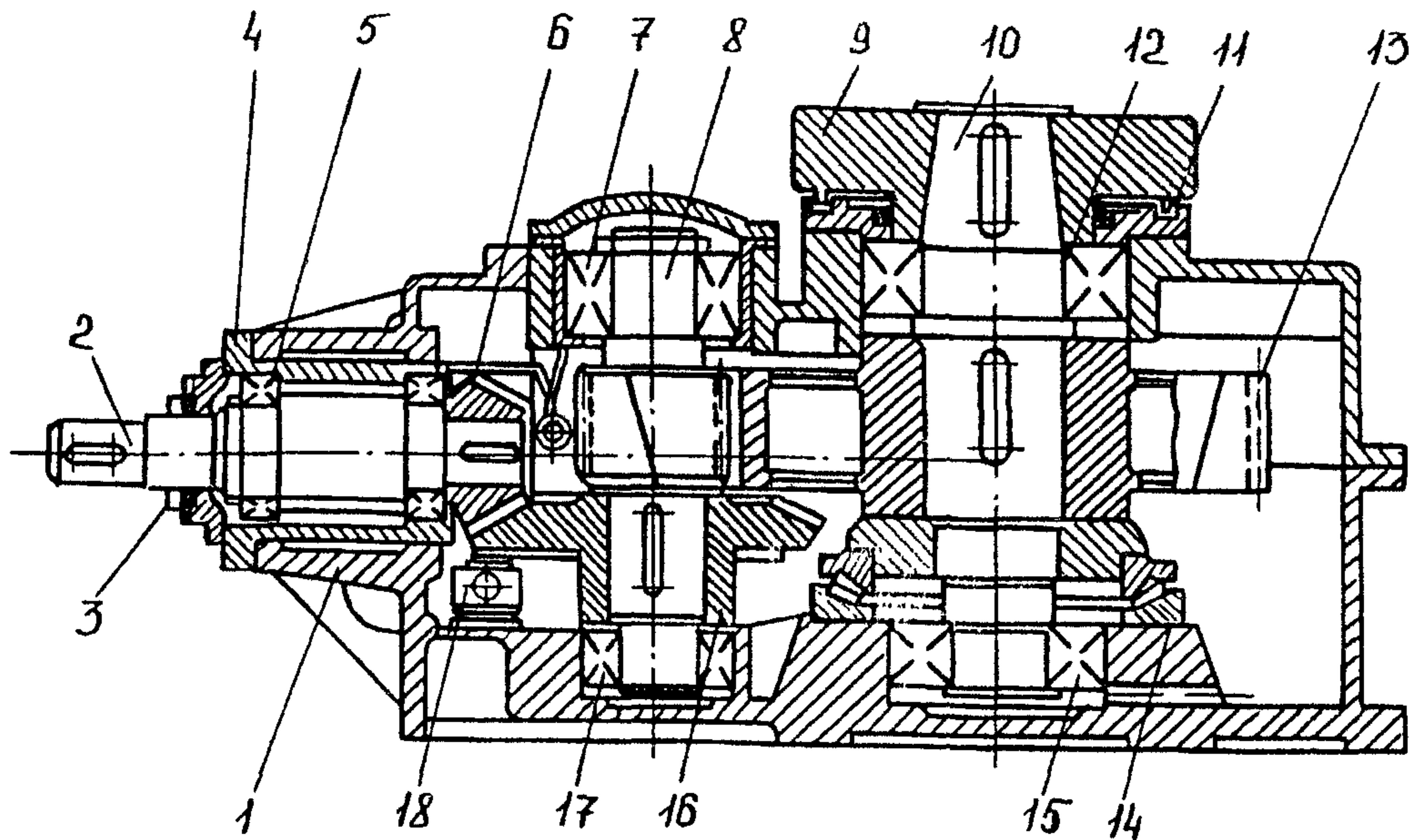
Рис. П1.3. Редуктор:
