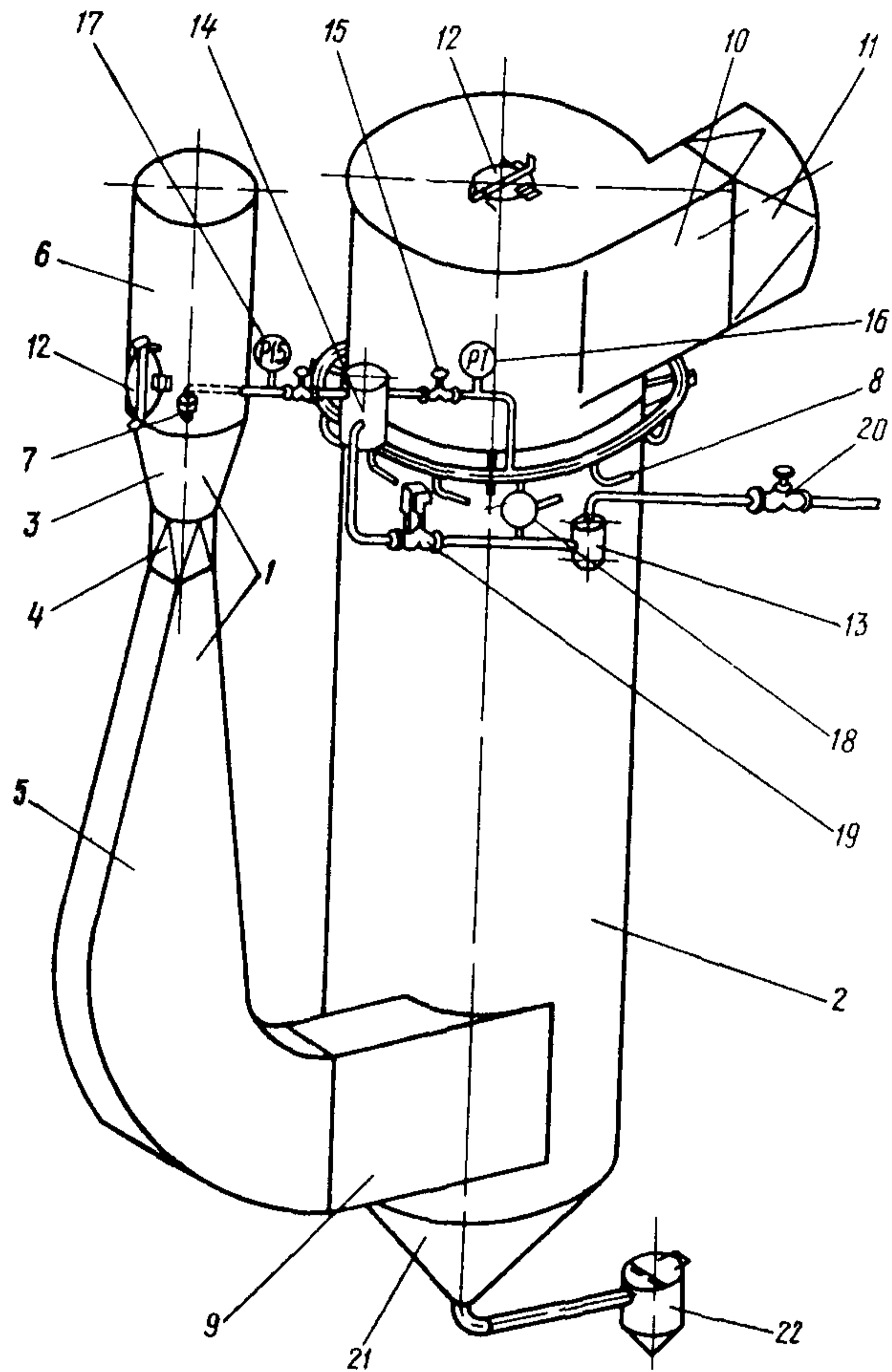
Рис. I. Скруббер:
