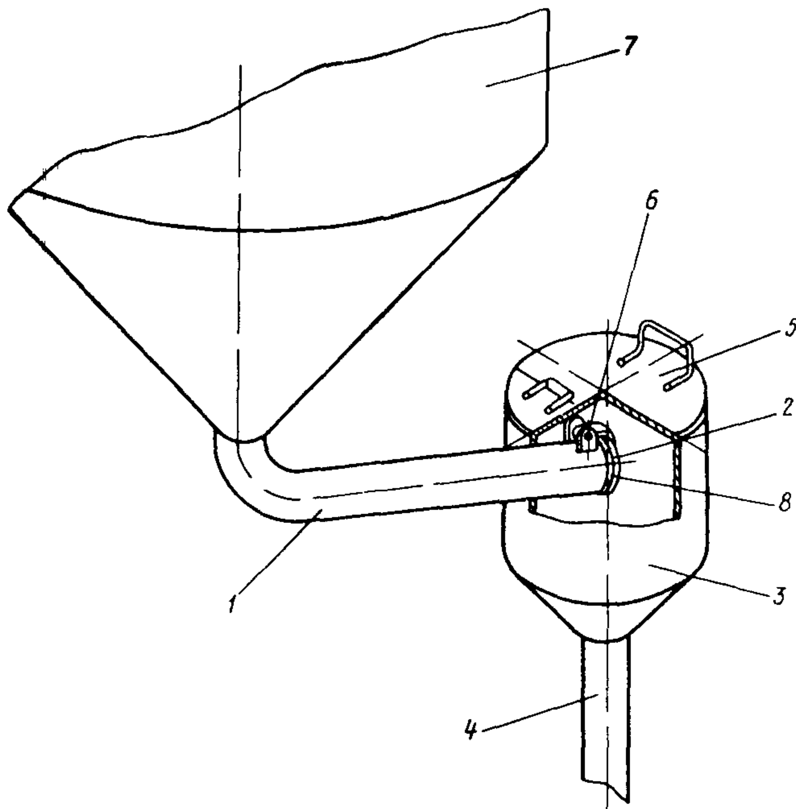
Рис. 2. Гидрозатор:
