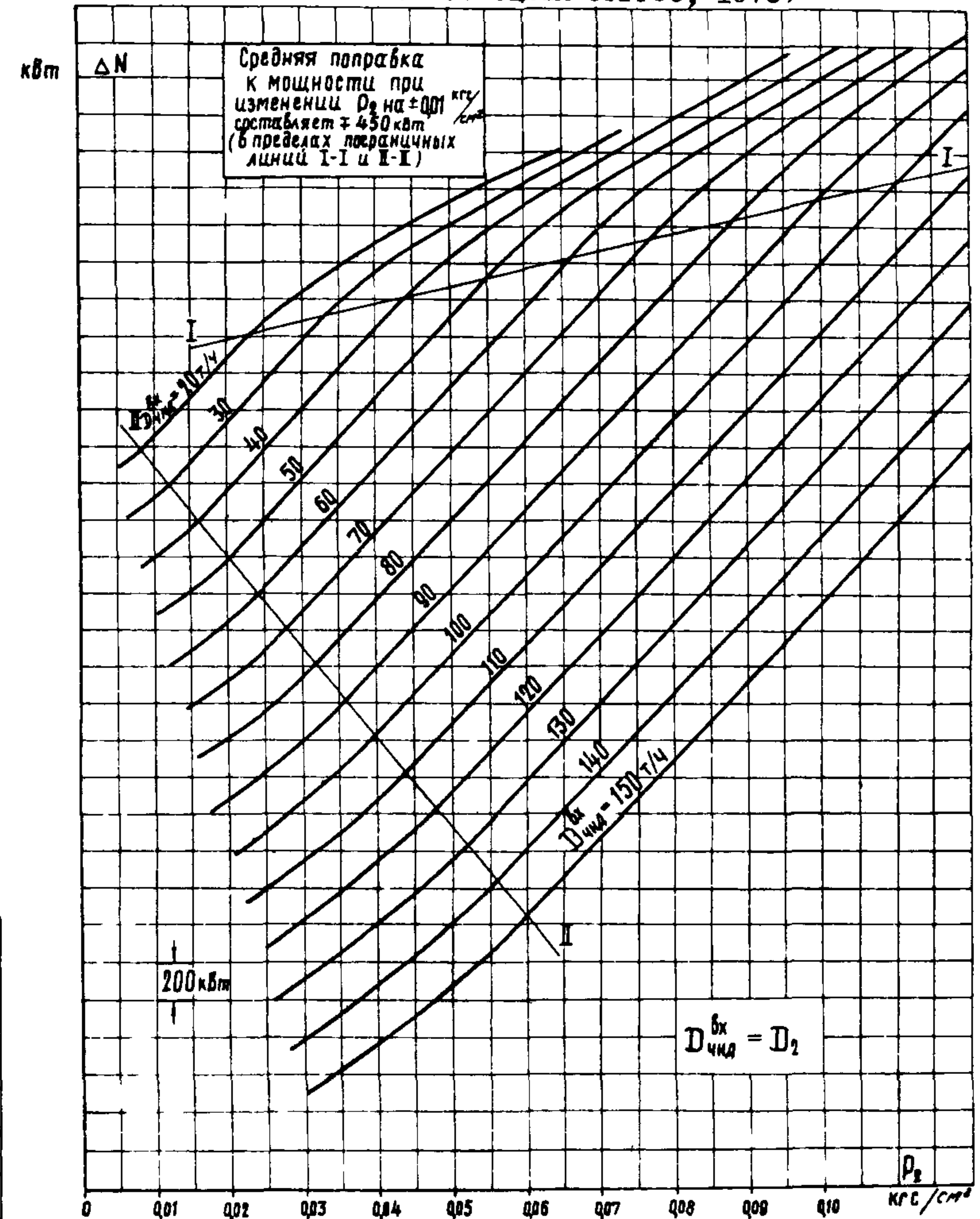
Рис. П-8. Поправки к мощности турбины ПТ-60-130/13 ЛМЗ на отклонение давления пара в конденсаторе (по данным "Типовой нормативной характеристики турбоагрегата ПТ-60-130/13 ЛМЗ". М.: СИНТИ ОГРЭС, 1975)
