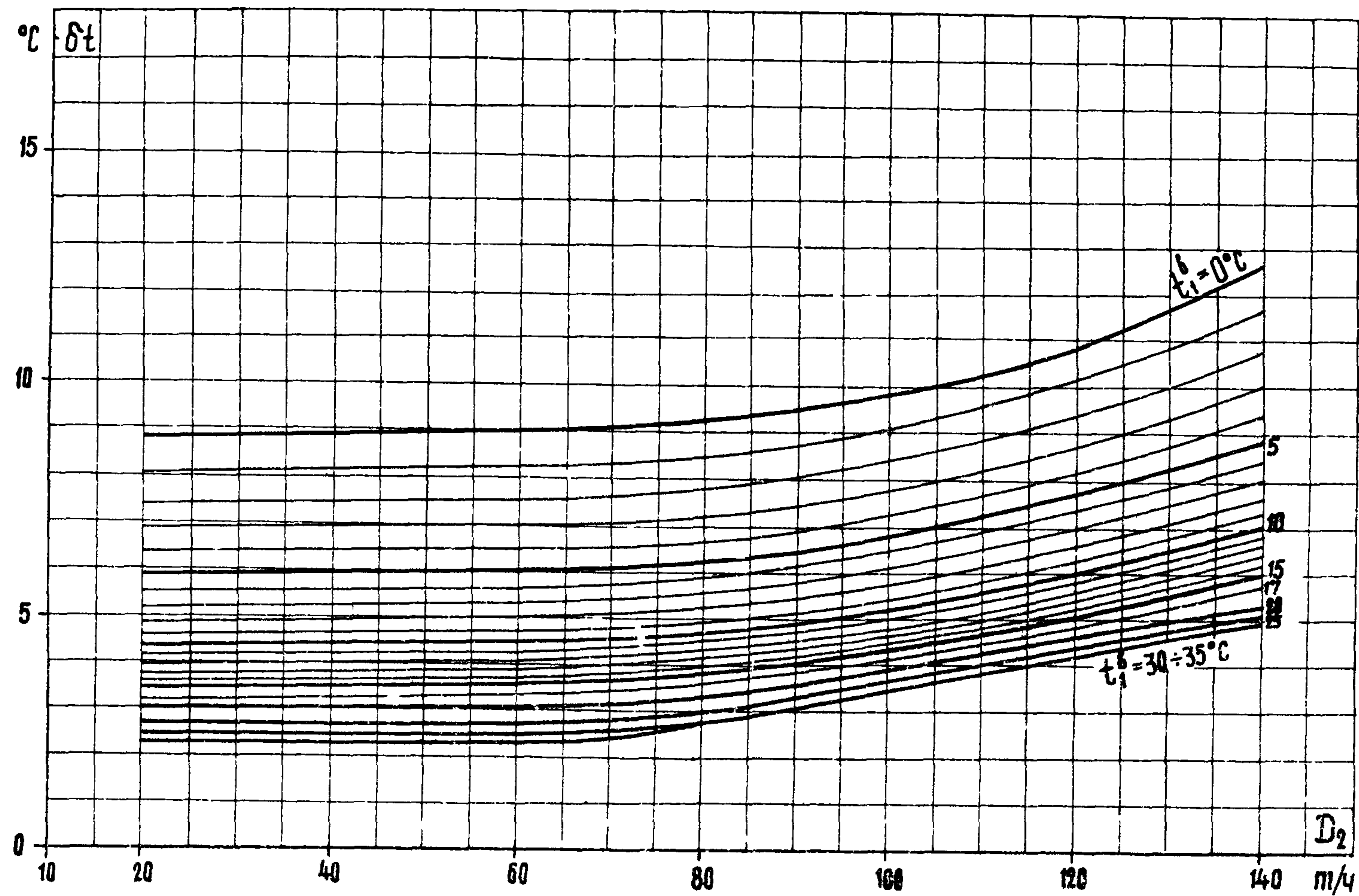
Рис. I-2. Зависимость температурного напора от расхода пара в конденсатор и температуры охлаждающей воды: W = 5000 \text{ м}^3/\text{ч} ; F_{\text{п}} = 3000 \text{ м}^2
