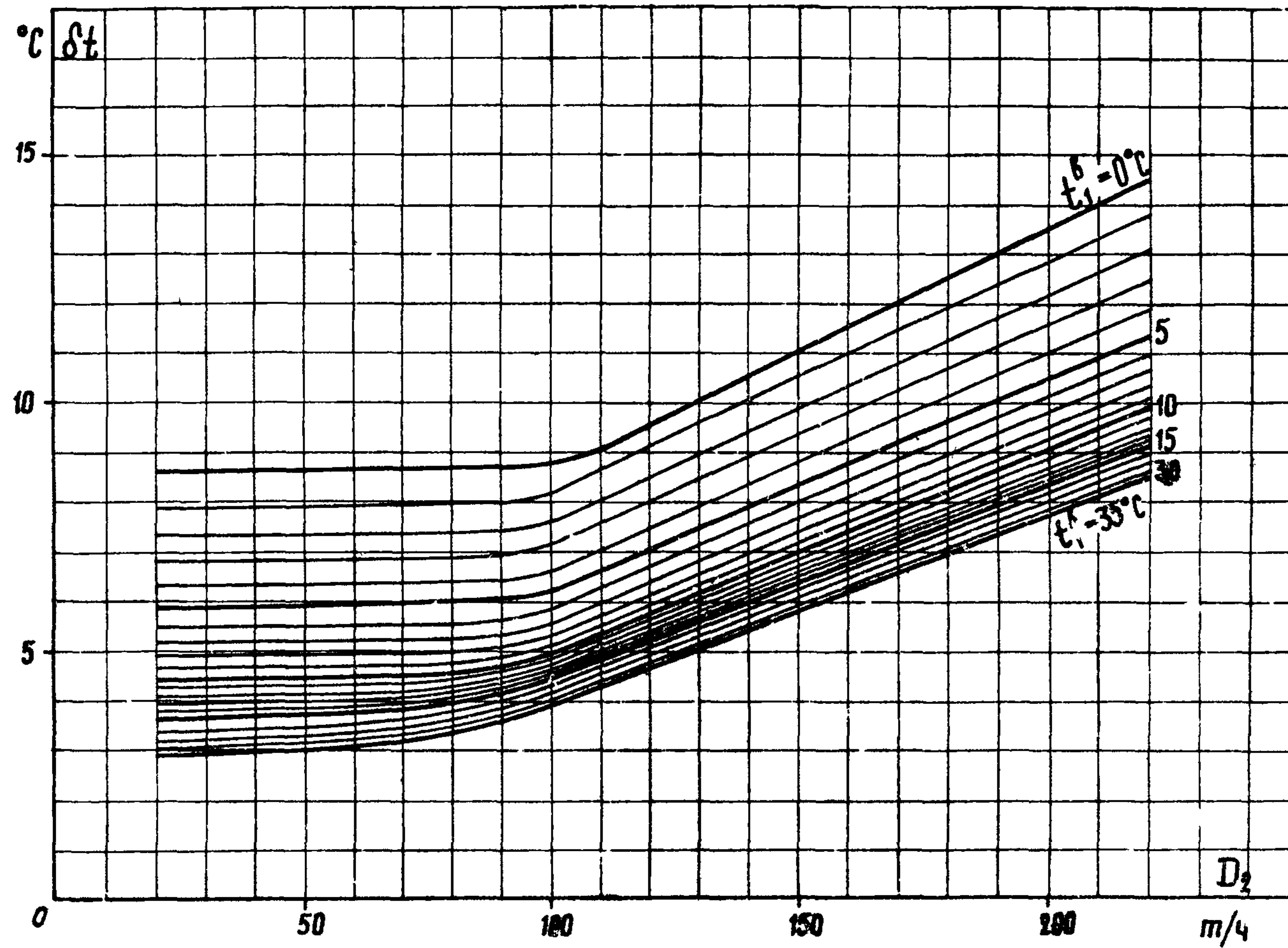
Рис. III-3. Зависимость температурного напора от расхода пара в конденсатор и температуры охлаждающей воды: W = 3500 \text{ м}^3/\text{ч} ; F_{\text{п}} = 3000 \text{ м}^2
