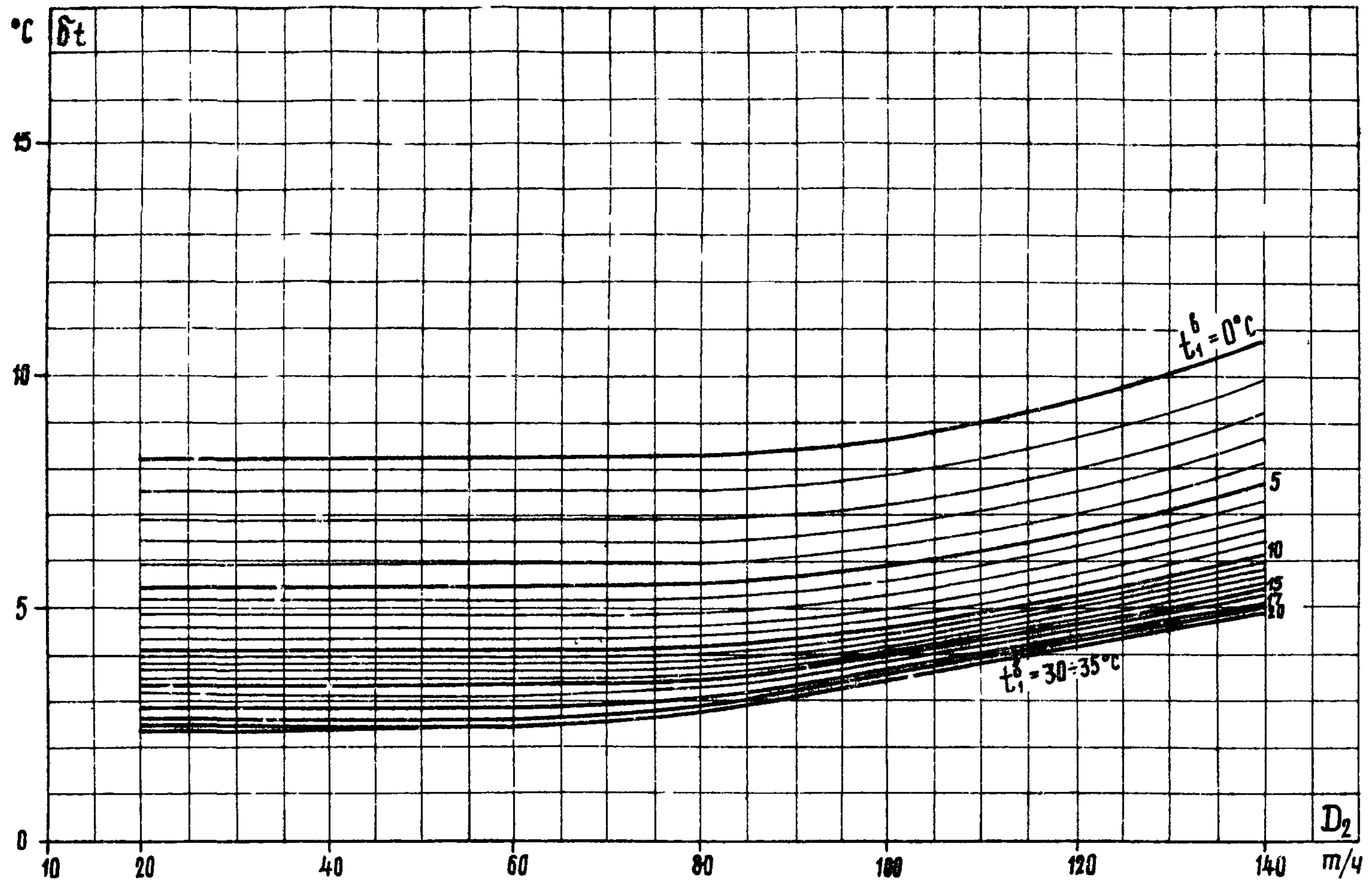
Рис. I-3. Зависимость температурного напора от расхода пара в конденсатор и температуры охлаждающей воды: W = 3500 \text{ м}^3/\text{ч}; F_{\text{п}} = 3000 \text{ м}^2
