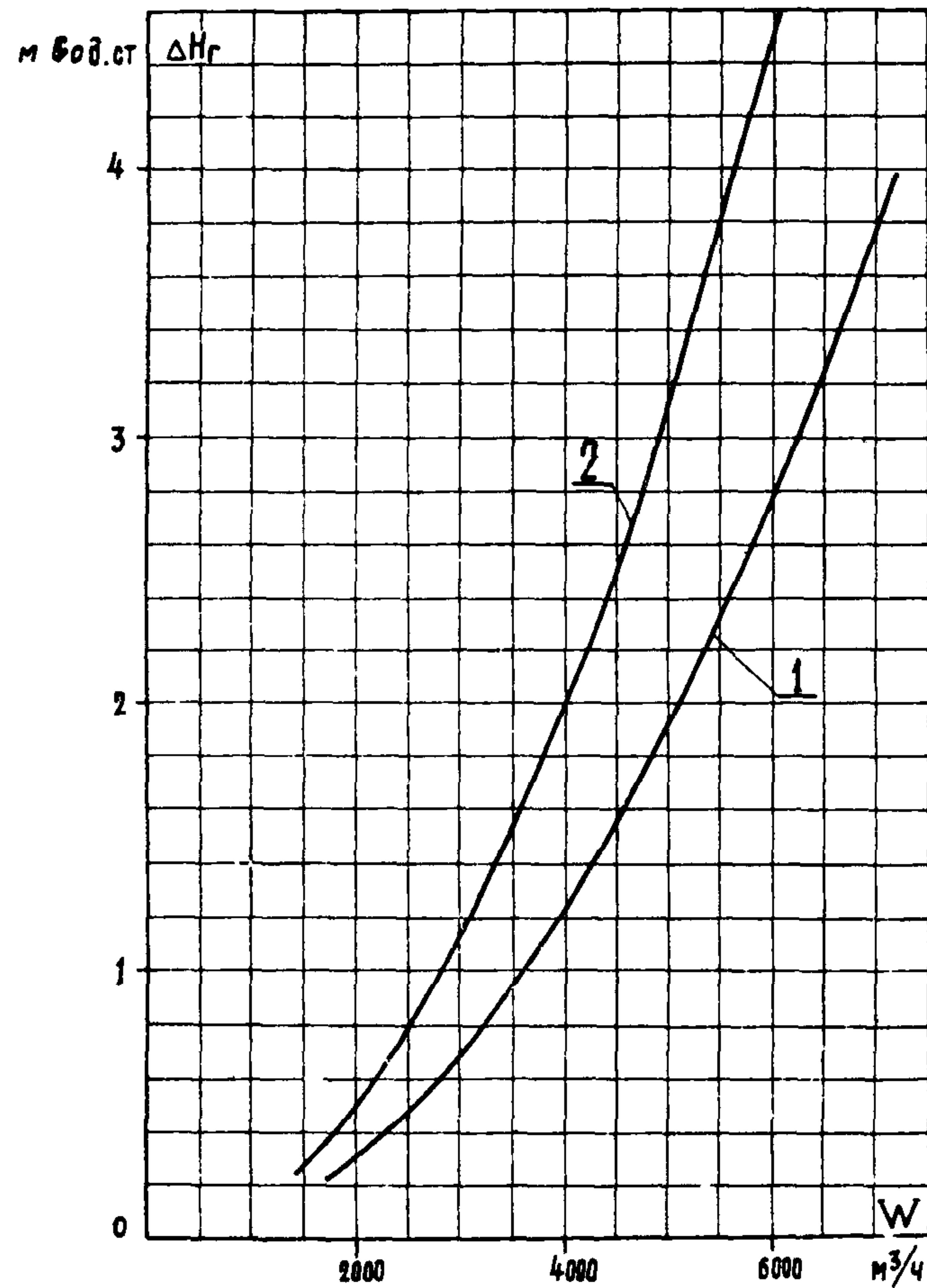
Рис. I-13. Зависимость гидравлического сопротивления от расхода охлаждающей воды в конденсатор: I - полная поверхность конденсатора; 2 - с отключенным встроенным пучком
