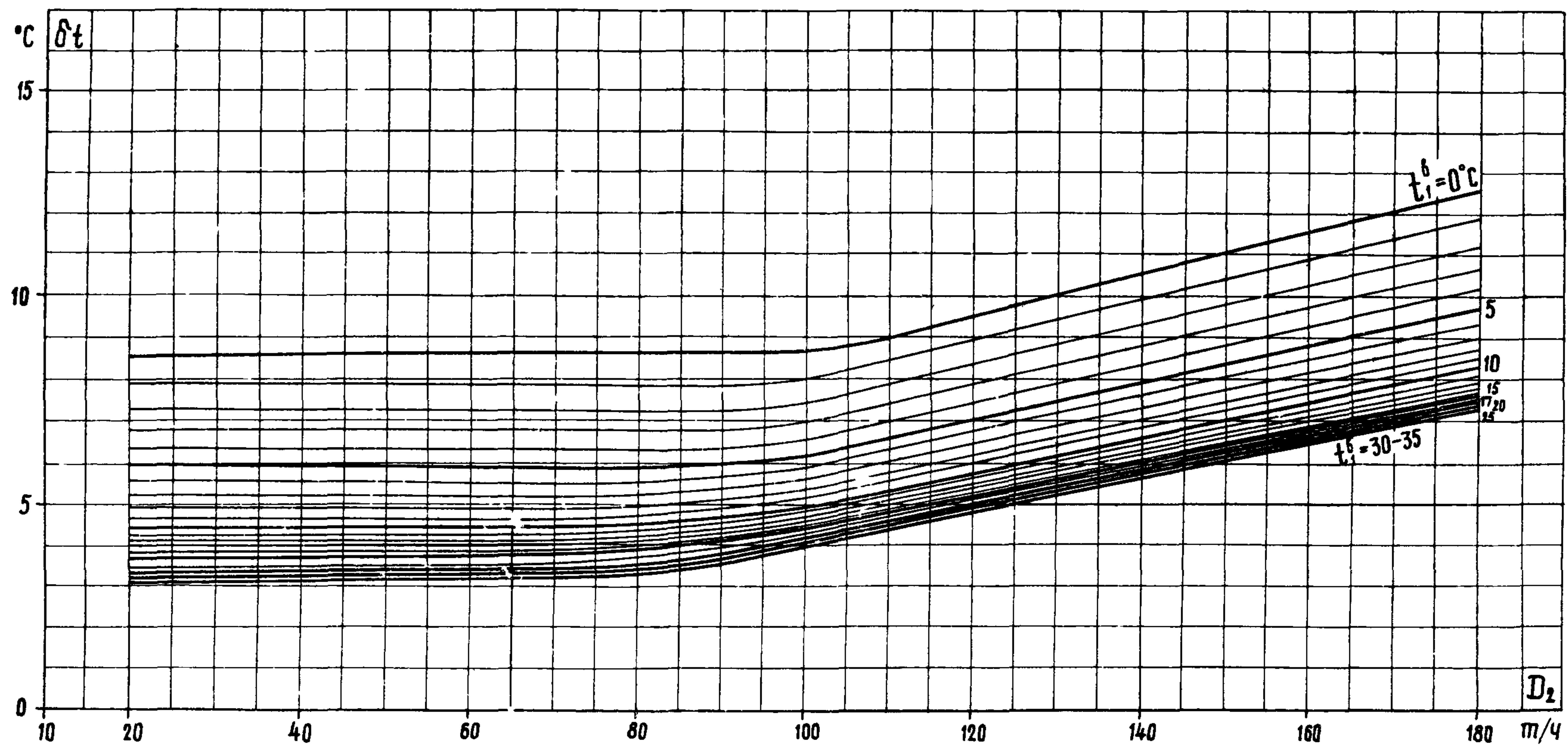
Рис. 1-3. Зависимость температурного напора от расхода пара в конденсатор и температуры охлаждающей воды: W = 3500 \text{ м}^3/\text{ч}
