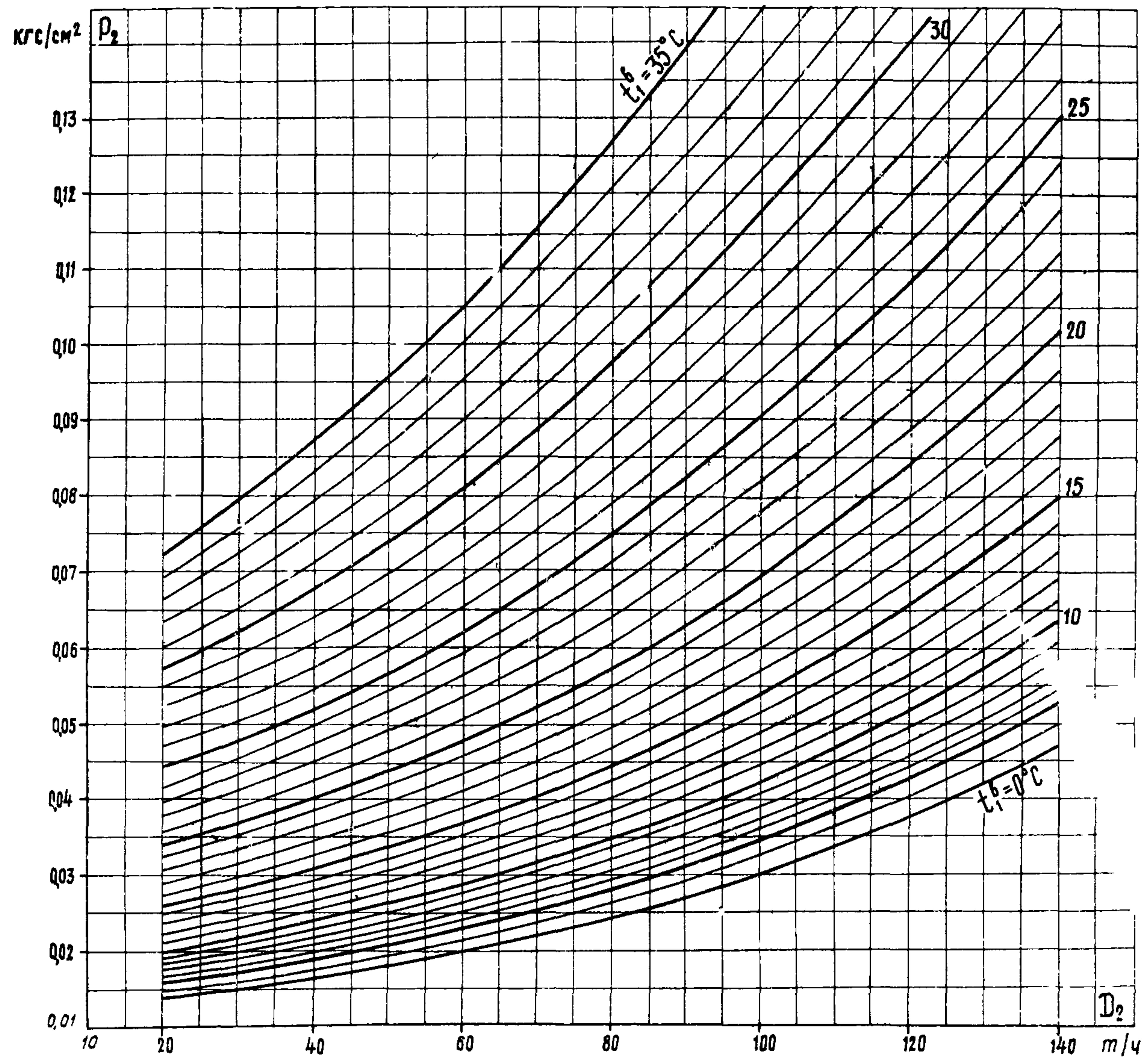
Рис. I-6. Зависимость абсолютного давления от расхода пара в конденсатор и температуры охлаждающей воды: W = 3500 \text{ м}^3/\text{ч} ; F_n = 3000 \text{ м}^2
