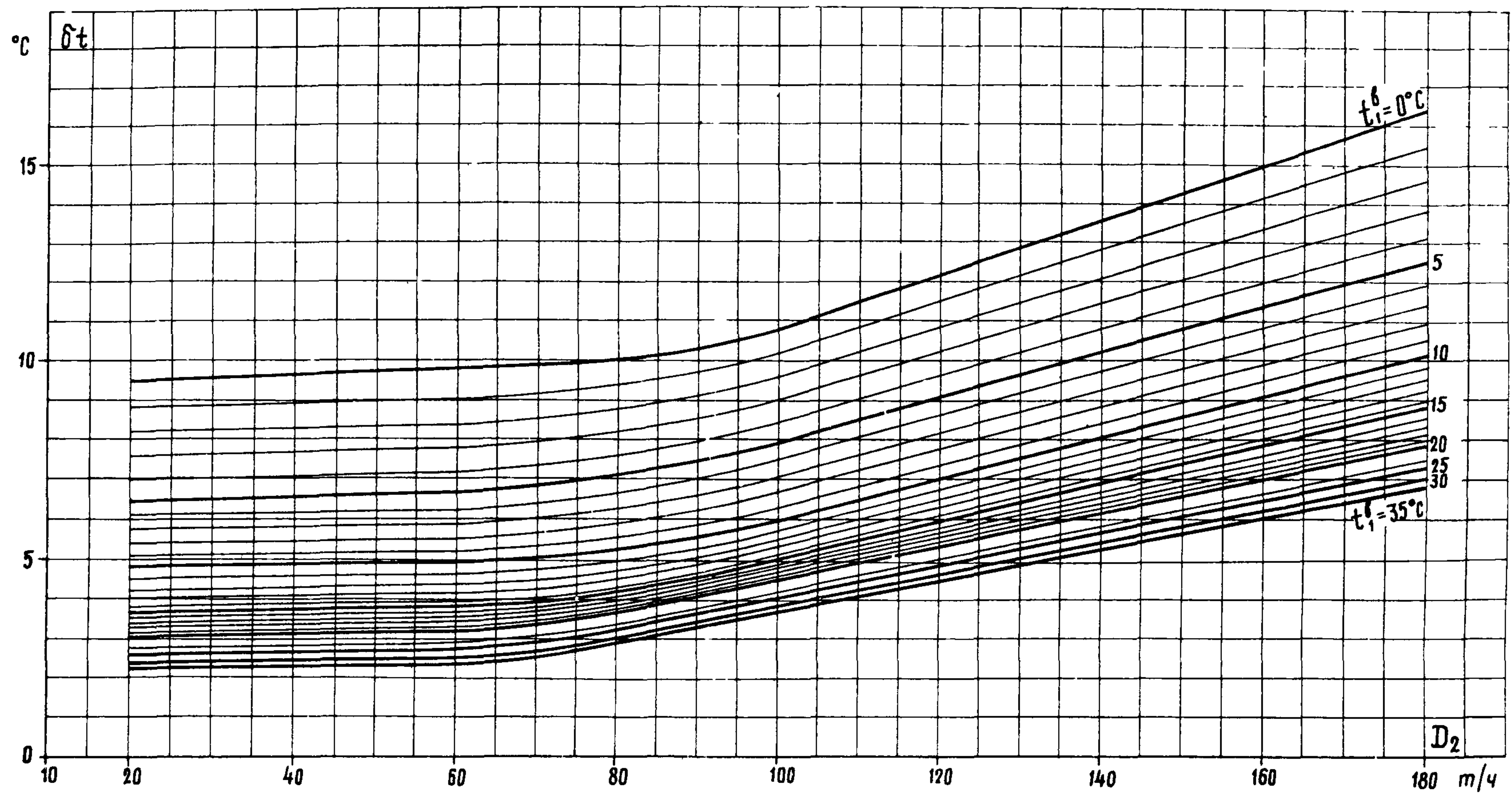
Рис. II-1. Зависимость температурного напора от расхода пара в конденсатор и температуры охлаждающей воды: W^H = 8000 \text{ м}^3/\text{ч}
