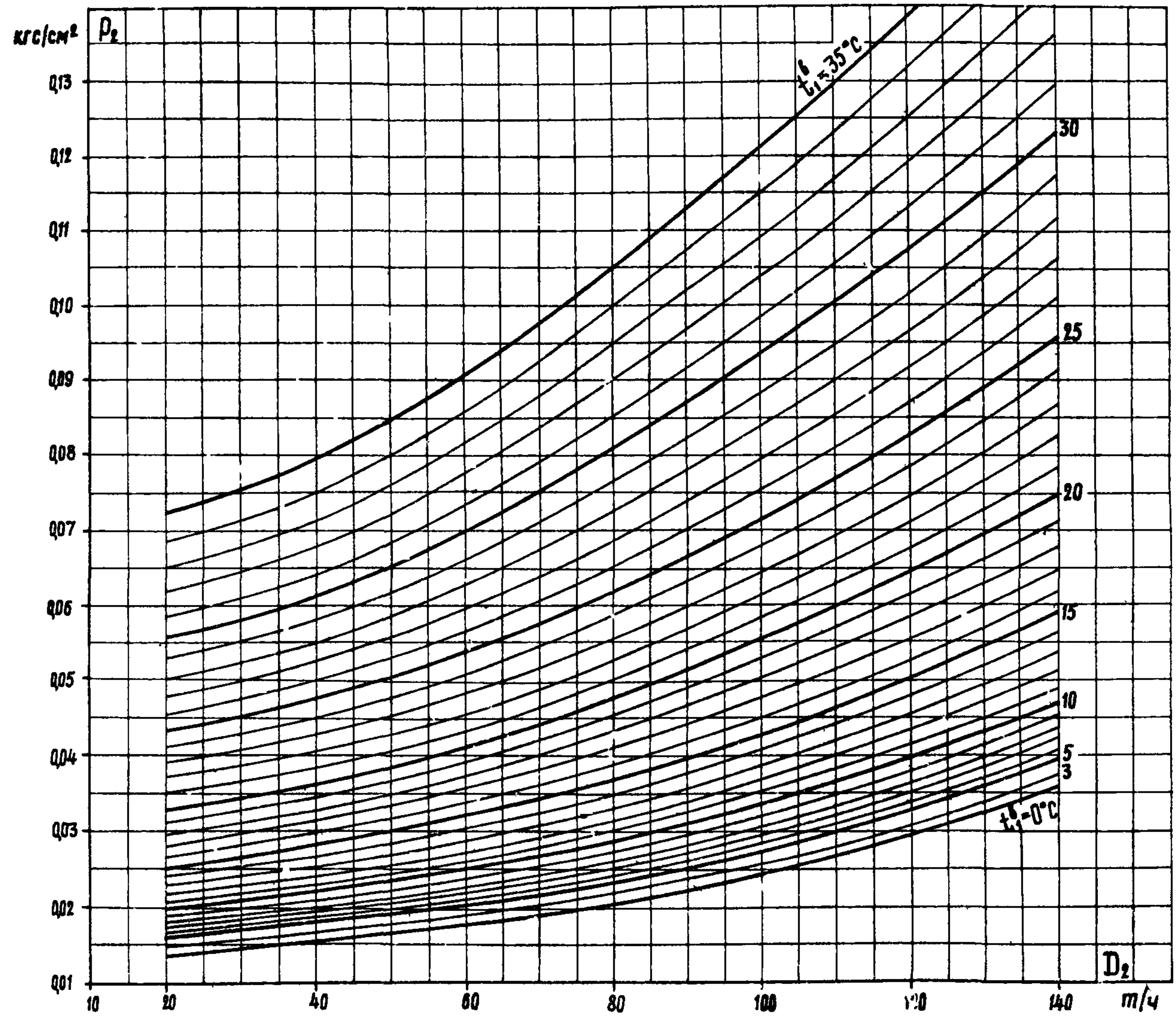
Рис. I-5. Зависимость абсолютного давления от расхода пара в конденсатор и температуры охлаждающей воды: W = 5000 \text{ м}^3/\text{ч}; F_{\text{п}} = 3000 \text{ м}^2
