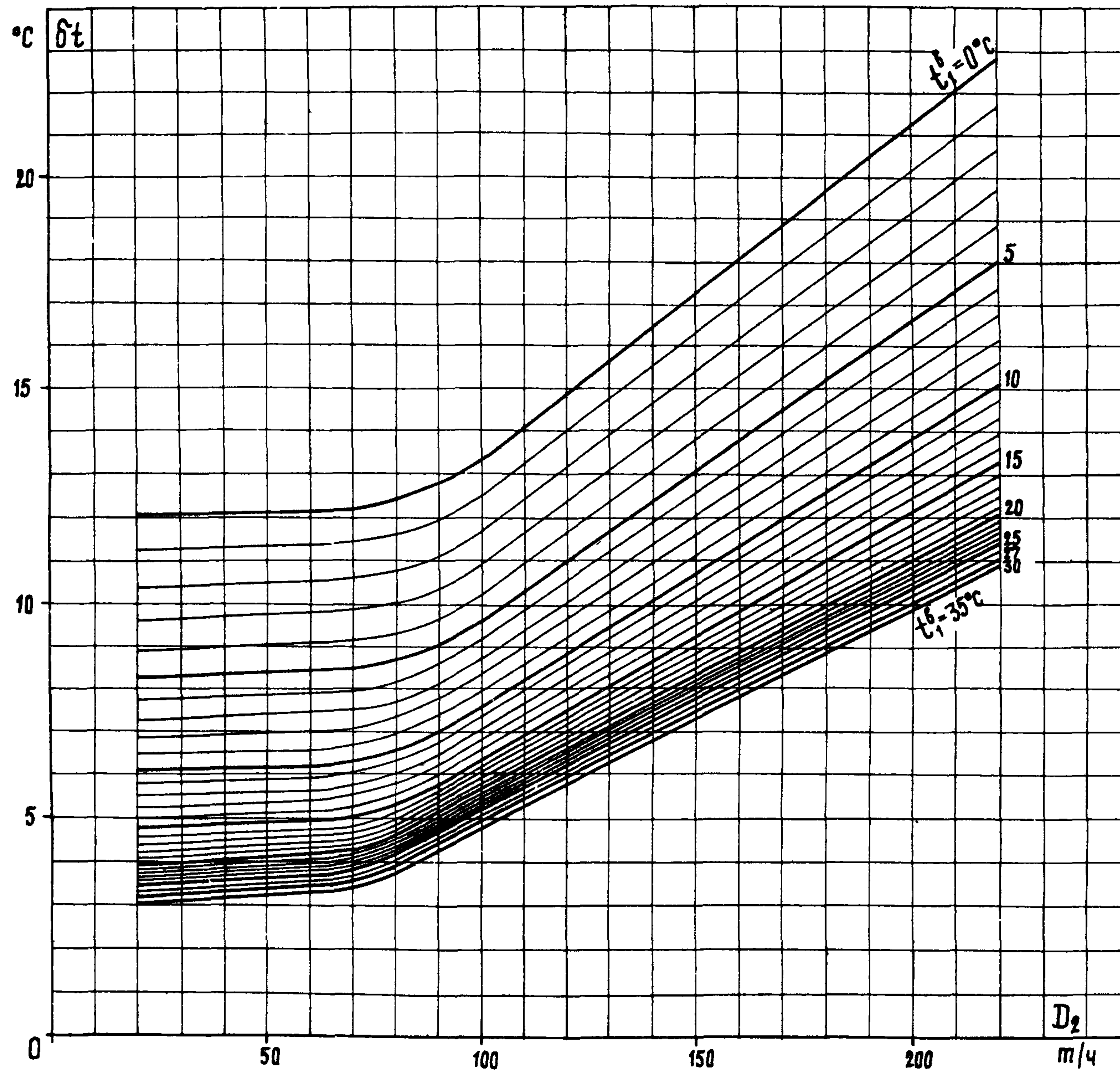
Рис. 11-8. Зависимость темпе- ратурного напора от расхода пара в конденсатор и темпе- ратуры охлаждающей воды: W = 6250 \text{ м}^3/\text{ч}; F = 2345 \text{ м}^2
