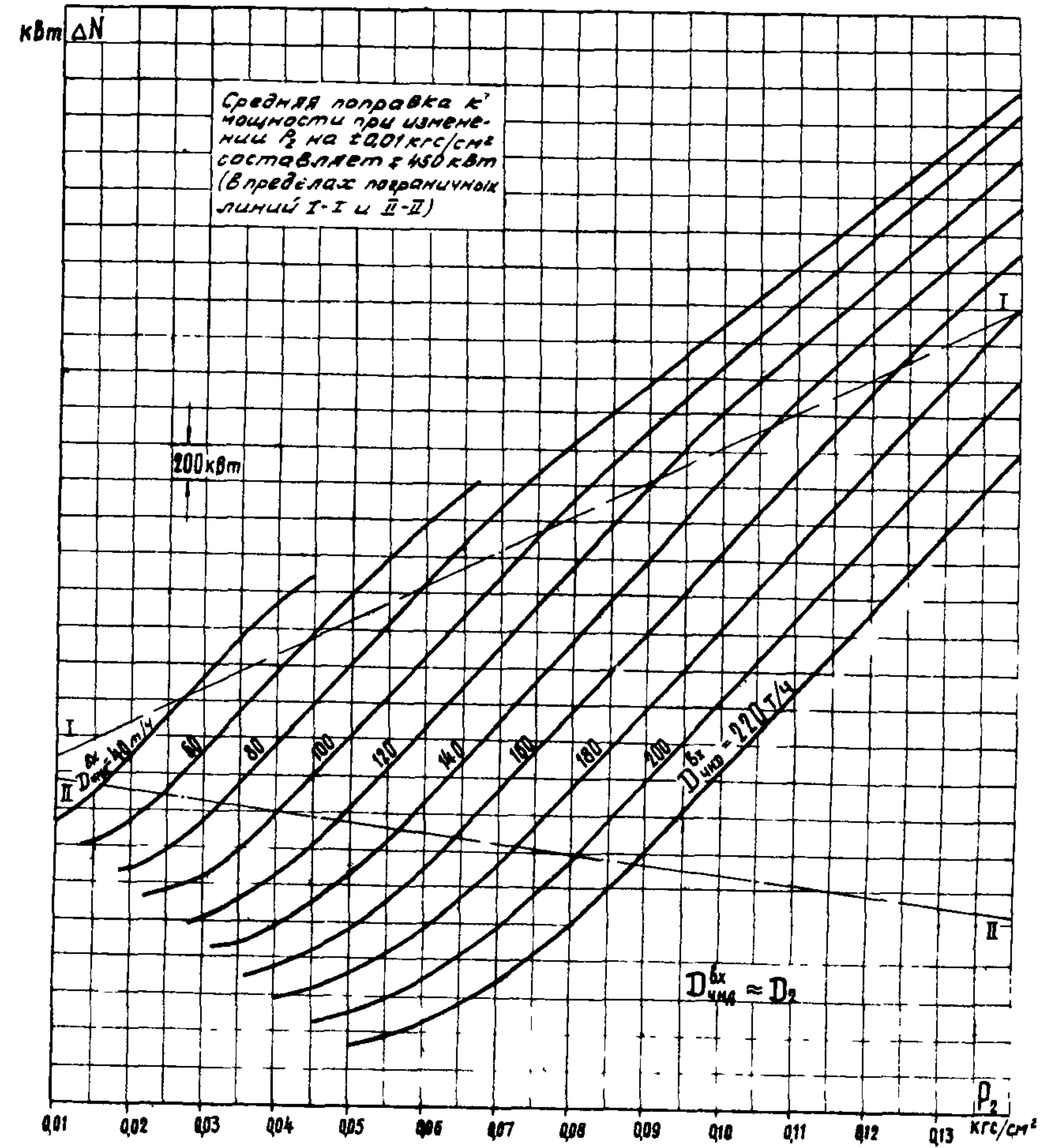
Рис. III-16. Поправка к мощности турбины ПТ-80/100-130/13 ЛМЗ на отклонение давления пара в конденсаторе (по данным испытания донтехэнерго) турбины ПТ-80/100-130/13 ЛМЗ
