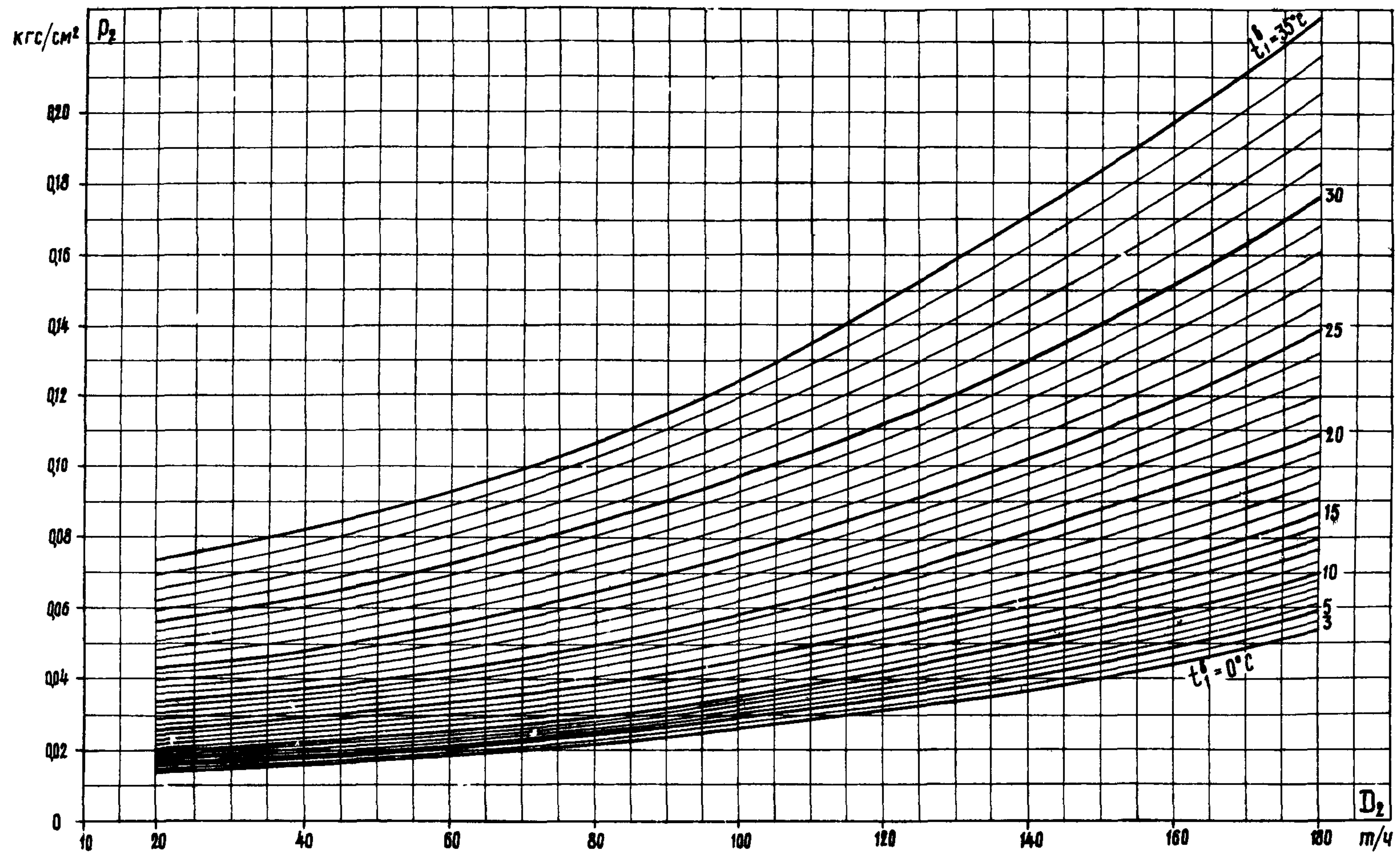
Рис.П-5. Зависимость абсолютного давления от расхода пара в конденсатор и температуры охлаждающей воды: W = 5000 \text{ м}^3/\text{ч}
