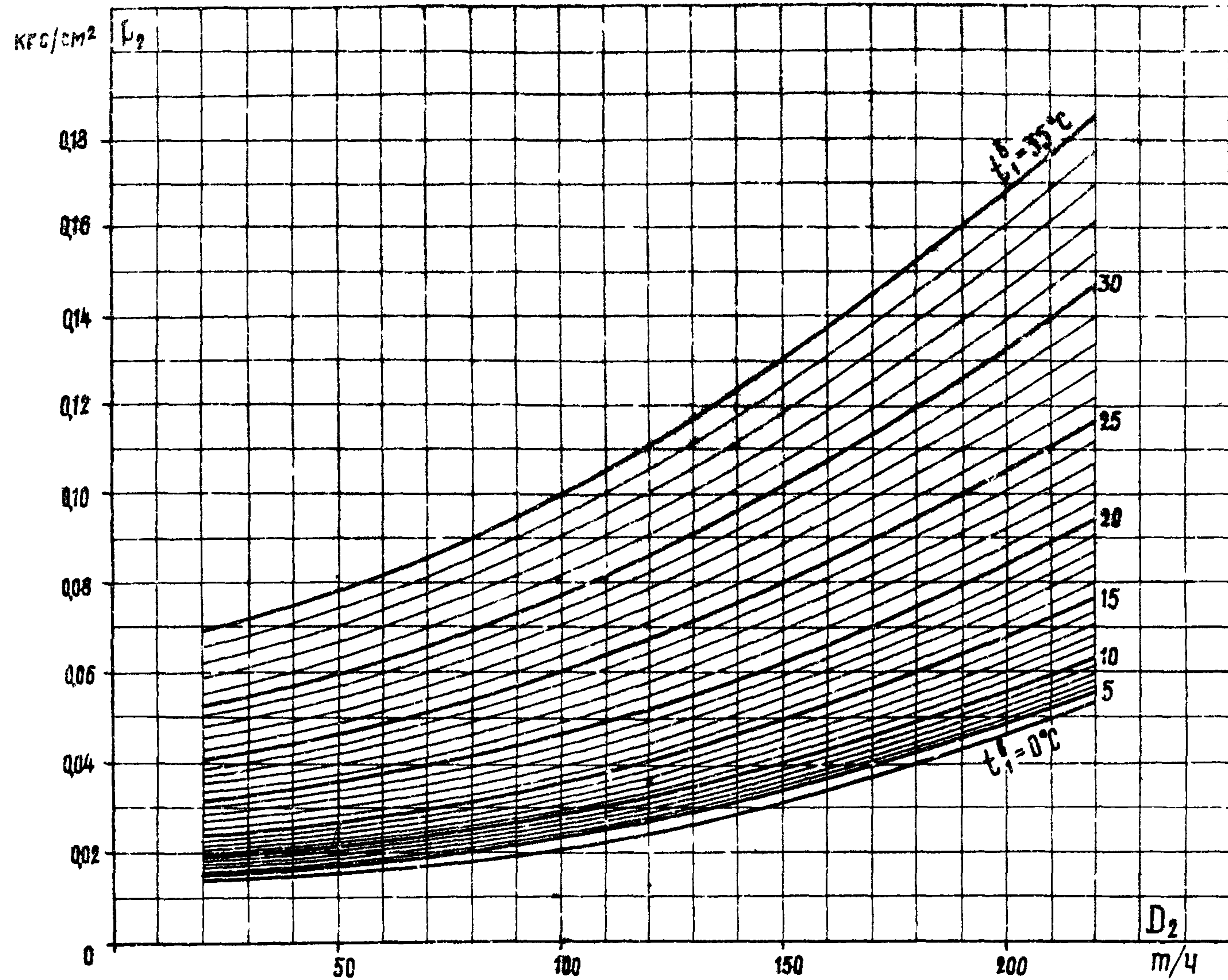
Рис. 11-4. Зависимость абсолютного давления от расхода пара в конденсатор и температуры охлаждающей воды: W^H = 8000 \text{ м}^3/\text{ч} ; F_n = 3000 \text{ м}^2
