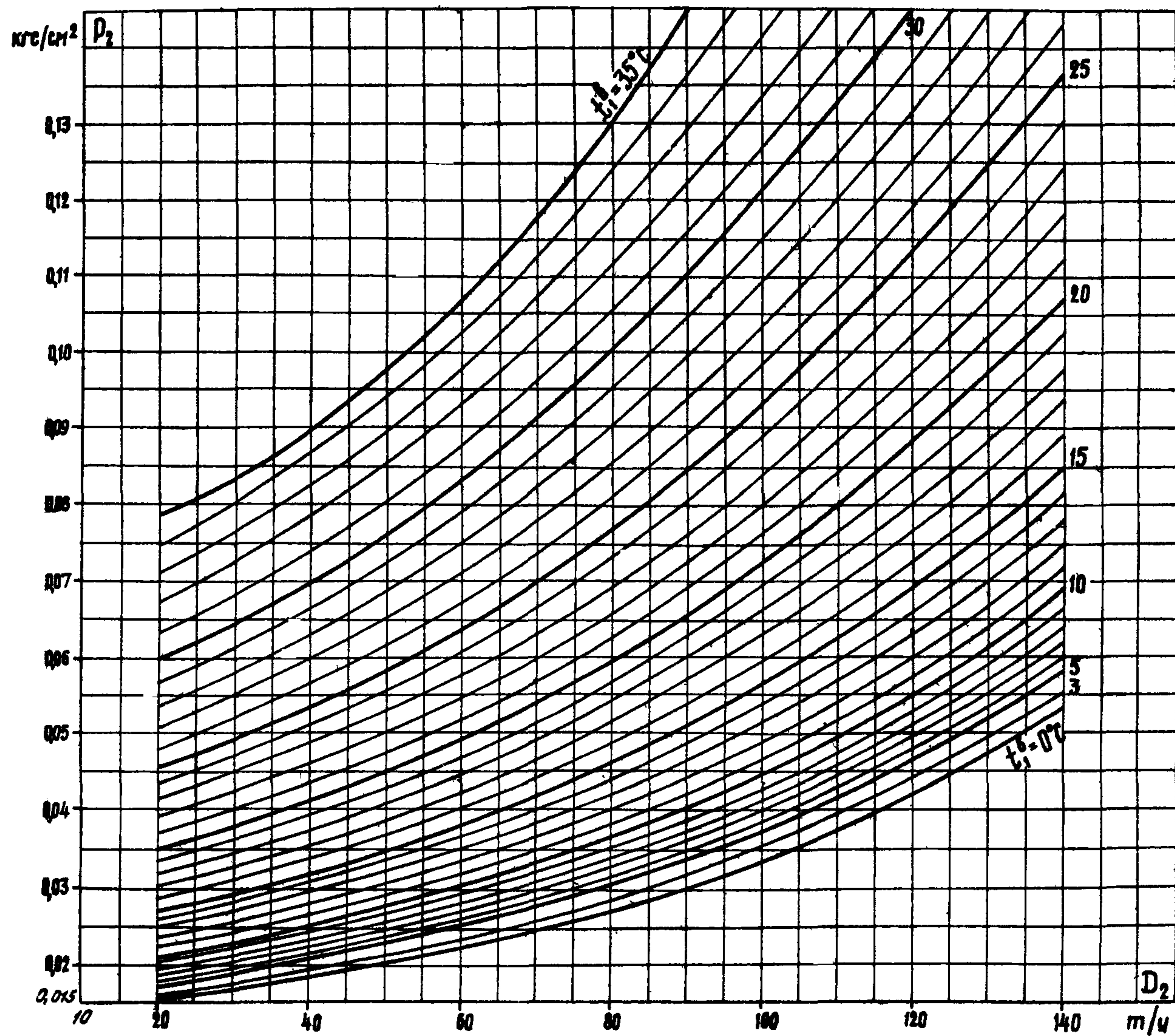
Рис. I-12. Зависимость абсолютного давления от расхода пара в конденсатор и температуры охлаждающей воды:
