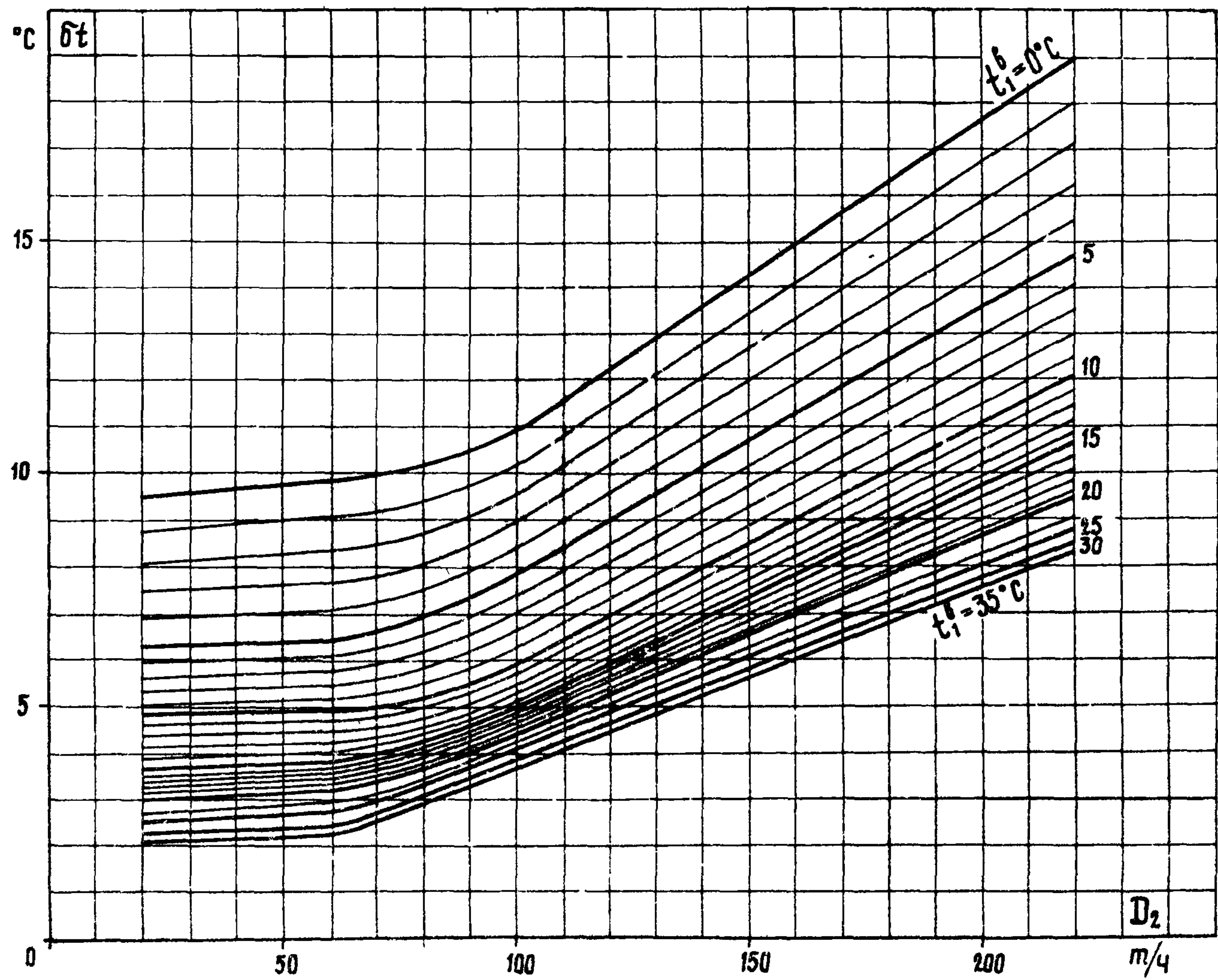
Рис. II-1. Зависимость температурного напора от расхода пара в конденсатор и температуры охлаждающей воды. W'' = 8000 \text{ м}^3/\text{ч} ; F_n = 3000 \text{ м}^2
