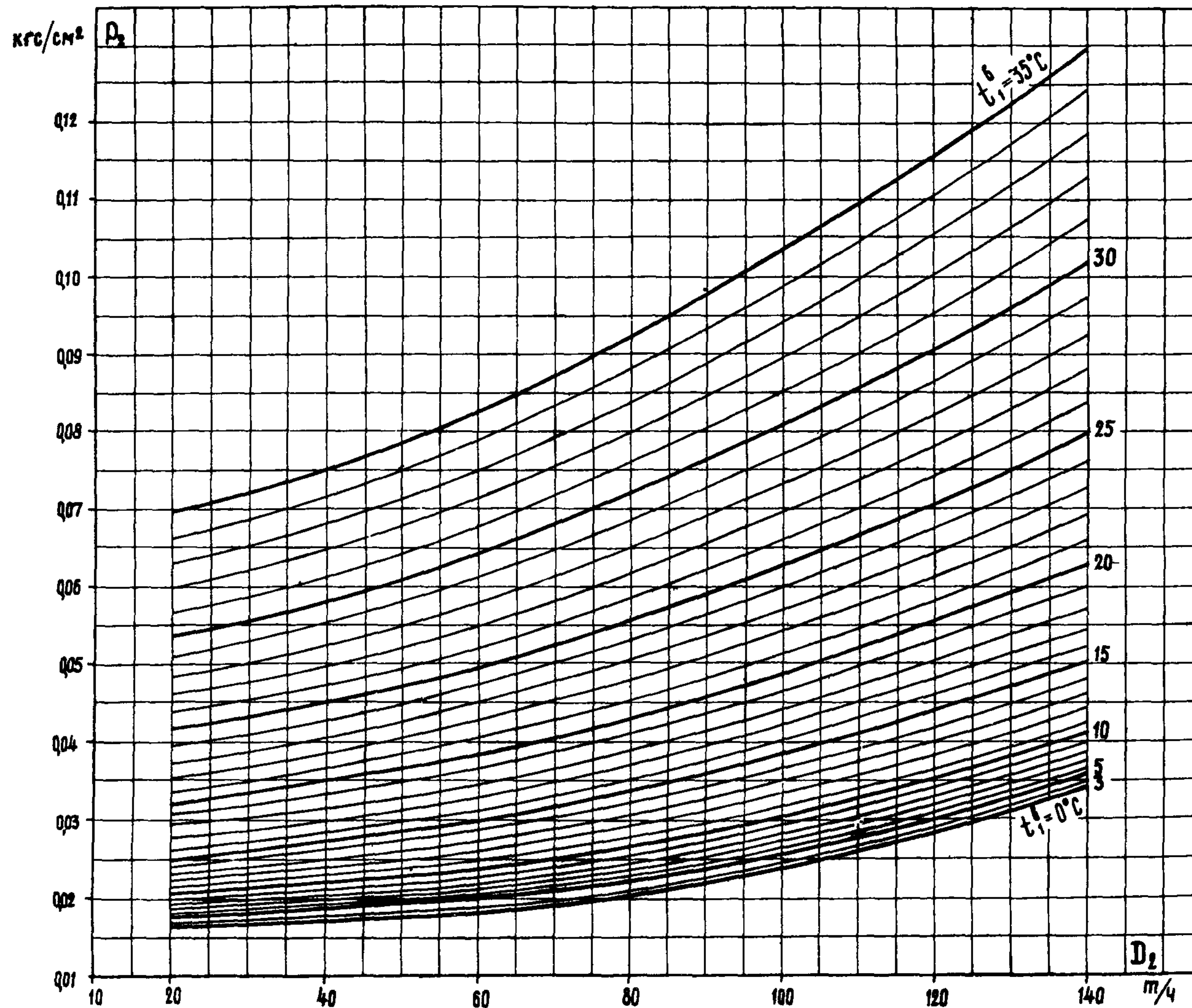
Рис. I-10. Зависимость абсолютного давления от расхода пара в конденсатор и температуры охлаждающей воды: W^H = 7000 \text{ м}^3/\text{ч}; \quad F = 2555 \text{ м}^2
