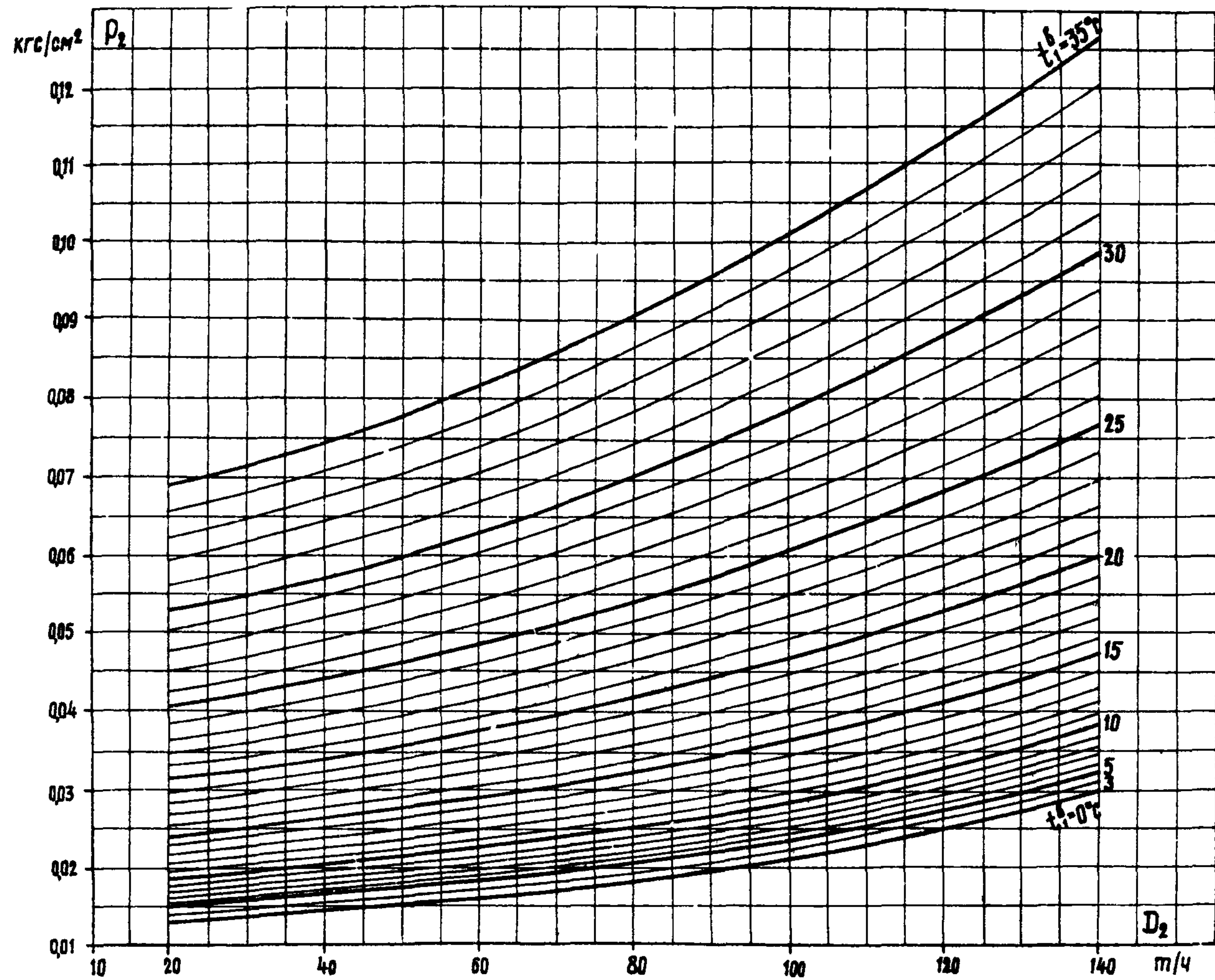
Рис. I-4. Зависимость абсолютного давления от расхода пара в конденсатор и температуры охлаждающей воды: W^H = 7000 \text{ м}^3/\text{ч}; F_{\Pi} = 3000 \text{ м}^2
