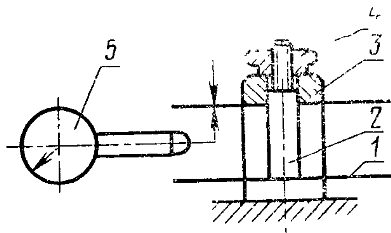
1—испытуемая бобина, 2—сердечник, 3—шайба, 4—гайка, 5—индикатор
