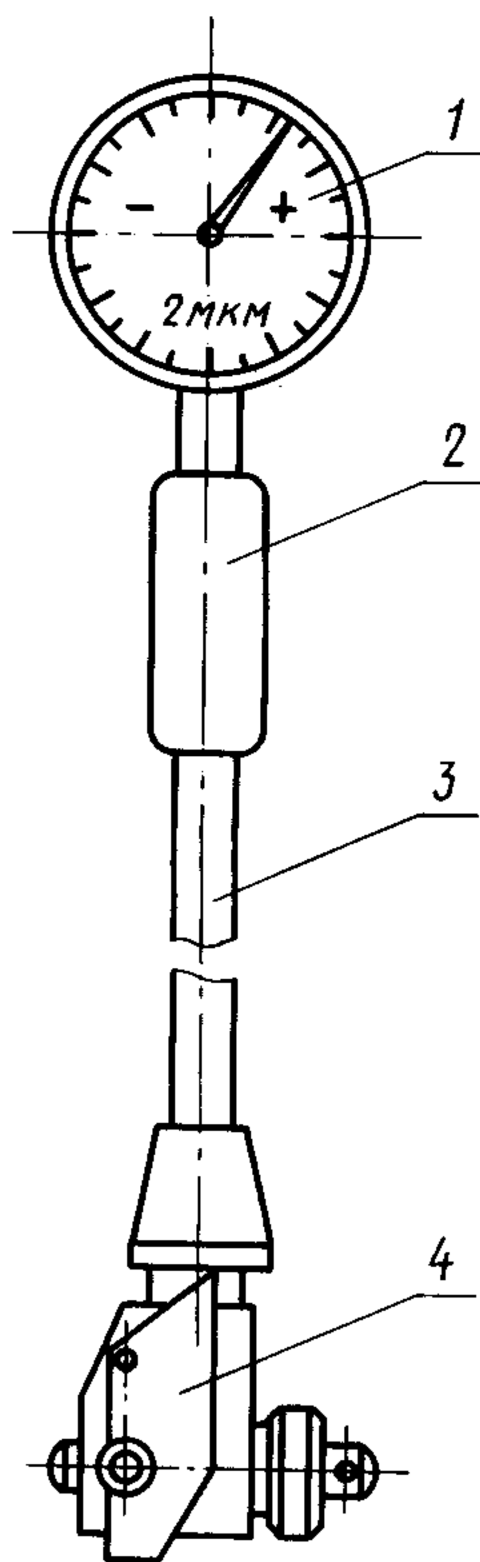
1 — отсчетное устройство; 2 — ручка; 3 — корпус; 4 — мостик
