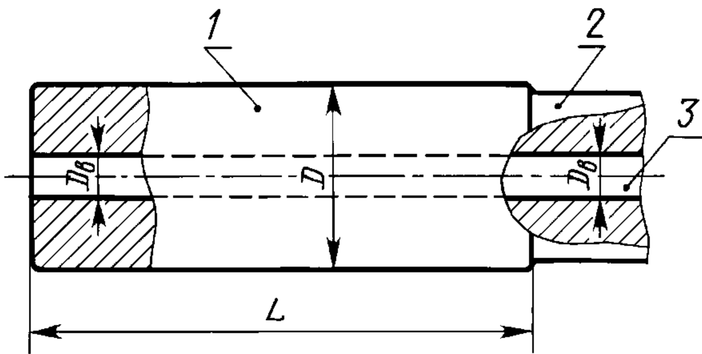
Исполнение 3 (для соединения типа IV)
