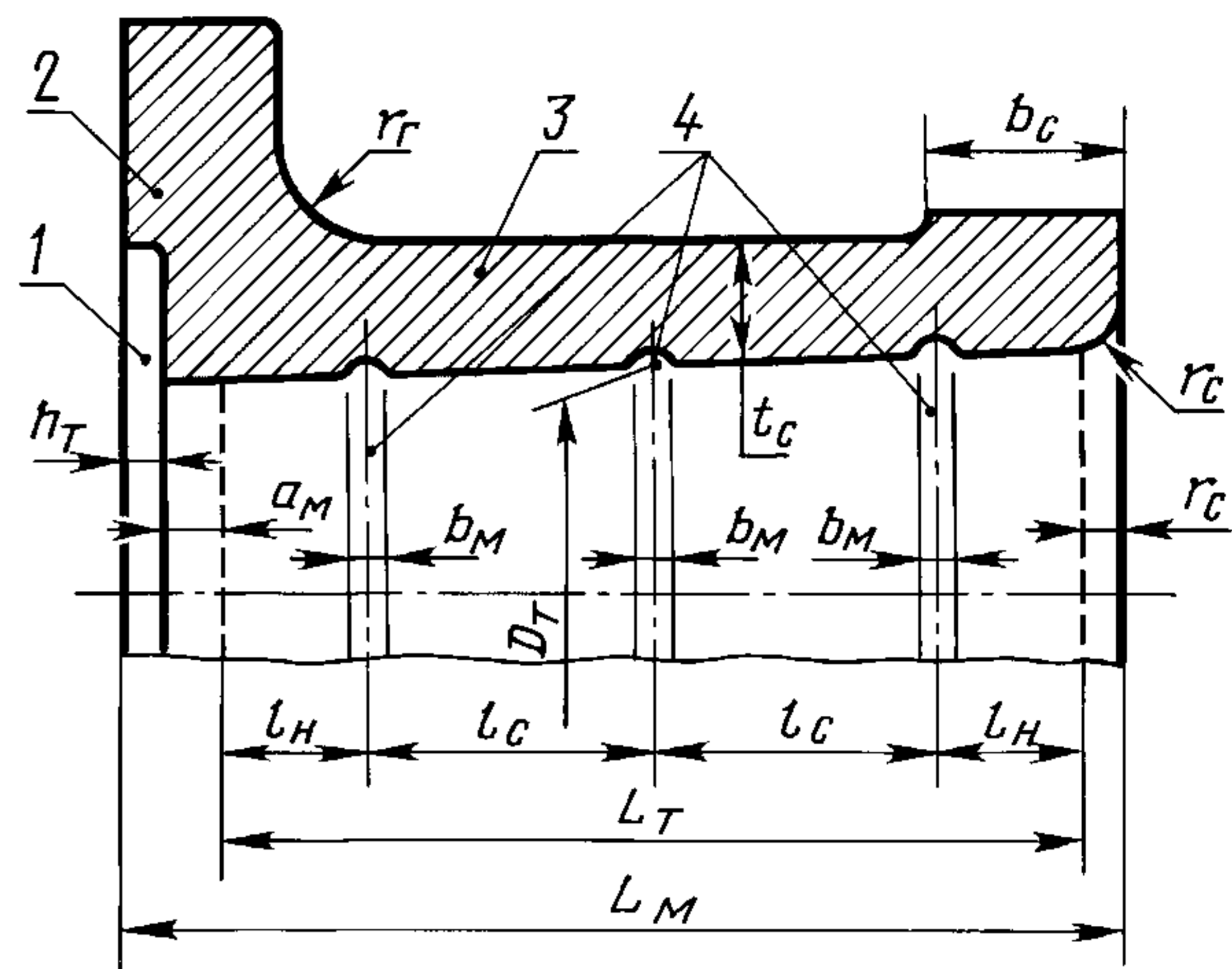
Полумуфта соединения типа III
