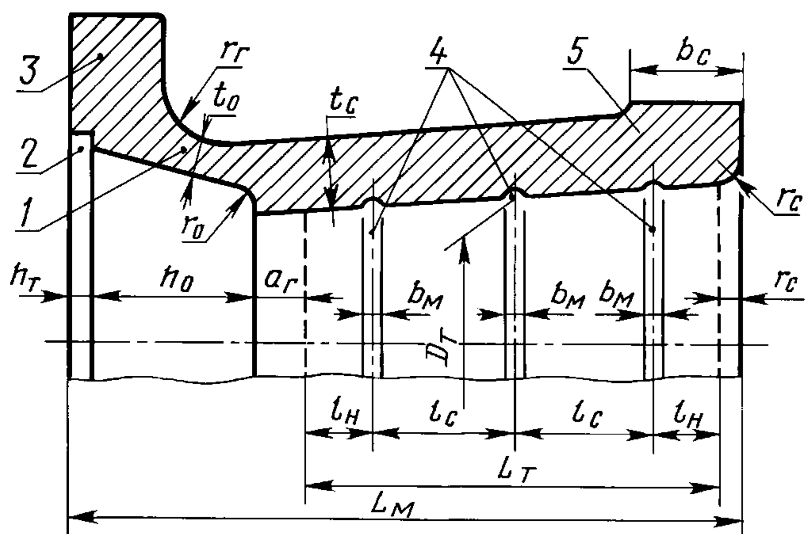
Полумуфта соединения типа II
