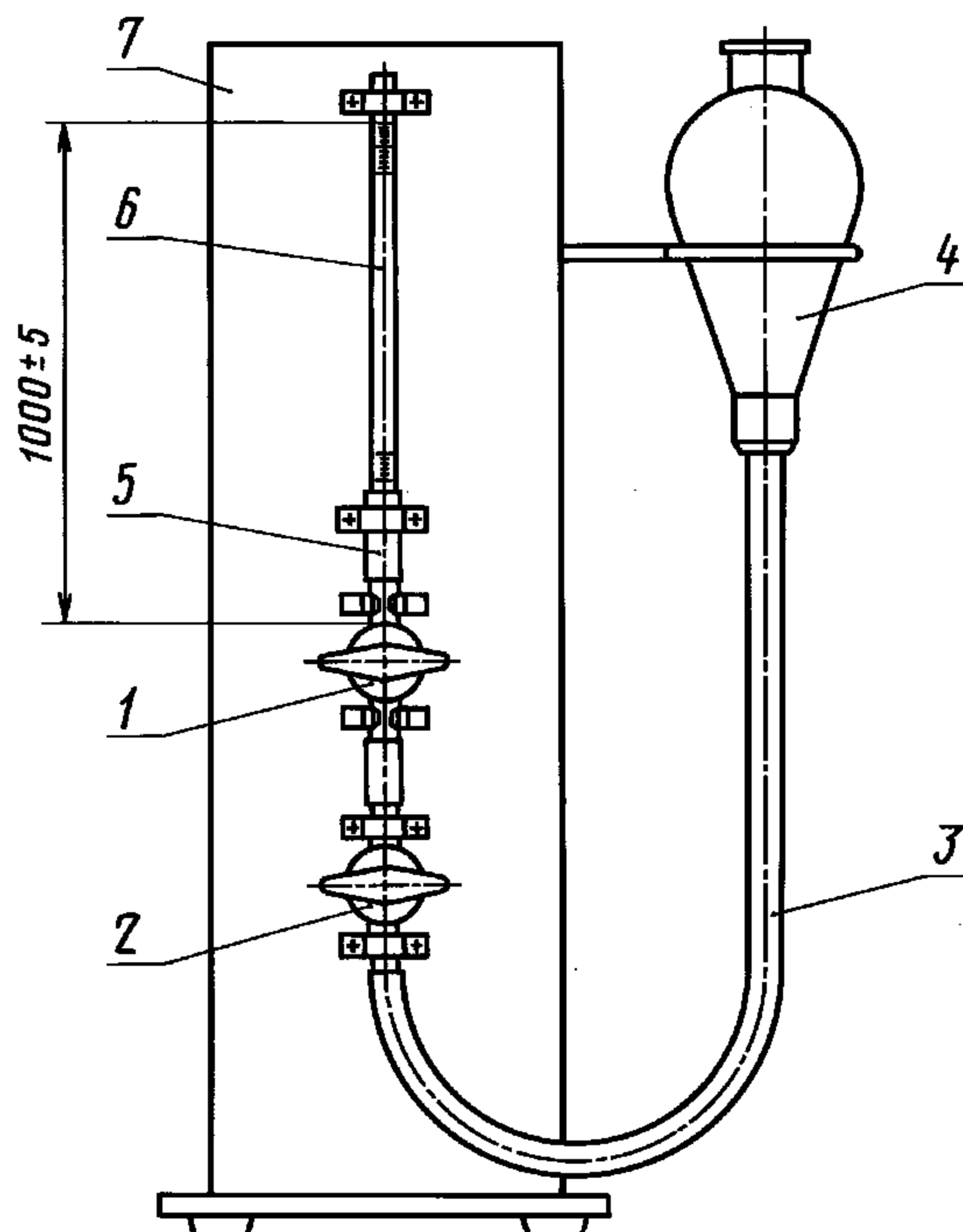
Схема проверки кранов на герметичность
