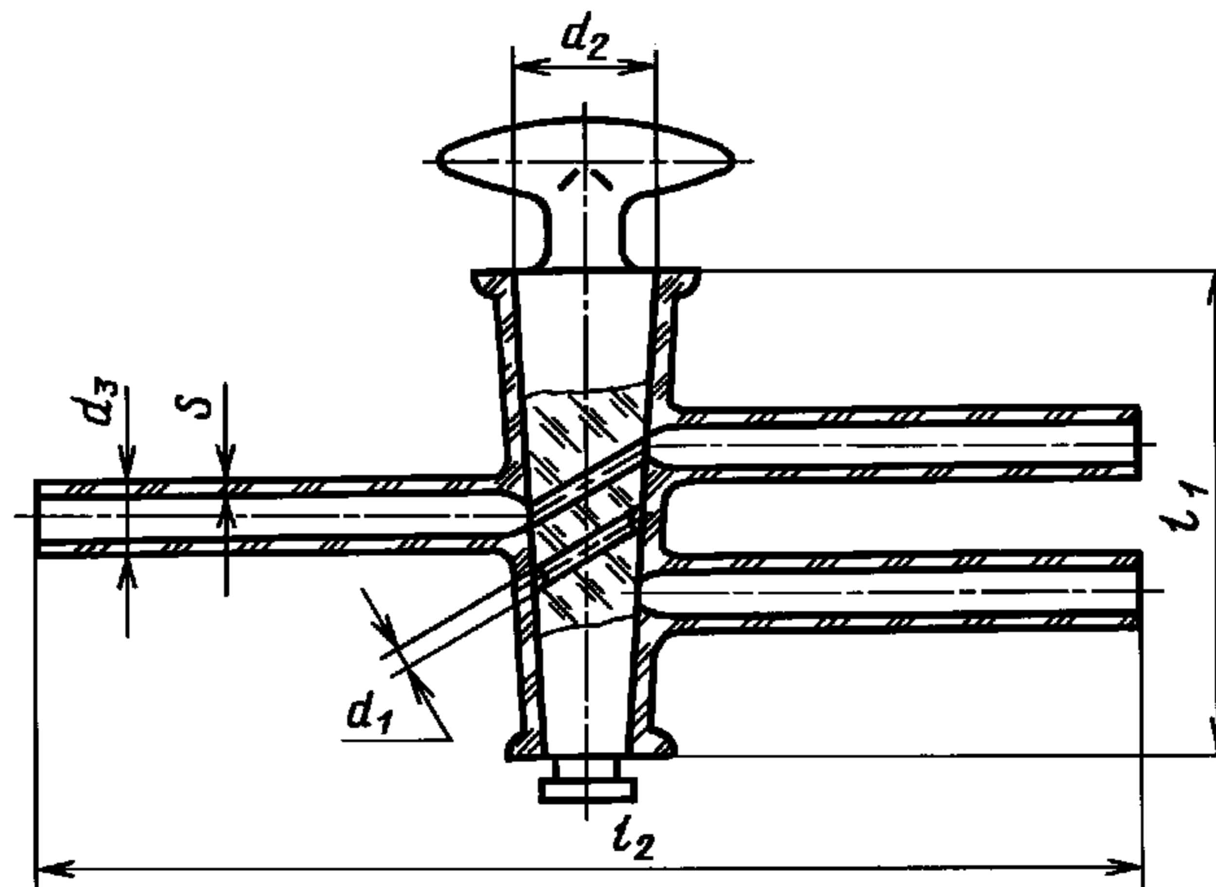
Кран типа К2Х
