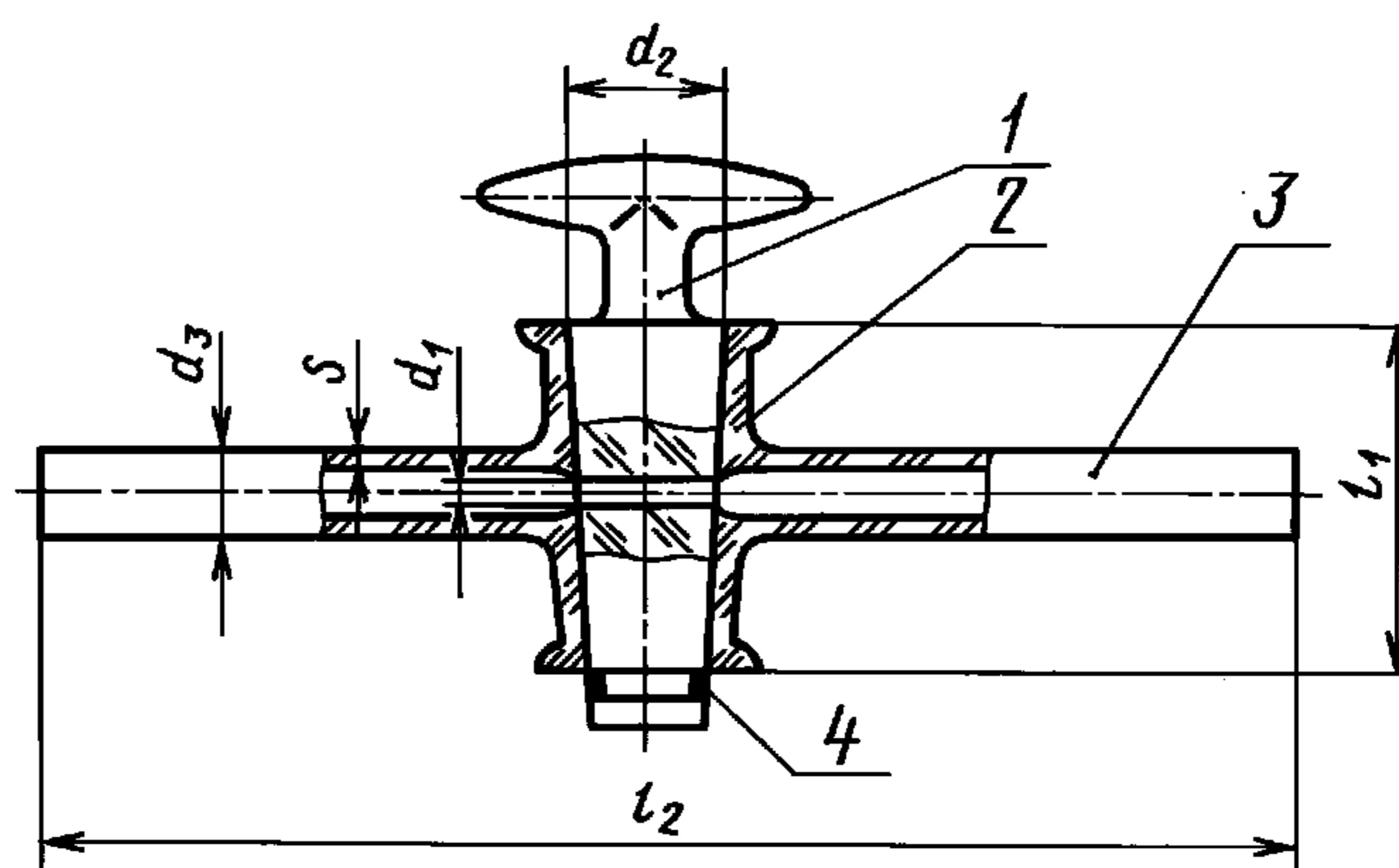
Краны типов К1Х и К1Х КШ
