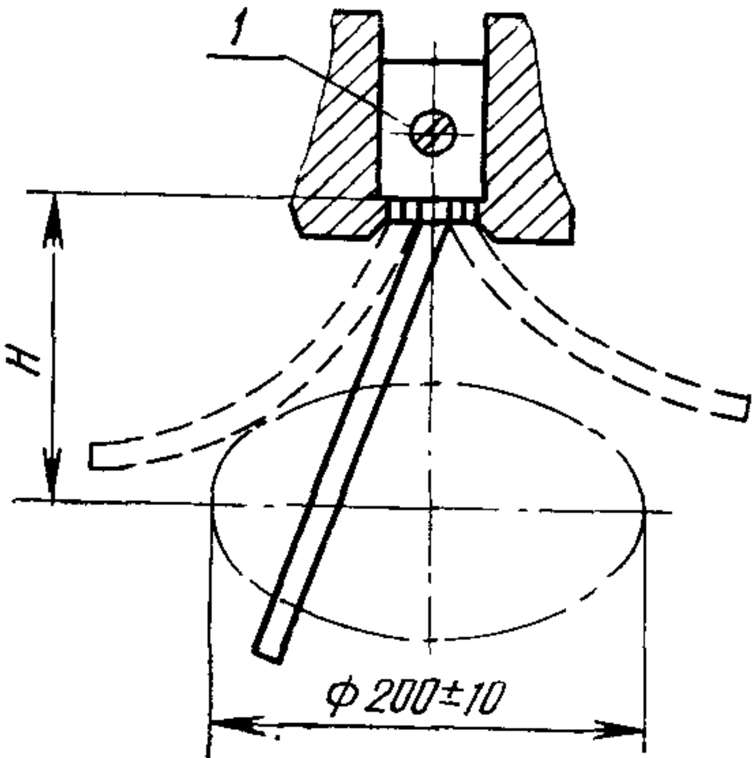
1 — зажим
