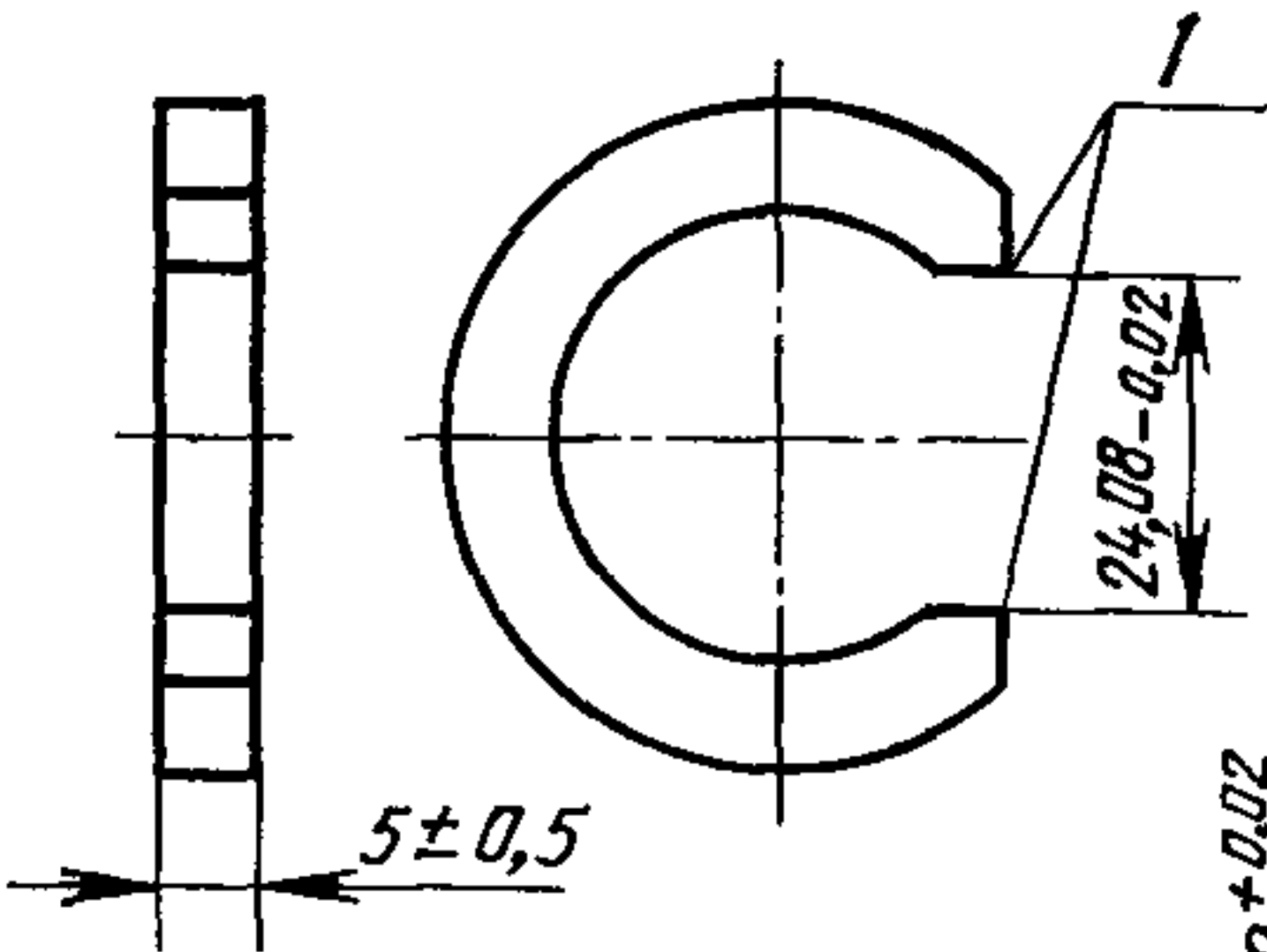
Калибр В
