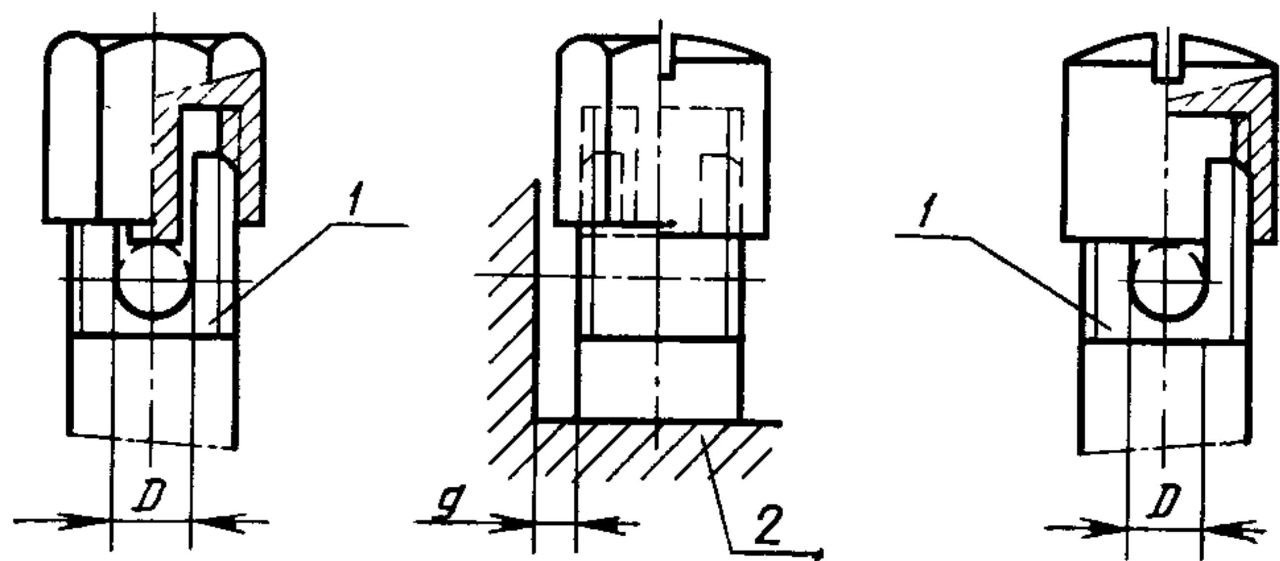
Колпачковый зажим
