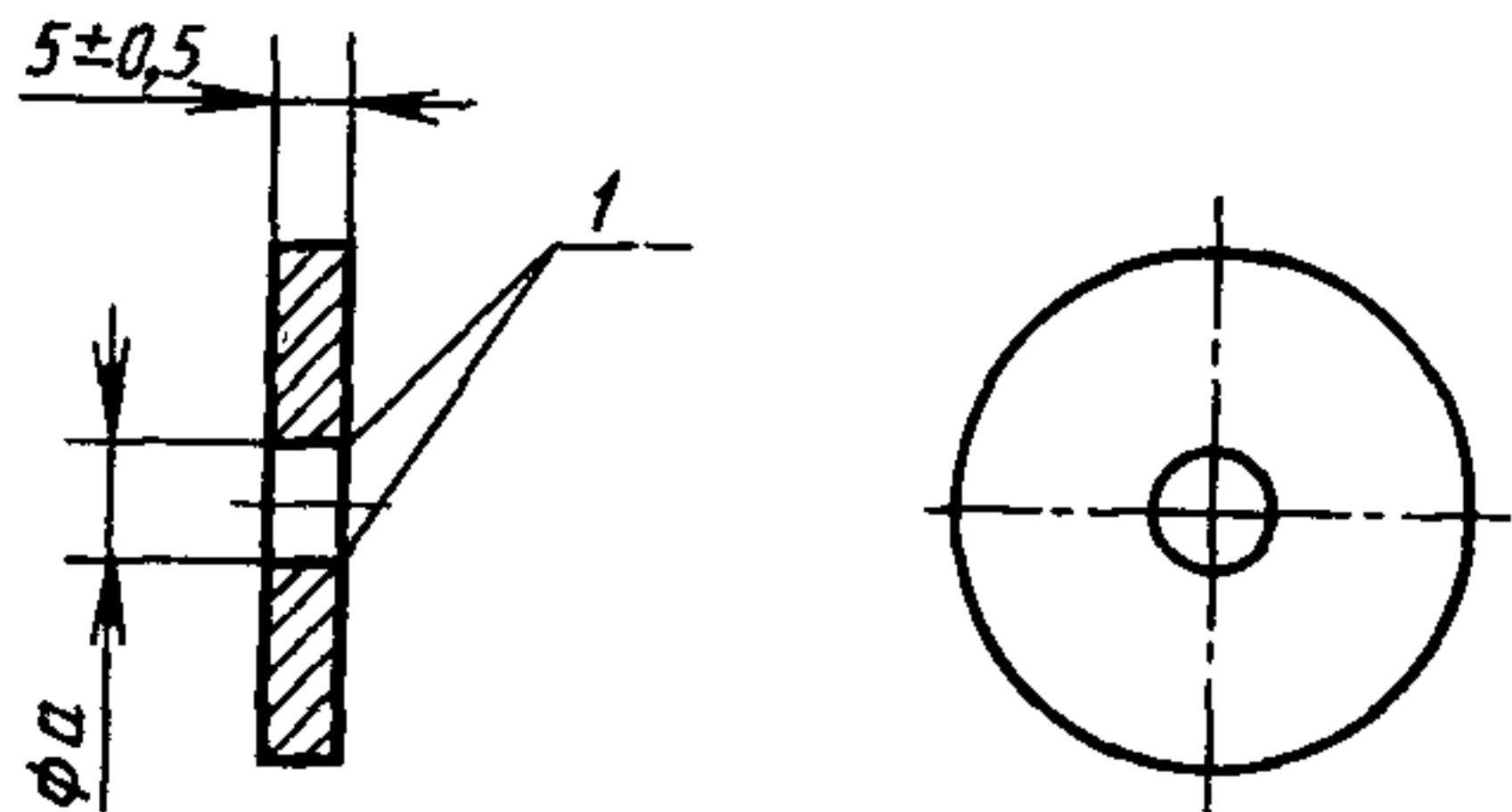
Непроходной калибр
