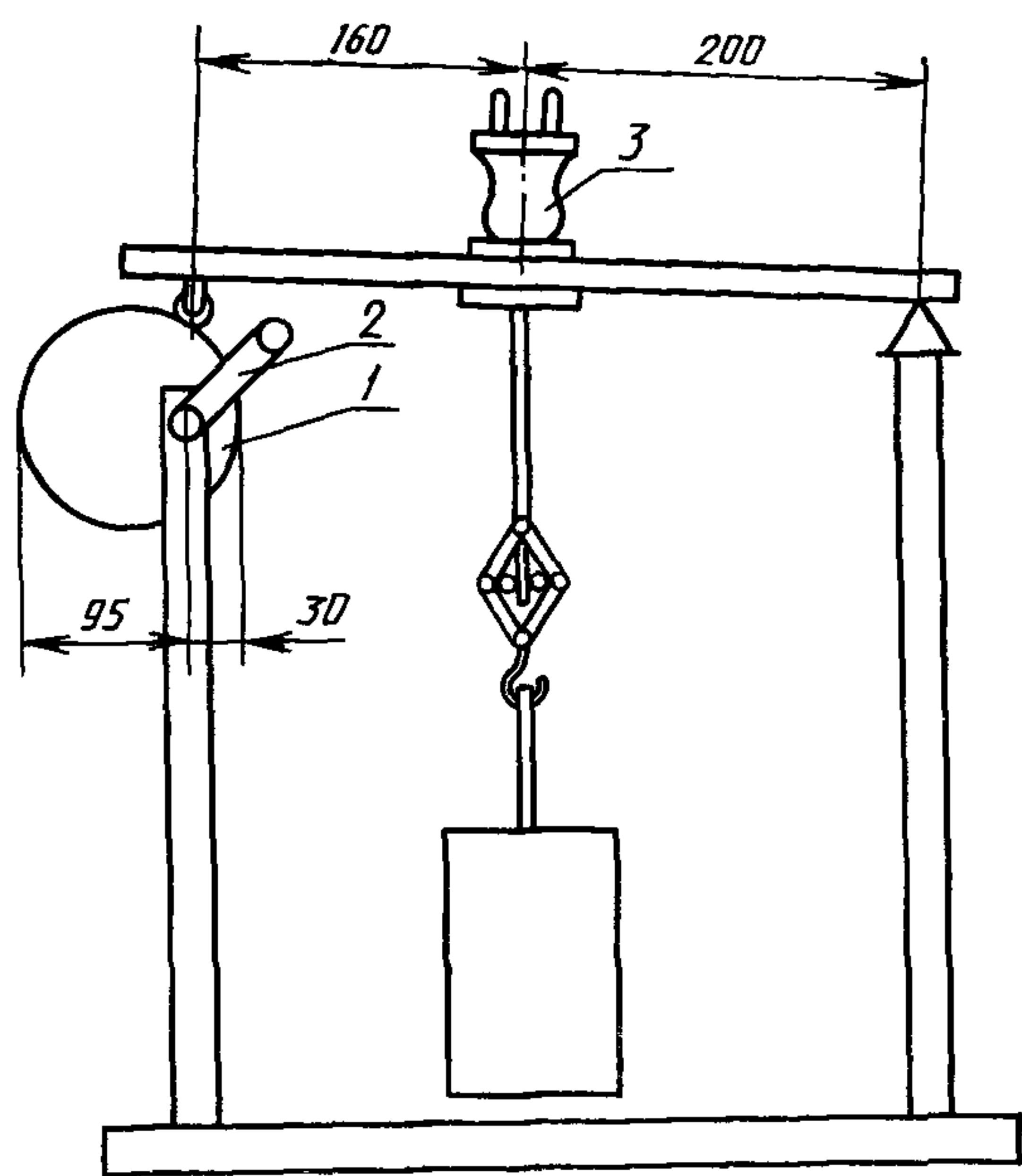
1 — эксцентрик; 2 — ручка; 3 — образец
