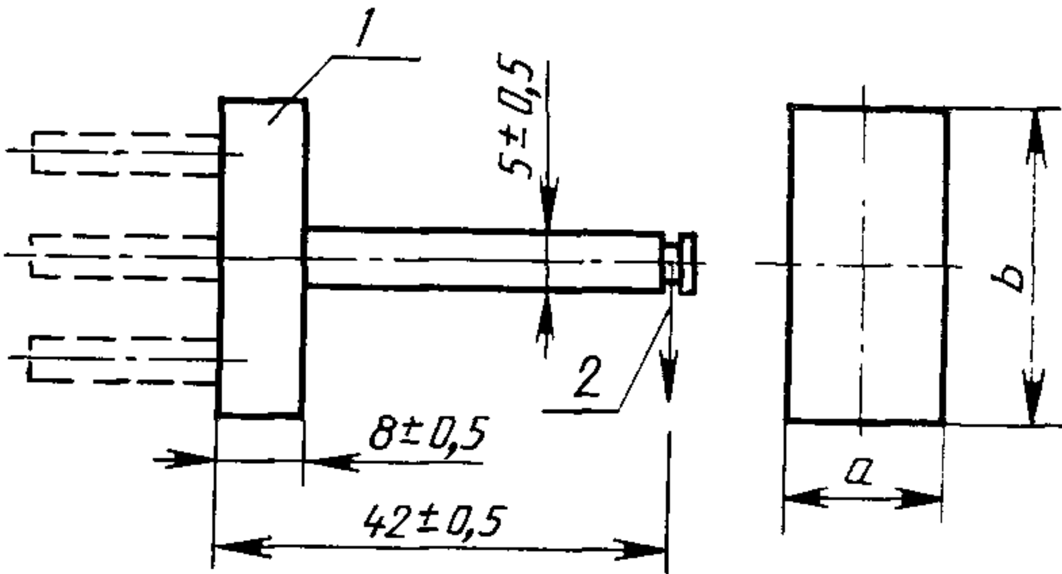
1 — материал (сталь); 2 — прилагаемая сила
