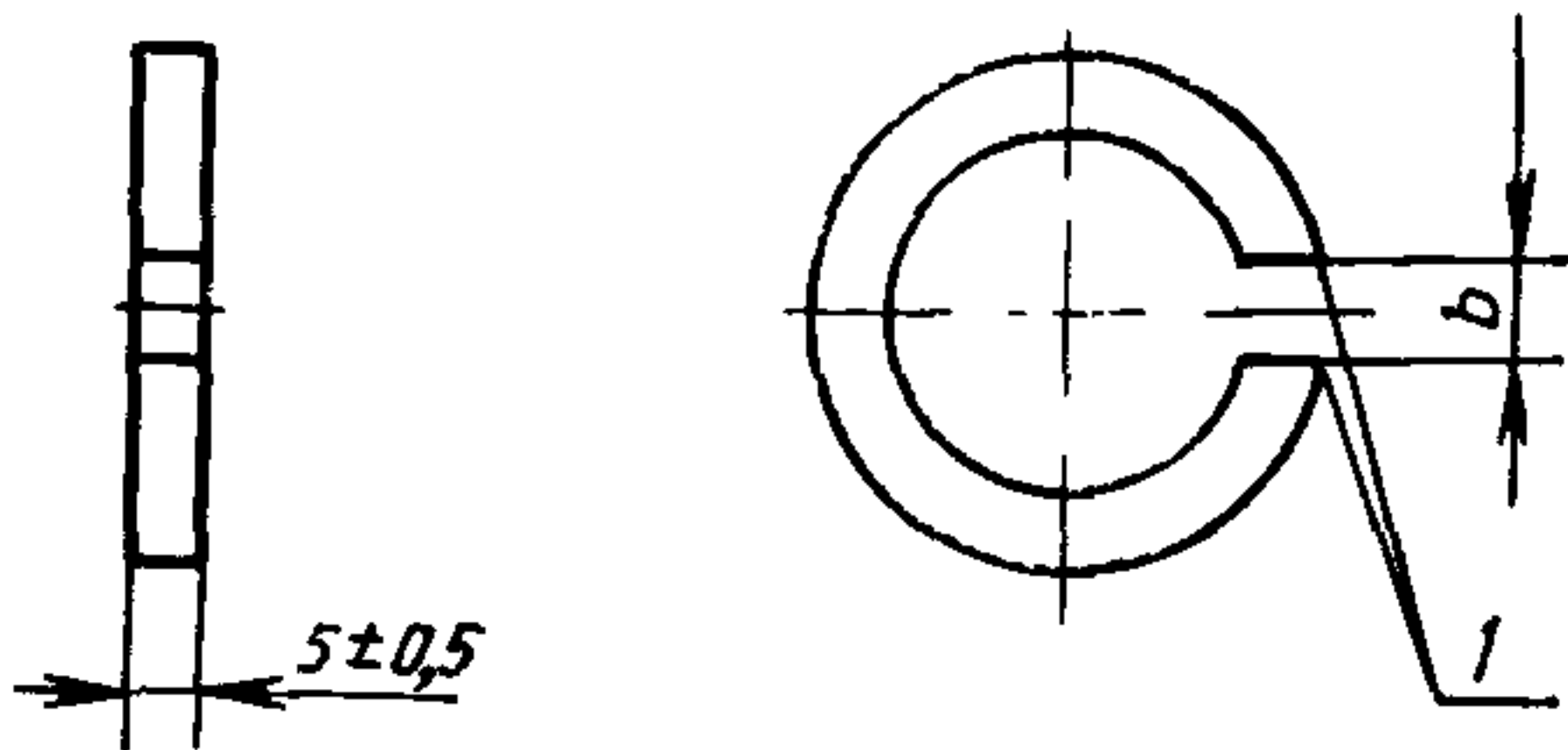
Непроходной калибр
