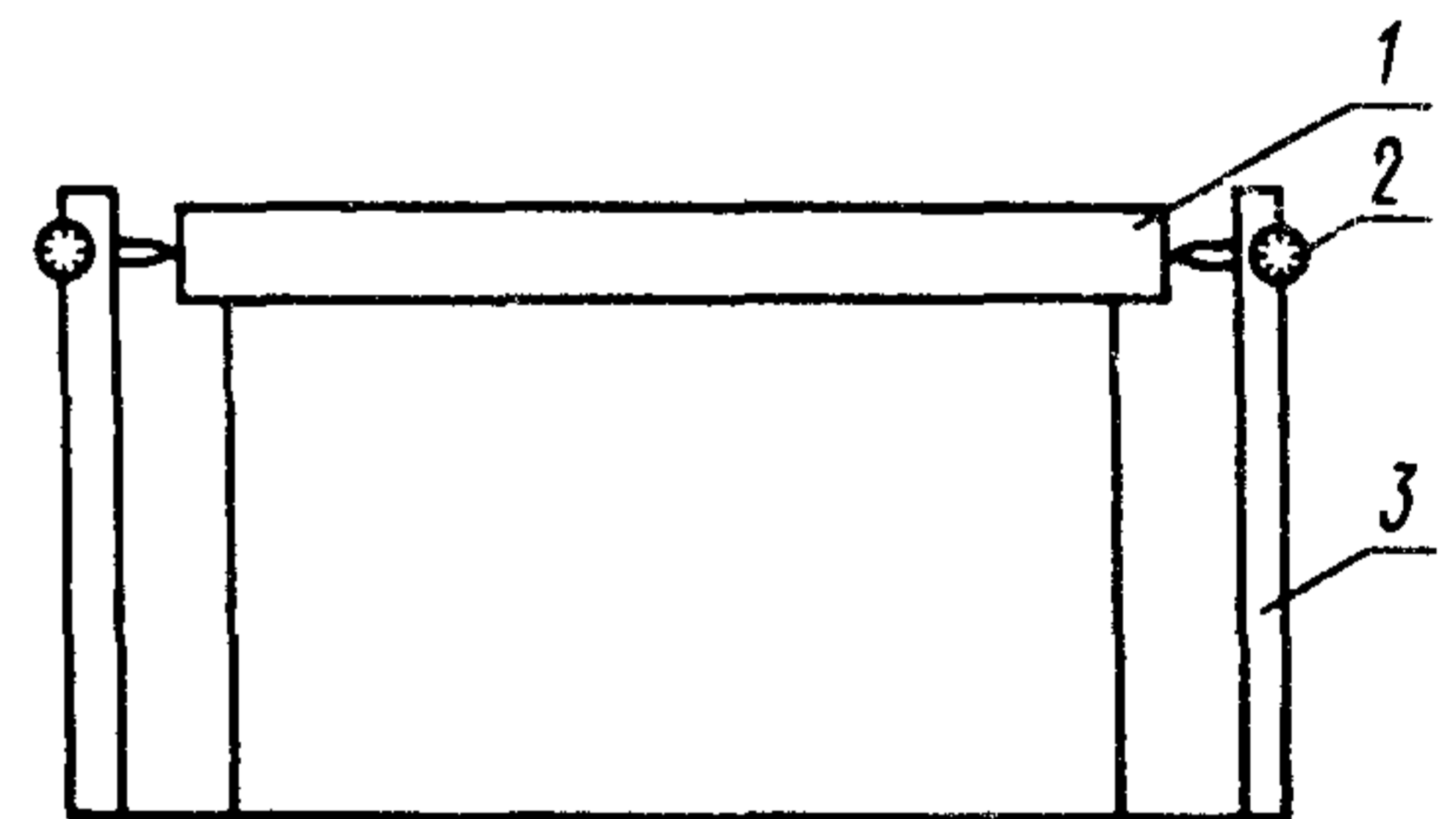
1 — моноблок; 2 — индикатор часового типа; 3 — стойка.
