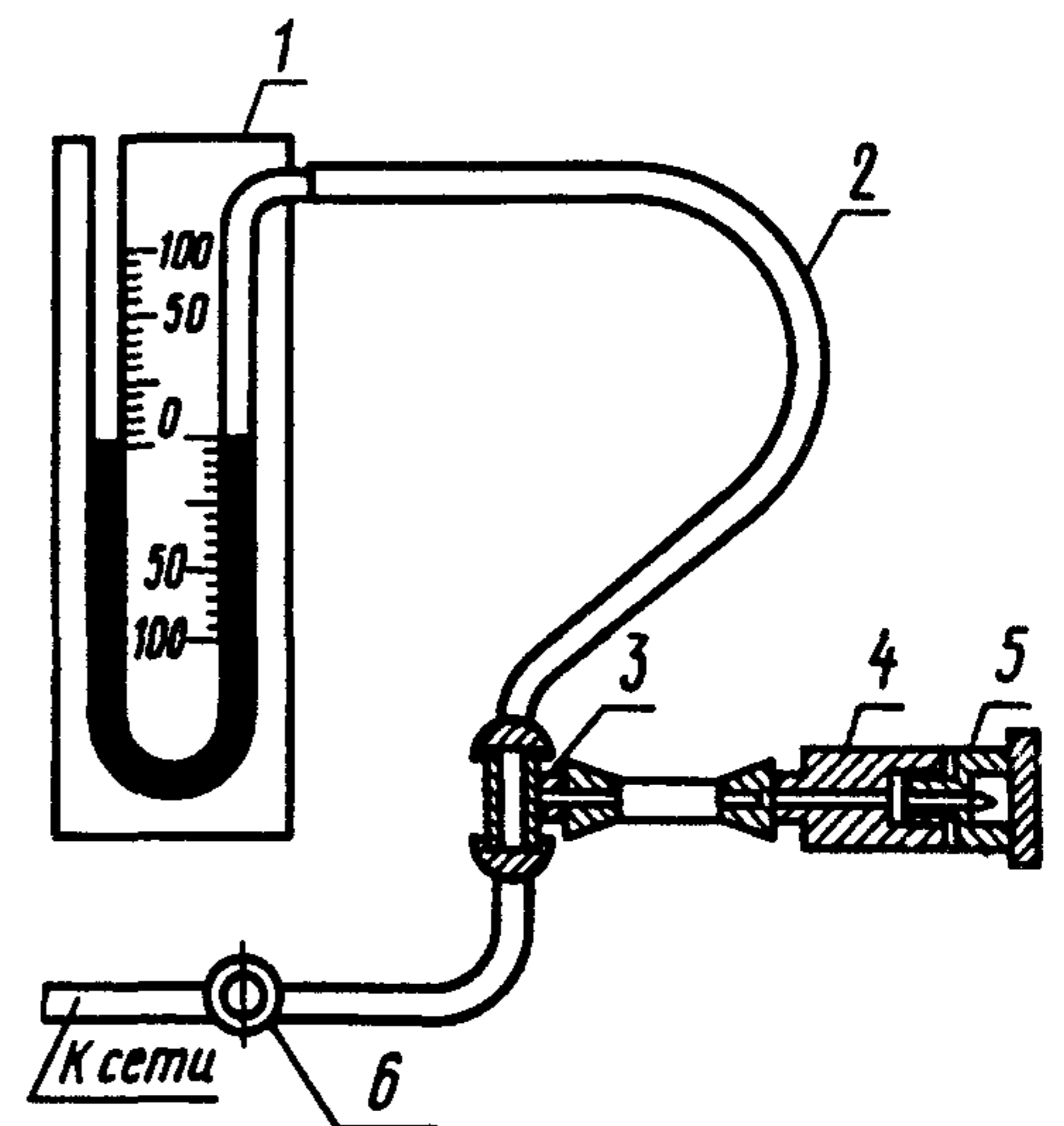
1 — ртутный манометр; 2 — шланг; 3 — тройник; 4 — патрон; 5 — пробка; 6 — кран
