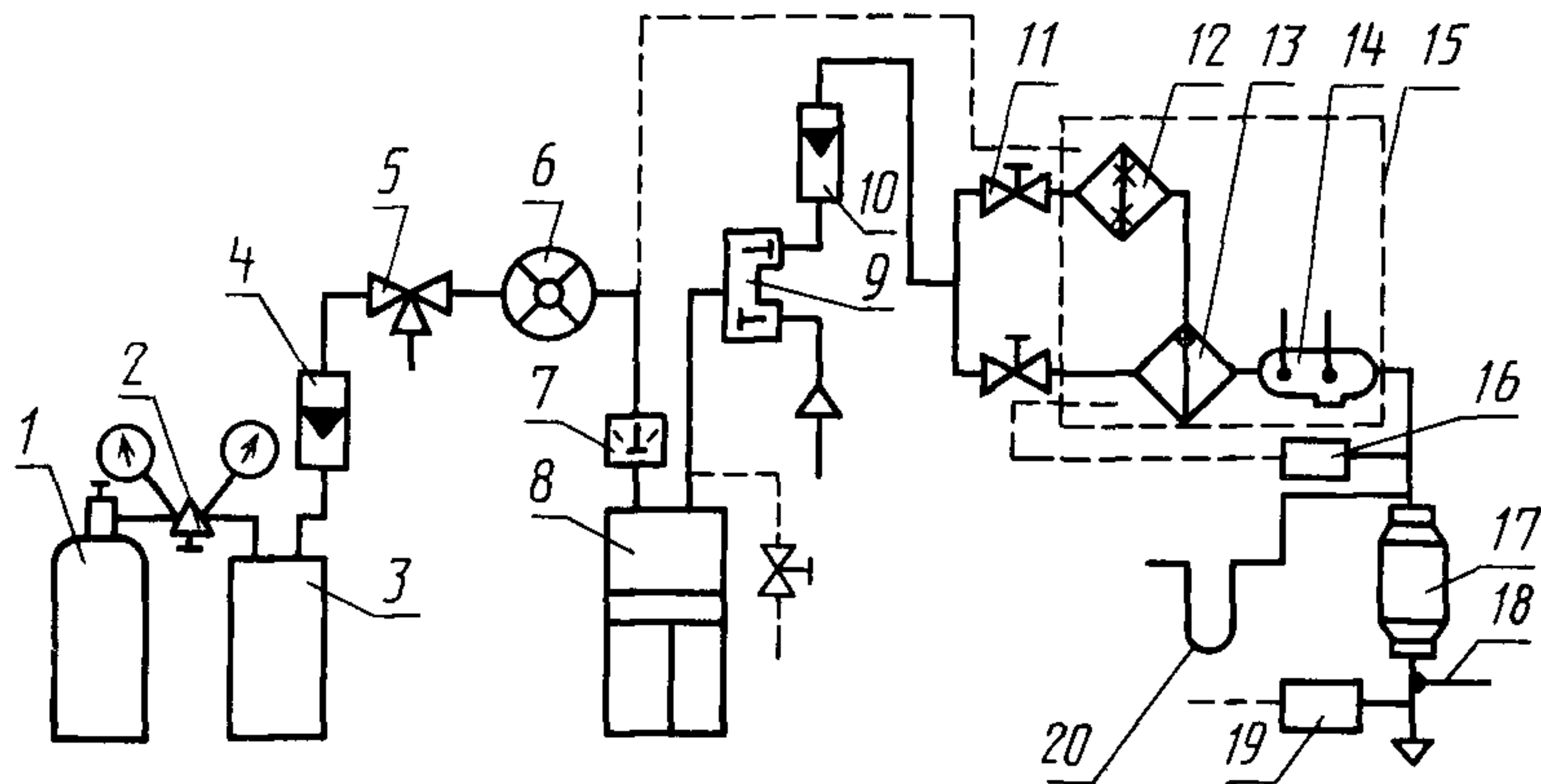
1 — баллон с двуокисью углерода; 2 — редуктор; 3 — ресивер; 4 — расходомер; 5, 11 — вентили (краны); 6 — газовый счетчик типа ГСБ-400; 7 — обратный клапан; 8 — «искусственные легкие»; 9 — клапанная коробка; 10 — индикатор расхода; 12 — увлажнитель; 13 — смеситель; 14 — психрометр; 15 — термостат-увлажнитель; 16, 19 — газоанализаторы; 17 — патрон; 18 — термометр; 20 — мановакуумметр
