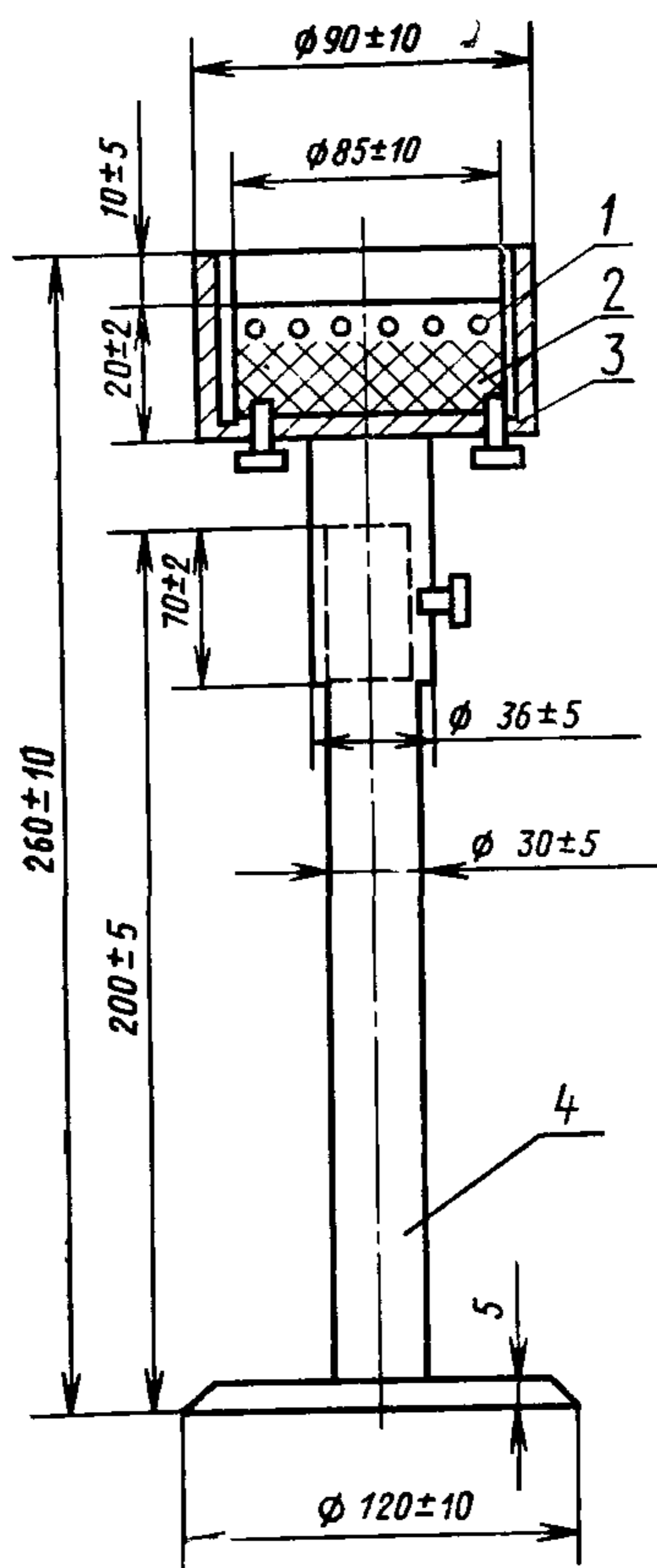
Колбонагреватель
