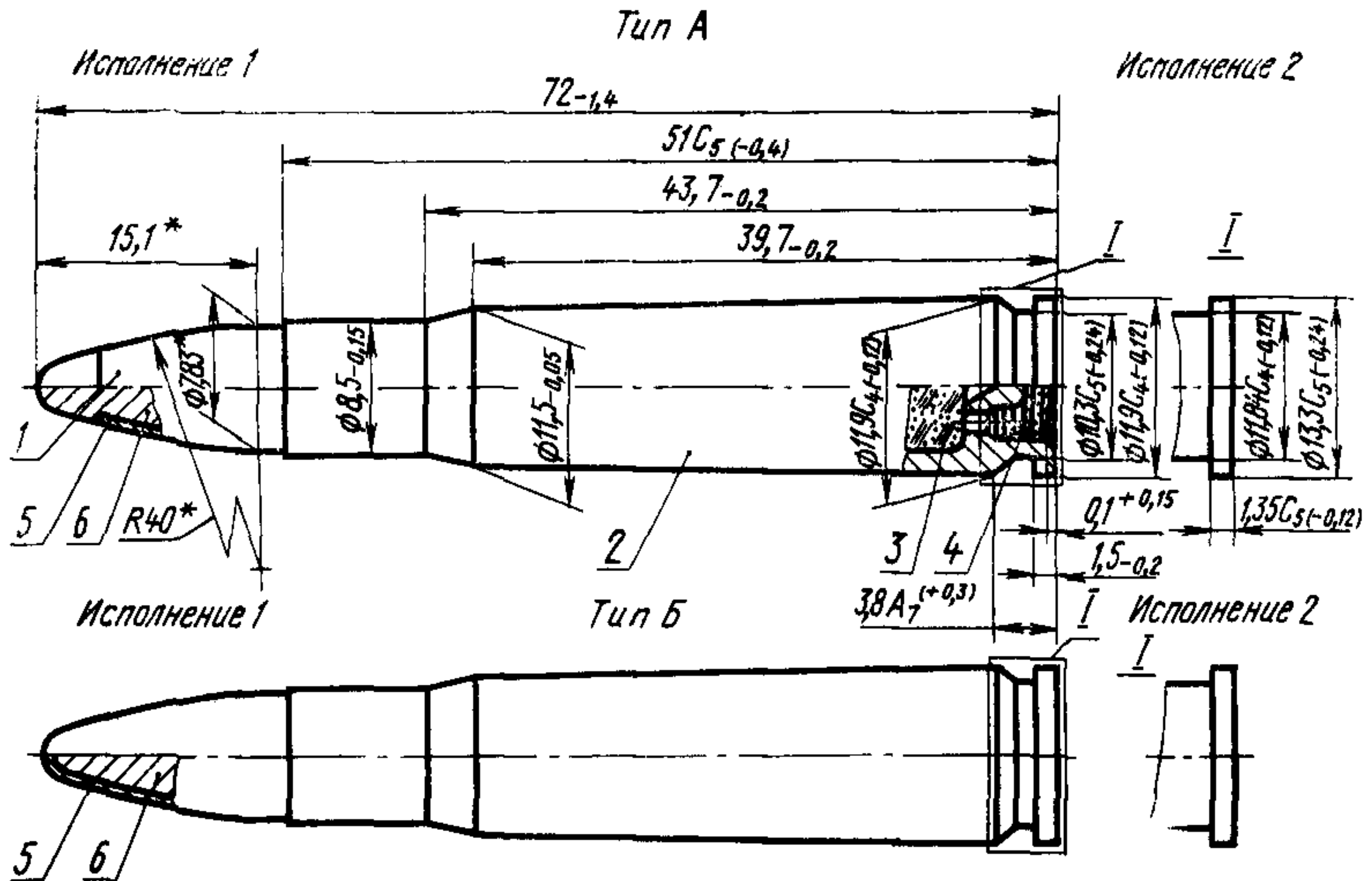
1—пуля; 2—гильза; 3—порох; 4—капсюль; 5—оболочка; 6—сердечник
