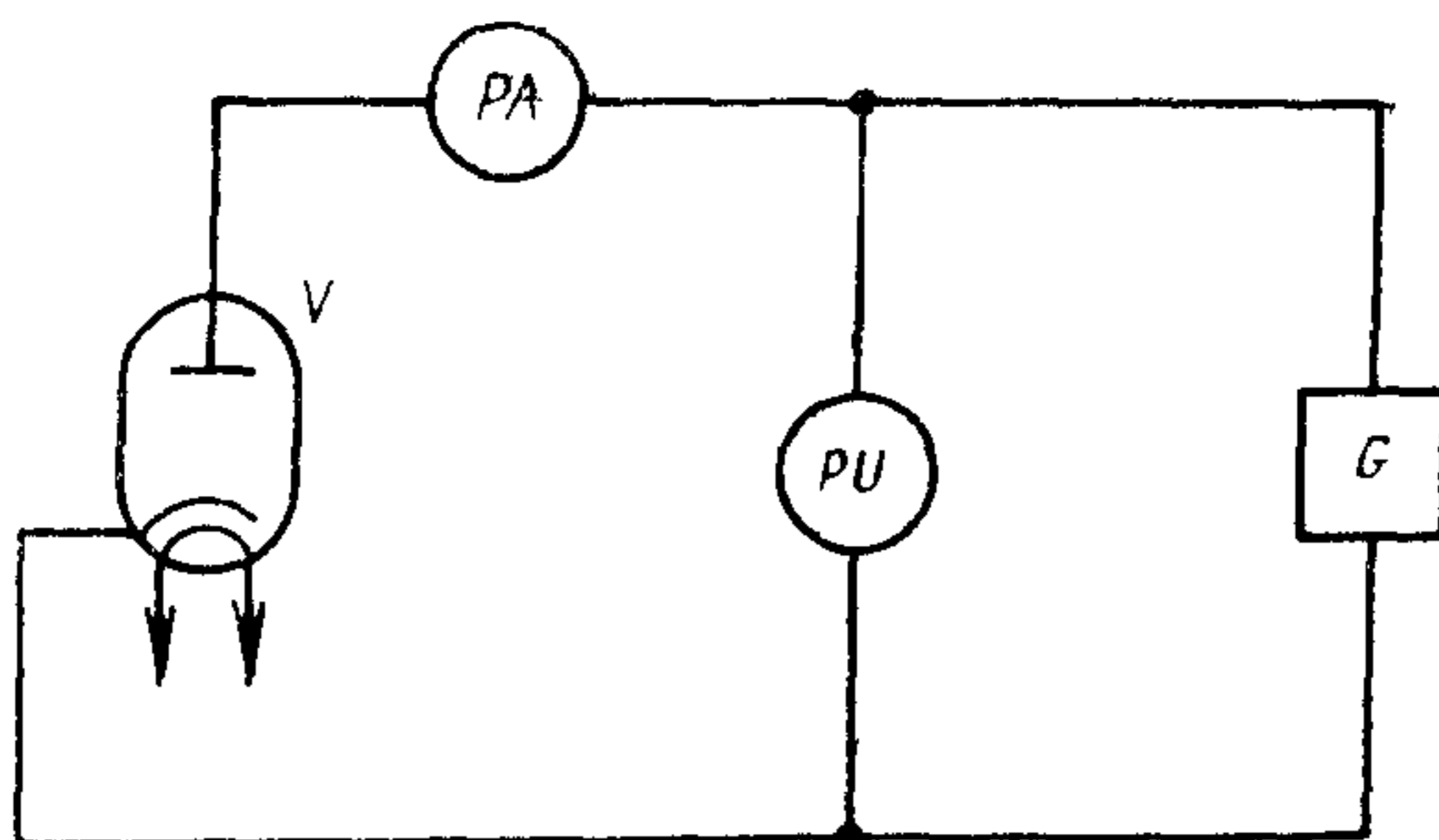
G —генератор постоянного тока; РА —миллиамперметр постоянного тока; PU —вольтметр постоянного тока; V —испытываемый кенотрон.
