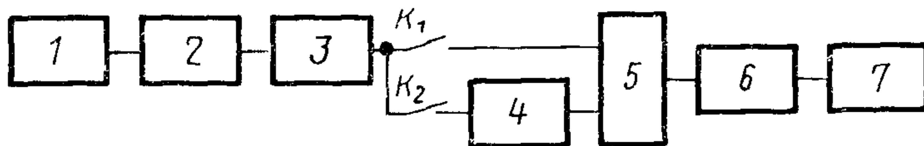
1—приемник; 2—формирователь; 3—дифференцирующая цепь; 4—инвертор; 5—схема совпадения; 6—ждуший мультивибратор с регулировкой длительности в зависимости от скорости; 7—осциллограф
