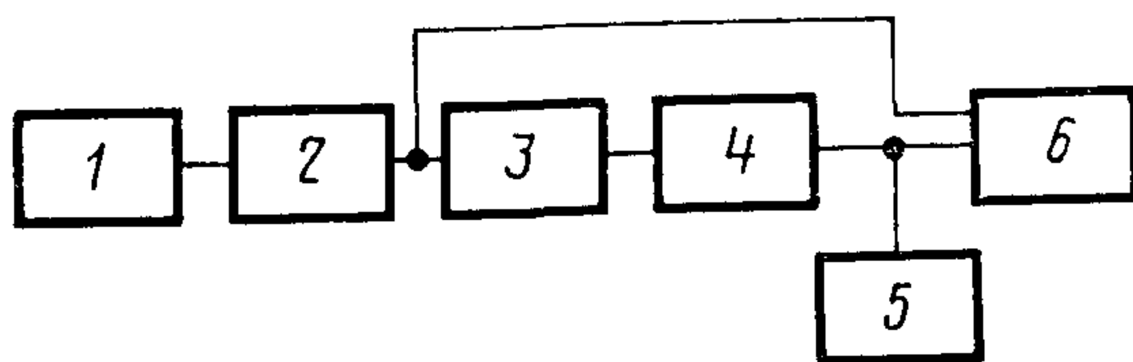
1—генератор НЧ, 2—датчик испытательных сигналов; 3—генератор сигналов ВЧ, 4—приемник; 5—эквивалент нагрузки, 6—осциллограф
