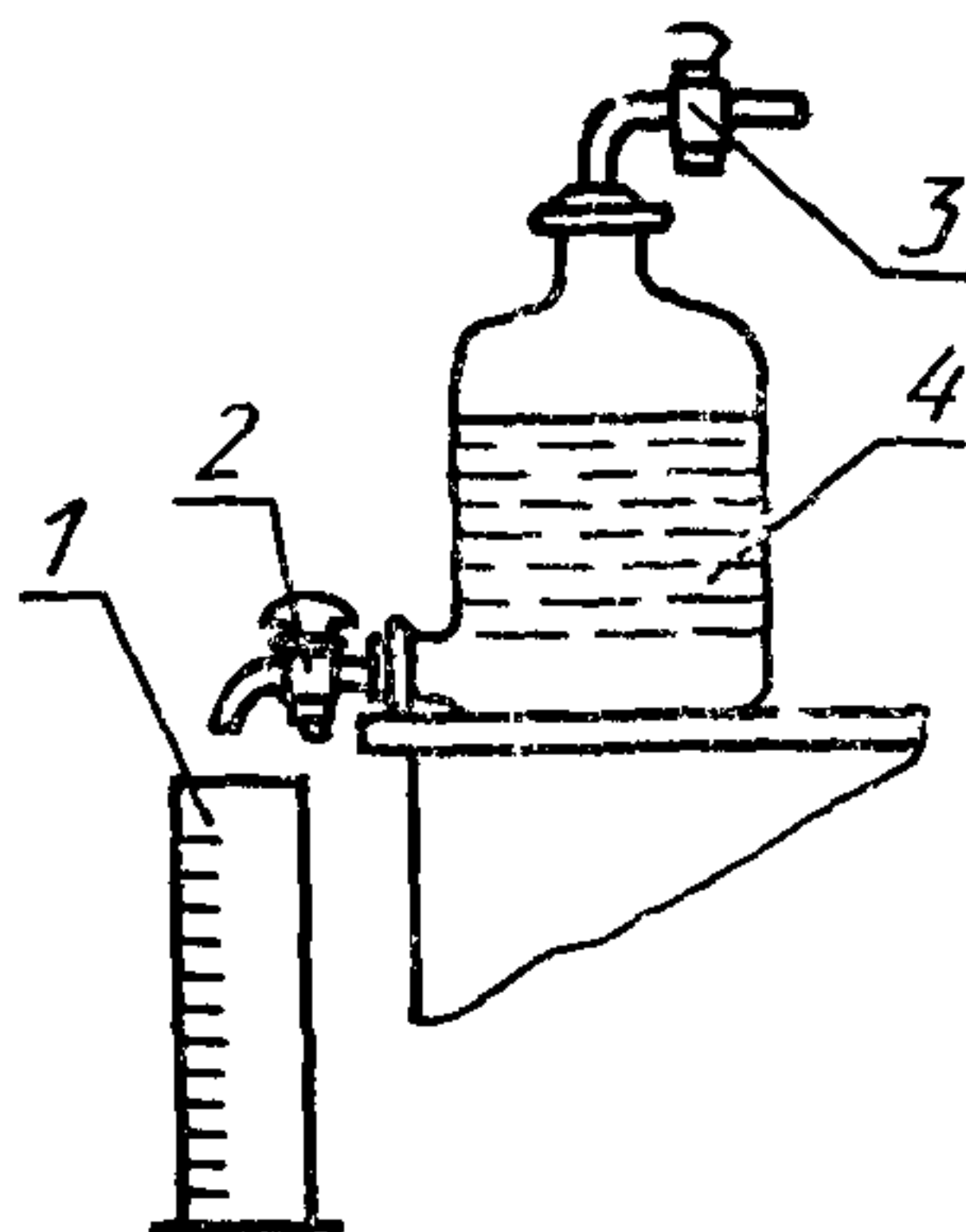
Аспиратор с измерительным цилиндром
