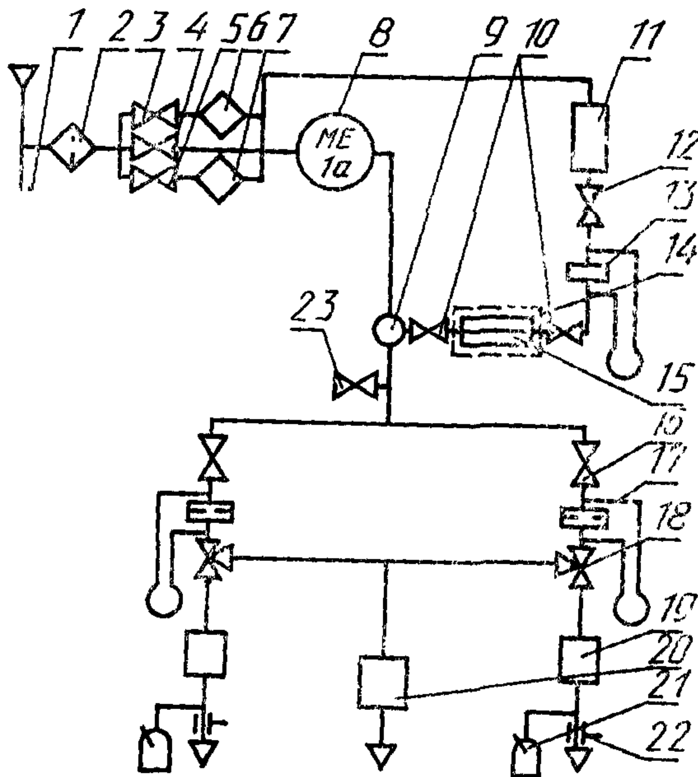
Схема динамической установки
