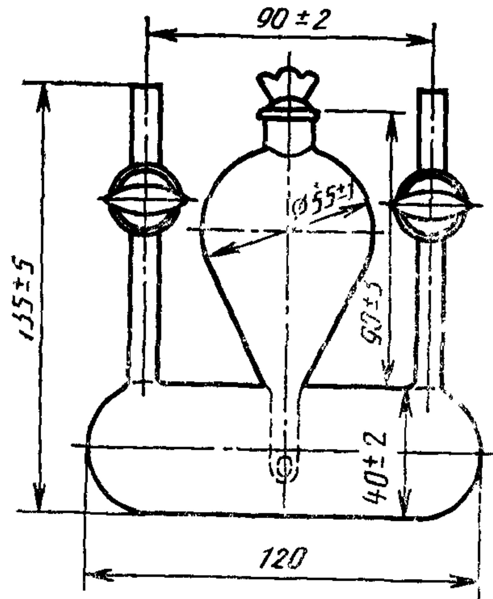
Испаритель («гусек»)
