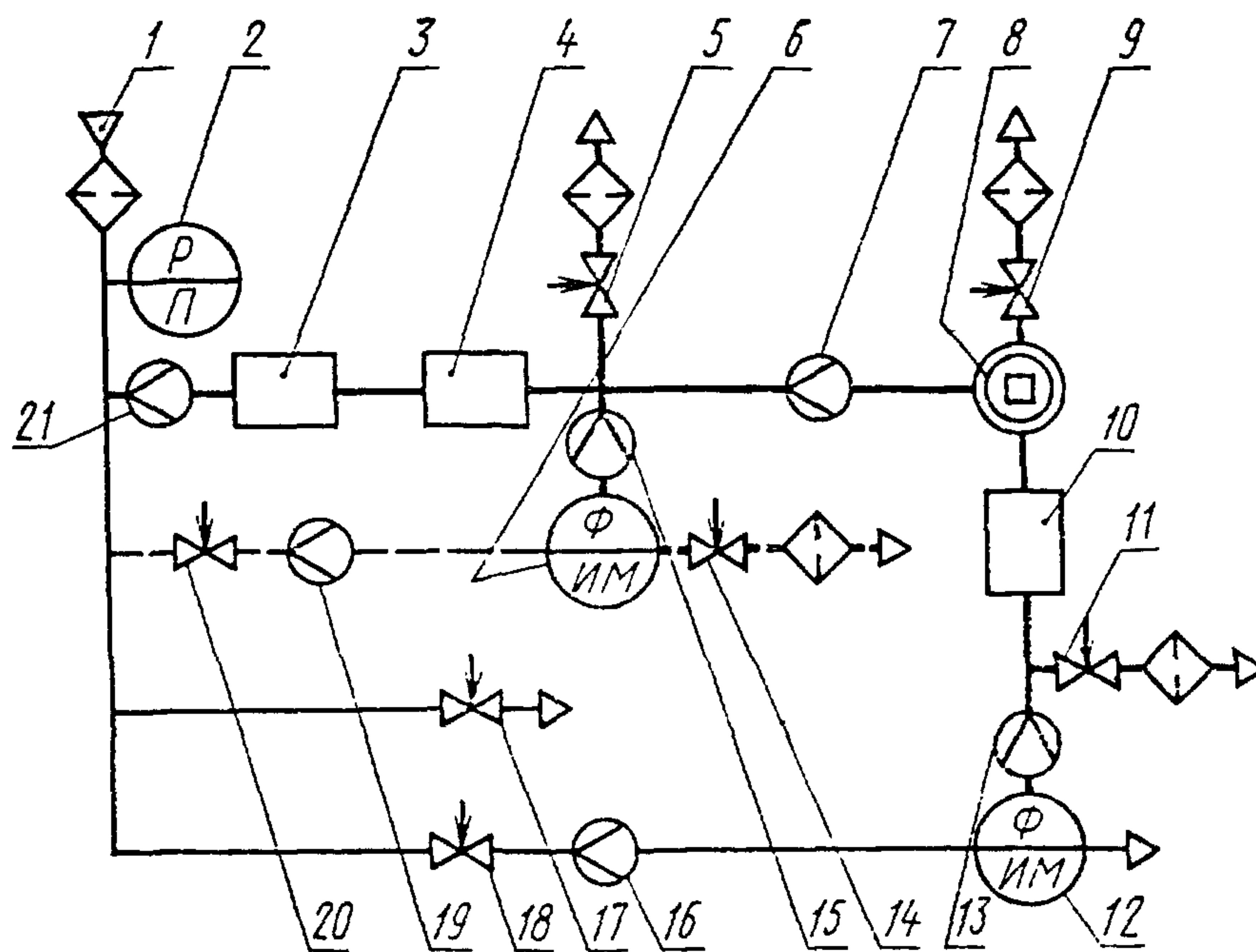
Принципиальная схема установки для контроля фильтрующих коробок по коэффициенту проскока масляного тумана
