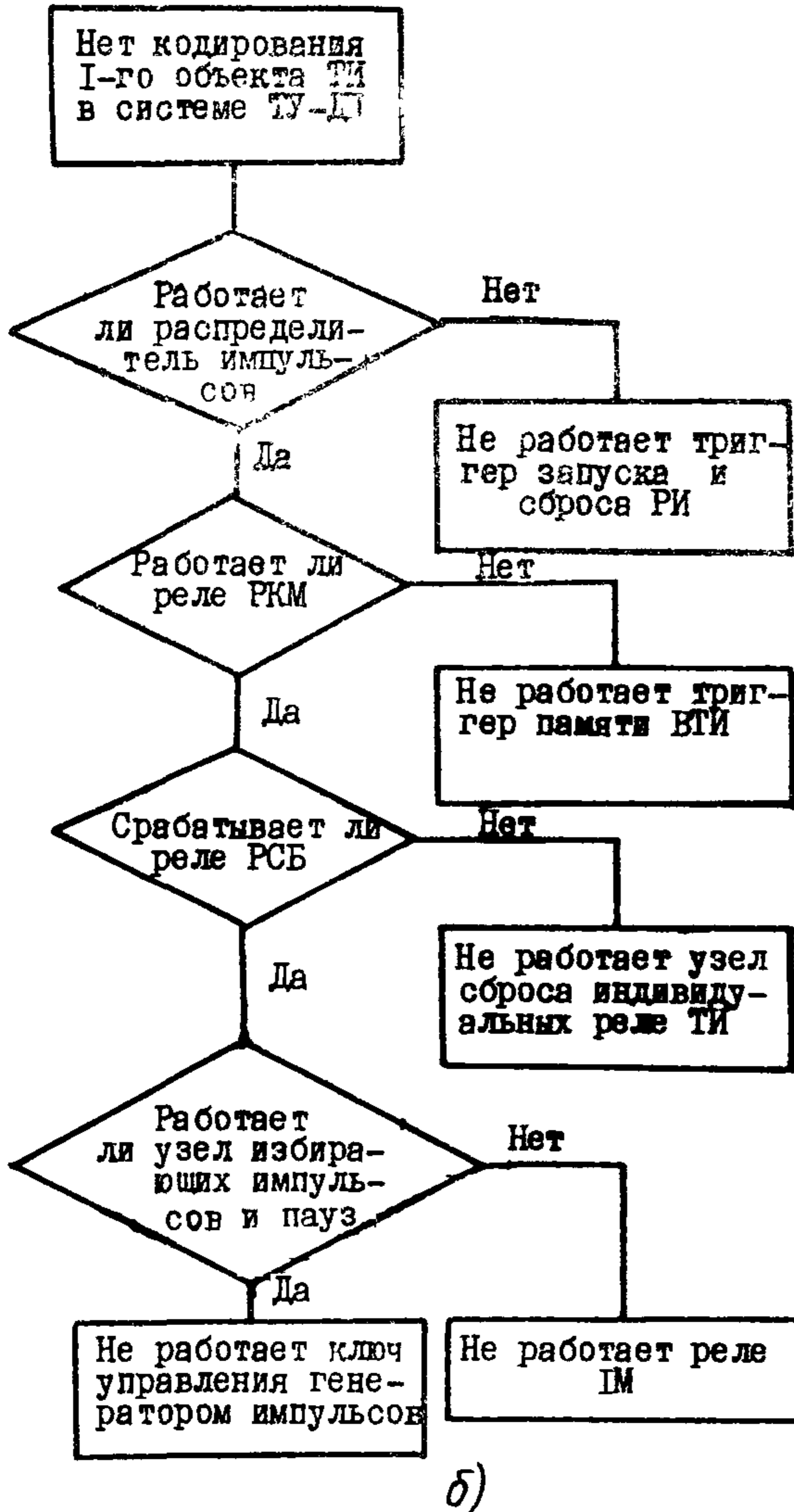
Рис.2. Диагностическая программа поиска неисправности в устройстве телемеханики ВРТО-3;
