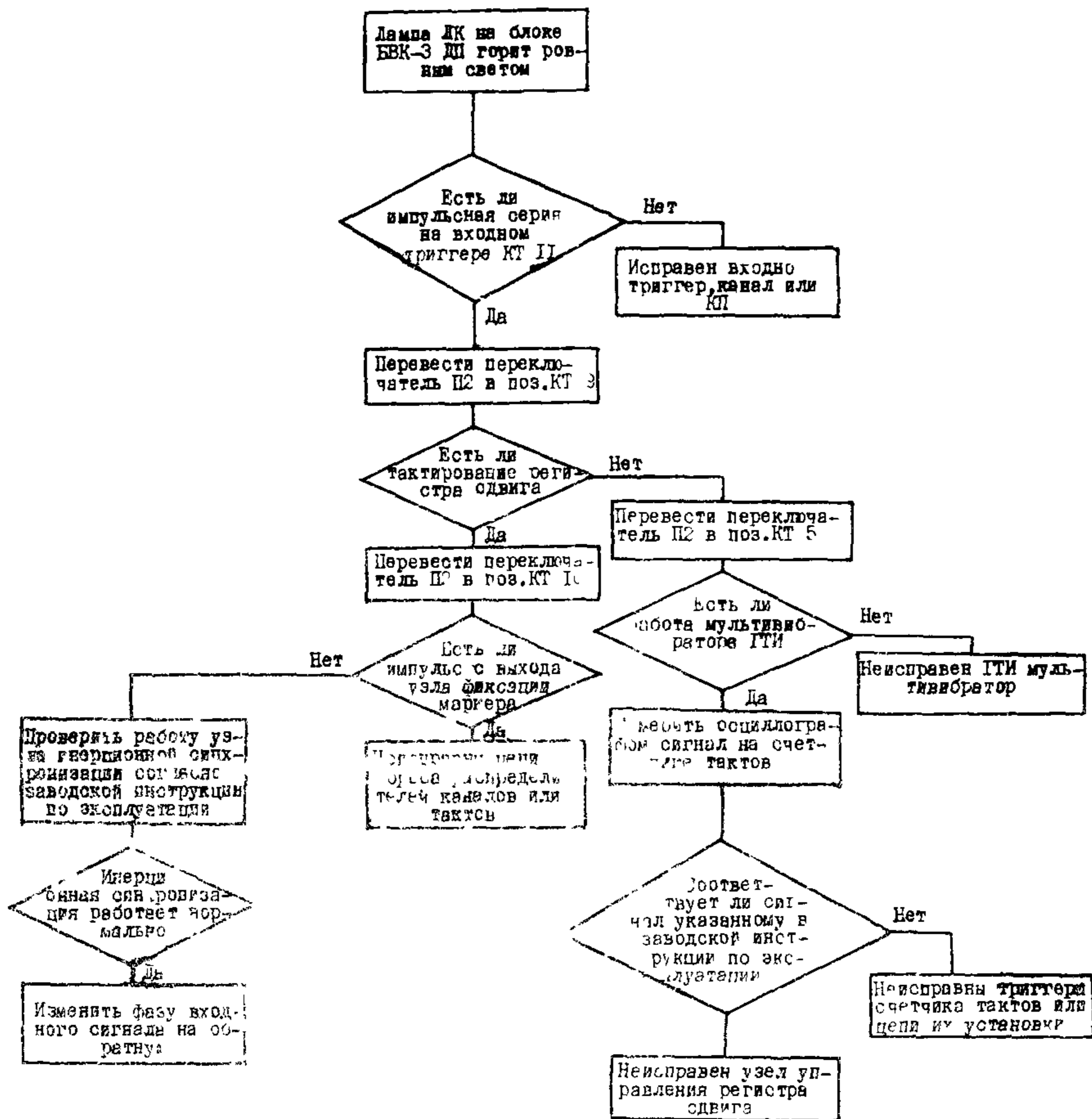
Рис. 5. Диагностическая программа поиска неисправности в устройстве телемеханики МКТ-I (полукomплект ДИ)
