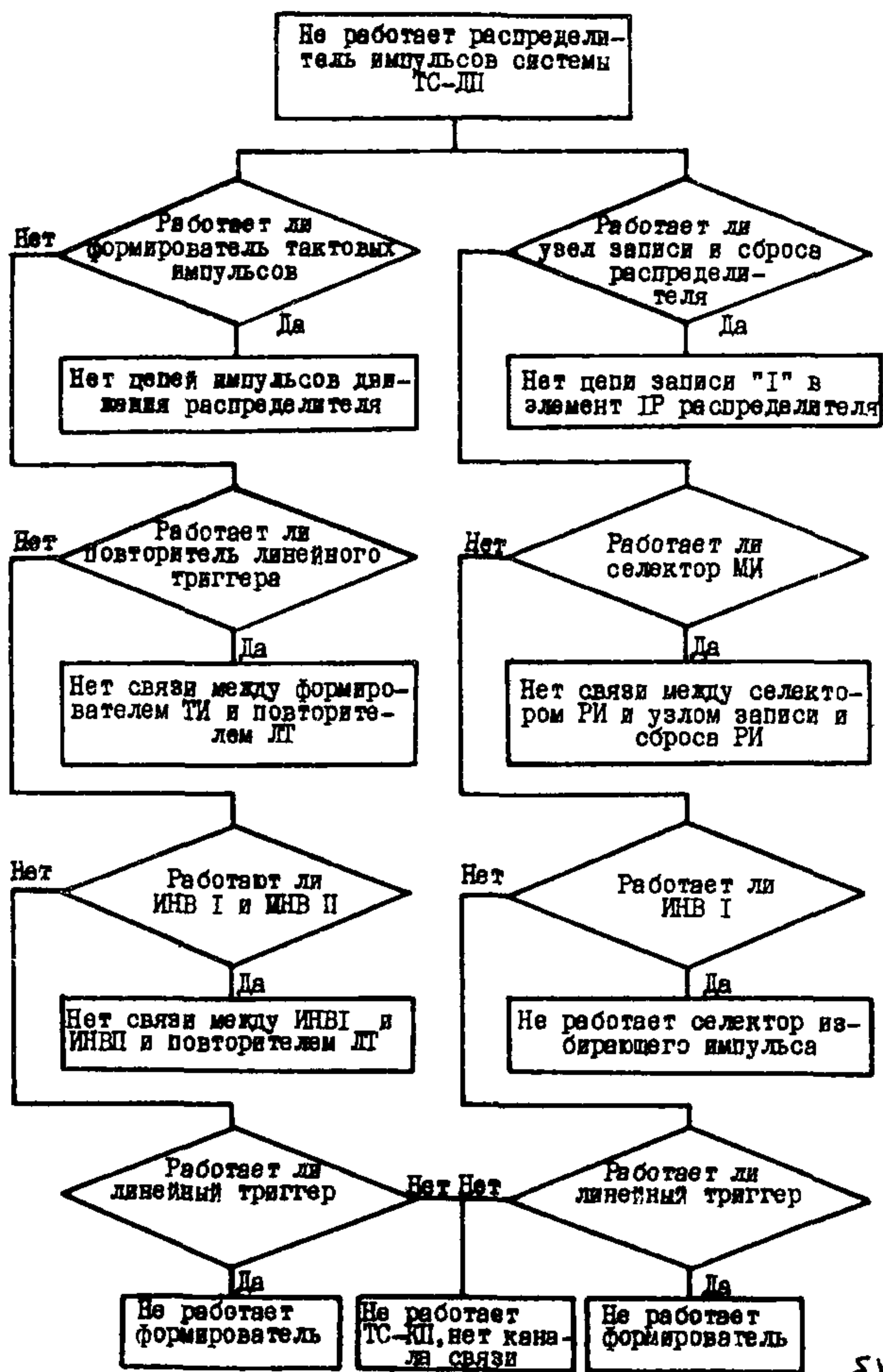
Рис. I. Диагностическая программа поиска неисправности в устройстве телемеханики ВРМ-3:
