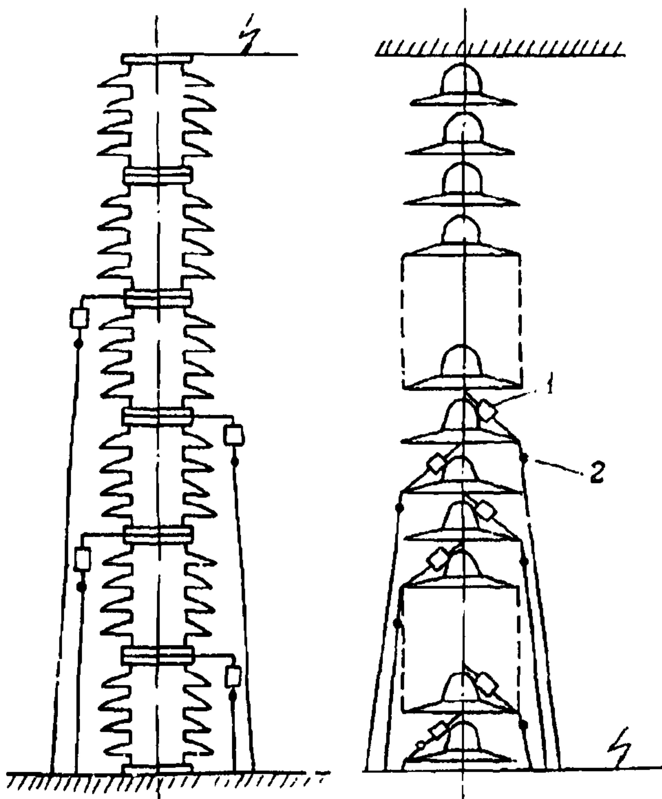
Установка регистраторов перекрытий на испытываемых объектах:
