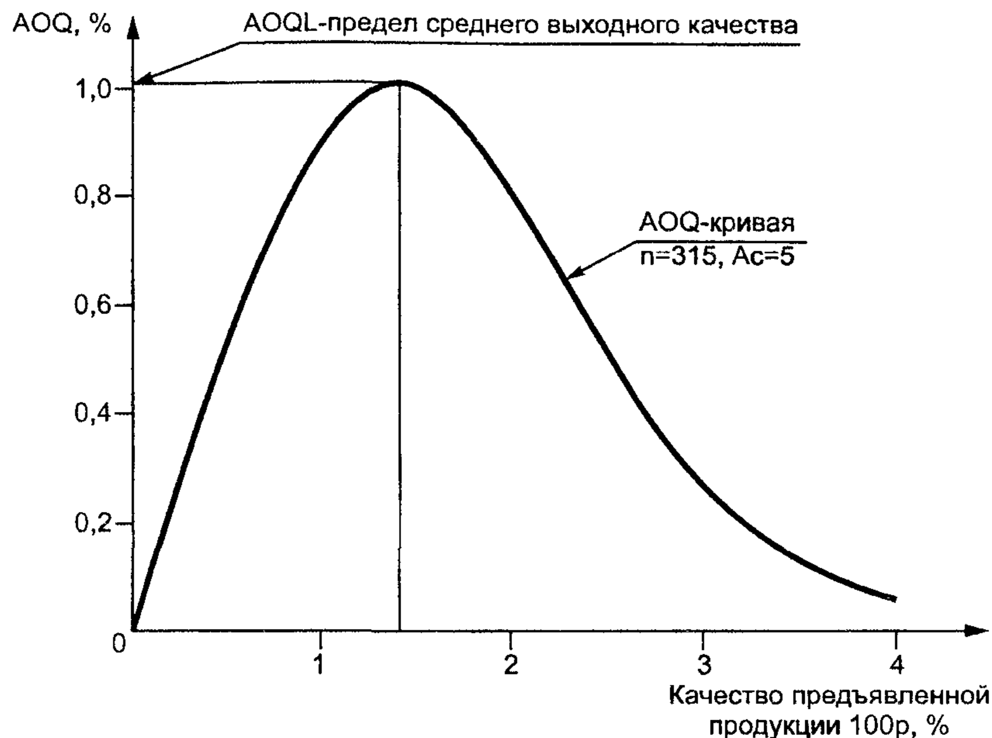
Рисунок 1 — AOQ и его предел AOQL
