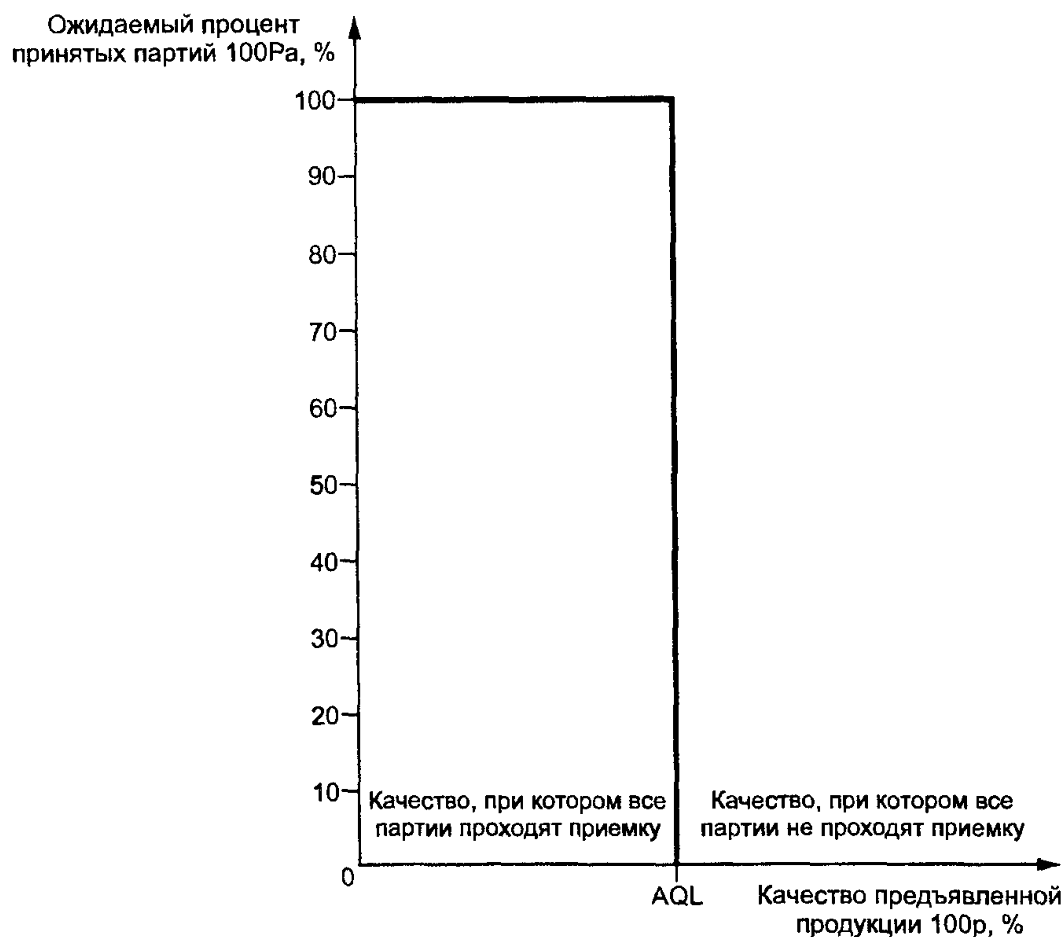
Рисунок 7 — Идеальная кривая оперативной характеристики
